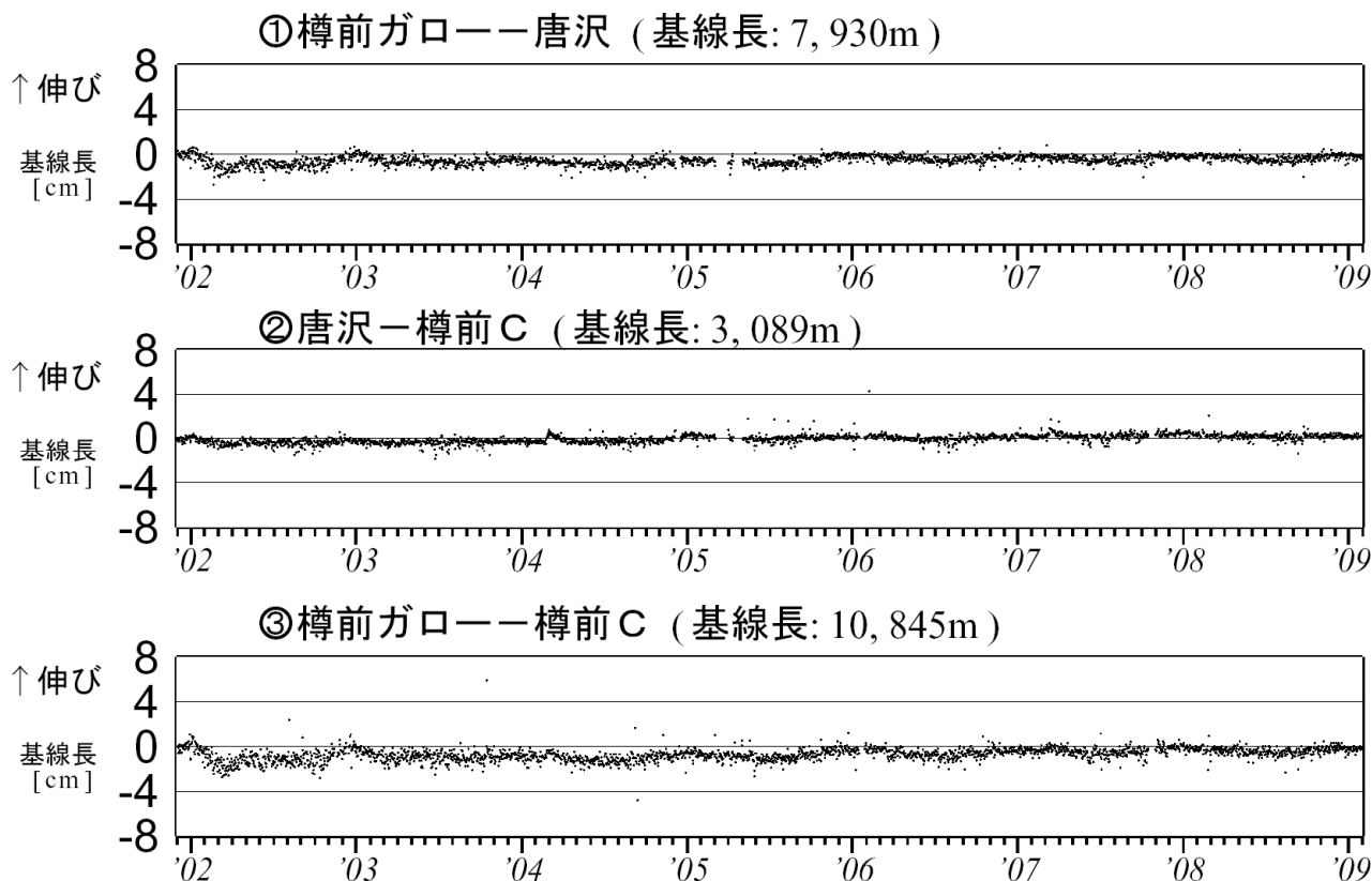
図5 樽前山 GPS 連続観測による基線長変化 (2001 年 12 月～2009 年 1 月) グラフの空白部分は欠測
