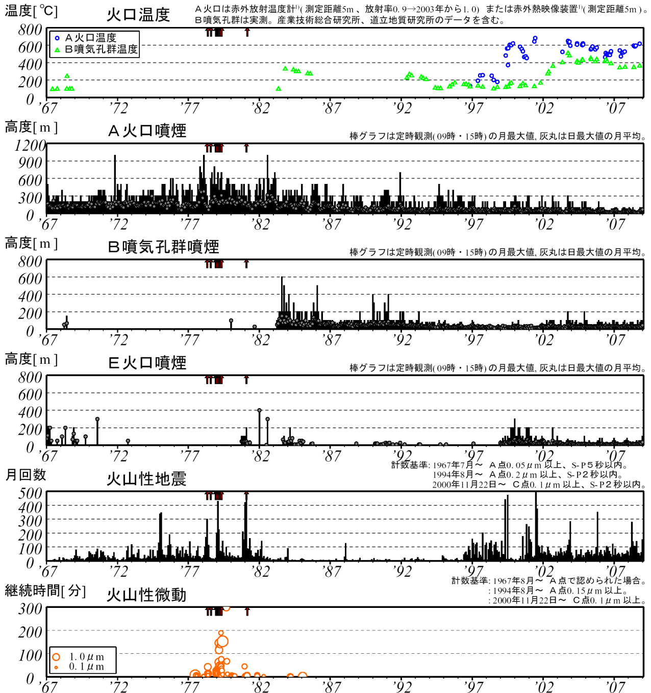
図 2※ 樽前山 長期の火山活動経過図 (1967 年 1 月～2009 年 1 月) ↑印は噴火
