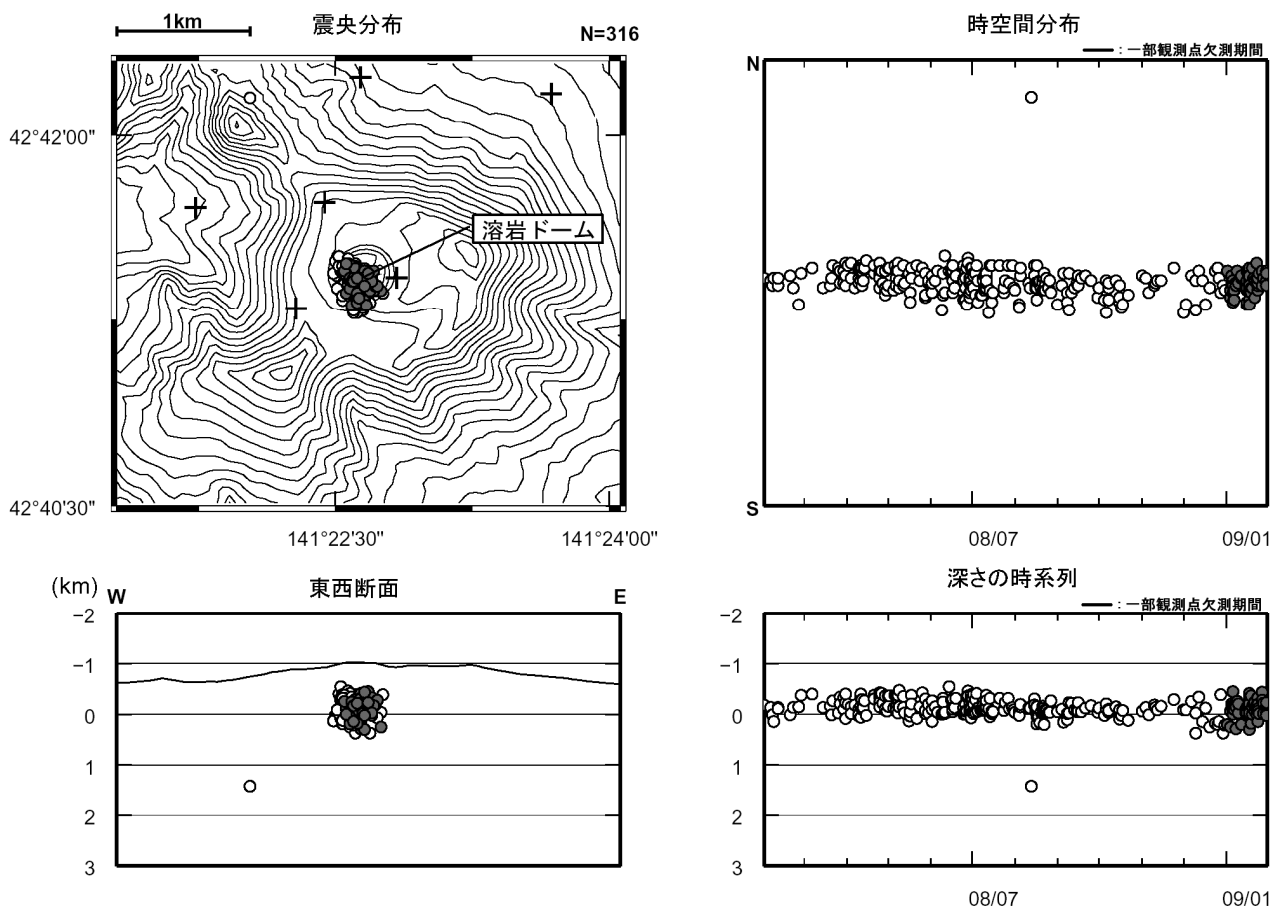
図 4※ 樽前山 震源分布図 (2008 年 2 月～2009 年 1 月、+は地震観測点)
