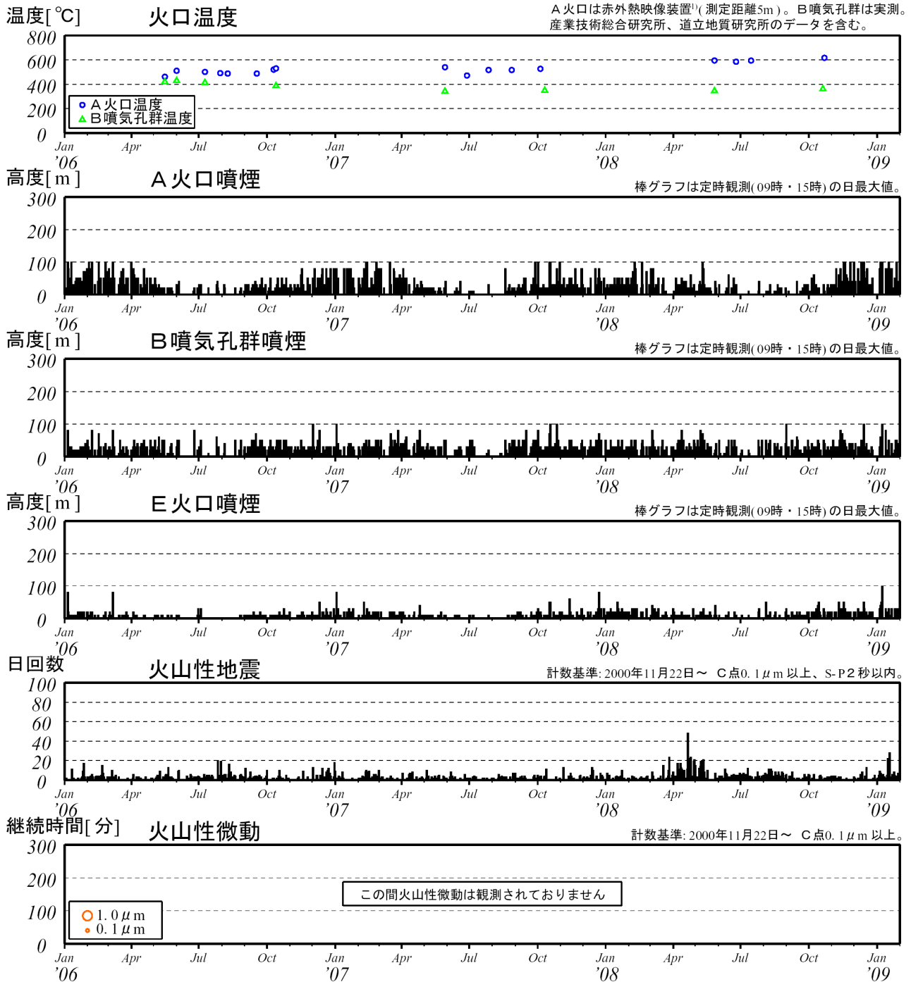
図3※ 樽前山 最近の火山活動経過図 (2006年1月～2009年1月)
