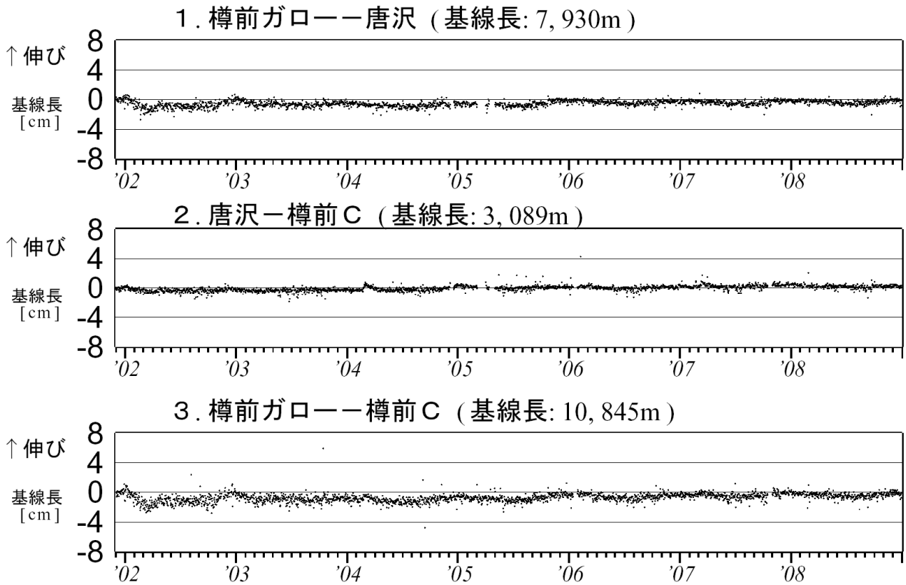
図5 樽前山 GPS 連続観測による基線長変化 (2001 年 12 月～2008 年 12 月) グラフの空白部分は欠測
