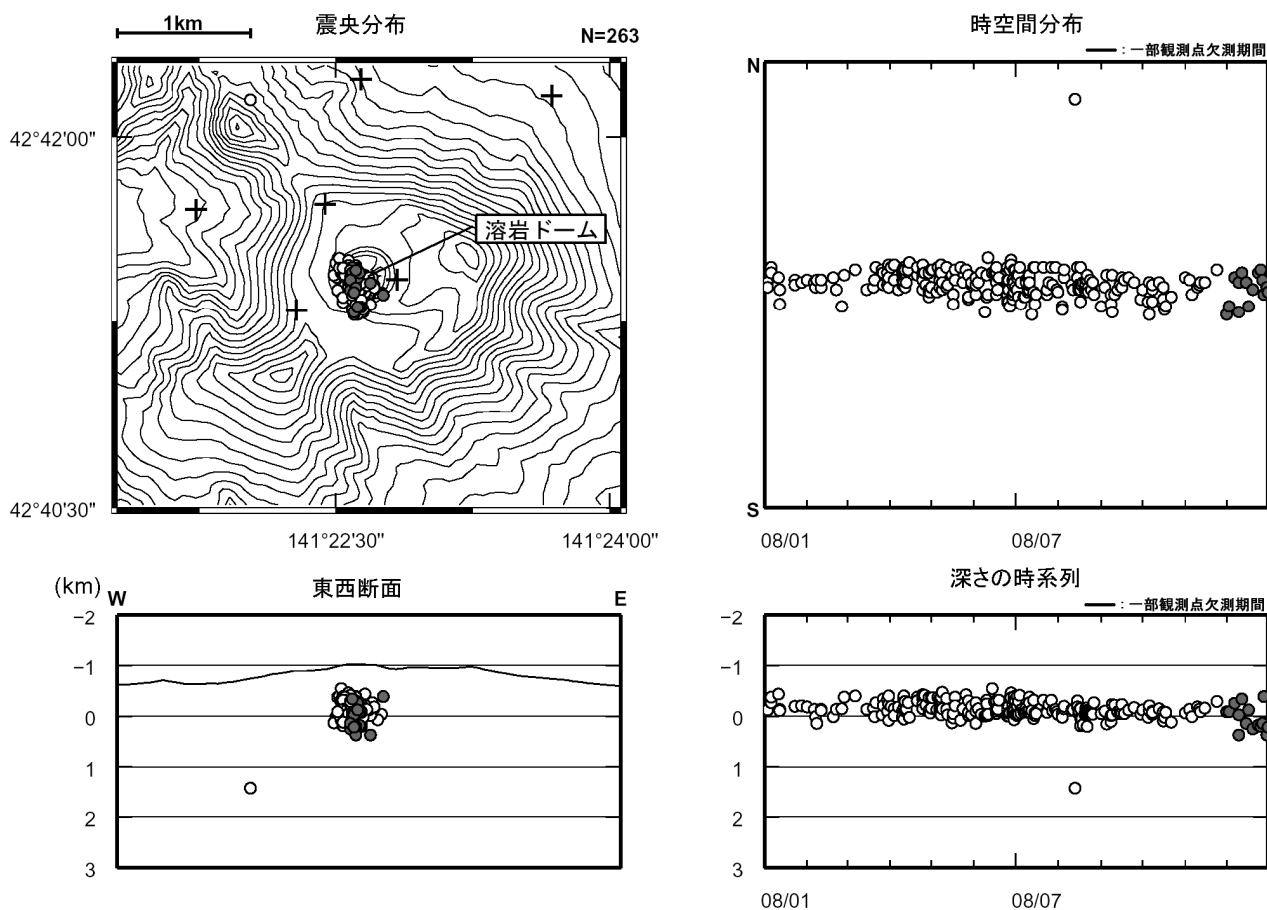
図 4※ 樽前山 震源分布図 (2008 年 1 月～2008 年 12 月、+は地震観測点)
