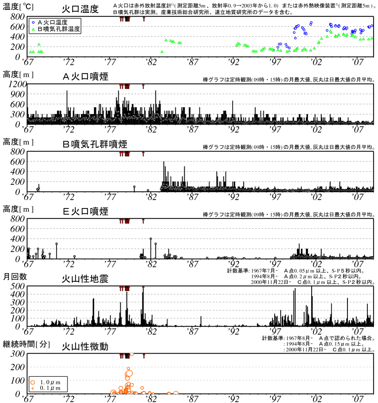
図 2※ 樽前山 長期の火山活動経過図 (1967 年 1 月～2008 年 12 月) ↑印は噴火
