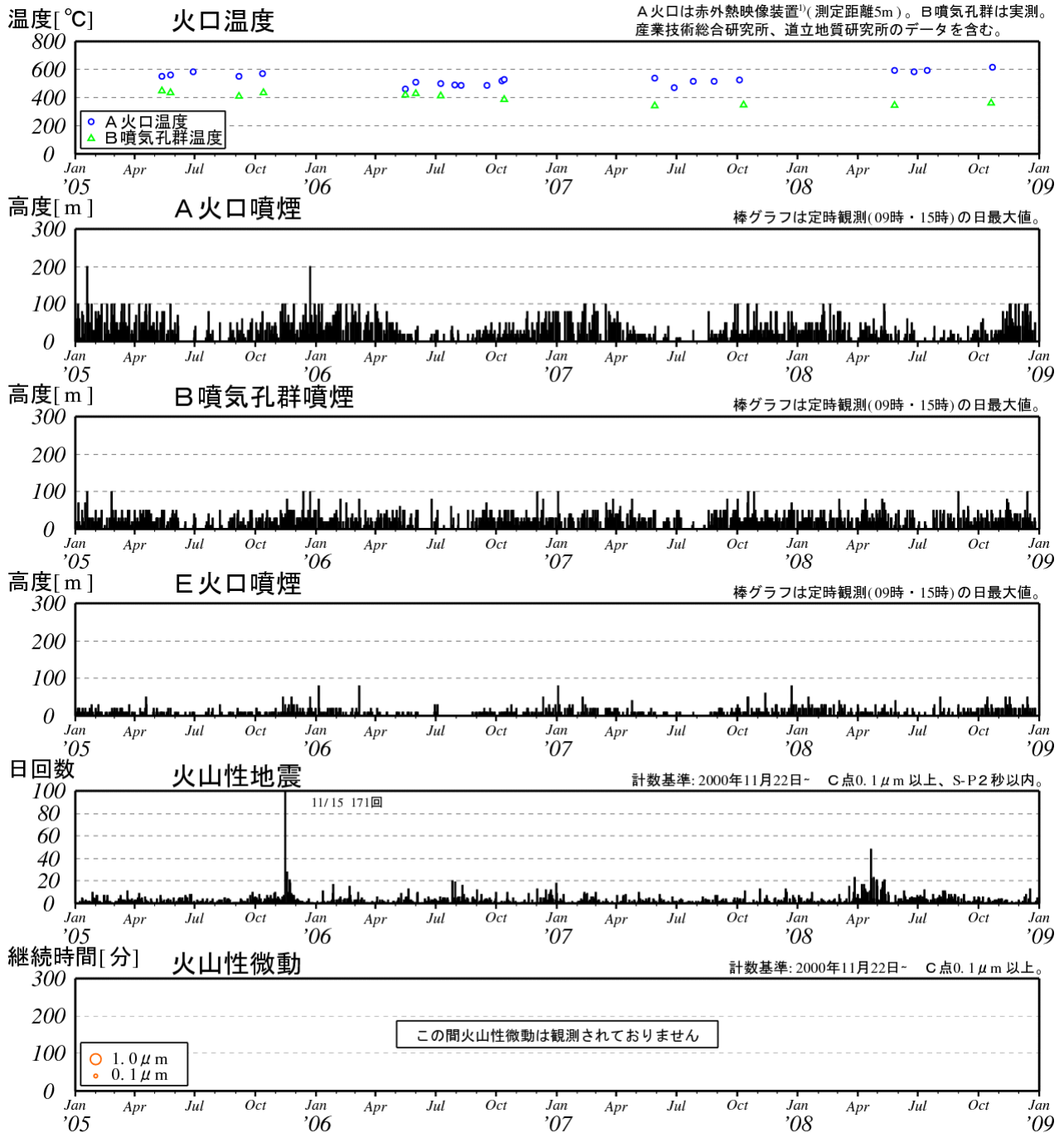
図3※ 樽前山 最近の火山活動経過図 (2005年1月~2008年12月)
