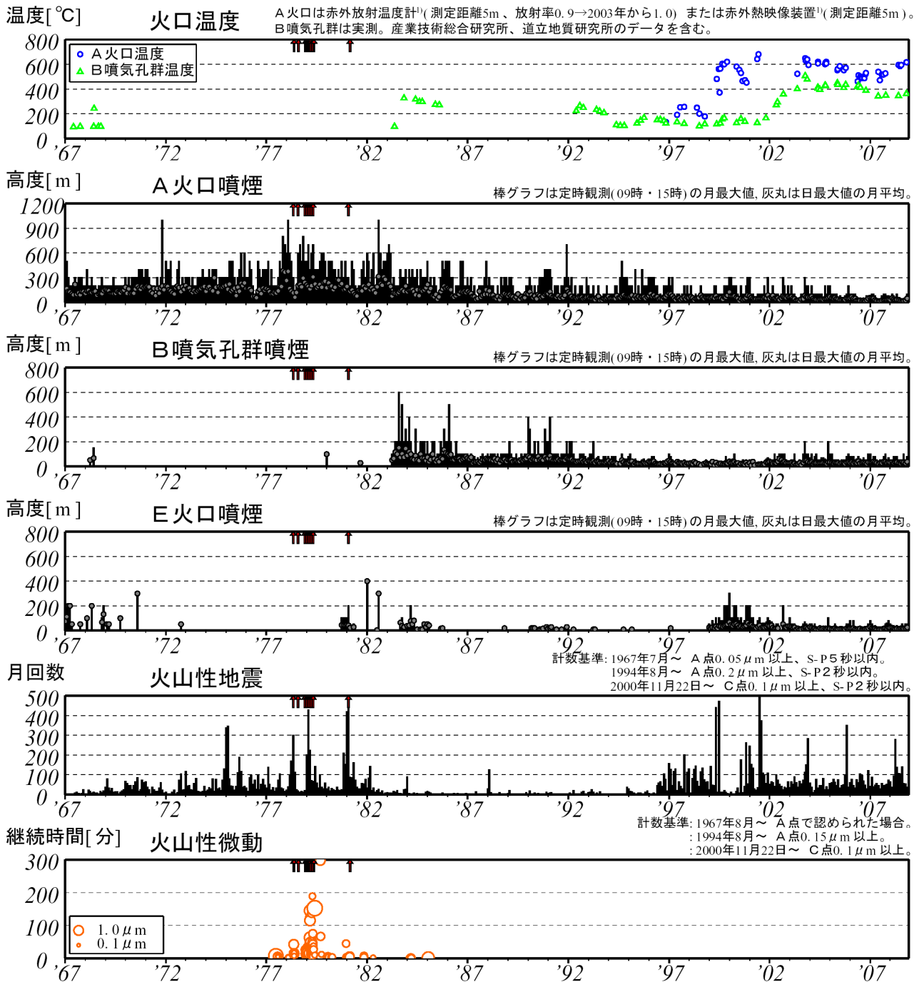
図 2※ 樽前山 長期の火山活動経過図 (1967 年 1 月～2008 年 11 月) ↑印は噴火
