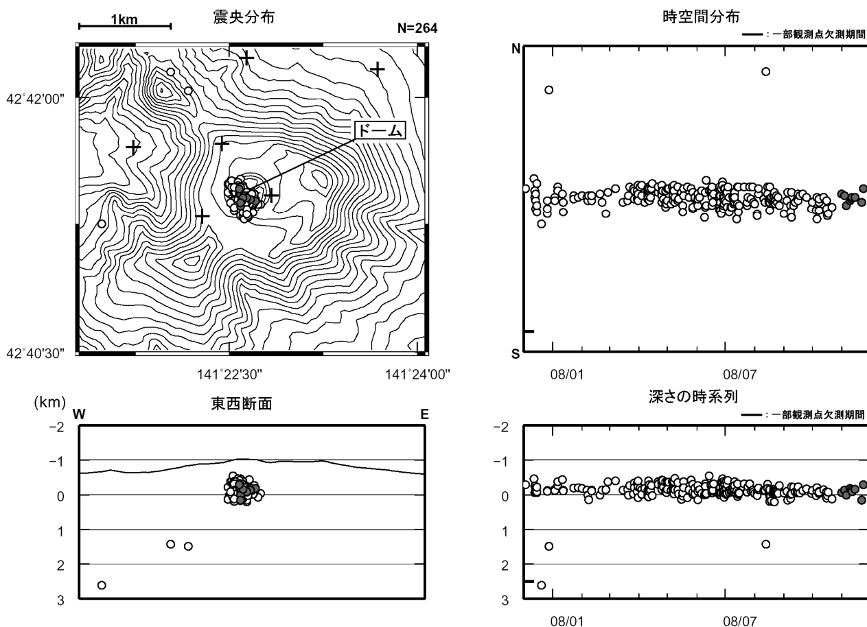
図 4※ 樽前山 震源分布図 (2007 年 12 月~2008 年 11 月、+は地震観測点)
