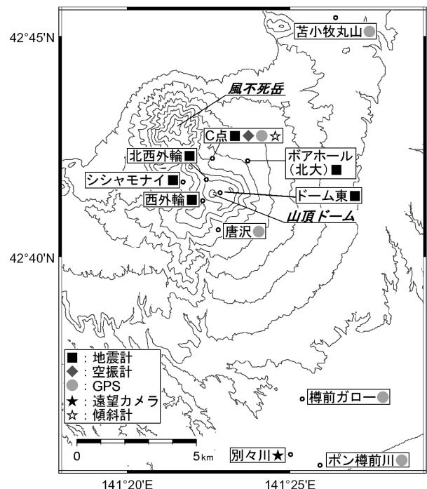
図 1 樽前山 火山観測点配置図
