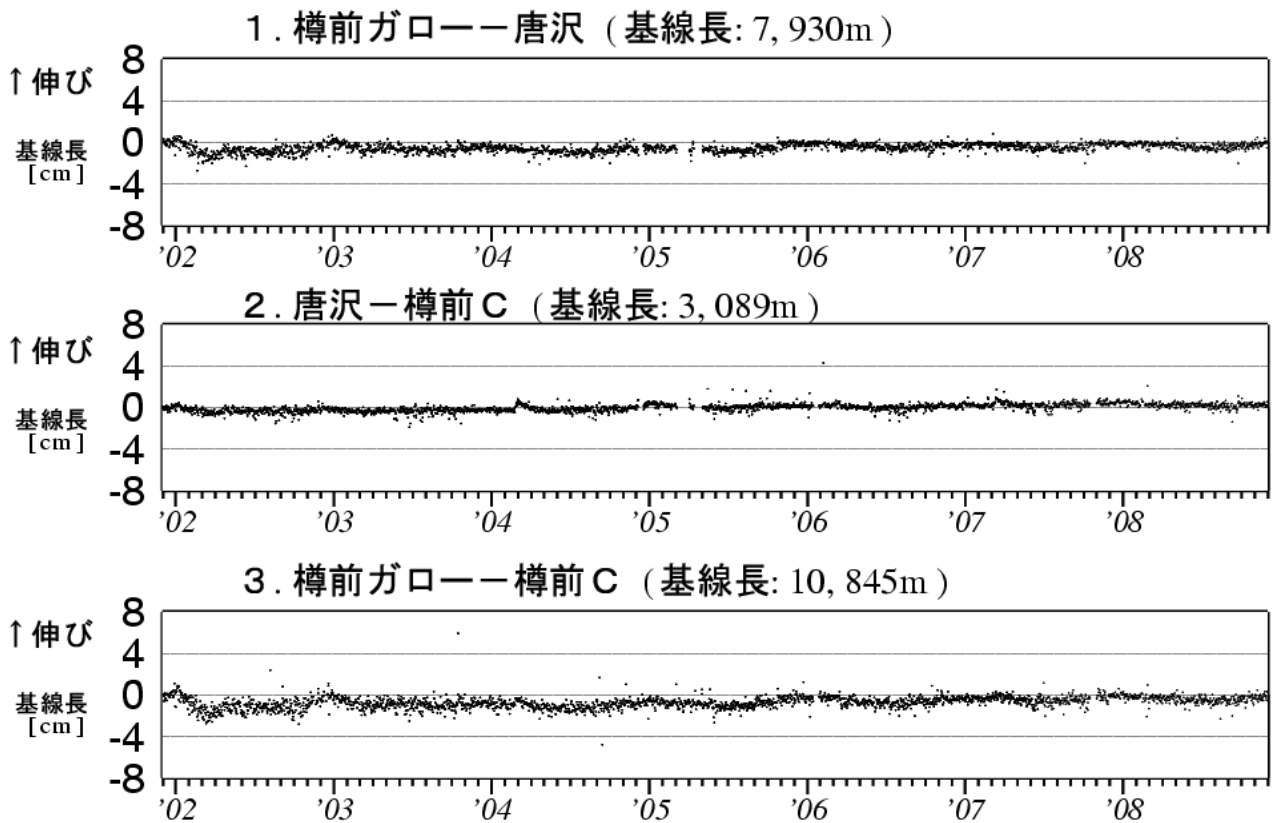
図5 樽前山 GPS 連続観測による基線長変化 (2001 年 12 月~2008 年 11 月)
