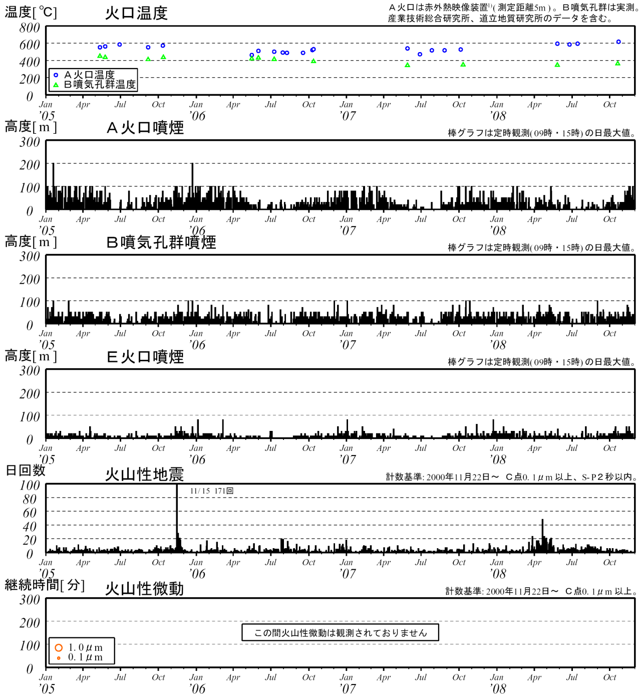
図 3※ 樽前山 最近の火山活動経過図 (2005 年 1 月～2008 年 11 月)
