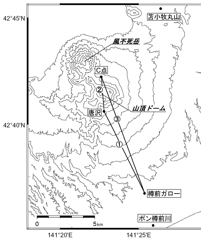
図6 樽前山 GPS 観測点配置図
