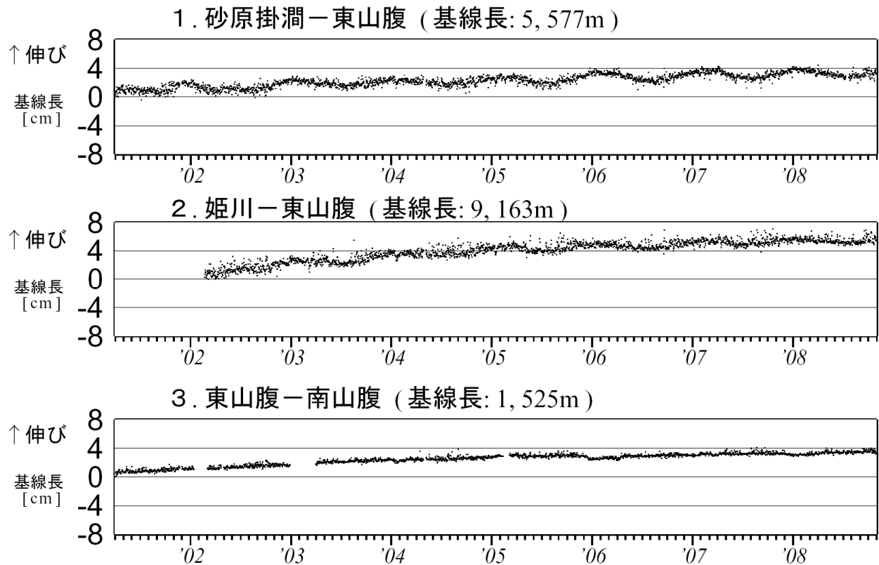
図 5 北海道駒ヶ岳 GPS 連続観測による基線長変化（2001 年 4 月～2008 年 10 月） グラフの空白部分は欠測 ・ 図 5 の 1～3 は、図 6 の GPS 基線①～③に対応しています。
