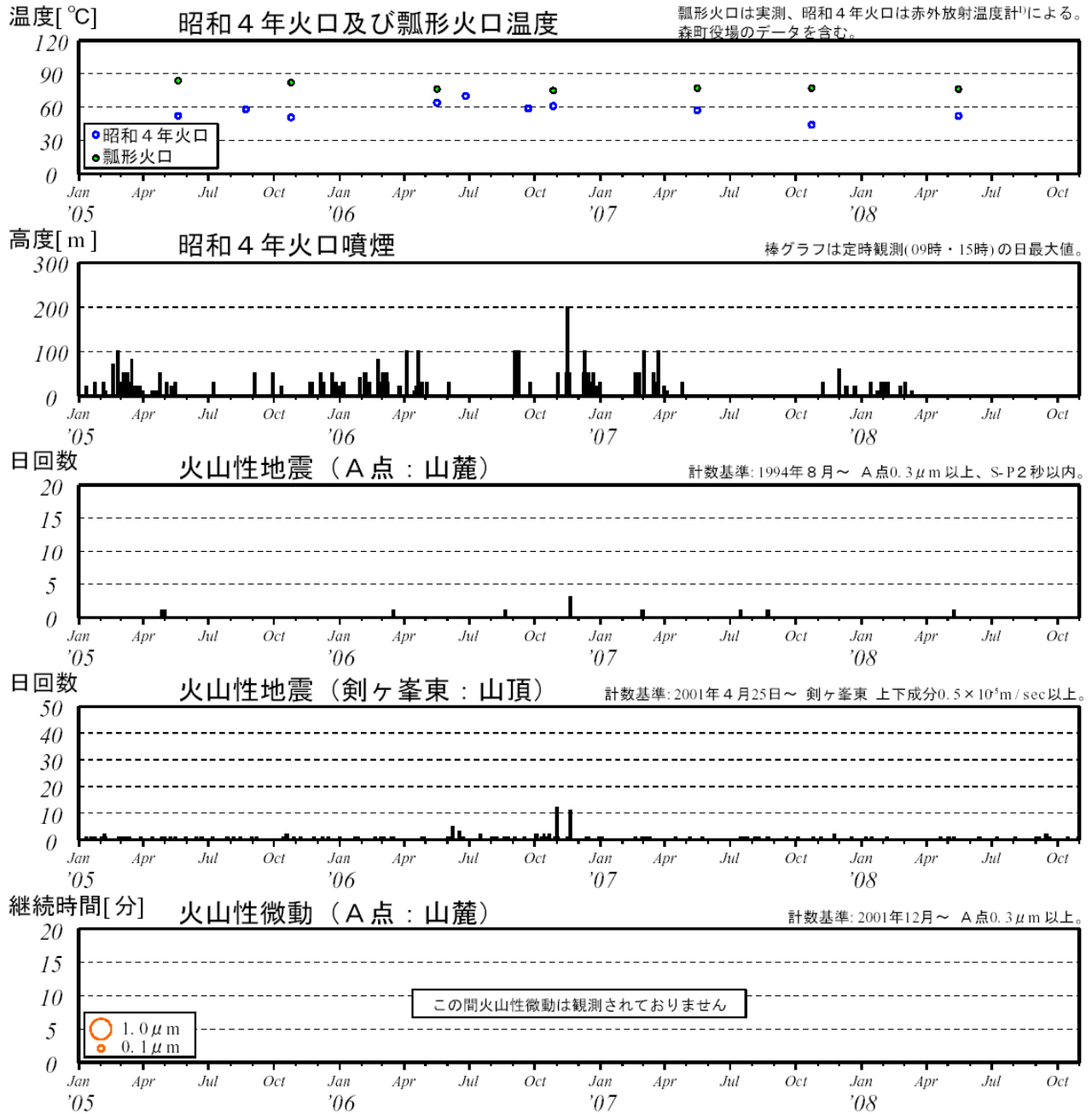
図3※ 北海道駒ヶ岳 最近の火山活動経過図（2005年1月～2008年10月）
