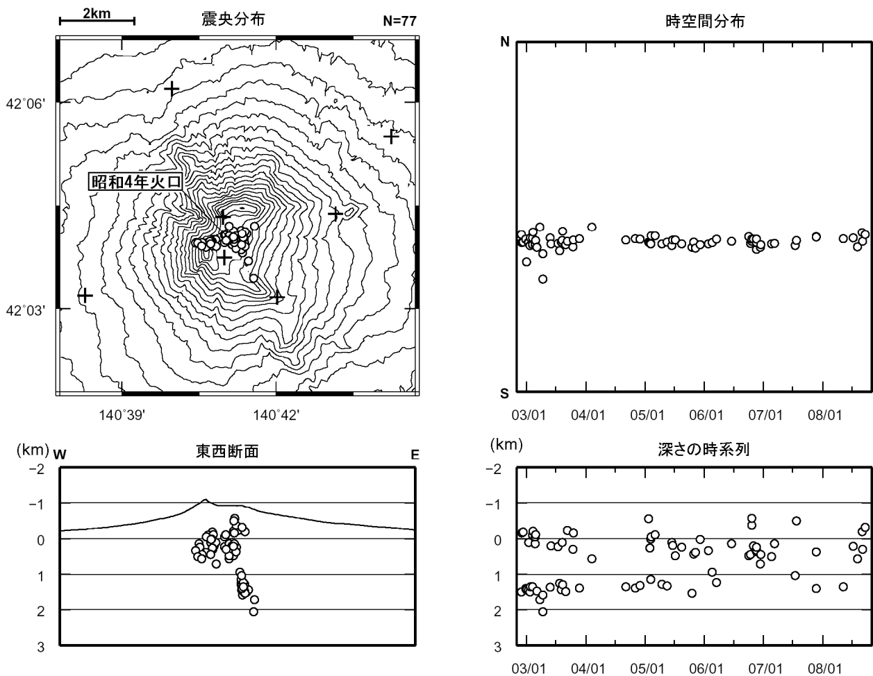
図 4※ 北海道駒ヶ岳 震源分布図（2002 年 11 月～2008 年 10 月、+は地震観測点）
