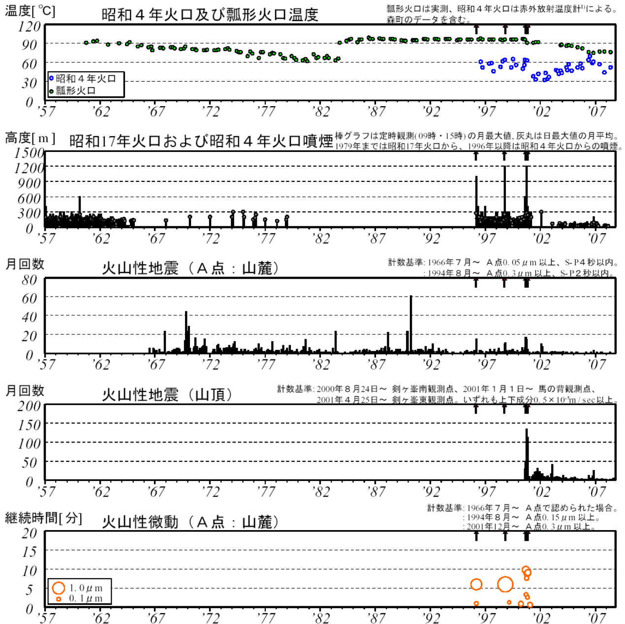
図2※ 北海道駒ヶ岳 長期の火山活動経過図（1957年1月～2008年10月）↑印は噴火
