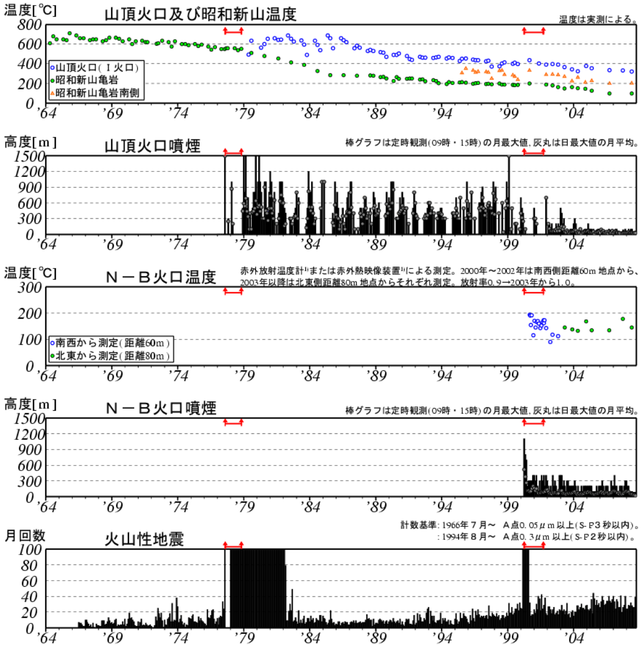
図 2 有珠山 長期の火山活動経過図（1964 年 1 月～2008 年 9 月）
