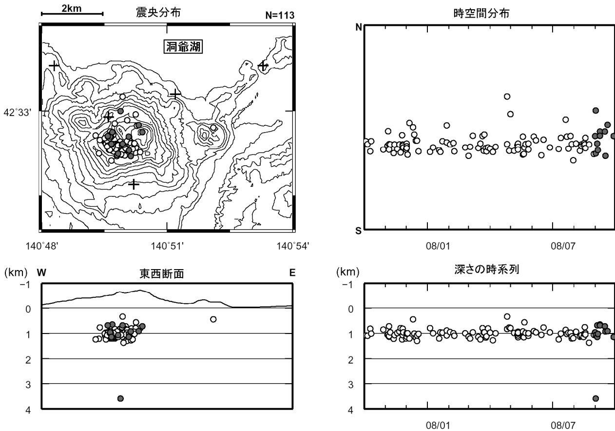
図 4 有珠山 震源分布図（2007 年 10 月～2008 年 9 月、+は地震観測点）
