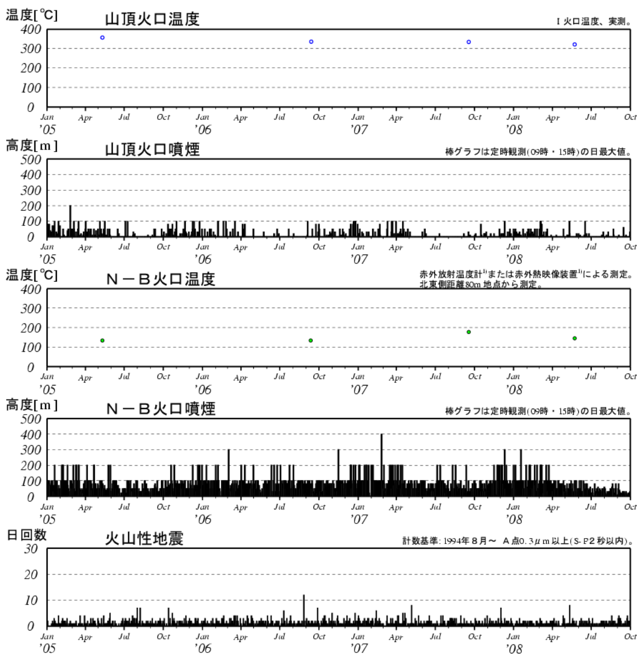
図3 有珠山 最近の火山活動経過図（2005年1月～2008年9月）
