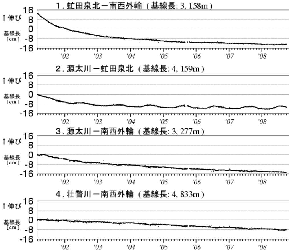
図5 有珠山 GPS 連続観測による基線長変化（2001年3月～2008年9月） グラフの空白部分は欠測 図5の1～4は、図6のGPS基線①～④に対応しています。
