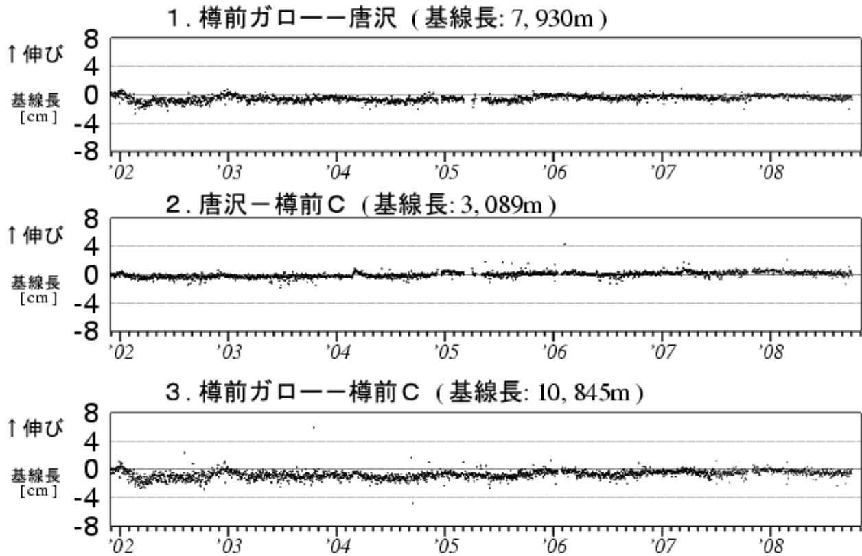
図5 樽前山 GPS 連続観測による基線長変化 (2001 年 12 月～2008 年 9 月) グラフの空白部分は欠測
