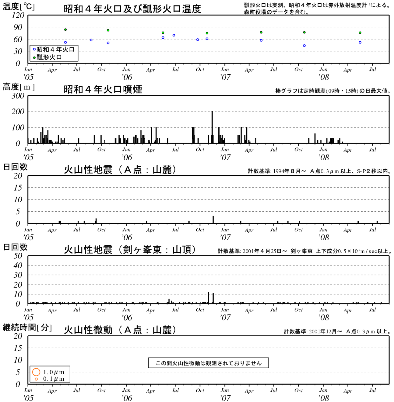
図 3※ 北海道駒ヶ岳 最近の火山活動経過図（2005 年 1 月～2008 年 8 月）
