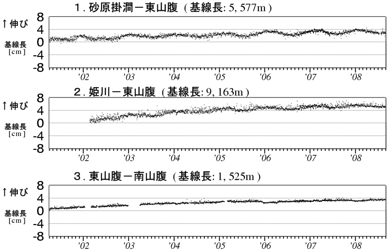
図5 北海道駒ヶ岳 GPS 連続観測による基線長変化（2001 年 4 月～2008 年 8 月）
