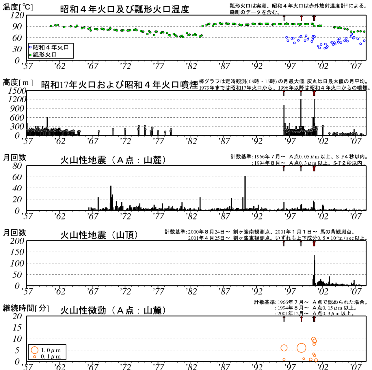
図 2 ※ 北海道駒ヶ岳 長期の火山活動経過図（1957 年 1 月～2008 年 8 月）↑印は噴火
