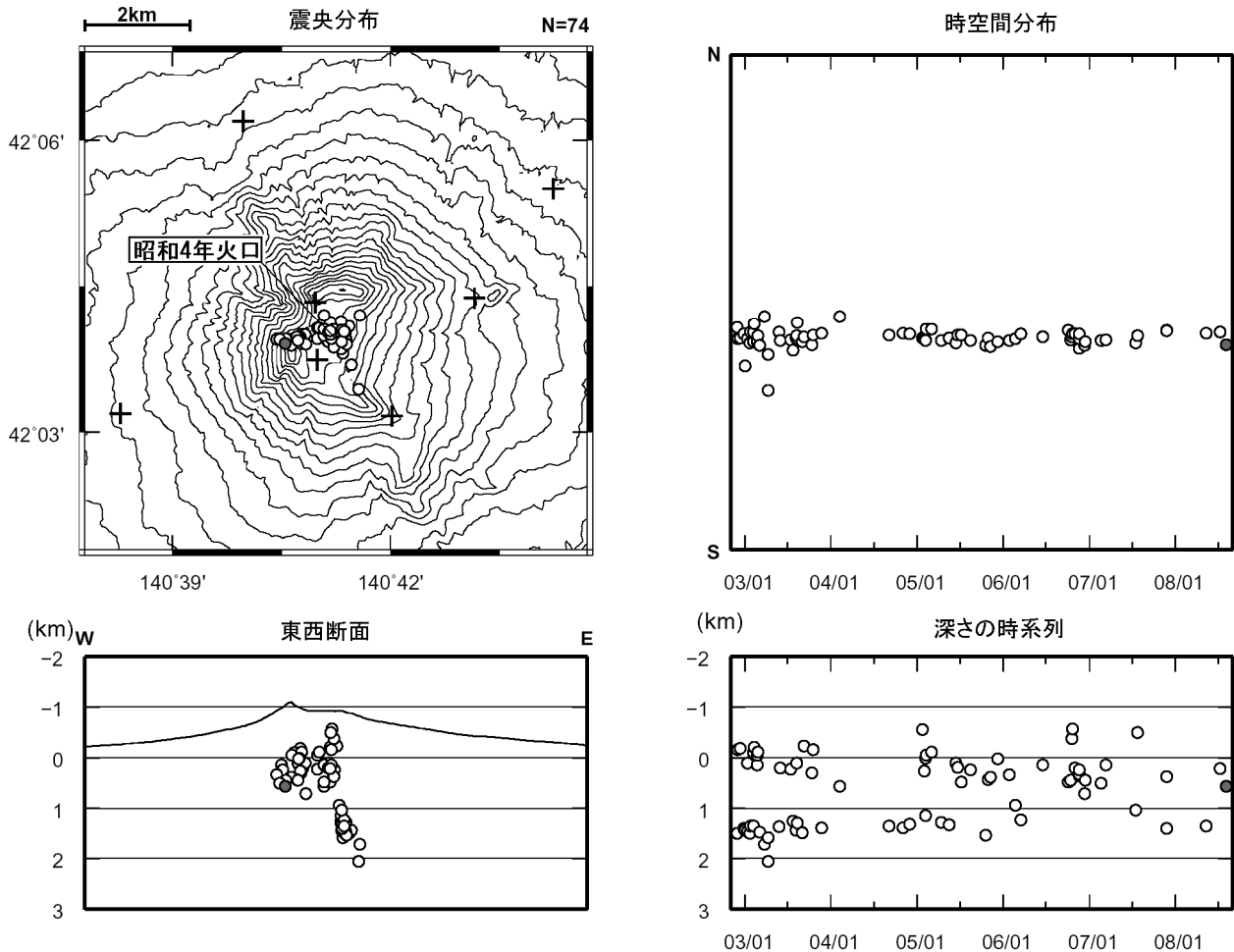
図 4 ※ 北海道駒ヶ岳 震源分布図（2002 年 11 月～2008 年 8 月、+は地震観測点）
