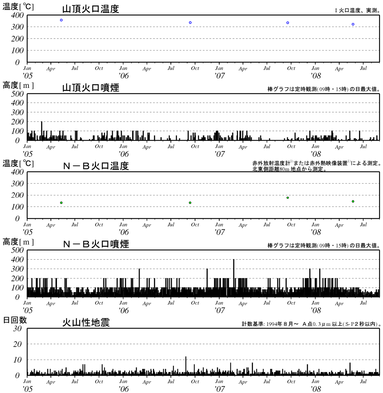
図3 有珠山 最近の火山活動経過図（2005年1月～2008年8月）
