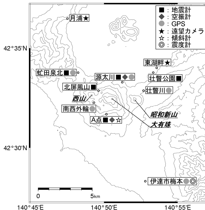
図 1 有珠山 火山観測点配置図
