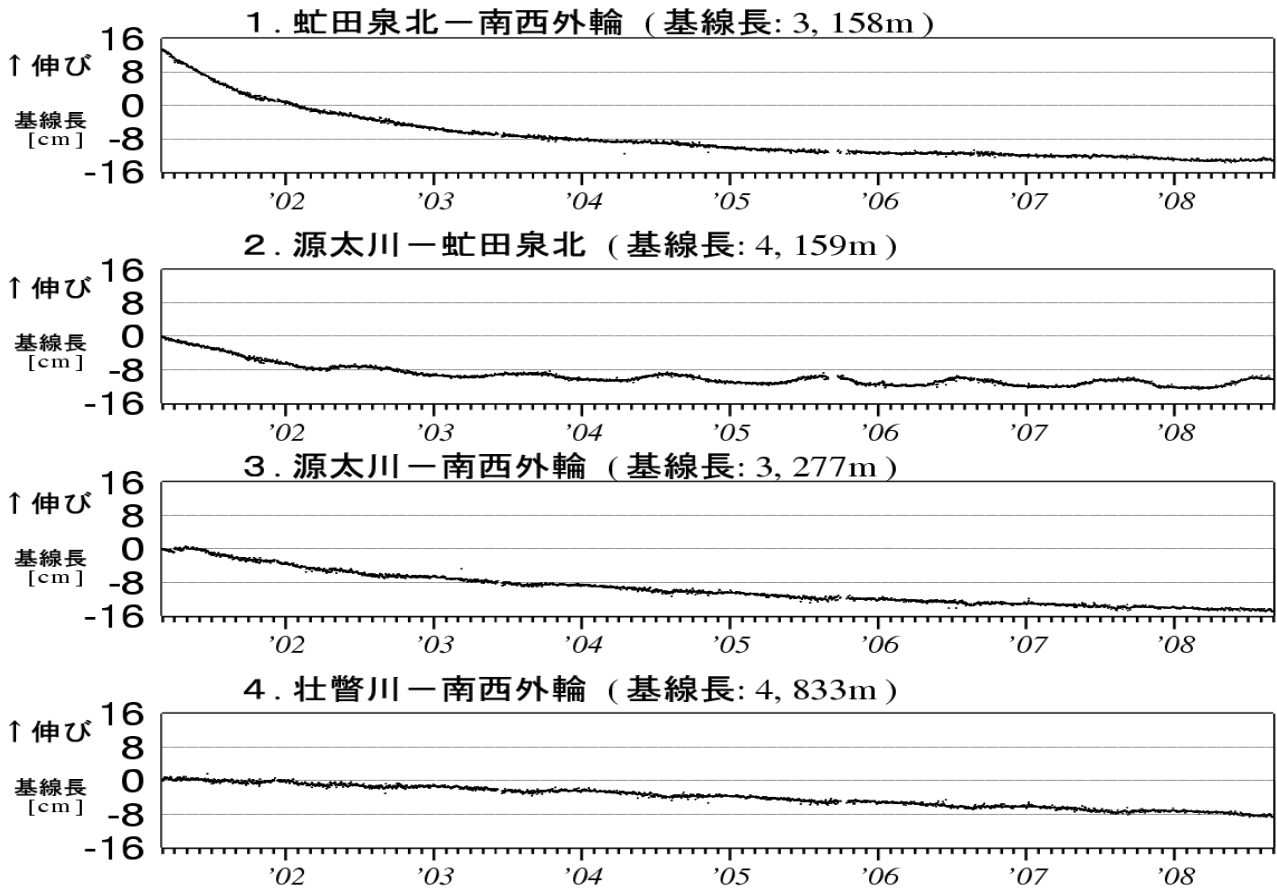
図5 有珠山 GPS 連続観測による基線長変化（2001年3月～2008年8月） グラフの空白部分は欠測 図5の1～4は、図6のGPS基線①～④に対応しています。
