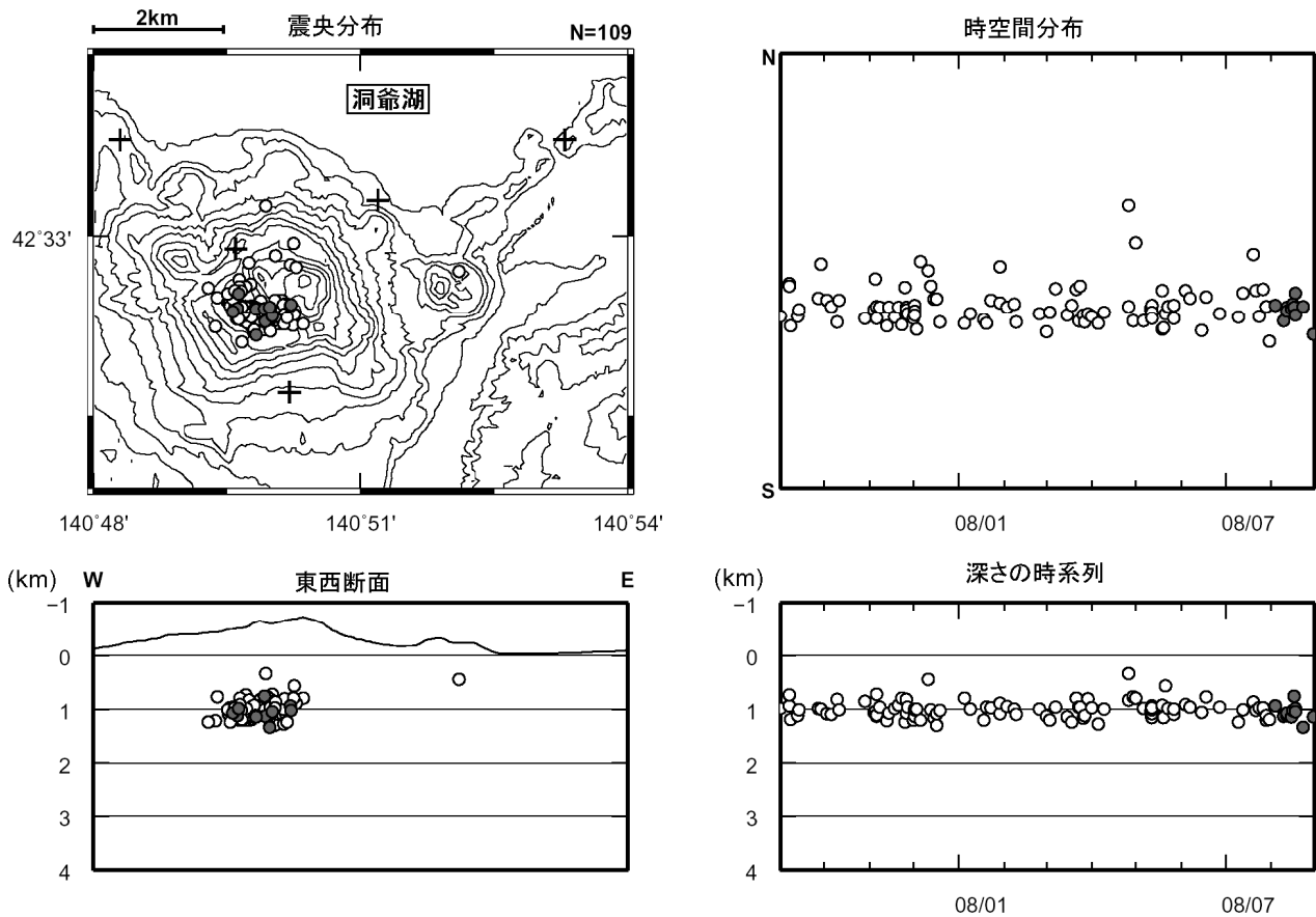
図 4 有珠山 震源分布図（2007 年 9 月～2008 年 8 月、+は地震観測点）
