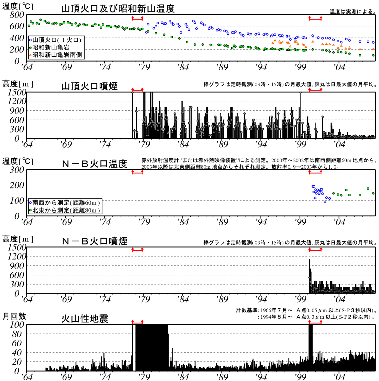
図2 有珠山 長期の火山活動経過図（1964年1月～2008年8月）
