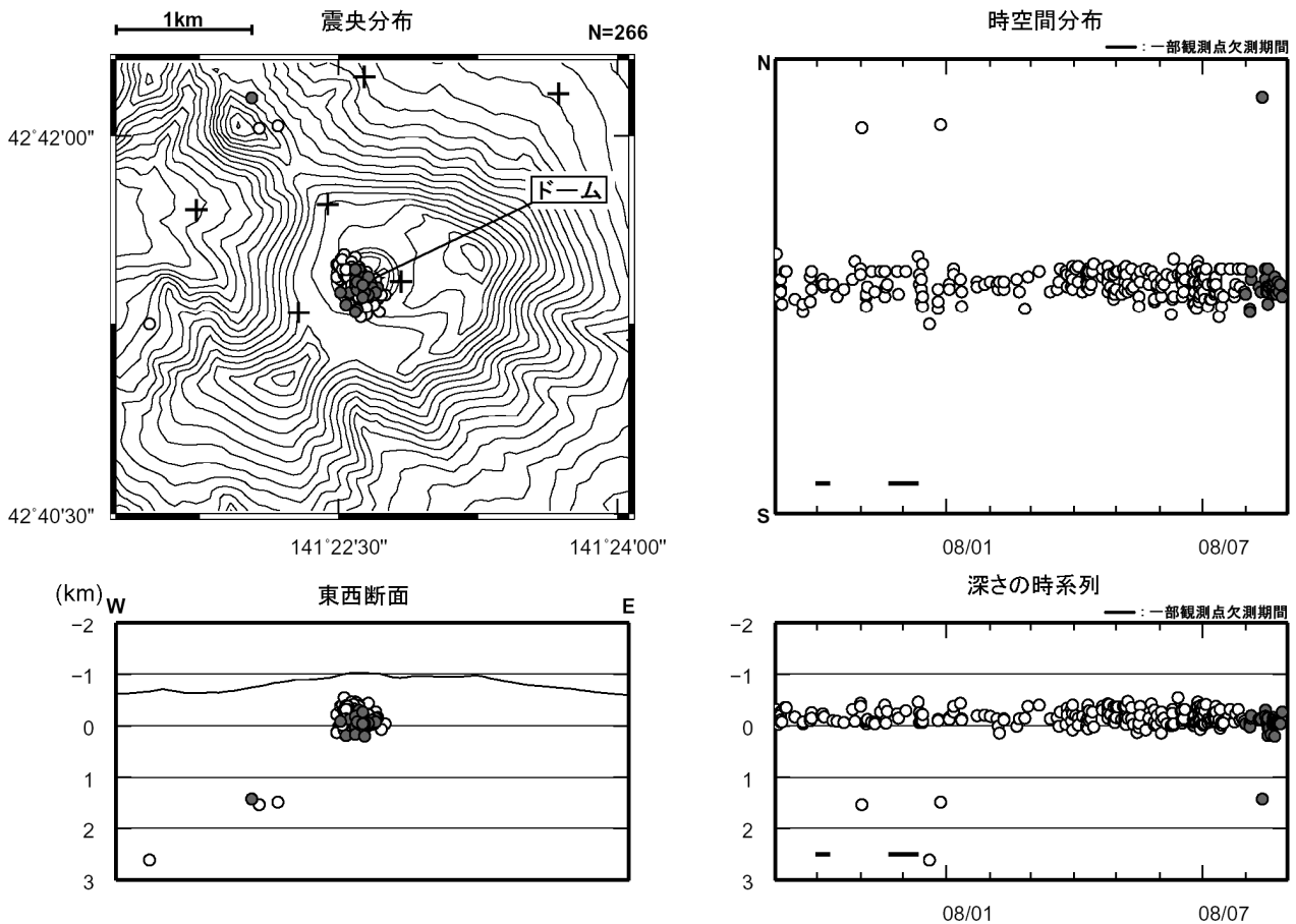
図 4※ 樽前山 震源分布図 (2007 年 9 月~2008 年 8 月、+は地震観測点)
