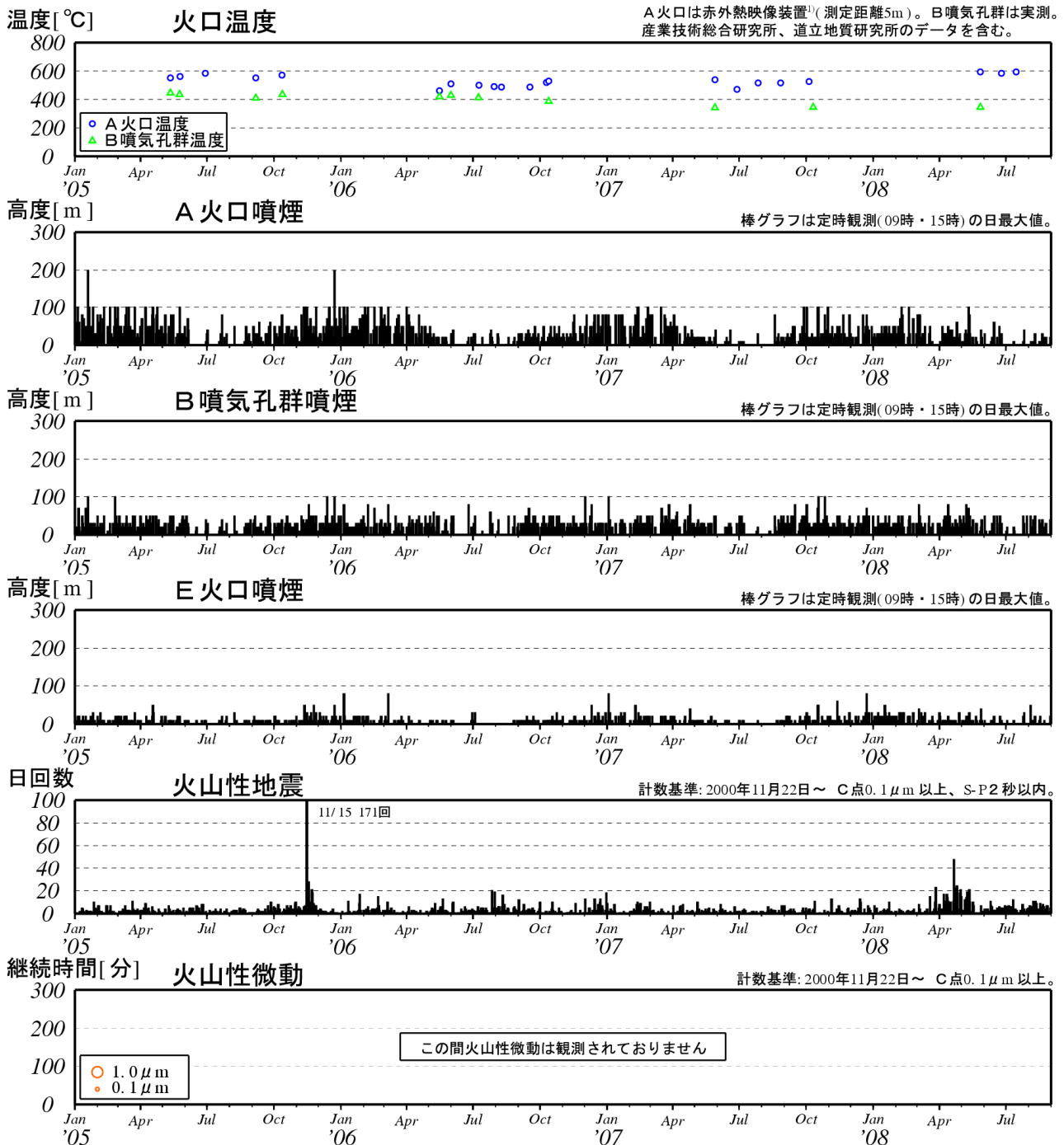
図3※ 樽前山 最近の火山活動経過図 (2005年1月～2008年8月)
