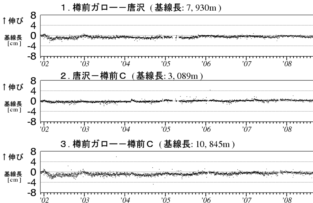
図5 樽前山 GPS 連続観測による基線長変化 (2001 年 12 月～2008 年 8 月) グラフの空白部分は欠測
