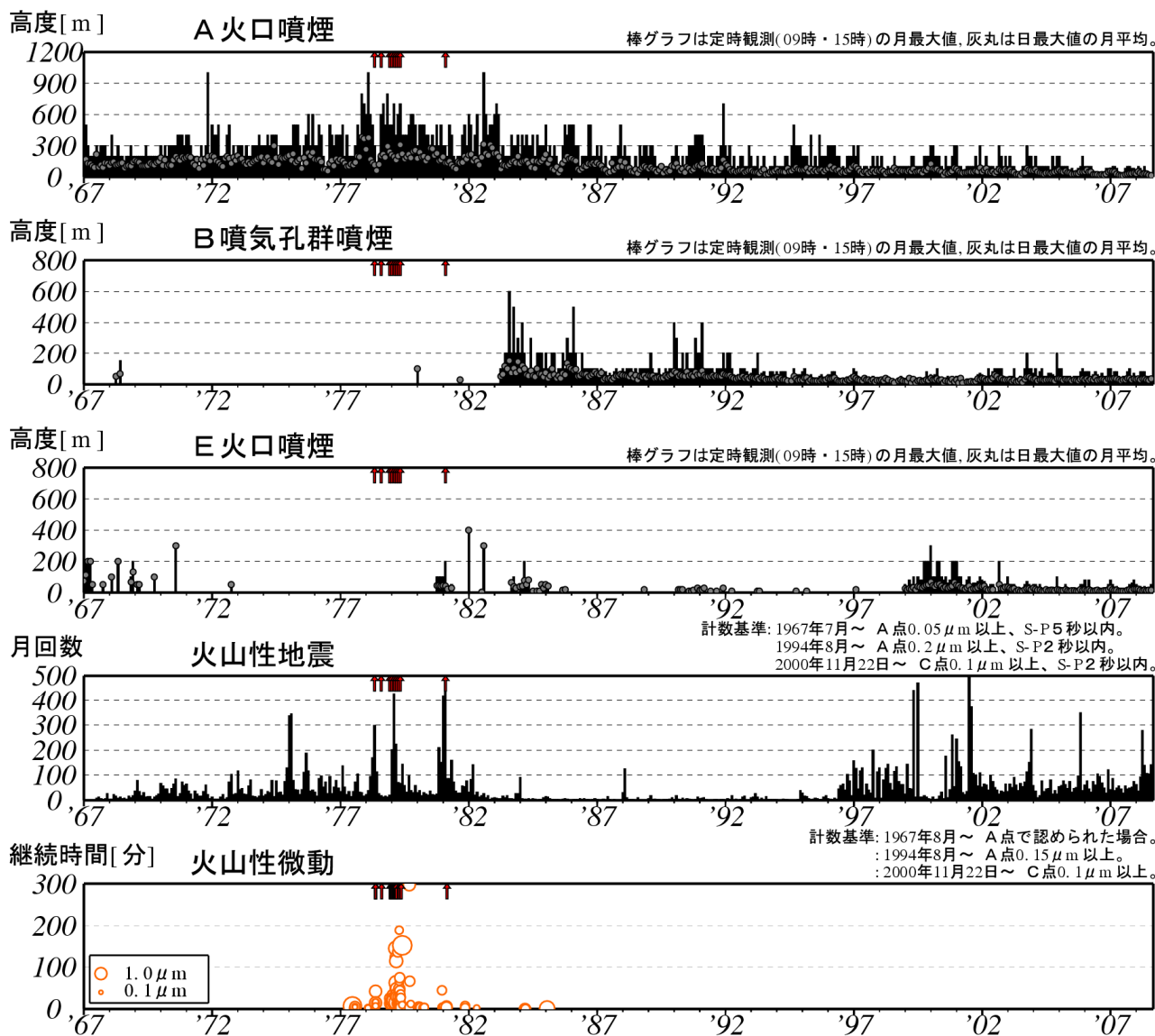
図 2※ 樽前山 長期の火山活動経過図 (1967 年 1 月～2008 年 8 月) ↑印は噴火
