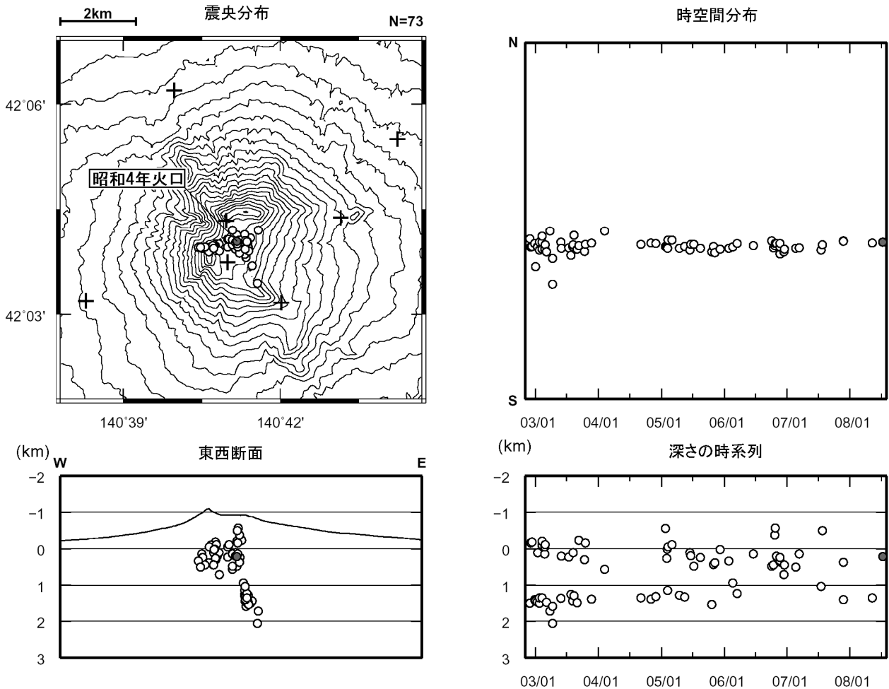
図 4 ※ 北海道駒ヶ岳 震源分布図（2002 年 11 月～2008 年 7 月、+は地震観測点）
