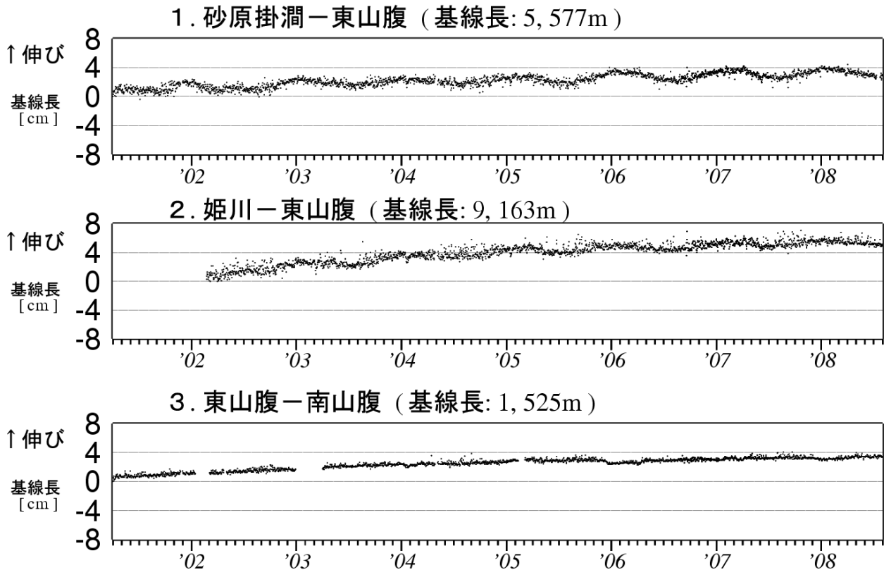
図 5 北海道駒ヶ岳 GPS 連続観測による基線長変化（2001 年 4 月～2008 年 7 月）
