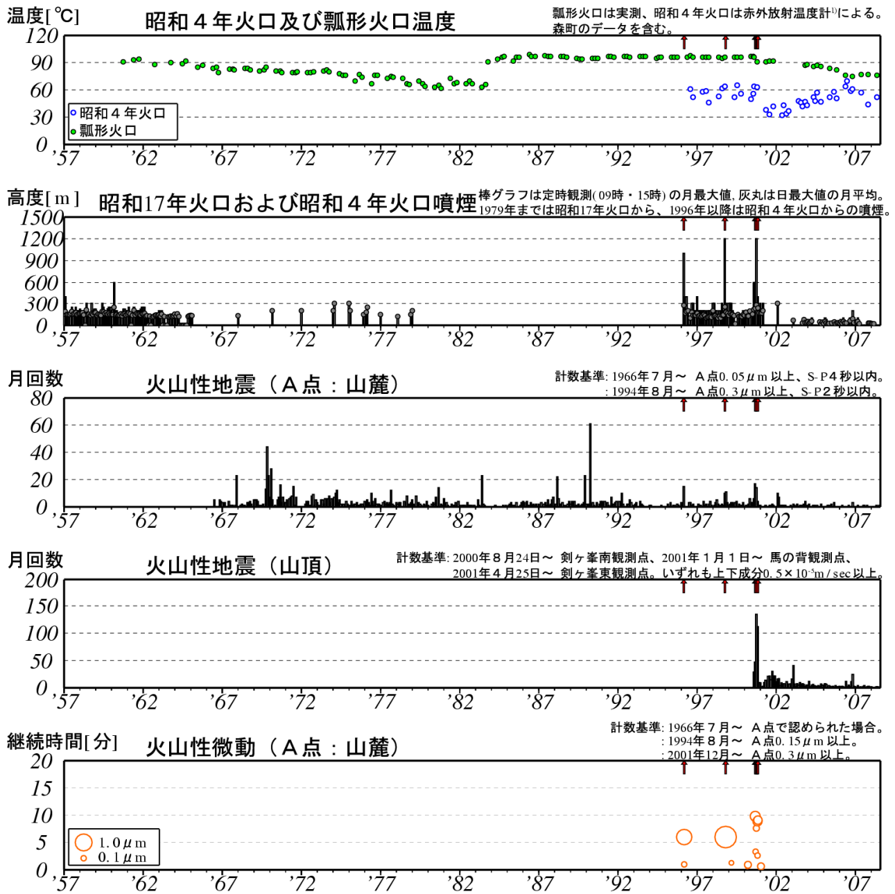
図2※ 北海道駒ヶ岳 長期の火山活動経過図（1957年1月～2008年7月）↑印は噴火
