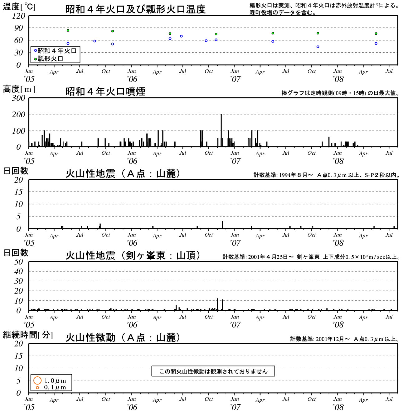
図 3※ 北海道駒ヶ岳 最近の火山活動経過図（2005 年 1 月～2008 年 7 月）
