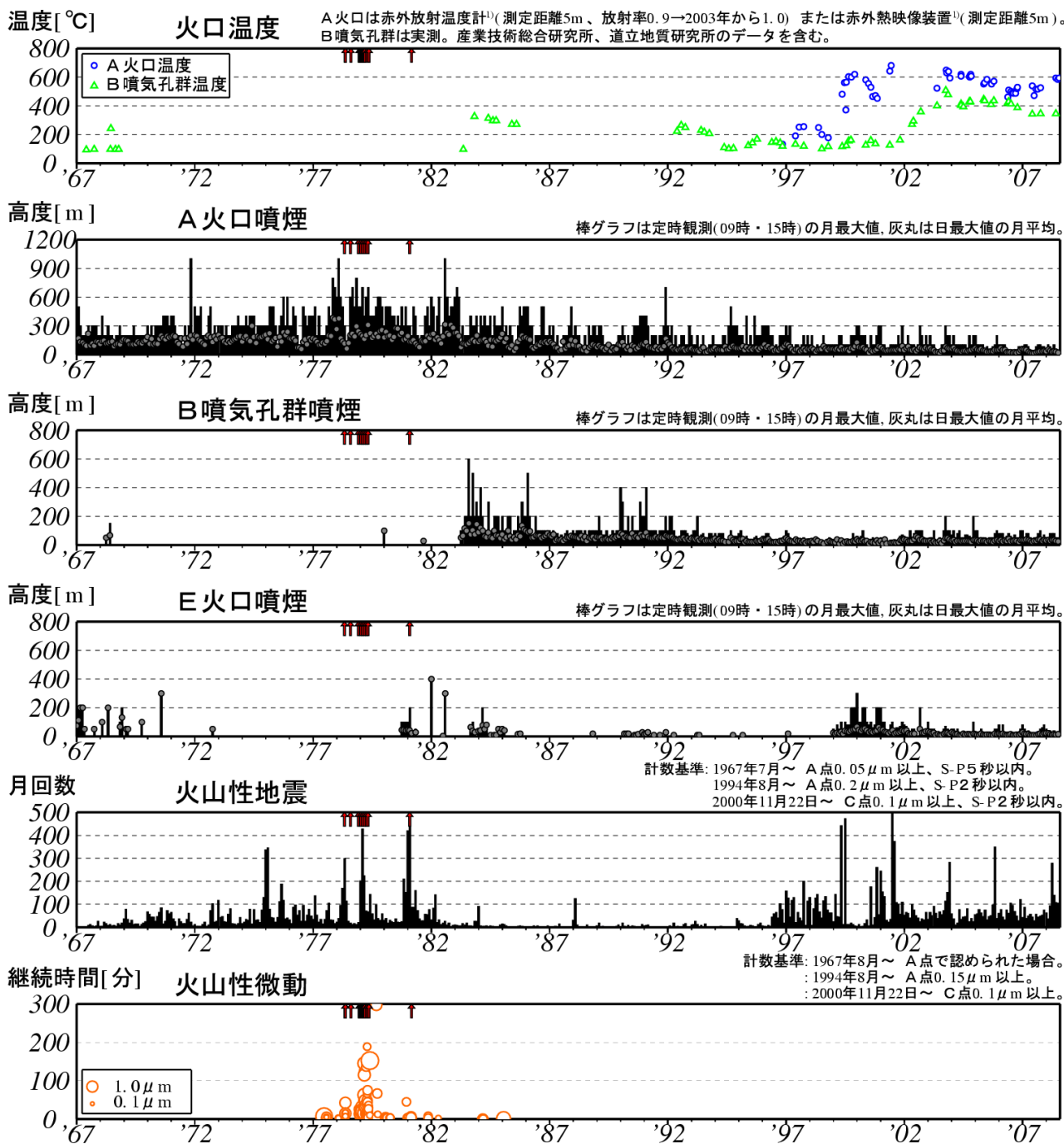
図 2※ 樽前山 長期の火山活動経過図 (1967 年 1 月~2008 年 7 月) ↑印は噴火
