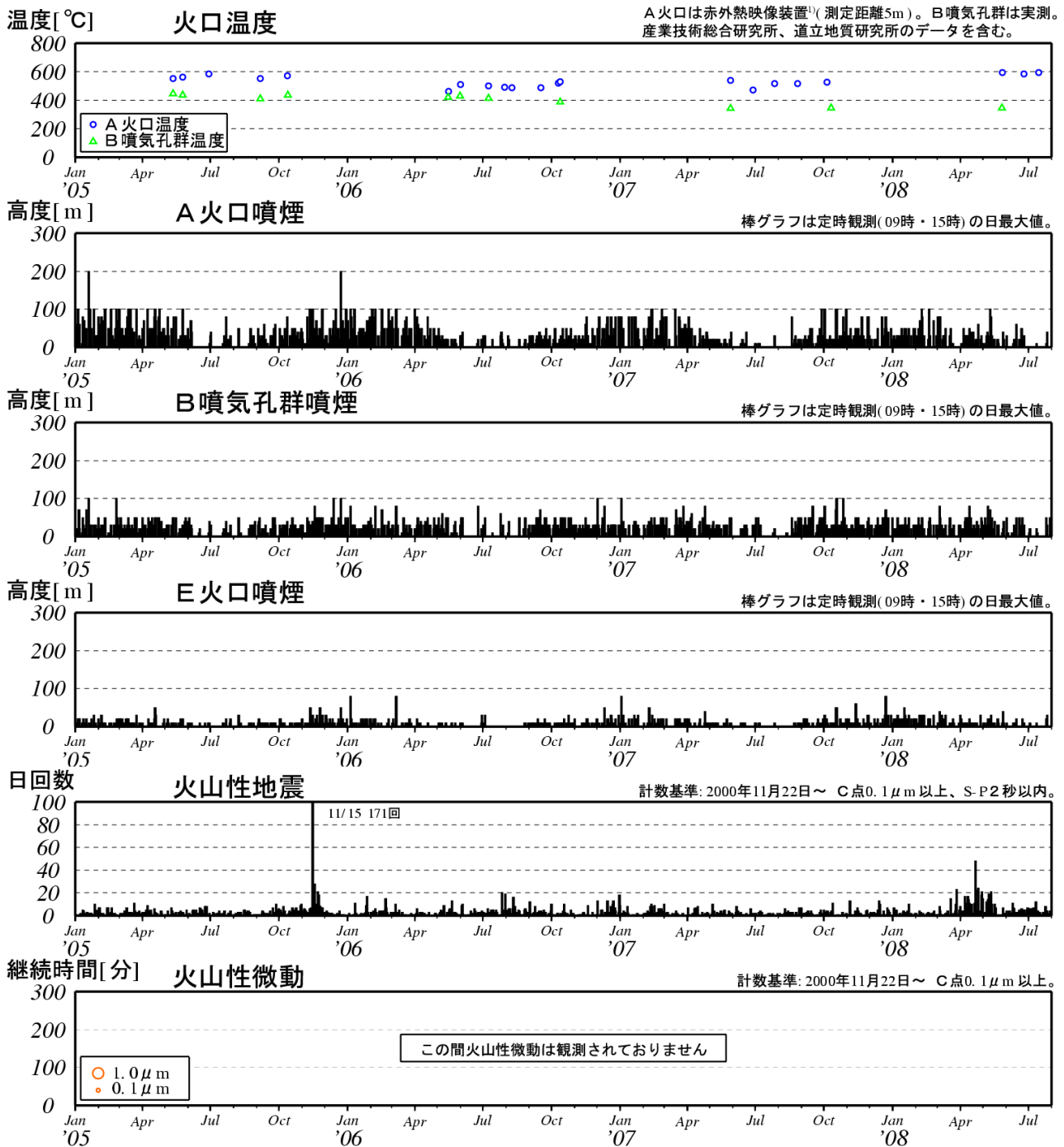
図3※ 樽前山 最近の火山活動経過図 (1995年1月～2008年7月)
