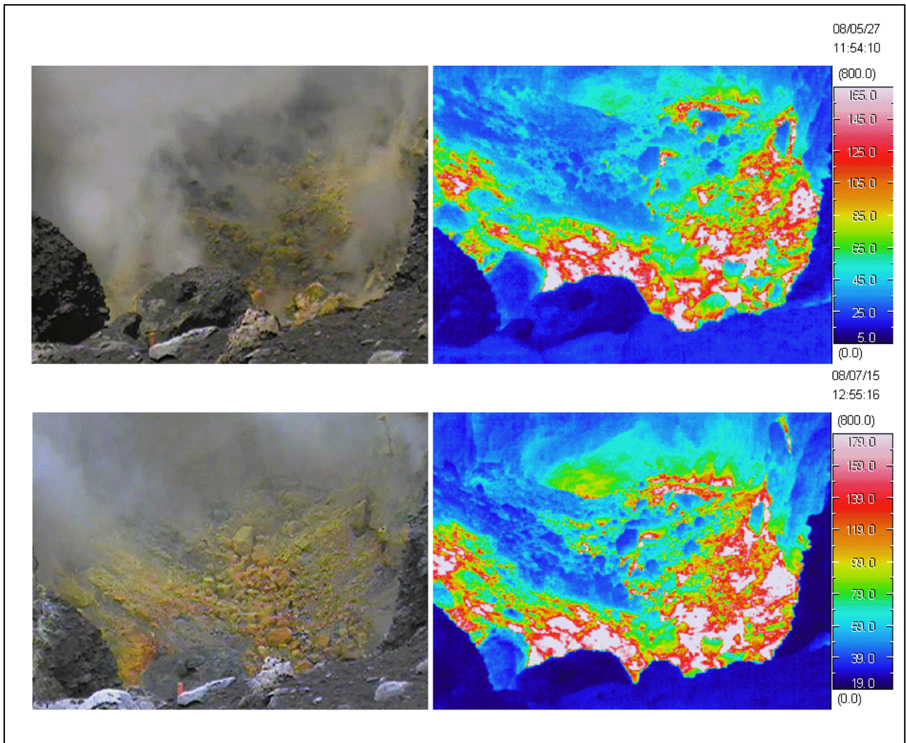
図4 樽前山 A火口内の赤外熱映像装置 1) による地表面温度分布 (南東側 40m付近から撮影) 撮影日：上段 2008年5月27日 下段 2008年7月15日
