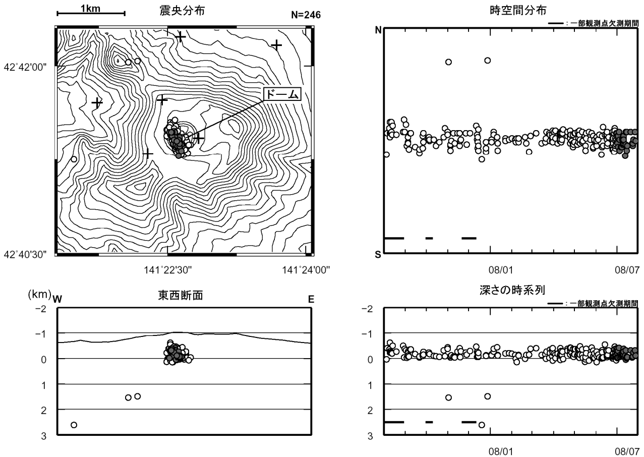
図 6※ 樽前山 震源分布図 (2007 年 8 月~2008 年 7 月、+は地震観測点)
