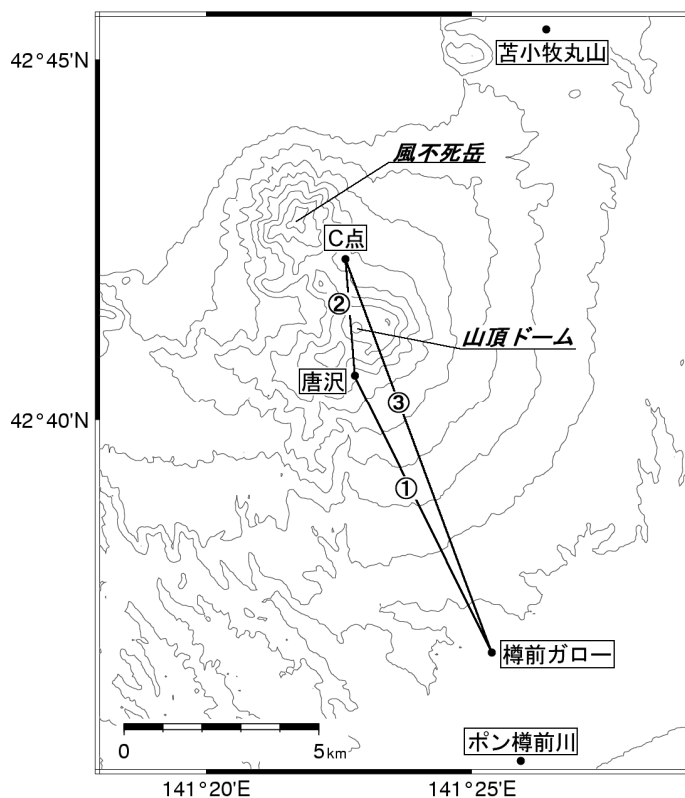
図8 樽前山 GPS 観測点配置図
