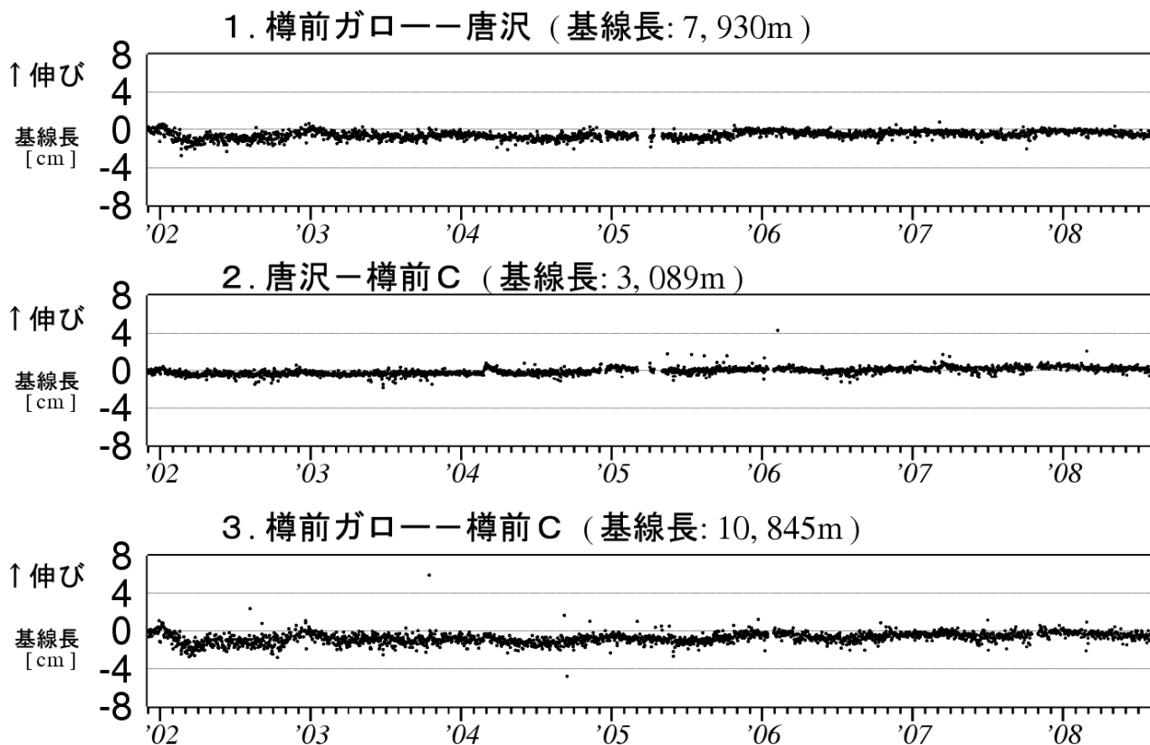
図7 樽前山 GPS 連続観測による基線長変化 (2001 年 12 月～2008 年 7 月) グラフの空白部分は欠測
