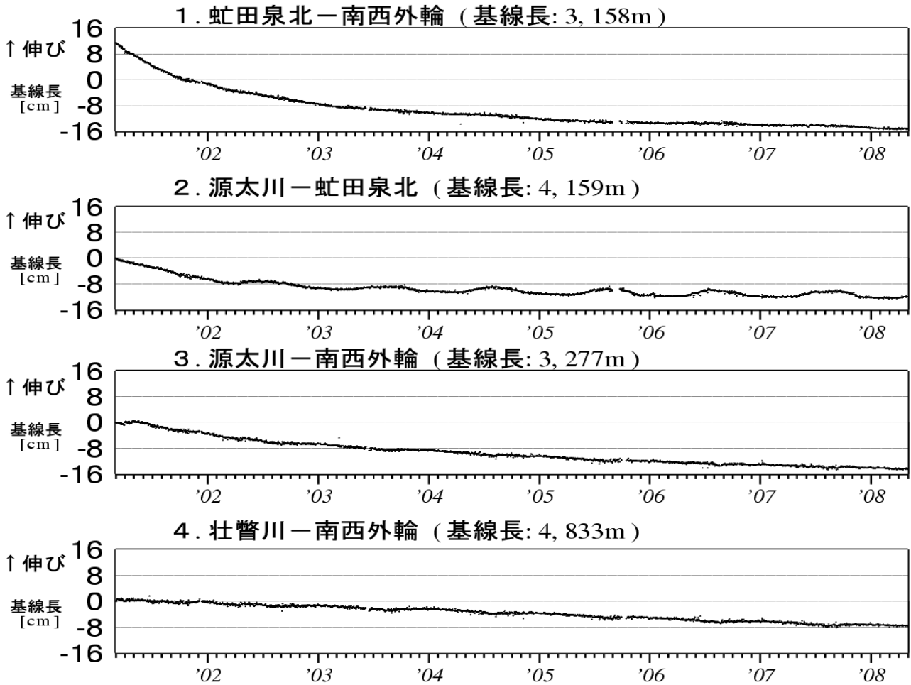
図5 有珠山 GPS 連続観測による基線長変化（2001年3月～2008年4月） グラフの空白部分は欠測 図6の1～4は、図5のGPS基線①～④に対応しています。
