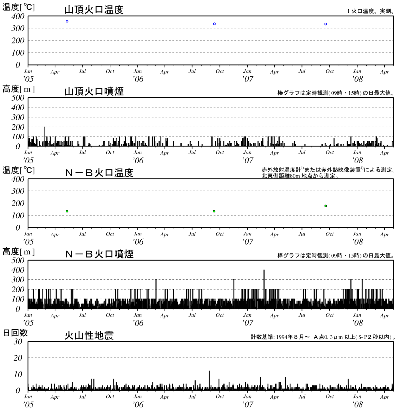
図3 有珠山 最近の火山活動経過図（2005年1月～2008年4月）
