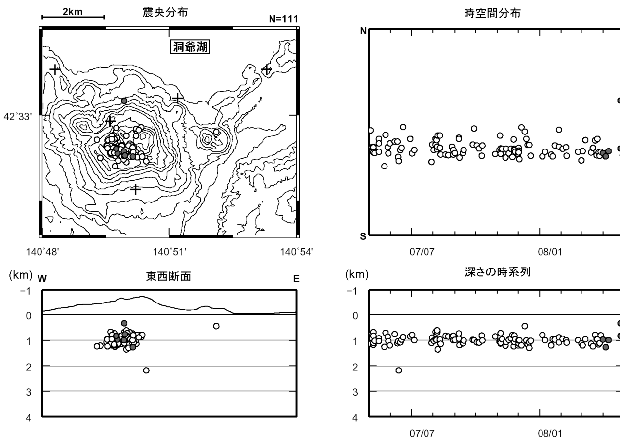
図 4 有珠山 震源分布図（2007 年 5 月～2008 年 4 月、+は地震観測点）
