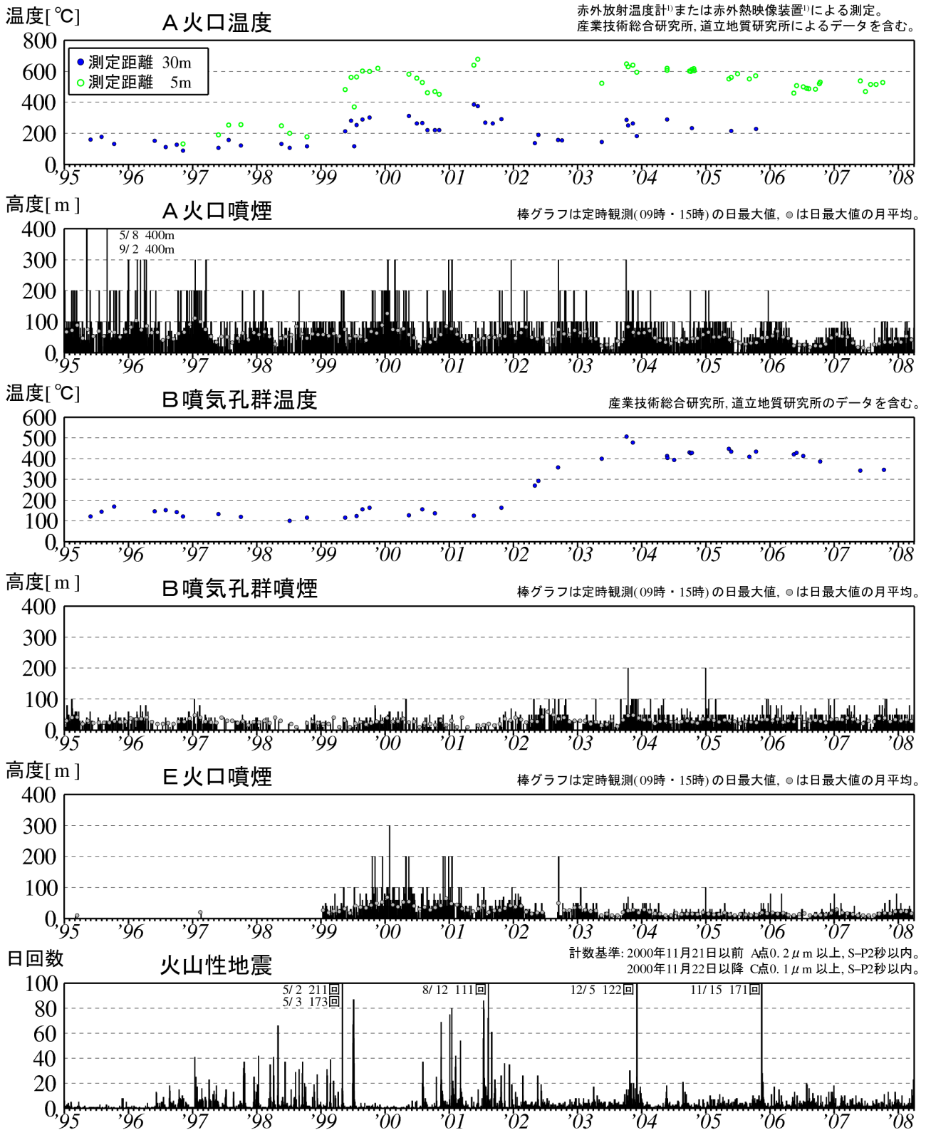
図 2※ 樽前山 最近の火山活動経過図 (1995 年 1 月～2008 年 3 月)
