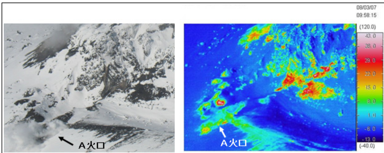
図5 樽前山 赤外熱映像装置 1) によるA火口周辺の地表面温度分布 (2008年3月7日 図4の②方向上空より撮影)
