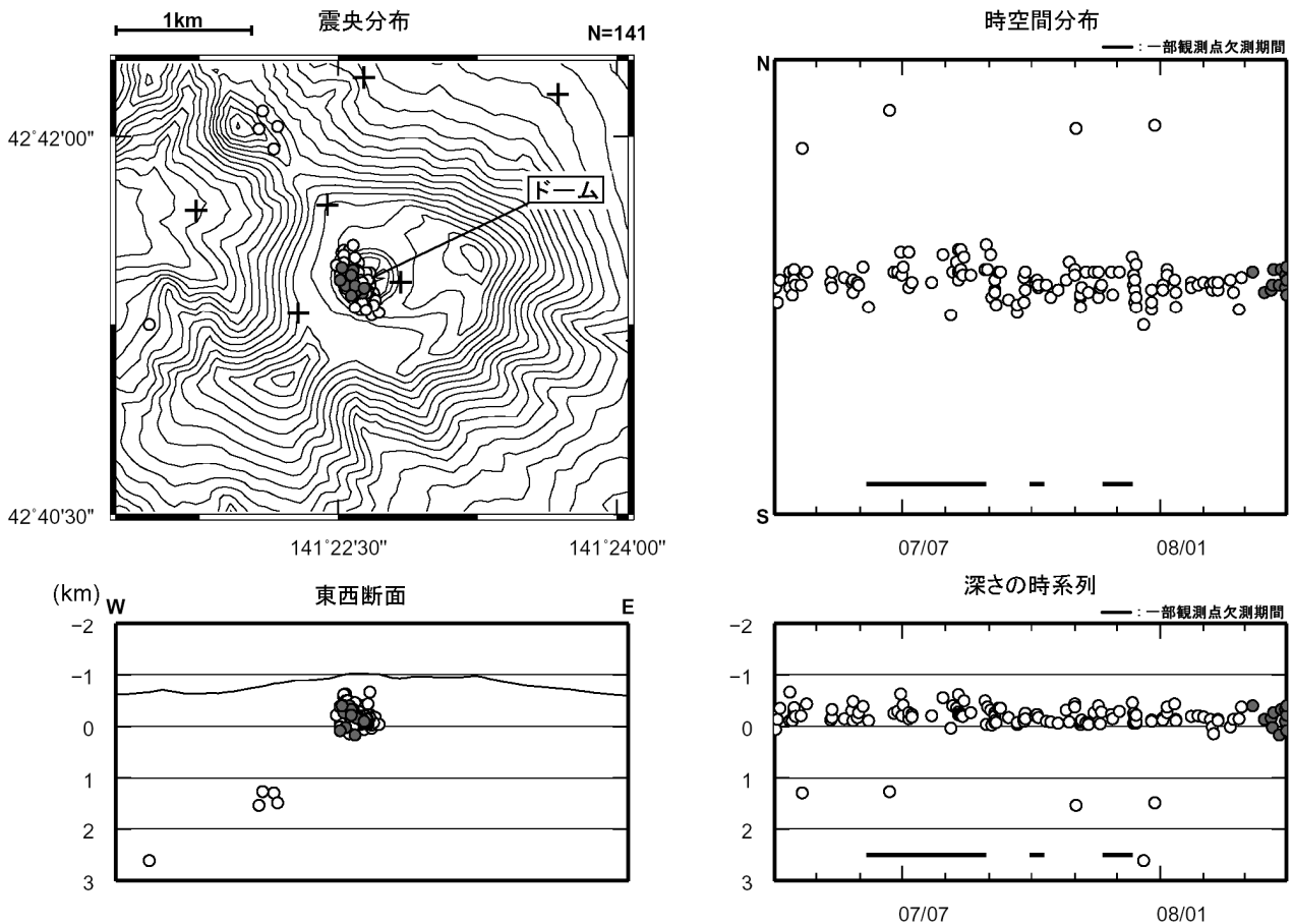
図 7※ 樽前山 震源分布図 (2007 年 4 月～2008 年 3 月、+は地震観測点)
