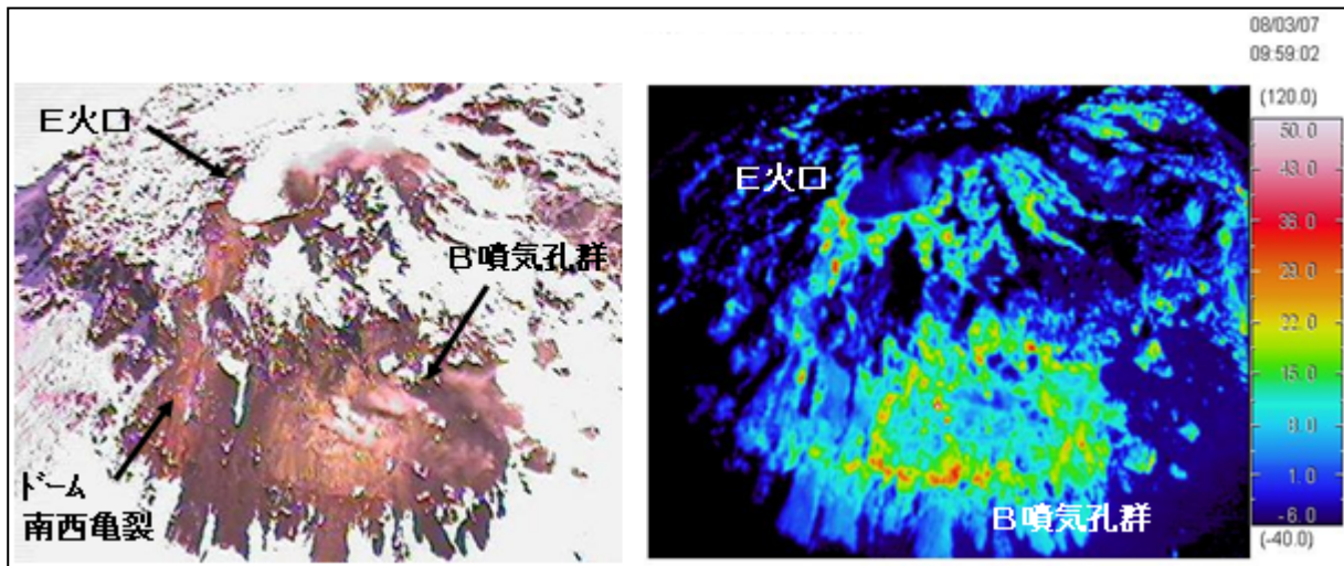
図6 樽前山 赤外熱映像装置 1) によるB噴気孔群、E火口周辺の地表面温度分布 (2008年3月7日 図4の③方向上空より撮影)
