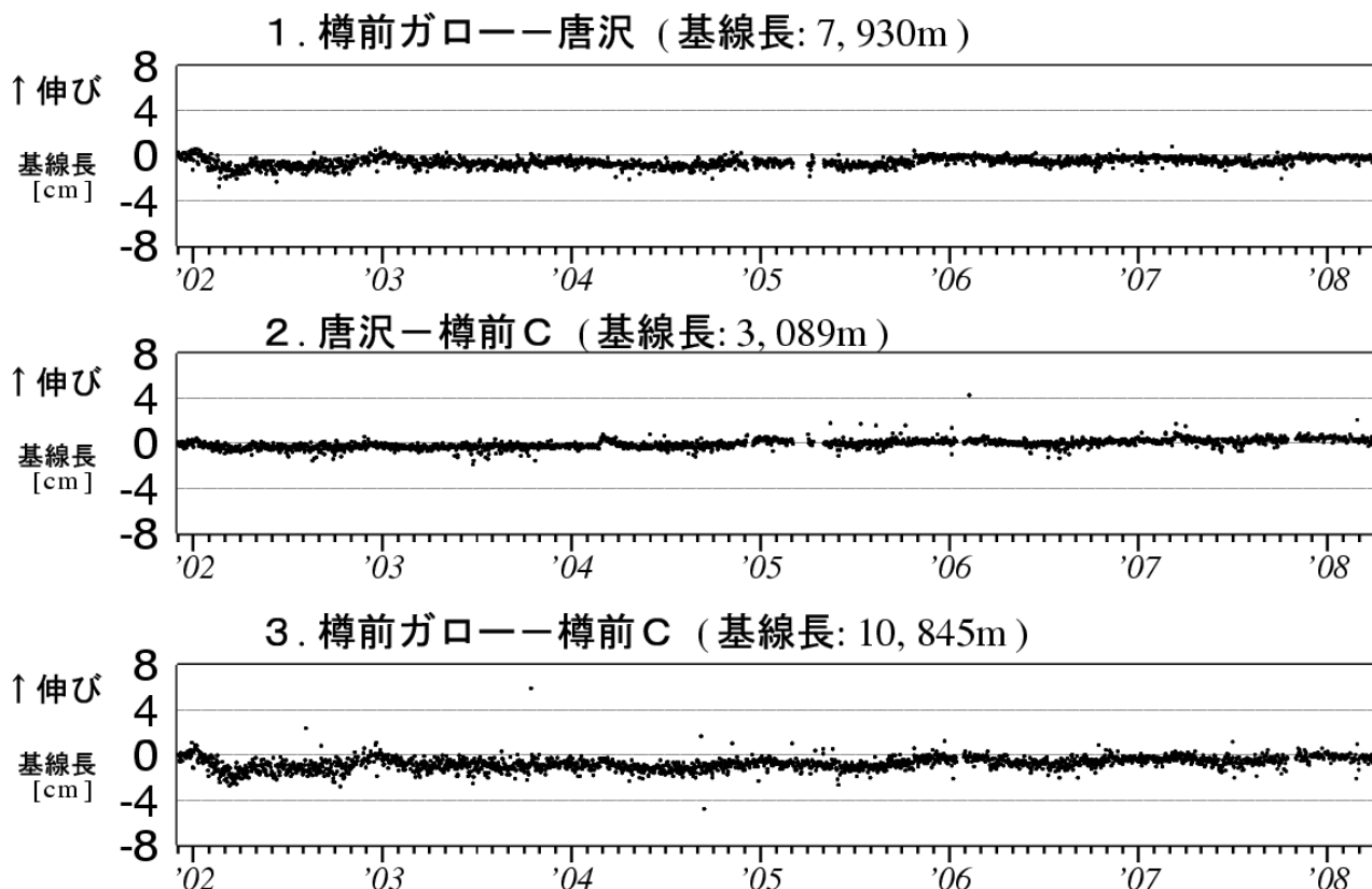
図8 樽前山 GPS 連続観測による基線長変化 (2001 年 12 月～2008 年 3 月) グラフの空白部分は欠測
