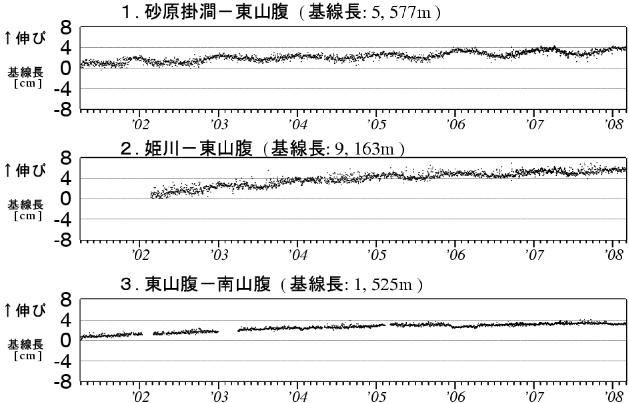
図 4 北海道駒ヶ岳 GPS 連続観測による基線長変化（2001 年 4 月～2008 年 2 月）
