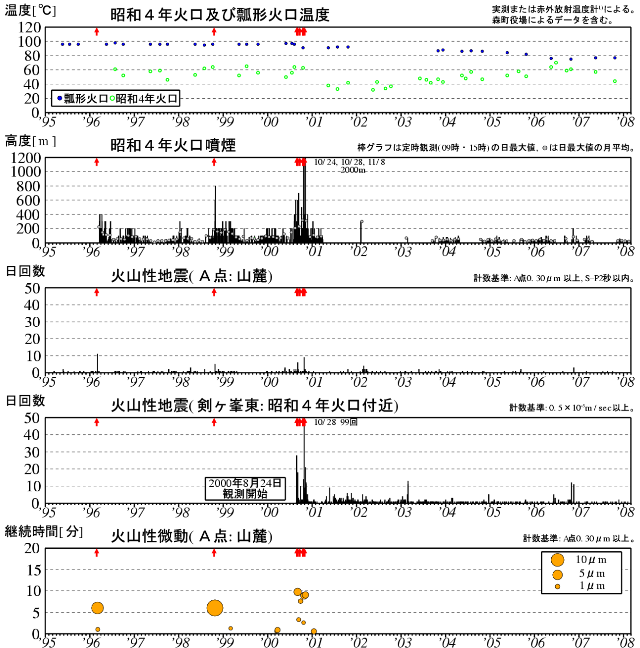
図 2※ 北海道駒ヶ岳 最近の火山活動経過図（1995 年 1 月～2008 年 2 月）↑印は噴火
