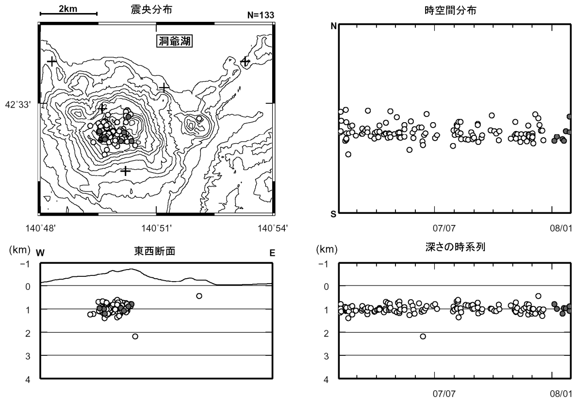
図5 有珠山 震源分布図（2007年2月～2008年1月、+は地震観測点）
