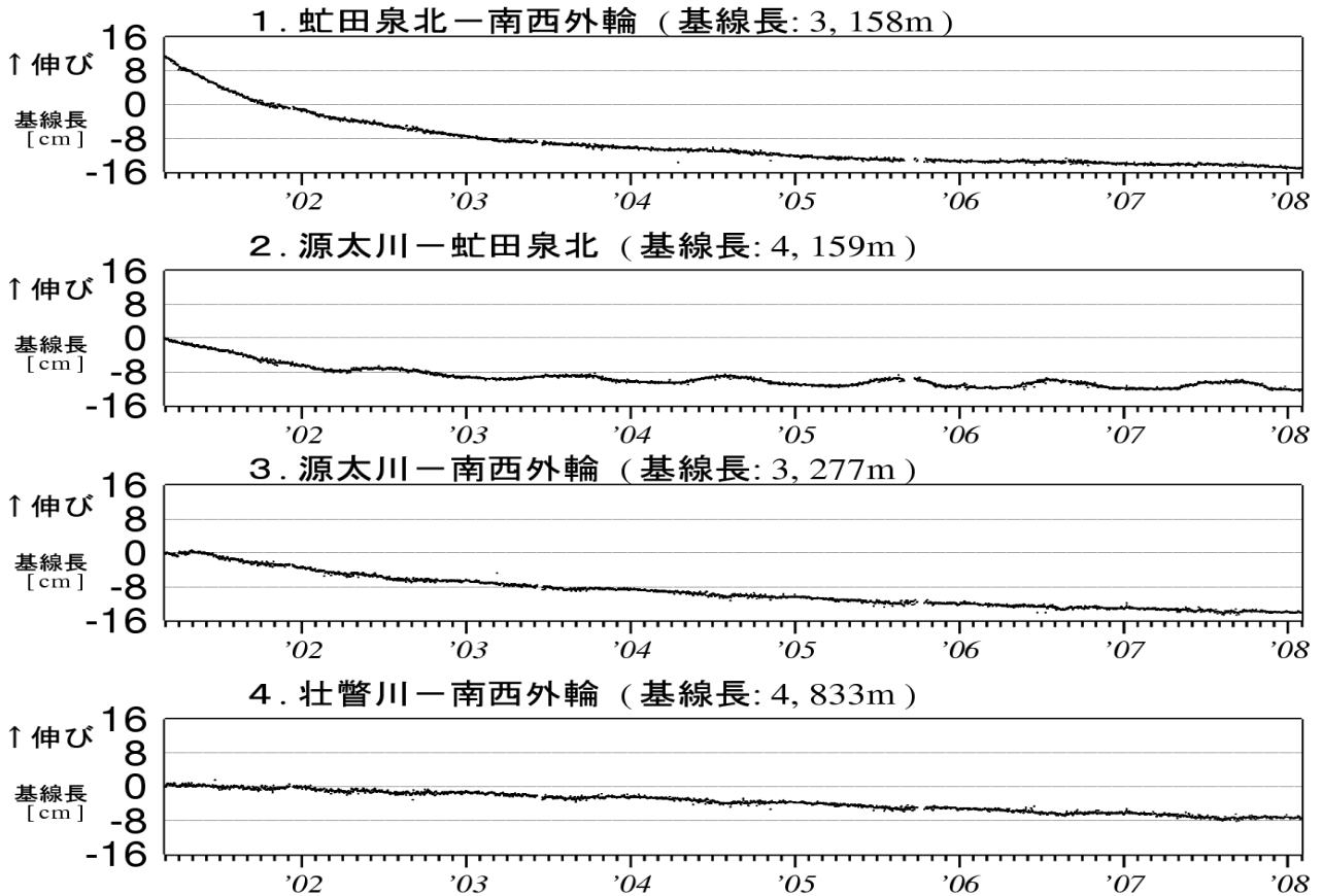
図 6 有珠山 GPS 連続観測による基線長変化（2001 年 3 月～2008 年 1 月） グラフの空白部分は欠測 図 6 の 1～4 は、図 7 の GPS 基線①～④に対応しています。
