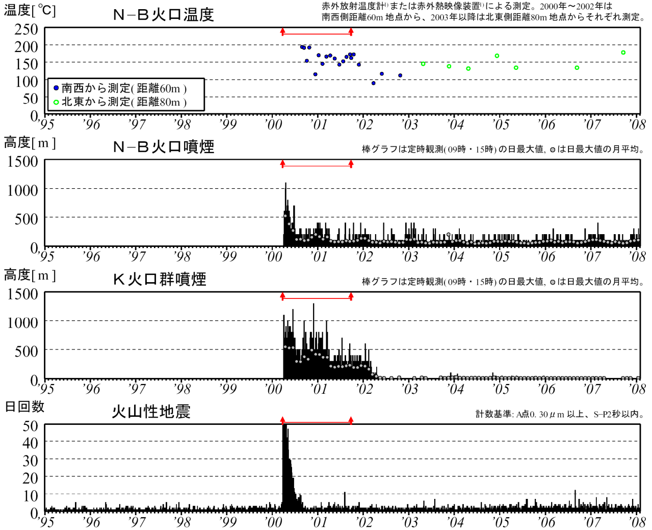
図2 有珠山 最近の火山活動経過図（1995年1月～2008年1月）
