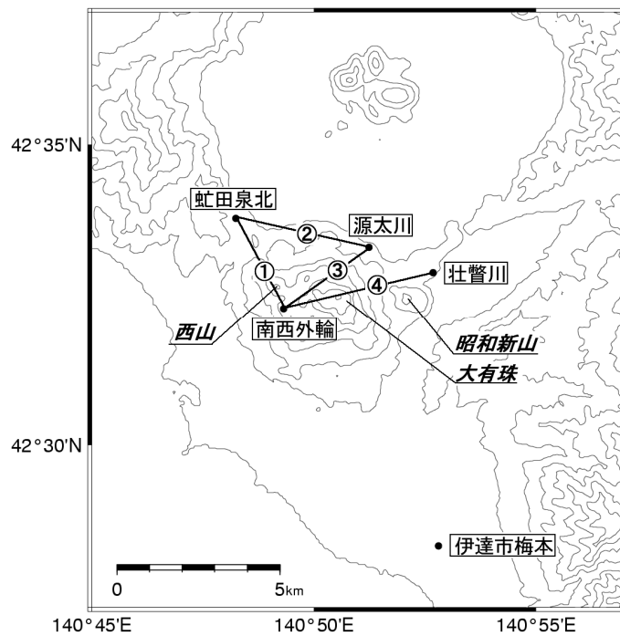
図 7 有珠山 GPS 連続観測点配置図
