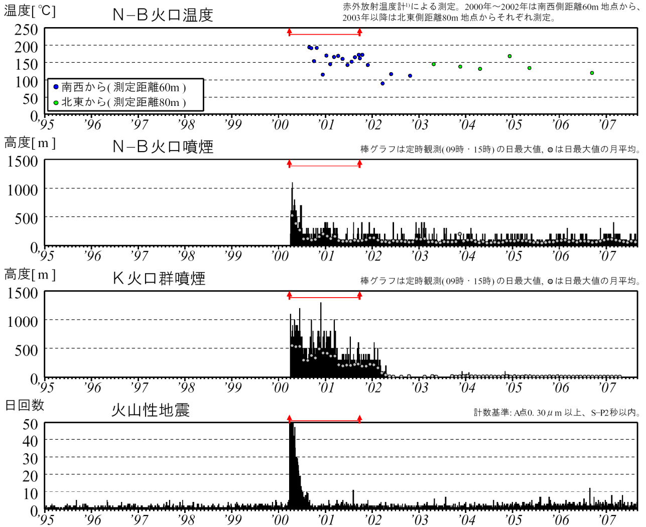
図2 有珠山 最近の火山活動経過図（1995年1月～2007年8月）
