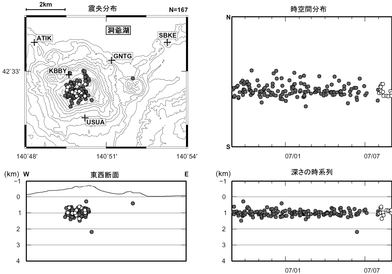
図 3 有珠山の震源分布図（2006年9月～2007年8月、+は地震観測点）
