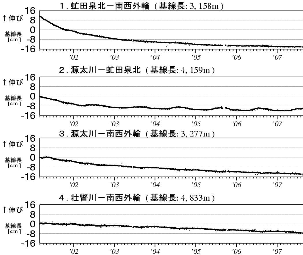
図4 有珠山 GPS 連続観測による基線長変化（2001年3月～2007年8月） グラフの空白部分は欠測 図4の1～4は、図5のGPS基線①～④に対応しています。
