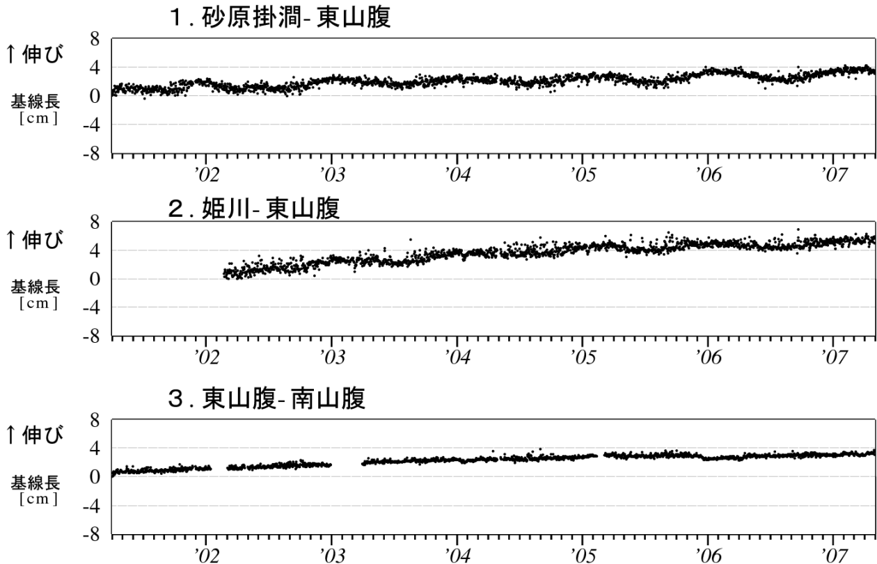
図 4 北海道駒ヶ岳 GPS 連続観測による基線長変化（2001 年 4 月～2007 年 4 月）
