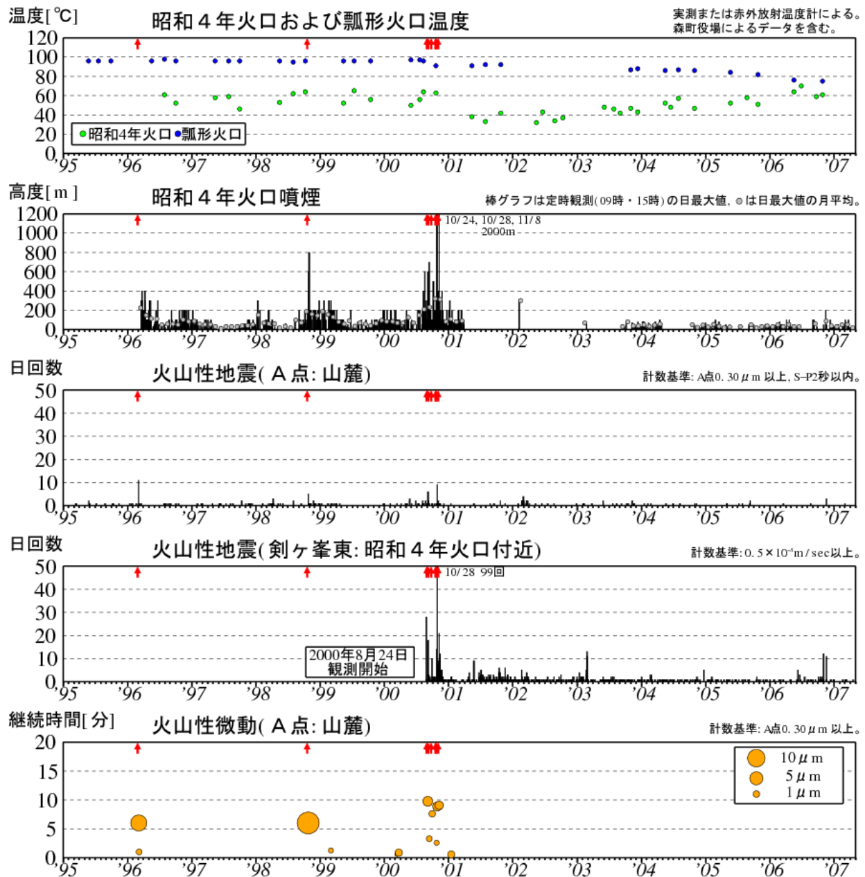
図 2※ 北海道駒ヶ岳 最近の火山活動経過図（1995 年 1 月～2007 年 4 月）↑印は噴火 ・昭和 4 年火口では 2003 年 9 月以降 10～50m 程度の噴煙が時折観測されています。 ・昭和 4 年火口の火口温度は、2002 年以降緩やかな上昇傾向が認められています。
