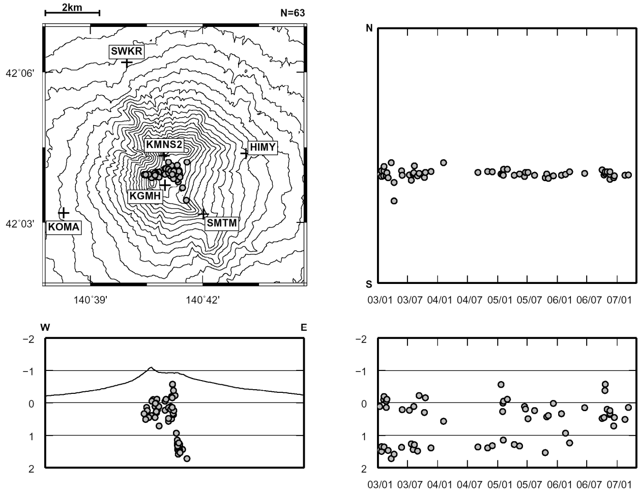
図 3 北海道駒ヶ岳の震源分布図（2003 年 1 月 1 日～2007 年 4 月 30 日、+は地震観測点）
