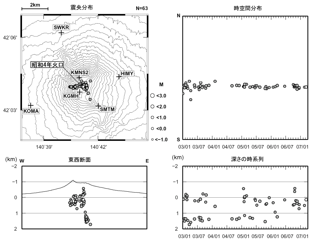
図 5 北海道駒ヶ岳の震源分布図（2003 年 1 月 1 日～2007 年 3 月 31 日、+は地震観測点） ○印は今期間（2007 年 3 月）の震源 ●印は 2003 年 1 月～2007 年 2 月に求まった震源 ・これまでに求まった震源は山頂火口原直下の浅い所（山頂から深さ約 1～3km 付近）に分布しています。今期間に求まった震源もこの領域内に分布しています。
