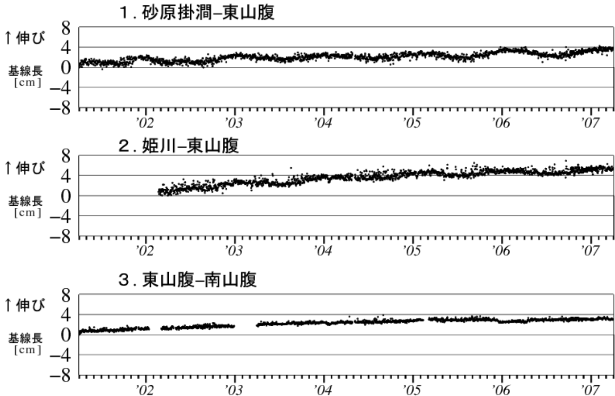
図 6 北海道駒ヶ岳 GPS 連続観測による基線長変化（2001 年 4 月～2007 年 3 月）
