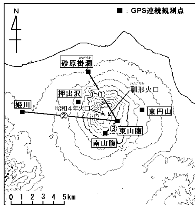
図 7 北海道駒ヶ岳 GPS 連続観測点配置図
