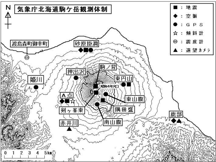
図 1 北海道駒ヶ岳火山観測点配置図
