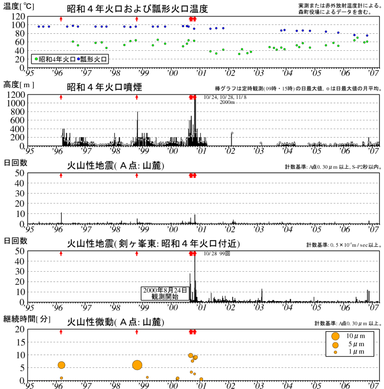
図 2※ 北海道駒ヶ岳 最近の火山活動経過図（1995 年 1 月～2007 年 3 月）↑印は噴火 ・昭和 4 年火口では 2003 年 9 月以降 10～50m 程度の噴煙が時折観測されています。 ・昭和 4 年火口の火口温度は、2002 年以降緩やかな上昇傾向が認められています。
