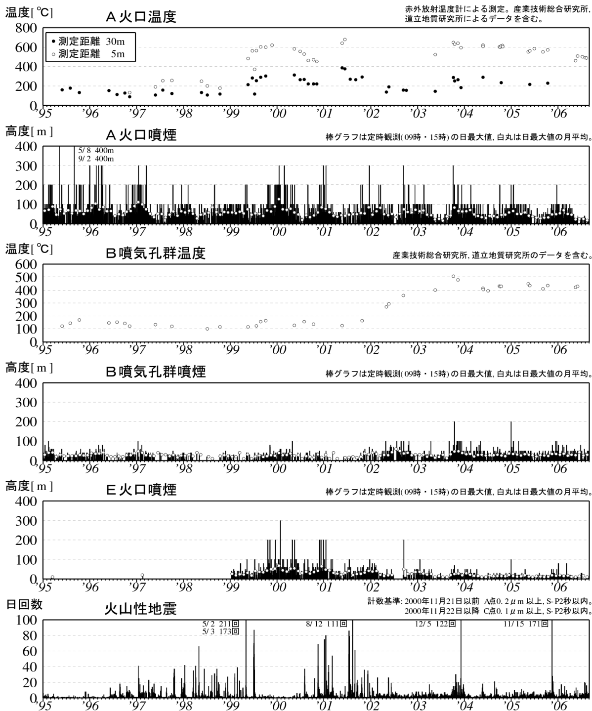
図1 樽前山 最近の火山活動経過図(1995年1月～2006年8月)
