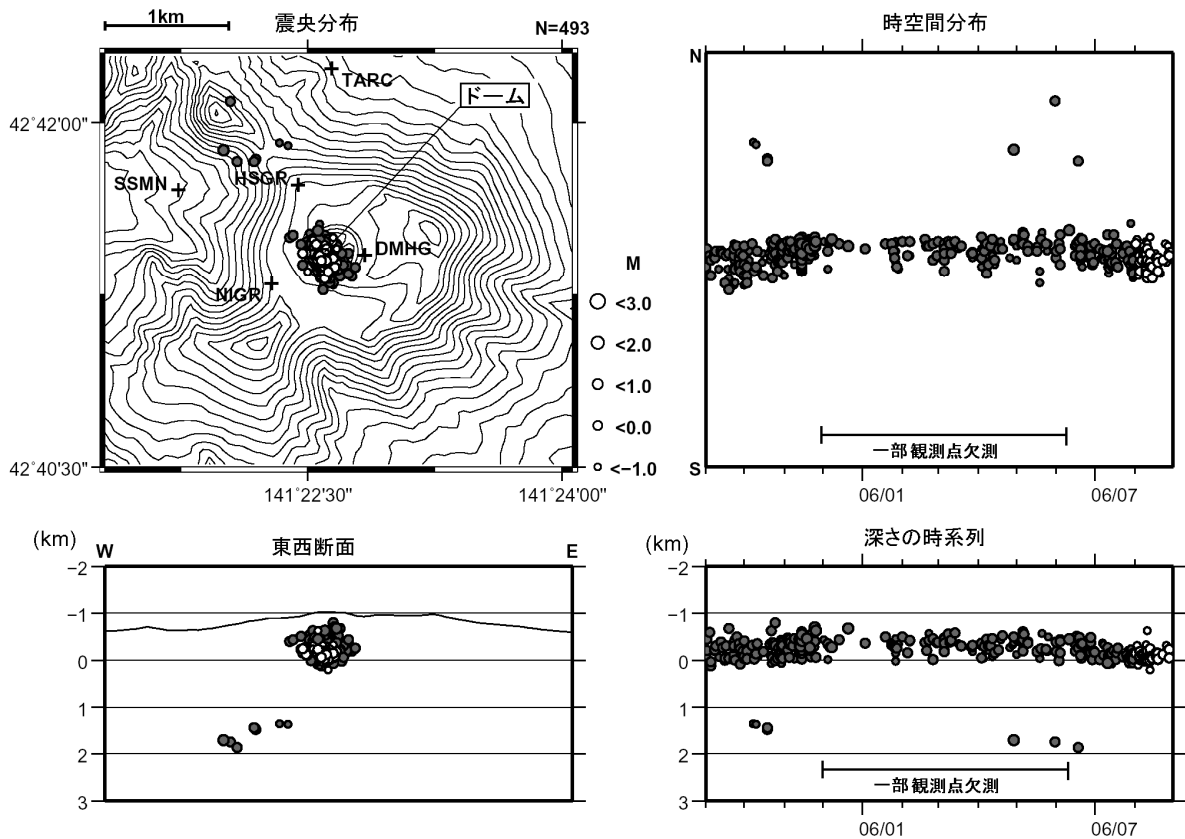
図6 樽前山の震源分布図 (2005年9月~2006年8月、+印: 地震観測点)
