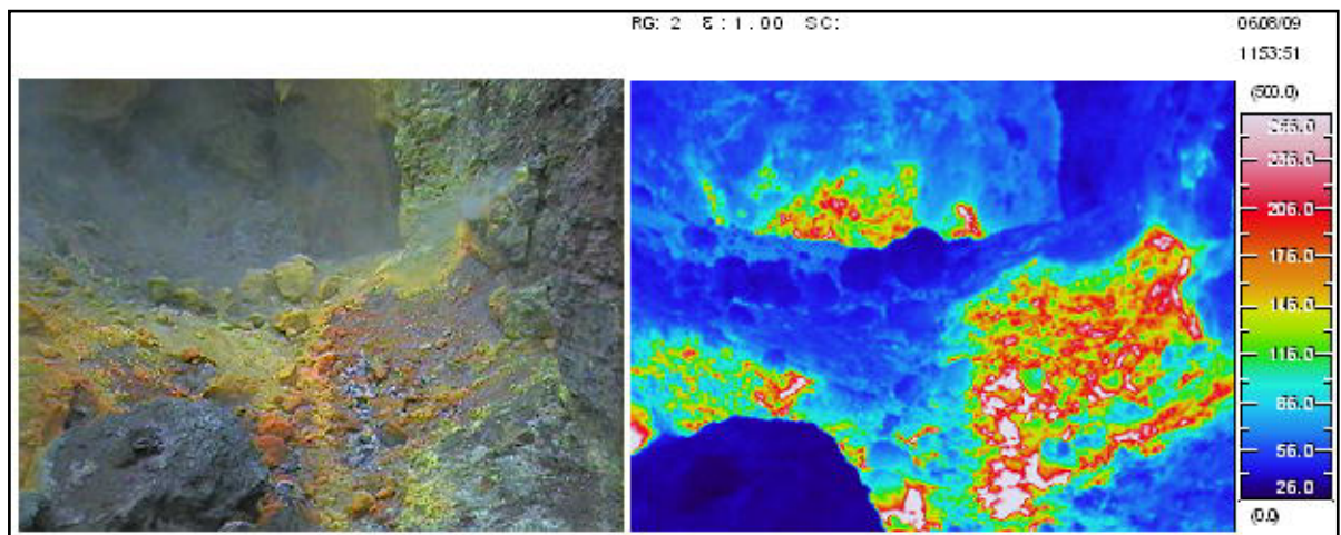
図5 樽前山 南東側から撮影したA火口の表面温度分布(2006 年 8 月 9 日)
