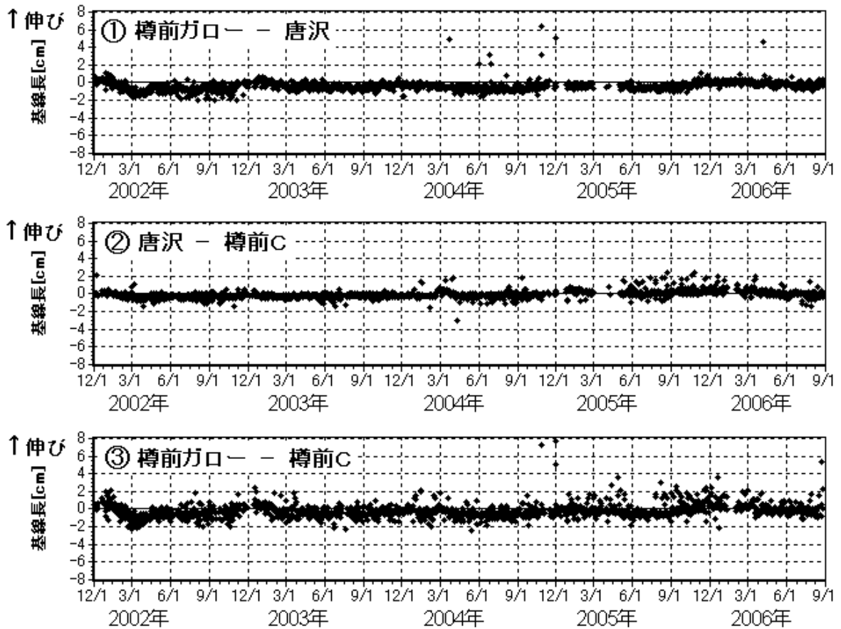
図7 樽前山 基線長変化 (2001 年 12 月～2006 年 8 月) グラフの空白部分は欠測
