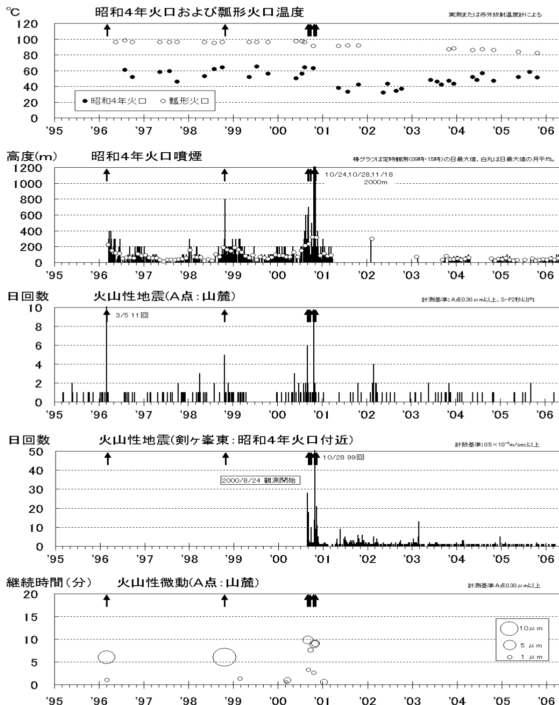
最近の火山活動経過図（1995 年 1 月 1 日～2006 年 4 月 30 日） ↑印は噴火
