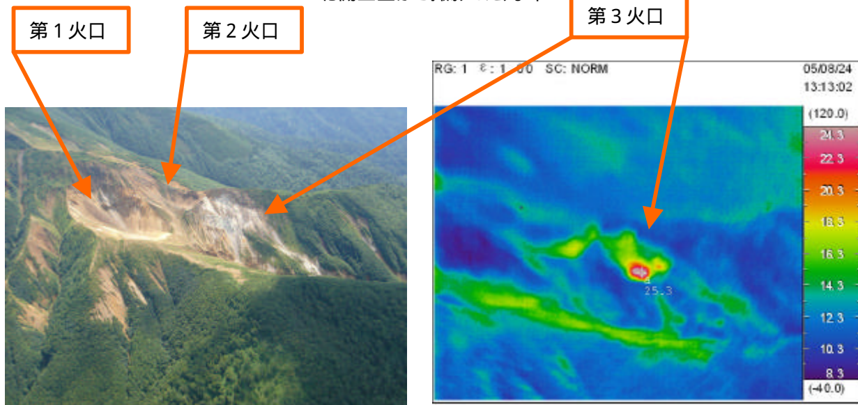
丸山北西山腹の火口列 (北東側上空から撮影)
