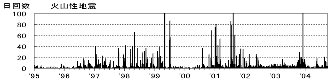
最近の火山活動経過図(1995年1月1日~2004年9月30日)
