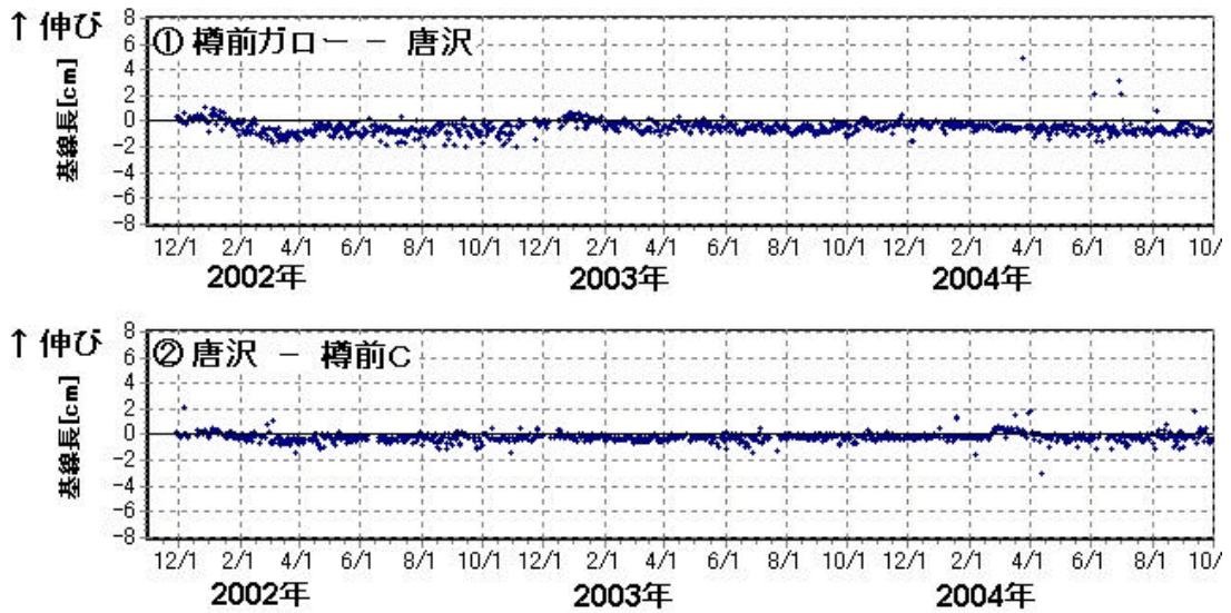
基線長変化 (2001年11月14日~2004年9月30日)
