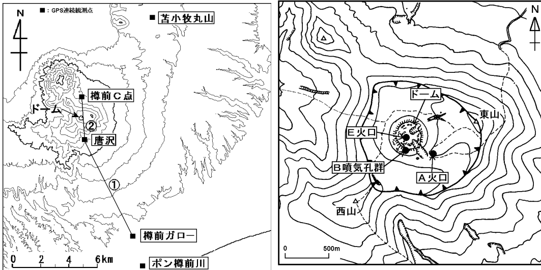
基線長変化 (2001年11月14日~2004年9月30日)
