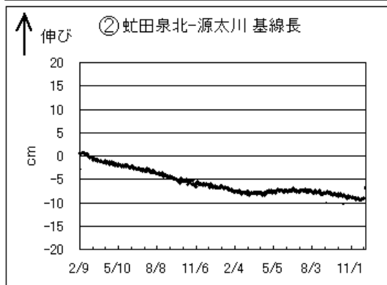
有珠山基線長変化(2001年2月9日~2002年11月30日)
