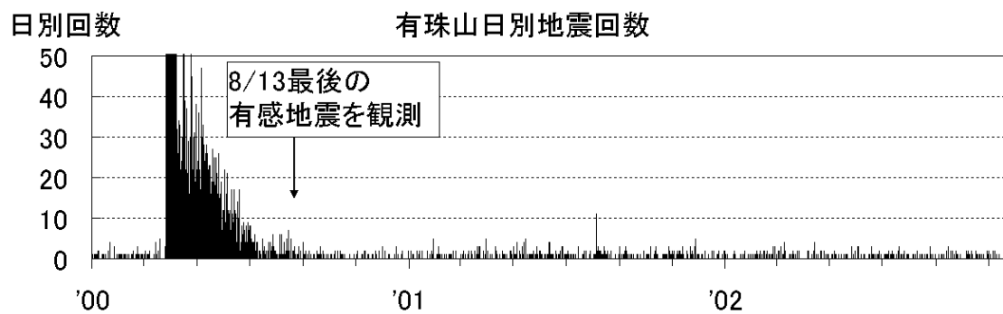
有珠山の火山活動経過図(2000年1月1日~2002年11月30日)
