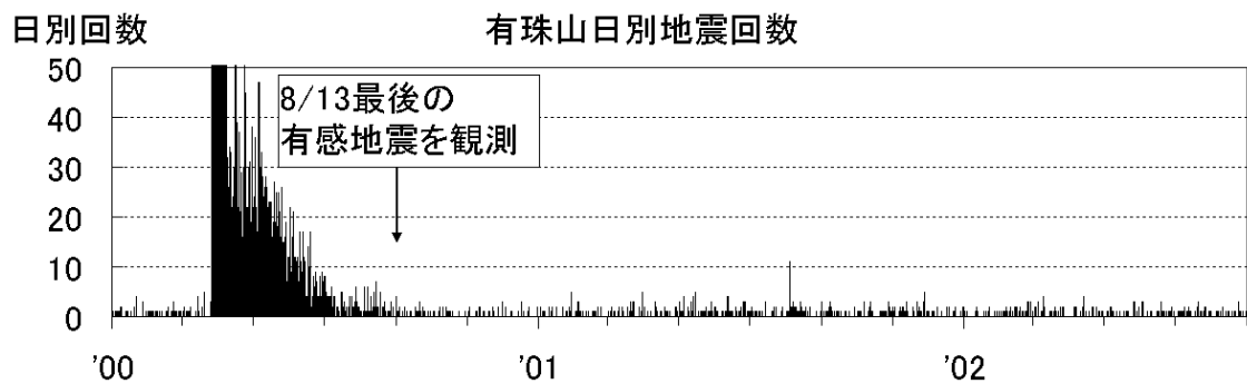
有珠山の火山活動経過図(2000年1月1日~2002年8月31日)
