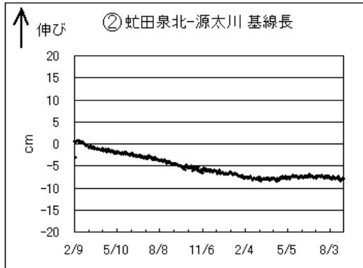
有珠山基線長グラフ（2001年2月9日～2002年8月31日）
