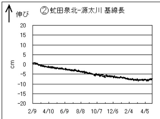
有珠山基線長グラフ（2001 年 2 月 9 日～2002 年 4 月 30 日）
