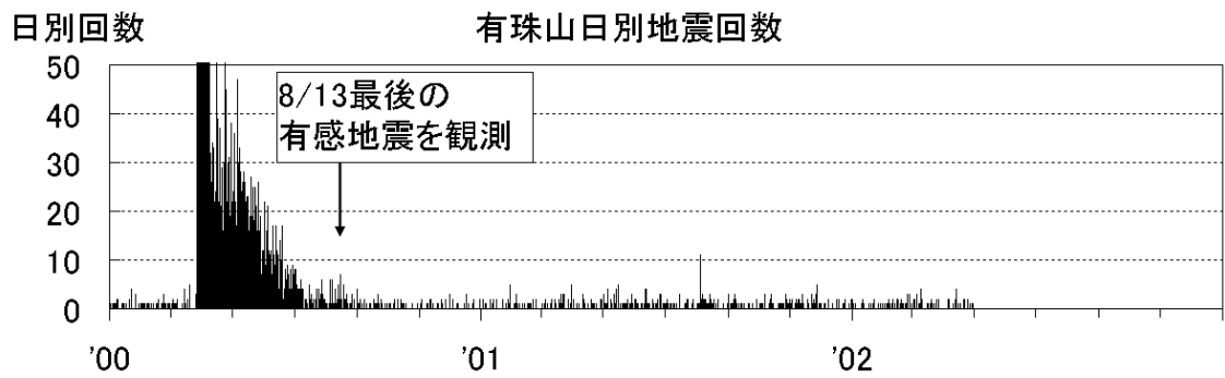
有珠山の火山活動経過図（2000年1月1日～2002年4月30日）
