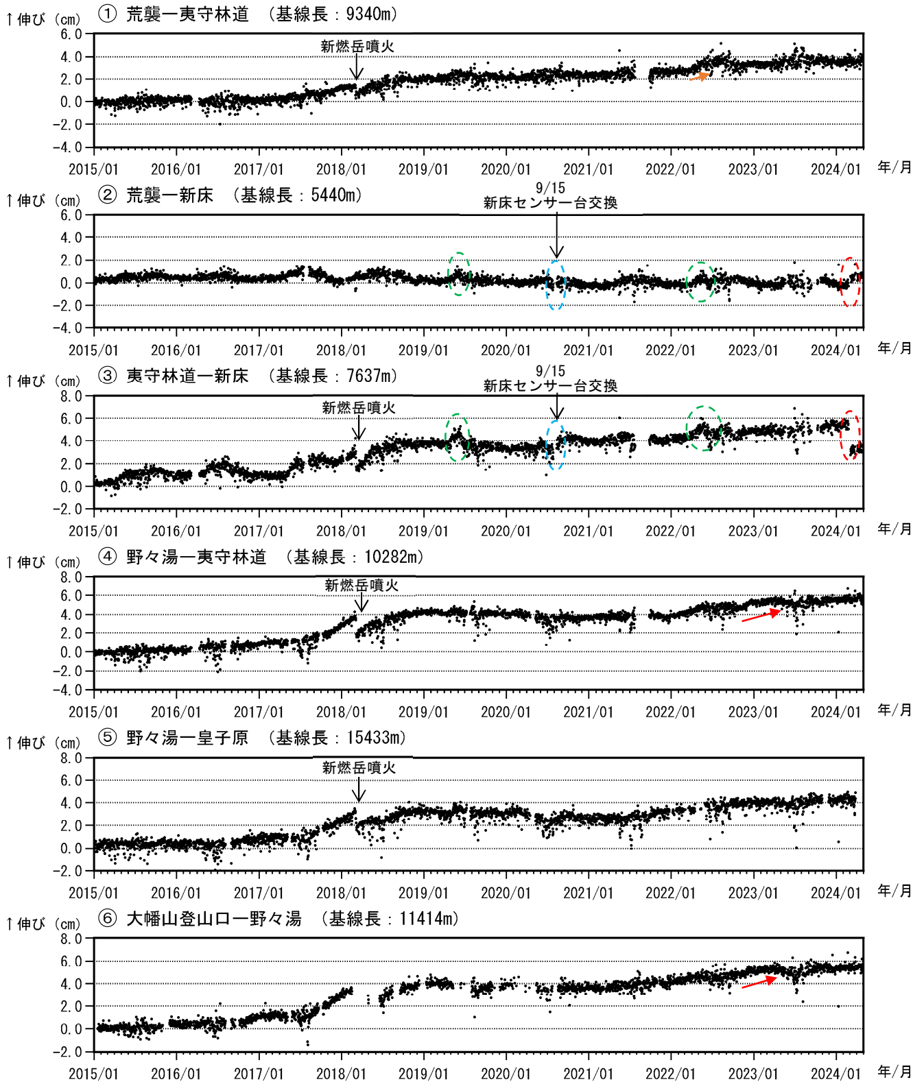
図4 霧島山（新燃岳） GNSS 連続観測による基線長変化（2015年1月～2024年4月）
