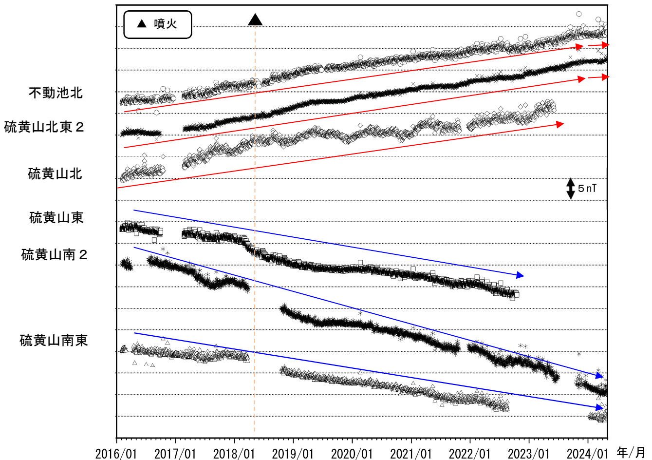
図 8-2 霧島山（えびの高原（硫黄山）周辺） 全磁力観測点で観測された全磁力変動（2016年1月～2024年4月）
