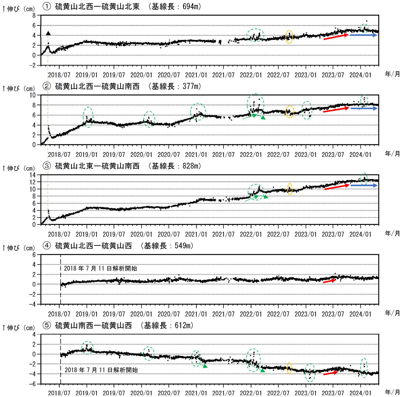
図7 霧島山（えびの高原（硫黄山）周辺） GNSS 連続観測による基線長変化 (2018年3月～2024年4月)
