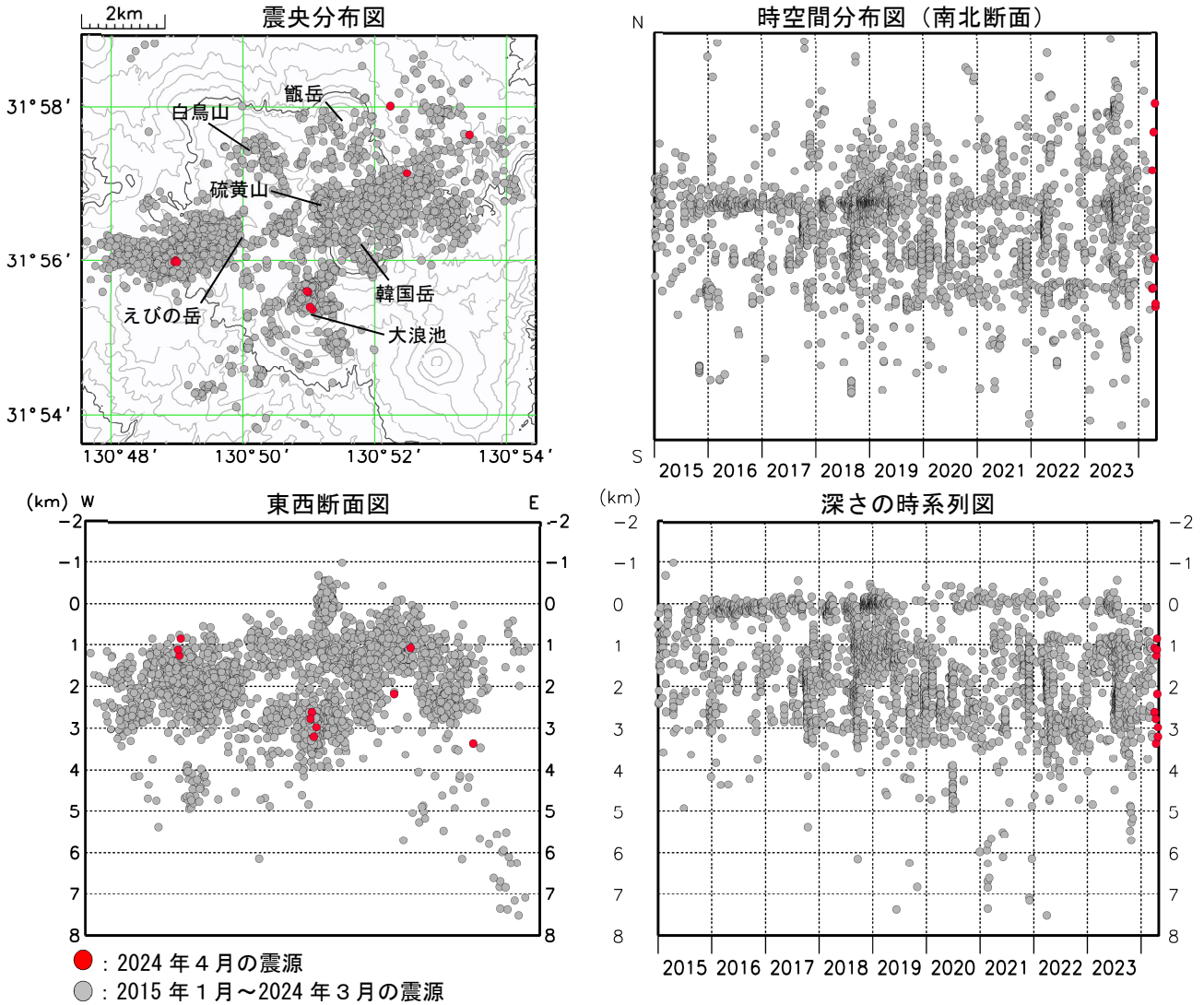
図5 霧島山（えびの高原（硫黄山）周辺） 震源分布図（2015年1月～2024年4月）
