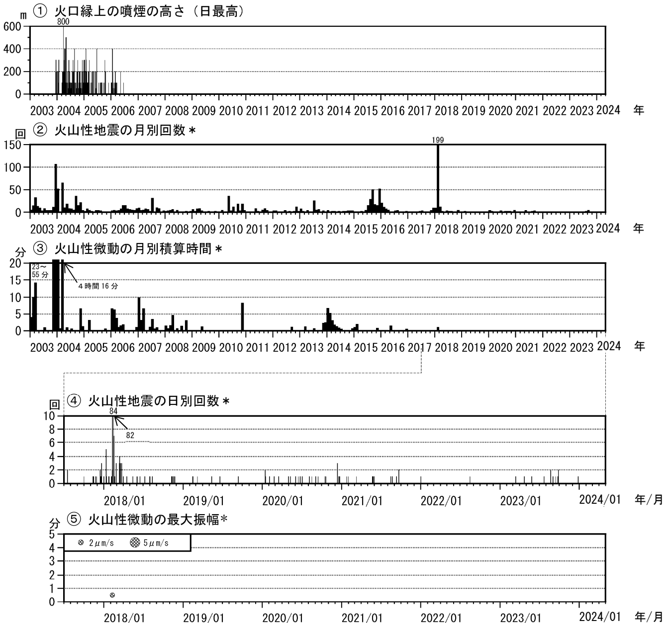
図3 霧島山（御鉢） 火山活動経過図（2003年1月～2024年4月）
