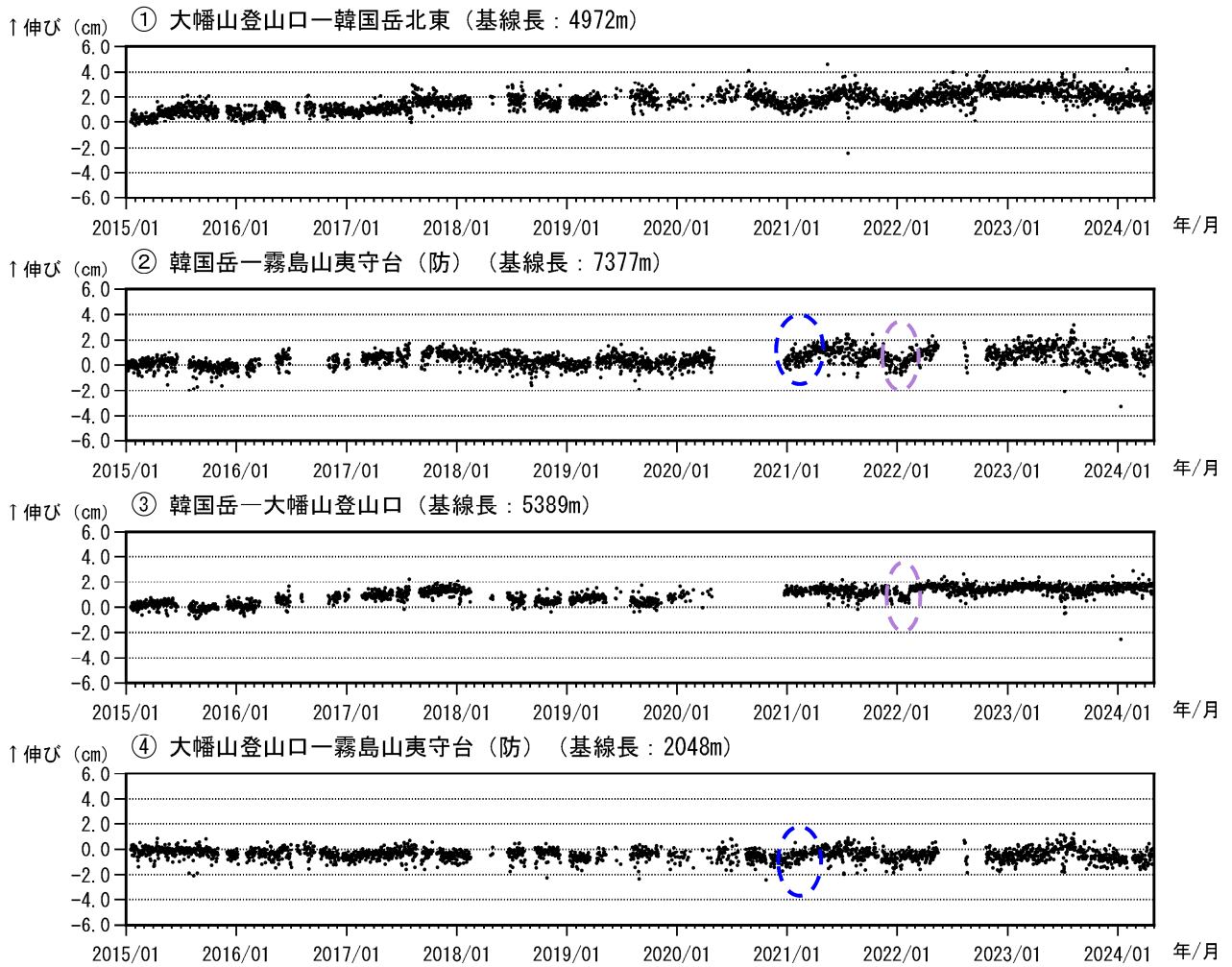
図4 霧島山（大幡池） GNSS 連続観測による基線長変化（2015年1月～2024年4月）
