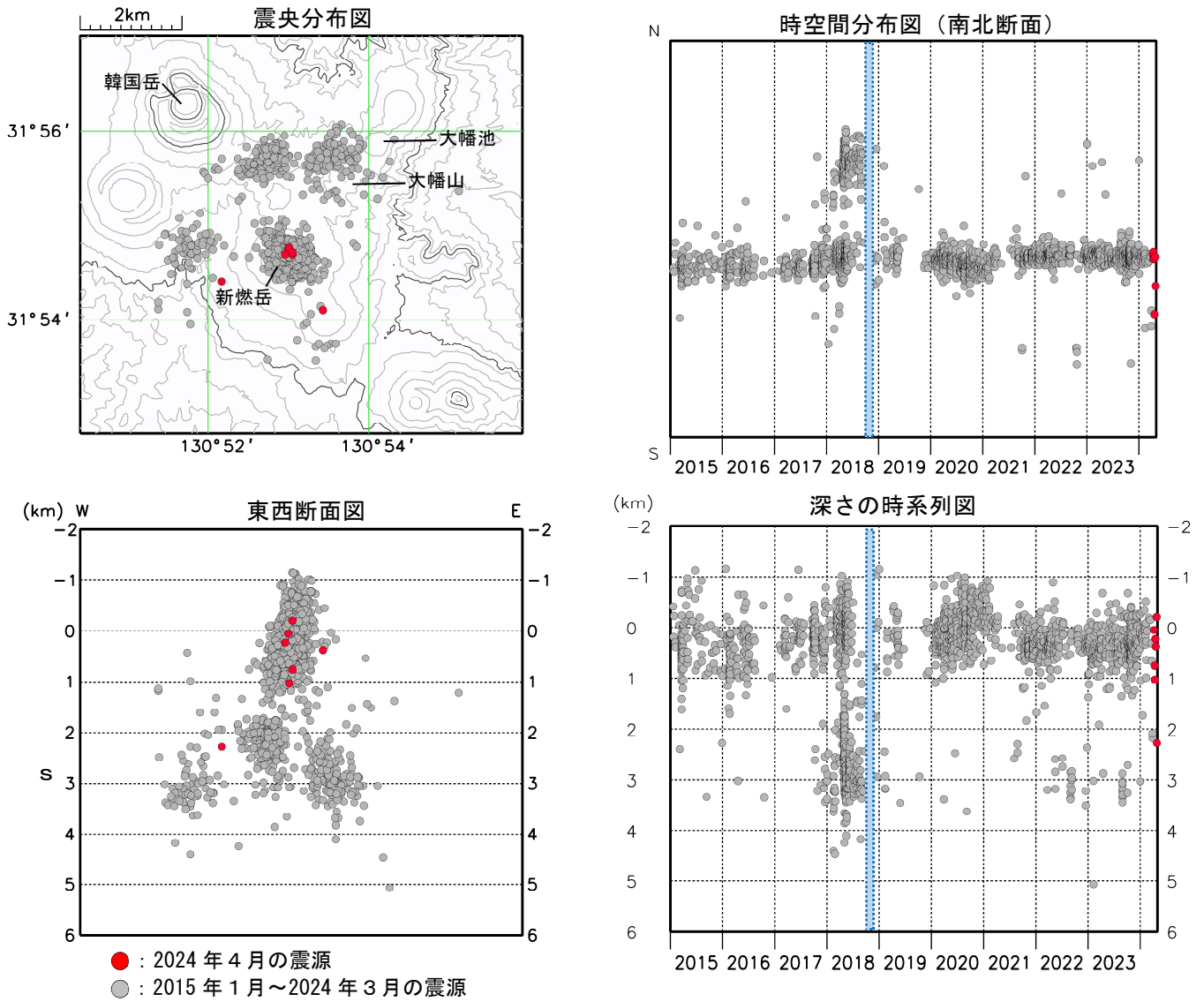
図3 霧島山（新燃岳） 震源分布図（2015年1月～2024年4月）
