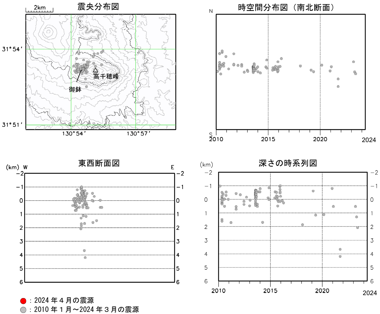
図2 霧島山（御鉢） 震源分布図（2010年1月～2024年4月）
