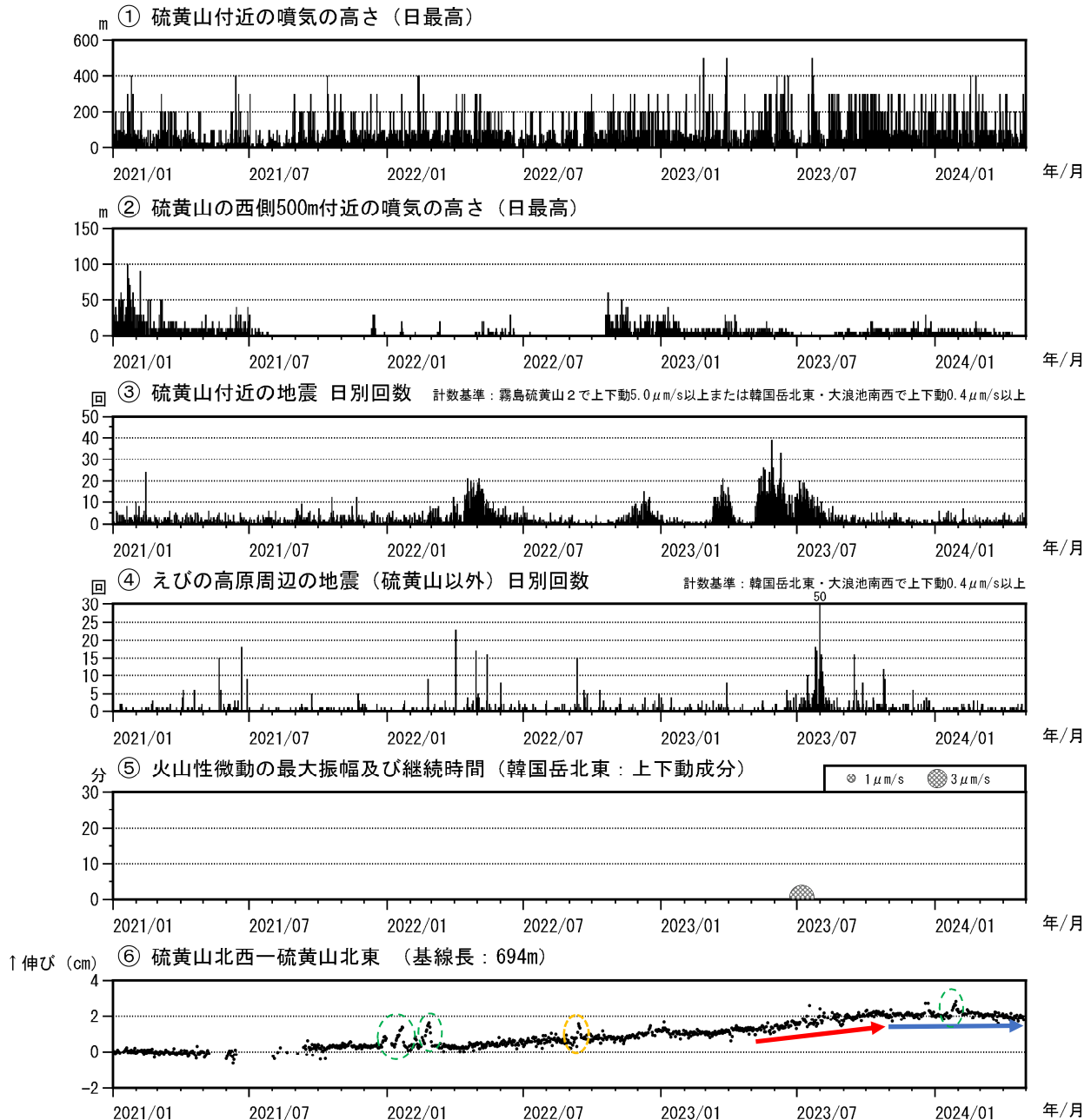
図4 霧島山（えびの高原（硫黄山）周辺）火山活動経過図（2021年1月～2024年4月）
