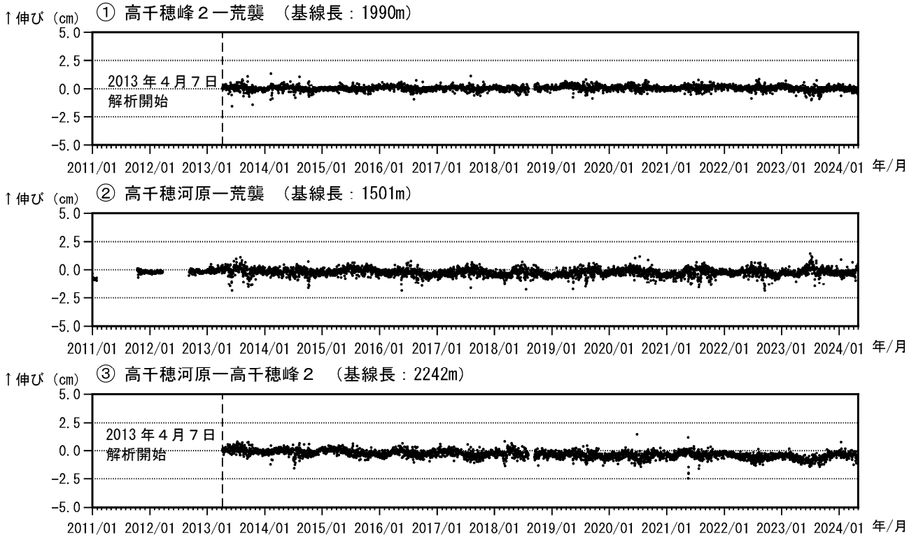
図4 霧島山（御鉢） GNSS 連続観測による基線長変化（2011年1月～2024年4月）
