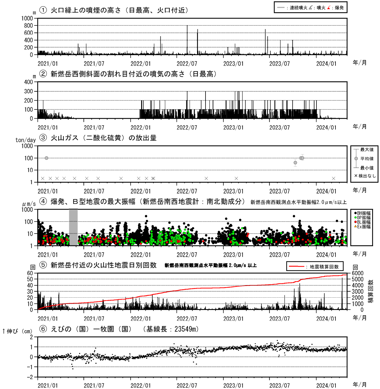
図2 霧島山（新燃岳） 火山活動経過図（2021年1月～2024年4月）
