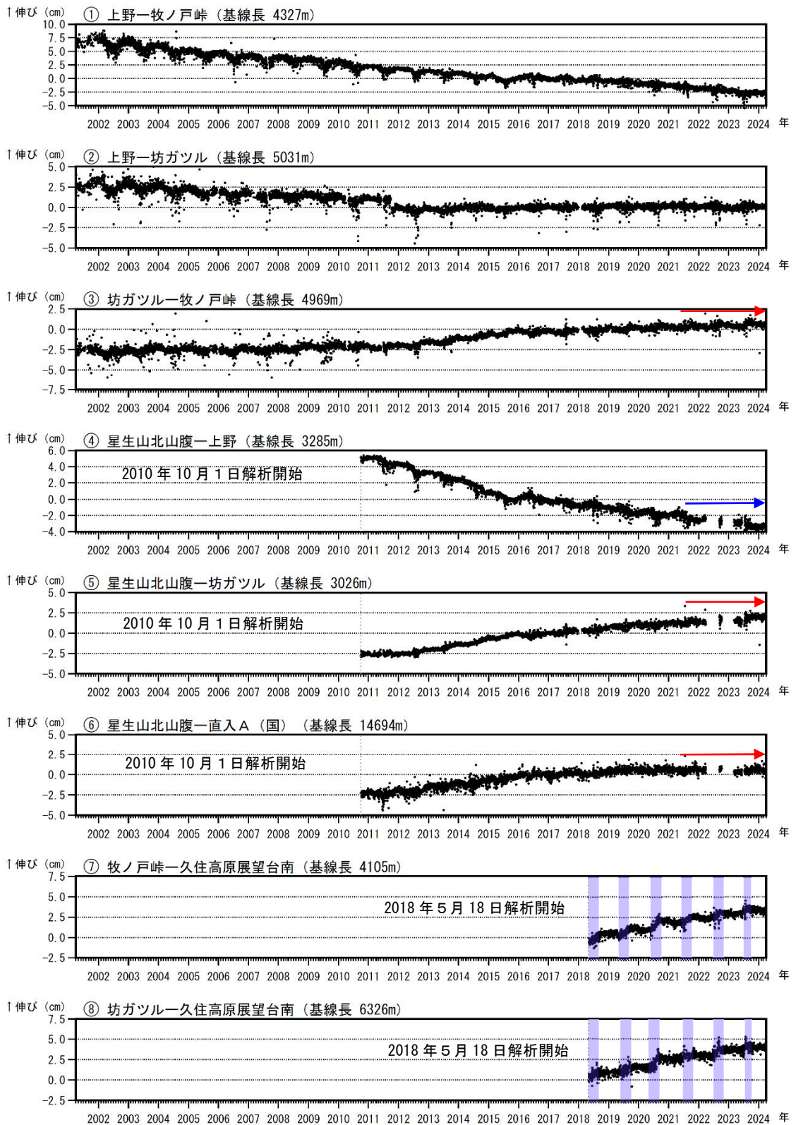
図6 九重山 GNSS連続観測による基線長変化（2001年4月～2024年3月）
