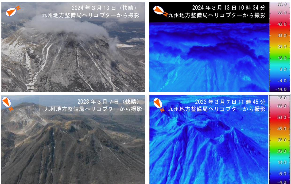
図 2-2 九重山 硫黄山周辺の状況（3月13日、九州地方整備局の協力により実施）
