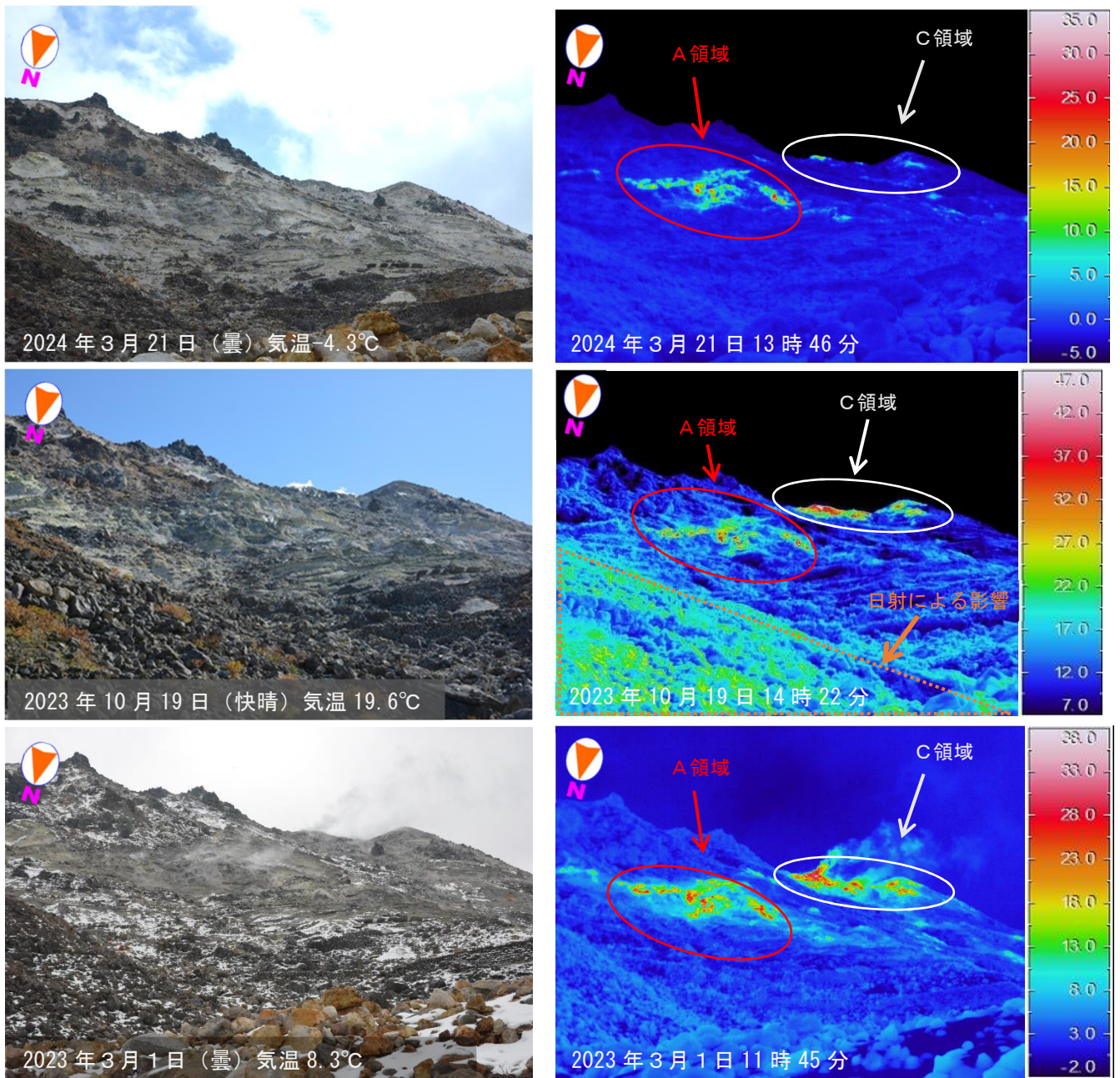
図 2-3 九重山 噴気地帯 A, C 領域の可視画像及び赤外熱映像装置による地表面温度分布（3 月 21 日）
