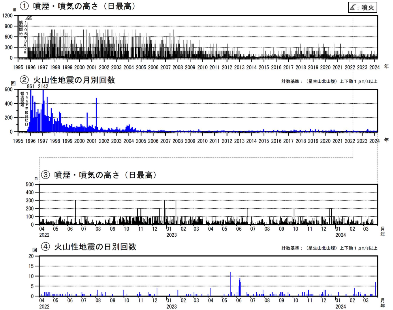
図3 九重山 火山活動経過図（1995年1月～2024年3月）
