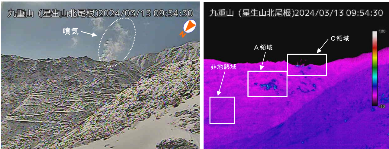
図 1-1 九重山 硫黄山の噴気及び地熱域の状況（3月13日 星生山北尾根監視カメラ）
