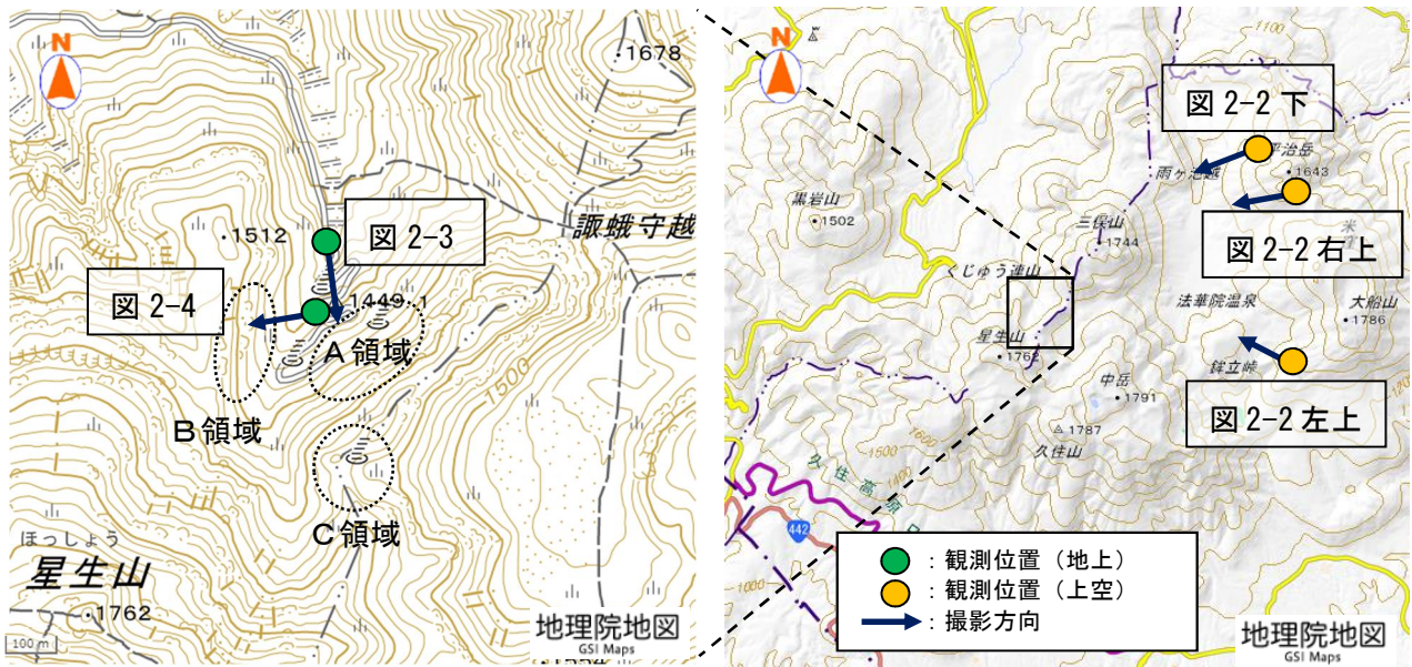
図 2-1 九重山 現地調査観測位置及び撮影方向
