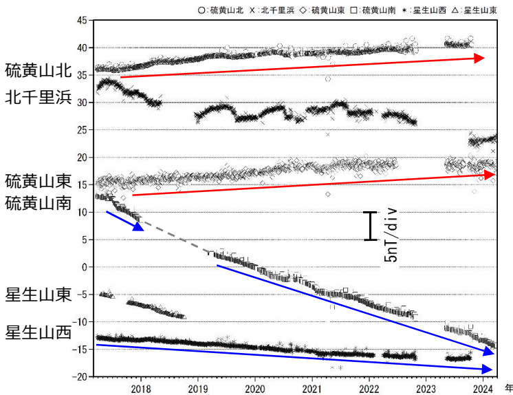
図 5-1 九重山 連続観測による全磁力の変化 (2017年3月～2024年3月)
