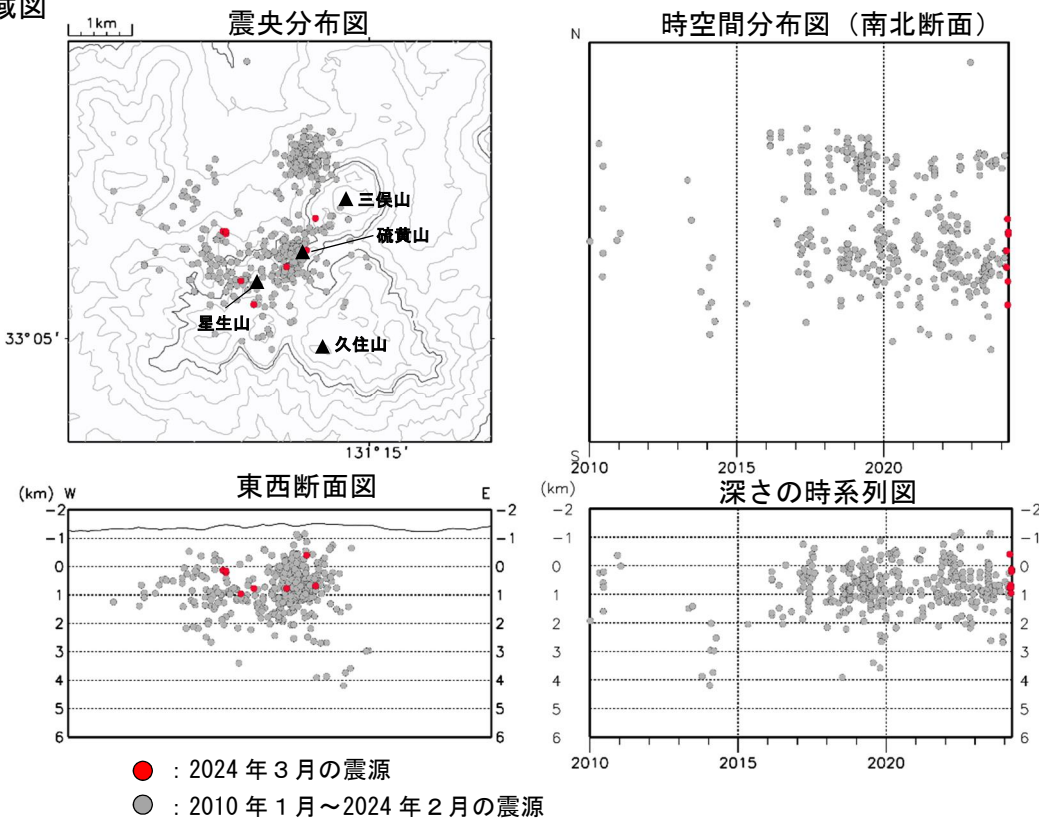
図4 九重山 震源分布図 ①広域図 ②狭域図 (2010年1月～2024年3月)
