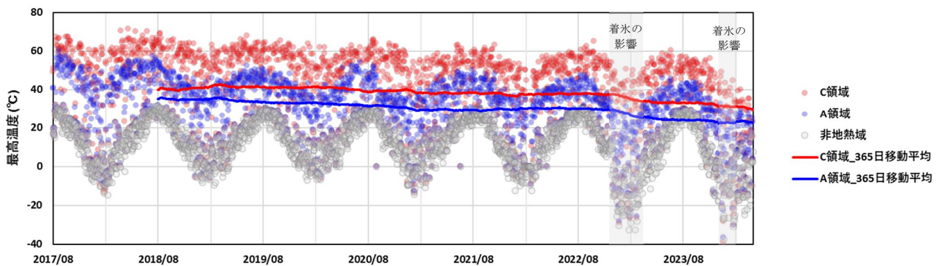
図 1-2 九重山 星生山北尾根の赤外熱映像装置による日別最高温度（2017年8月～2024年3月）
