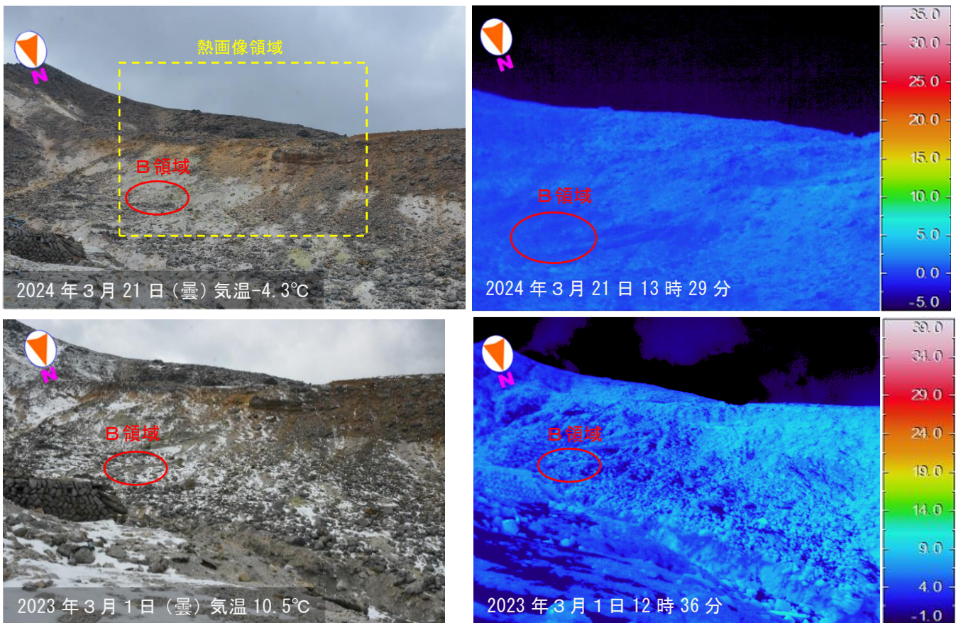
図2-4 九重山 B領域の可視画像及び地表面温度分布（3月21日）
