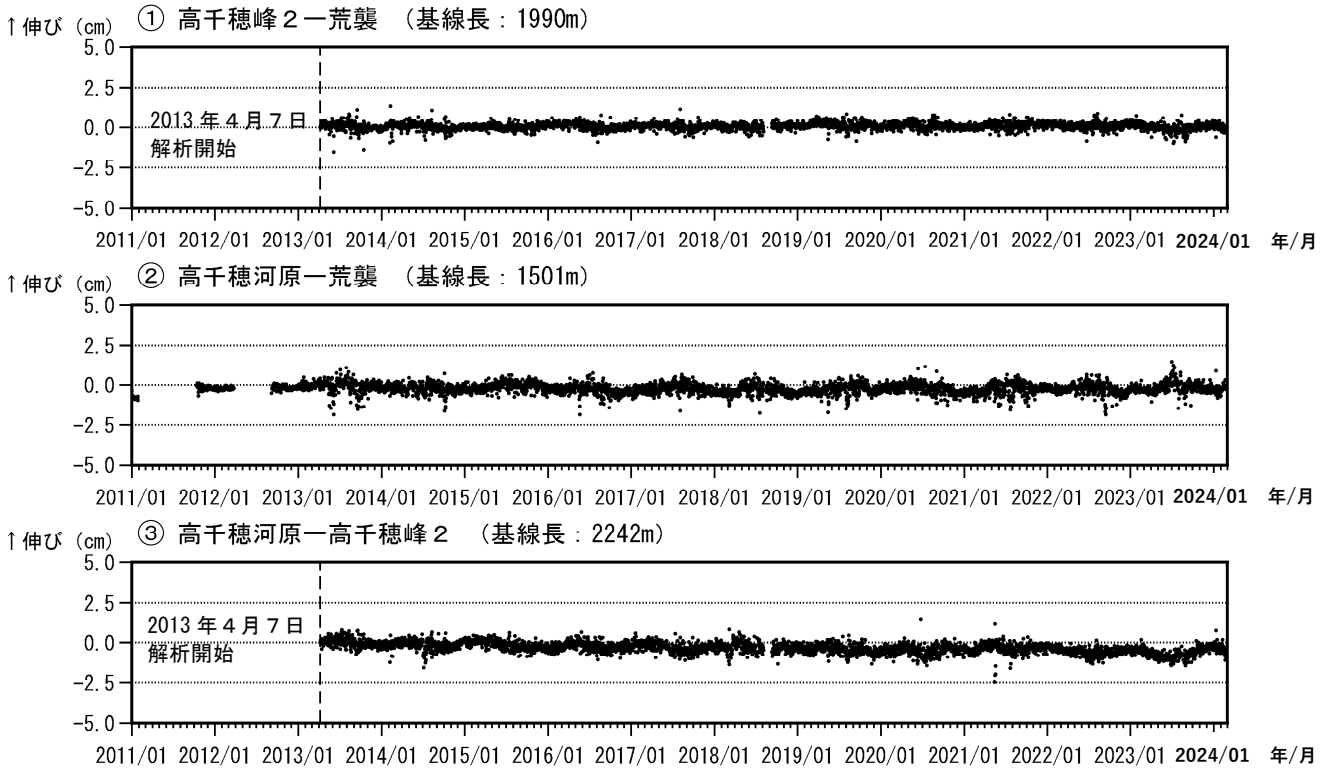
図4 霧島山（御鉢） GNSS連続観測による基線長変化（2011年1月～2024年2月）
