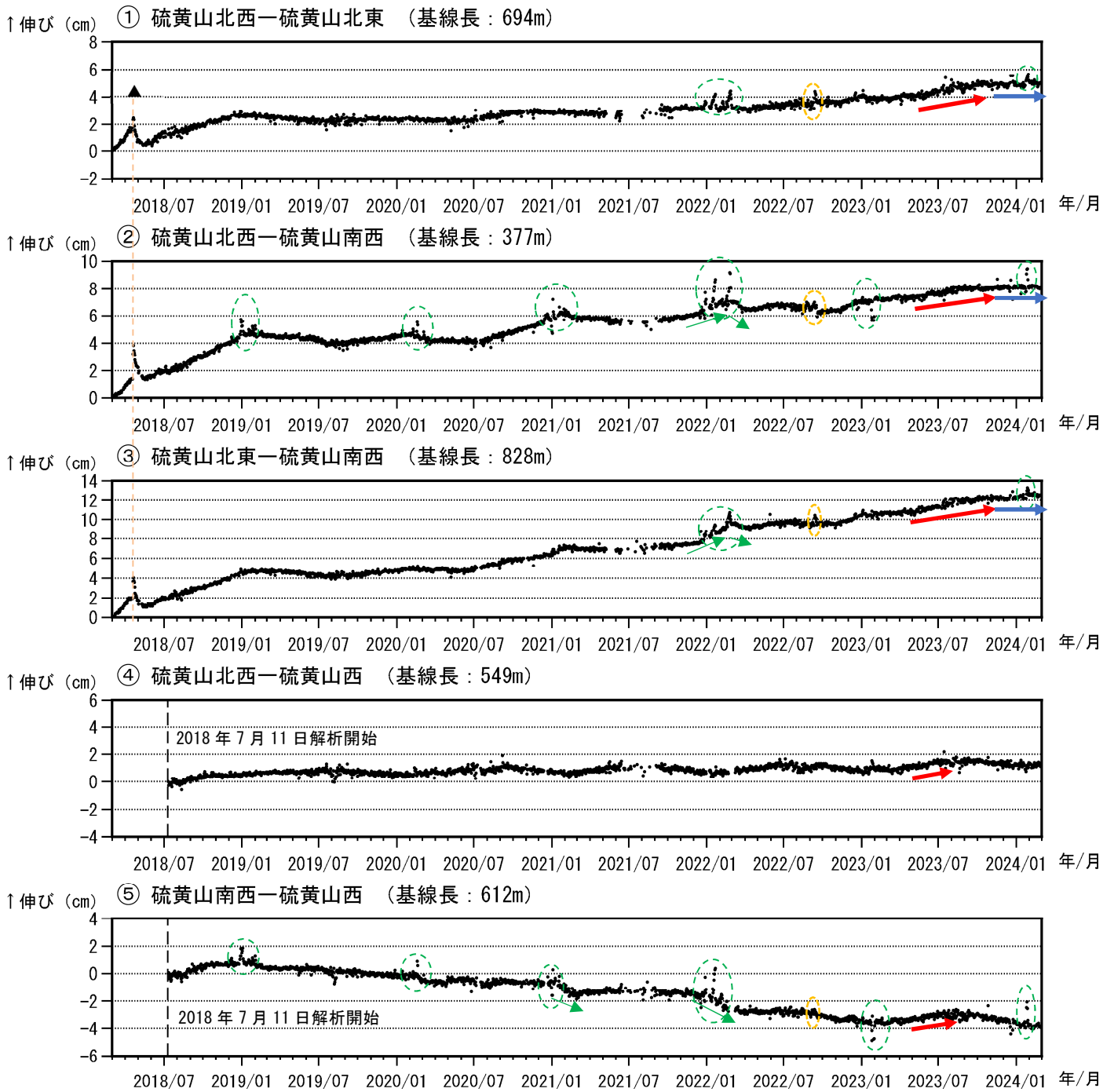
図5 霧島山（えびの高原（硫黄山）周辺） GNSS 連続観測による基線長変化 （2018年3月～2024年2月）
