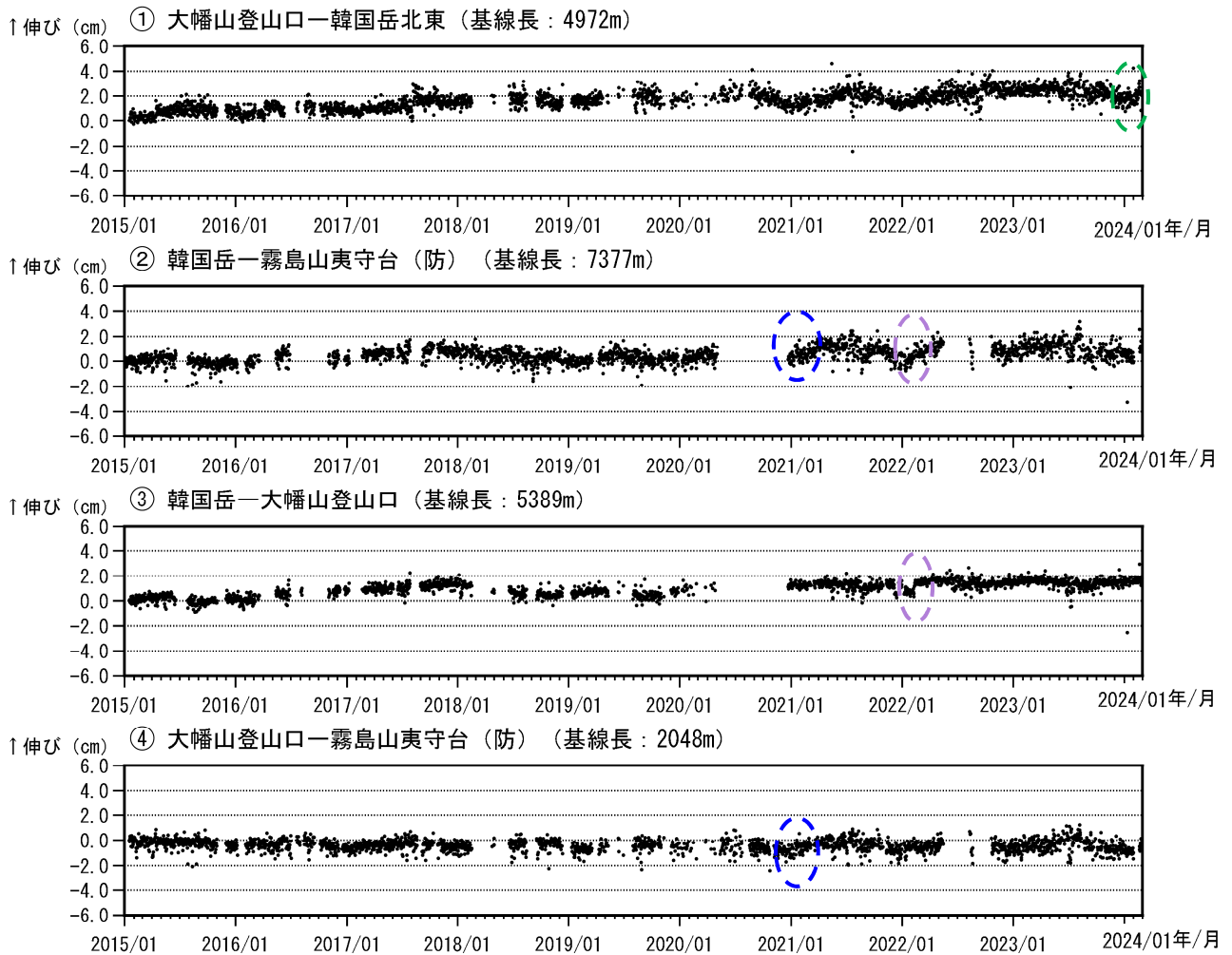
図4 霧島山（大幡池） GNSS 連続観測による基線長変化（2015年1月～2024年2月）
