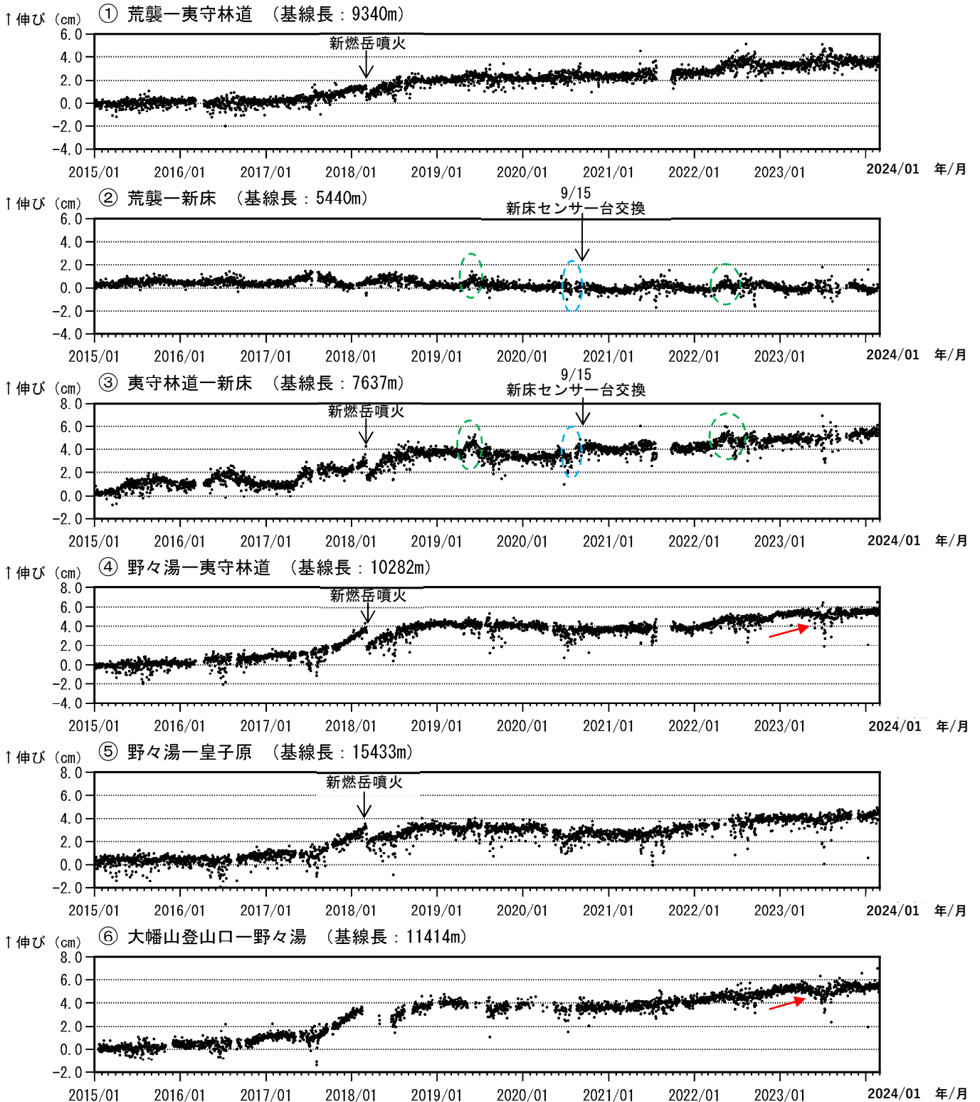
図4 霧島山(新燃岳) GNSS連続観測による基線長変化(2015年1月~2024年2月)
