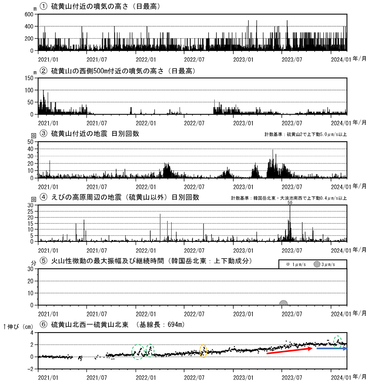
図2 霧島山（えびの高原（硫黄山）周辺）火山活動経過図（2021年1月～2024年2月）
