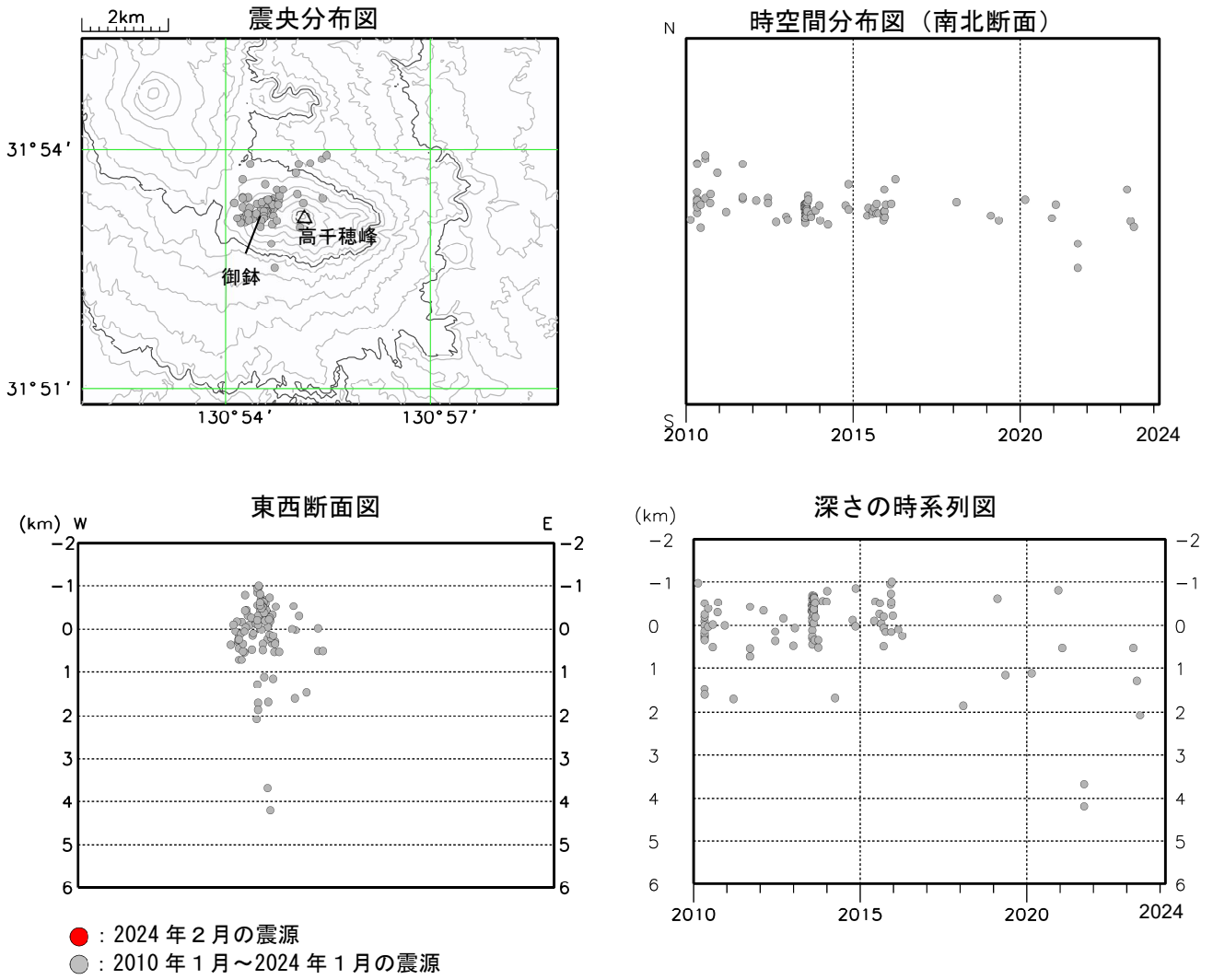
図2 霧島山（御鉢） 震源分布図（2010年1月～2024年2月）
