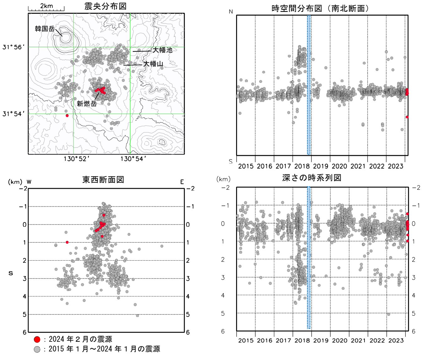
図3 霧島山（新燃岳） 震源分布図（2015年1月～2024年2月）
