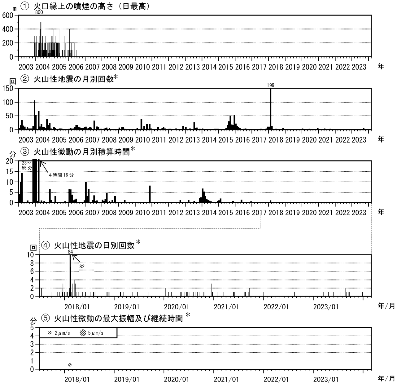
図3 霧島山（御鉢） 火山活動経過図（2003年1月～2024年2月）
