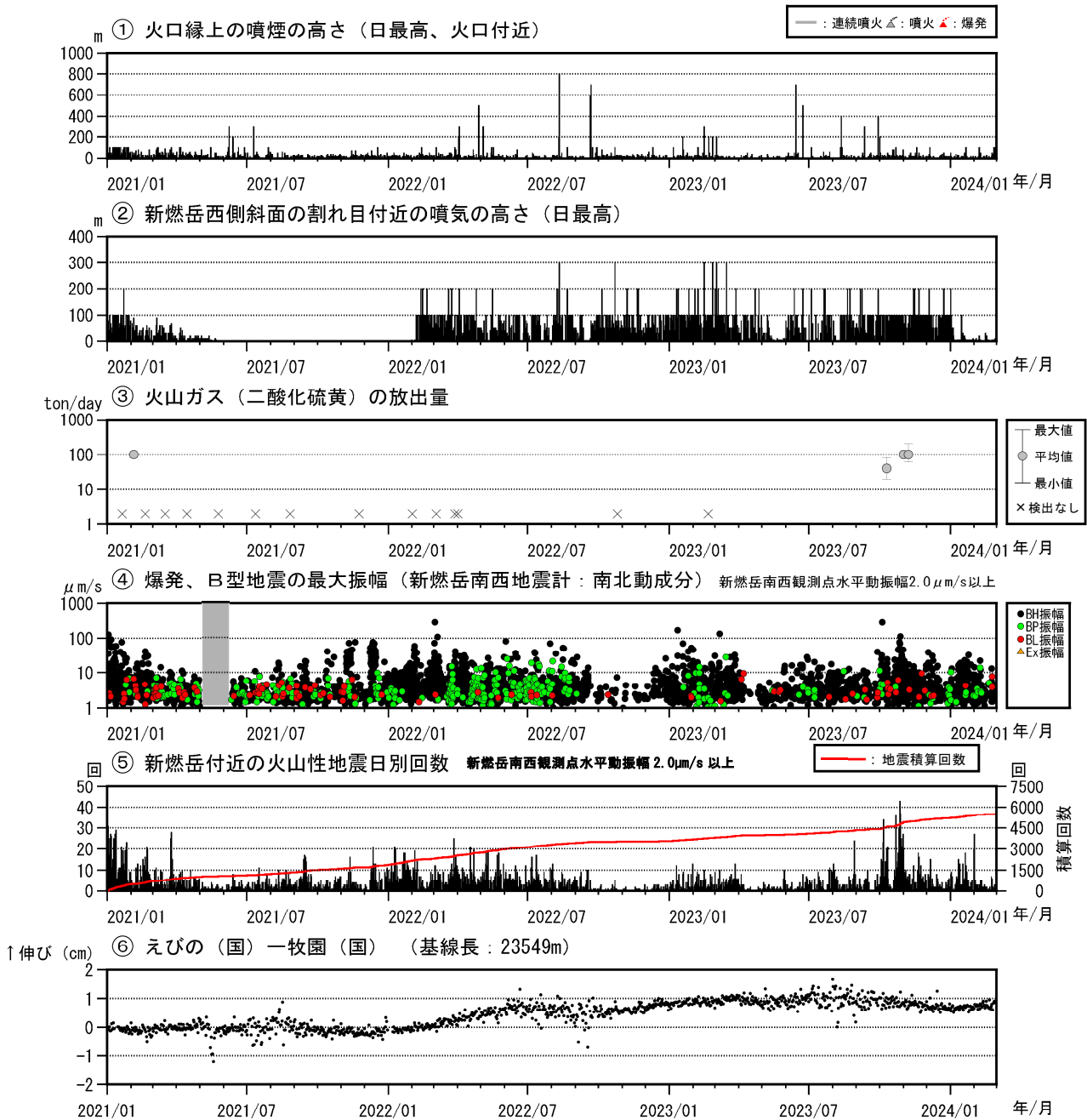
図2 霧島山（新燃岳） 火山活動経過図（2021年1月～2024年2月）
