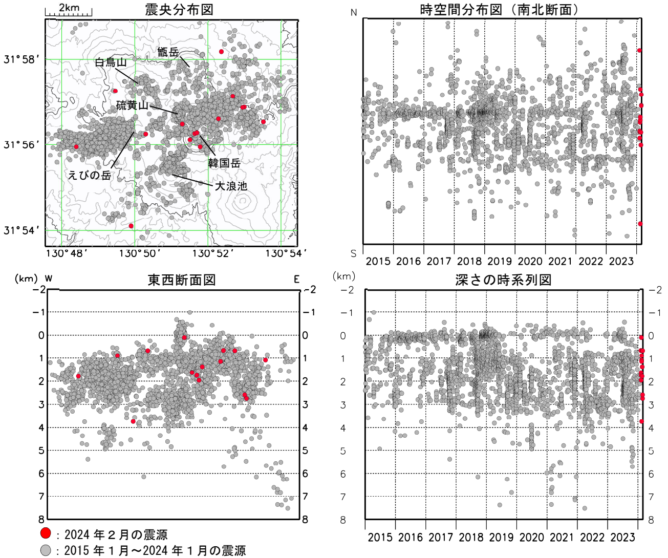
図3 霧島山（えびの高原（硫黄山）周辺） 震源分布図（2015年1月～2024年2月）
