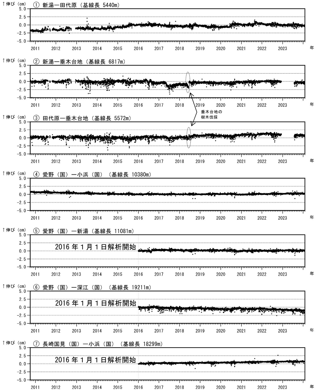
図4 雲仙岳 GNSS連続観測による基線長変化（2010年10月～2024年1月）
