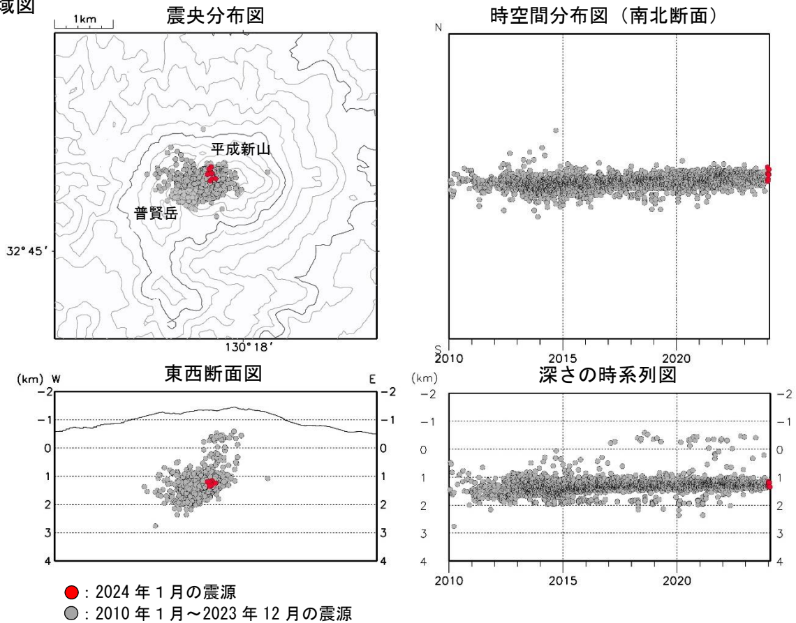
図3 雲仙岳 震源分布図 ①広域図 ②狭域図 (2010年1月～2024年1月)
