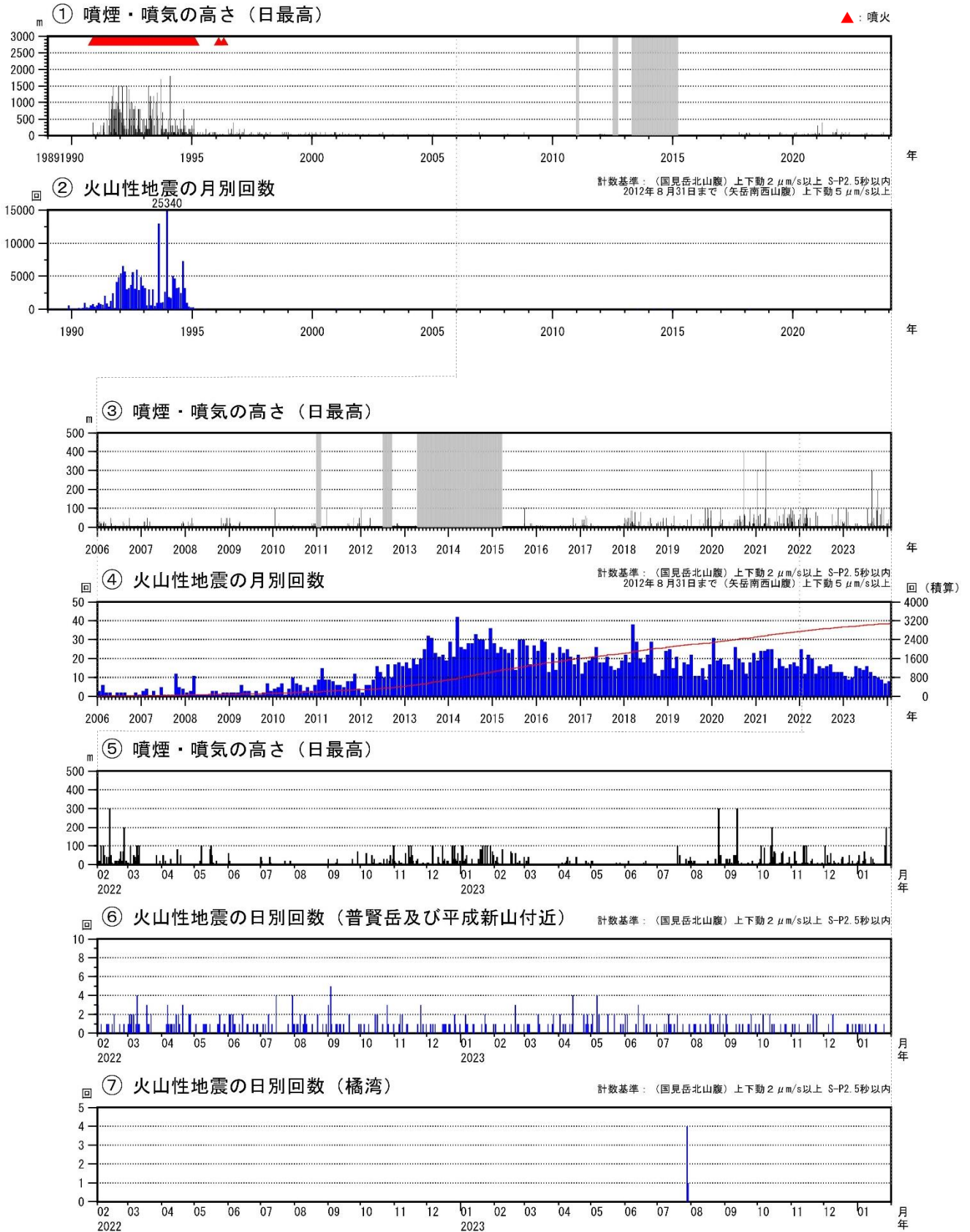
図2 雲仙岳 火山活動経過図（1989年1月～2024年1月）
