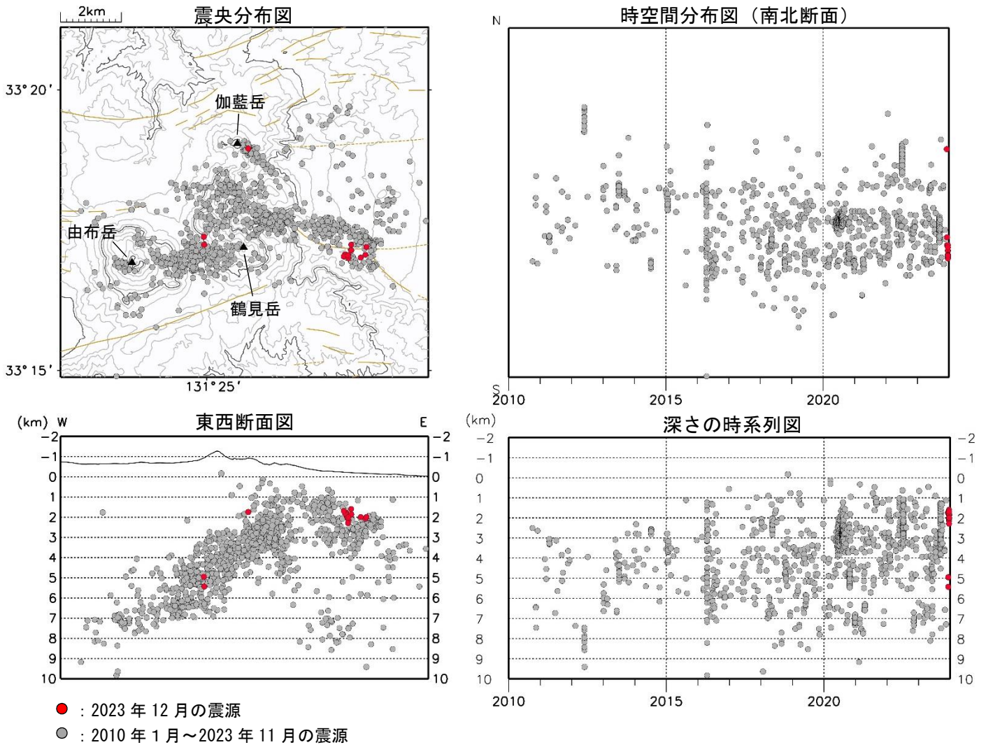
図3 鶴見岳・伽藍岳 震源分布図（2010年1月～2023年12月）
