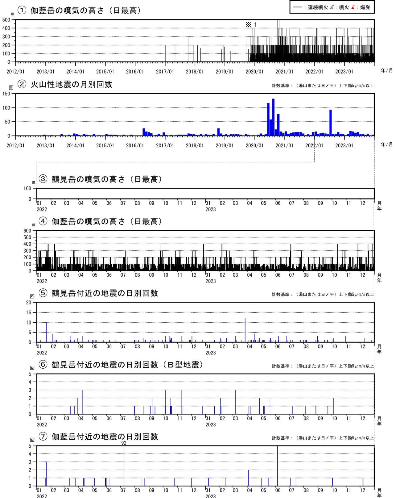
図2 鶴見岳・伽藍岳 火山活動経過図（2012年1月～2023年12月）
