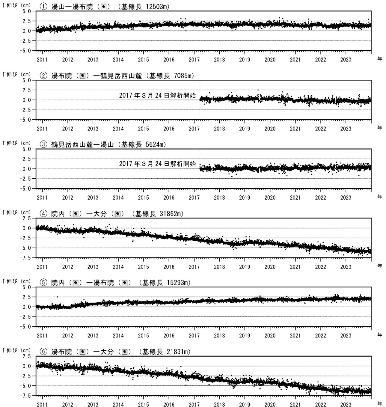
図4 鶴見岳・伽藍岳 GNSS連続観測による基線長変化（2010年10月～2023年12月）
