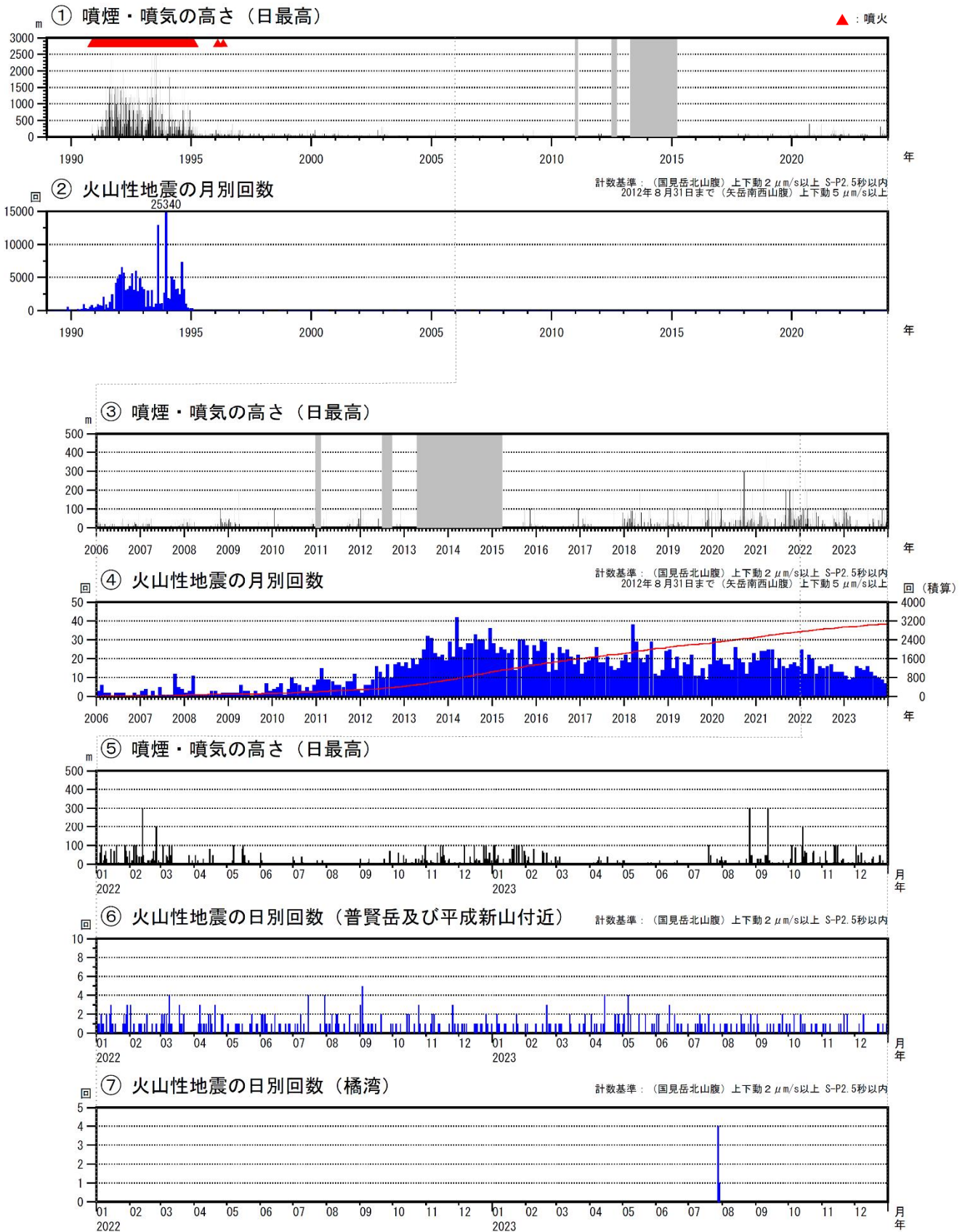
図2 雲仙岳 火山活動経過図（1989年1月～2023年12月）
