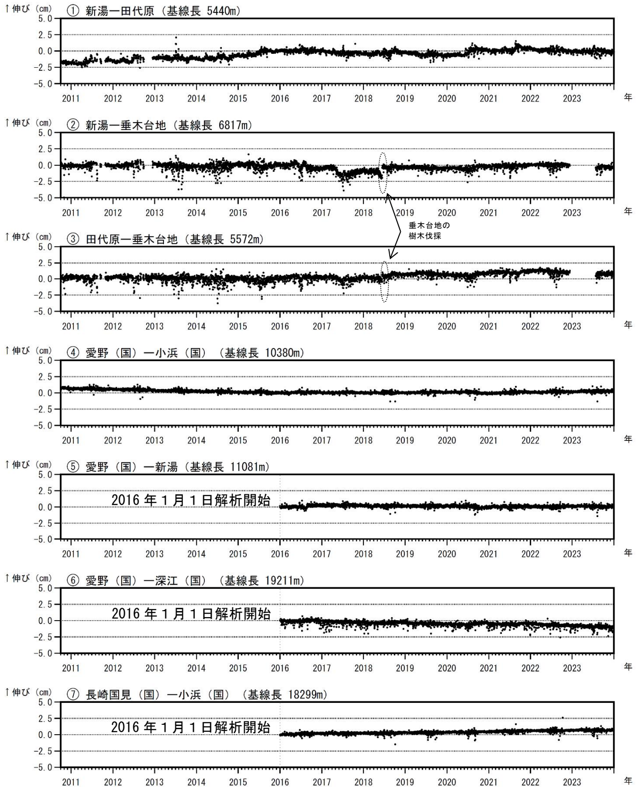
図4 雲仙岳 GNSS連続観測による基線長変化 (2010年10月～2023年12月)
