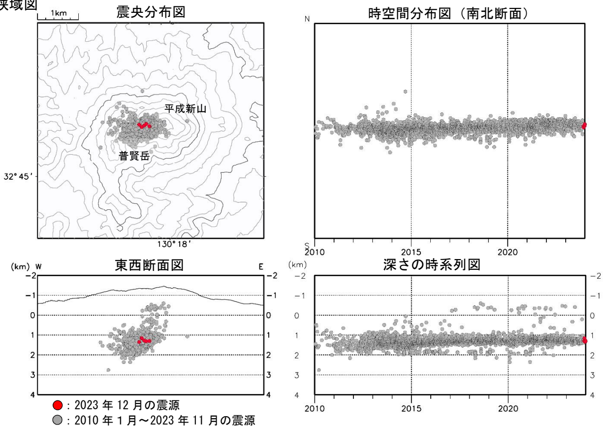
図3 雲仙岳 震源分布図 ①広域図 ②狭域図 (2010年1月～2023年12月)
