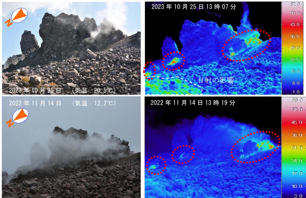
図 3-1 赤外熱映像装置による平成新山の地表面温度分布および可視画像（平成新山山腹から観測） ・前回（2022年11月14日）の観測と同様に、平成新山の山頂部に複数箇所に地熱域（図中赤丸）を確認しましたが、地熱域の分布や温度に特段の変化は認められませんでした。 ・前回の観測と同様に、山頂付近から弱い噴気が上がっているのを確認しました。
