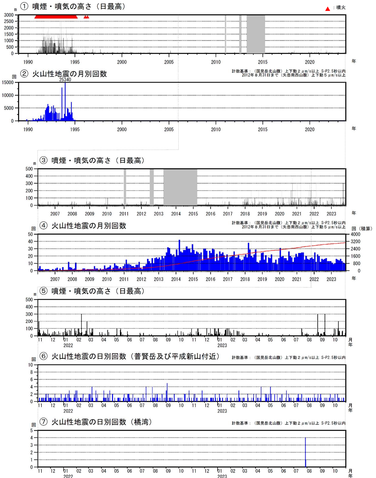
図4 雲仙岳 火山活動経過図（1989年1月～2023年10月）
