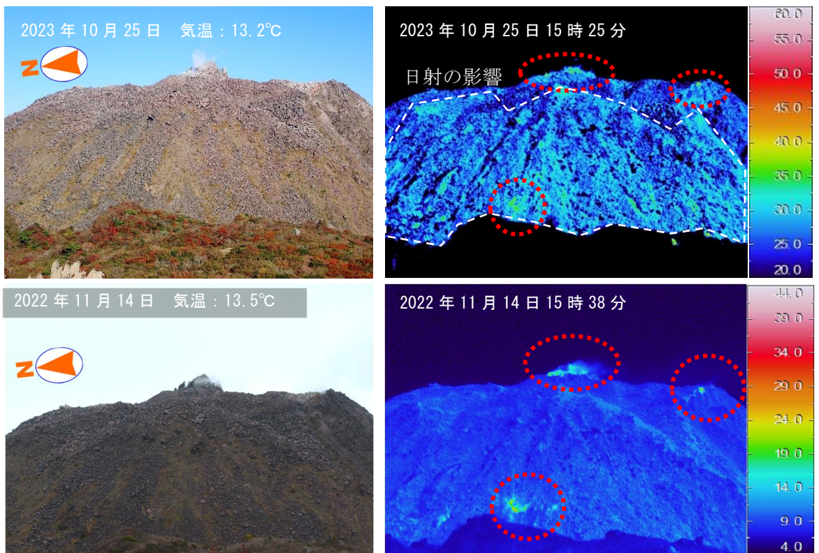
図 3-2 赤外熱映像装置による平成新山の地表面温度分布および可視画像（普賢岳山頂から観測） ・前回（2022年11月14日）の観測と同様に、平成新山の山腹と山頂部の複数箇所に地熱域（図中赤丸）を確認しましたが、特段の変化は認められませんでした。 ・前回の観測と同様に、山頂付近から弱い噴気が上がっているのを確認しました。
