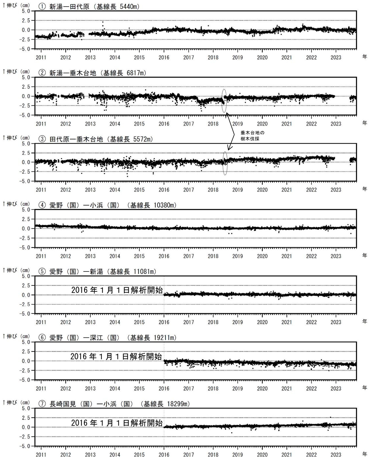
図6 雲仙岳 GNSS連続観測による基線長変化（2010年10月～2023年10月）
