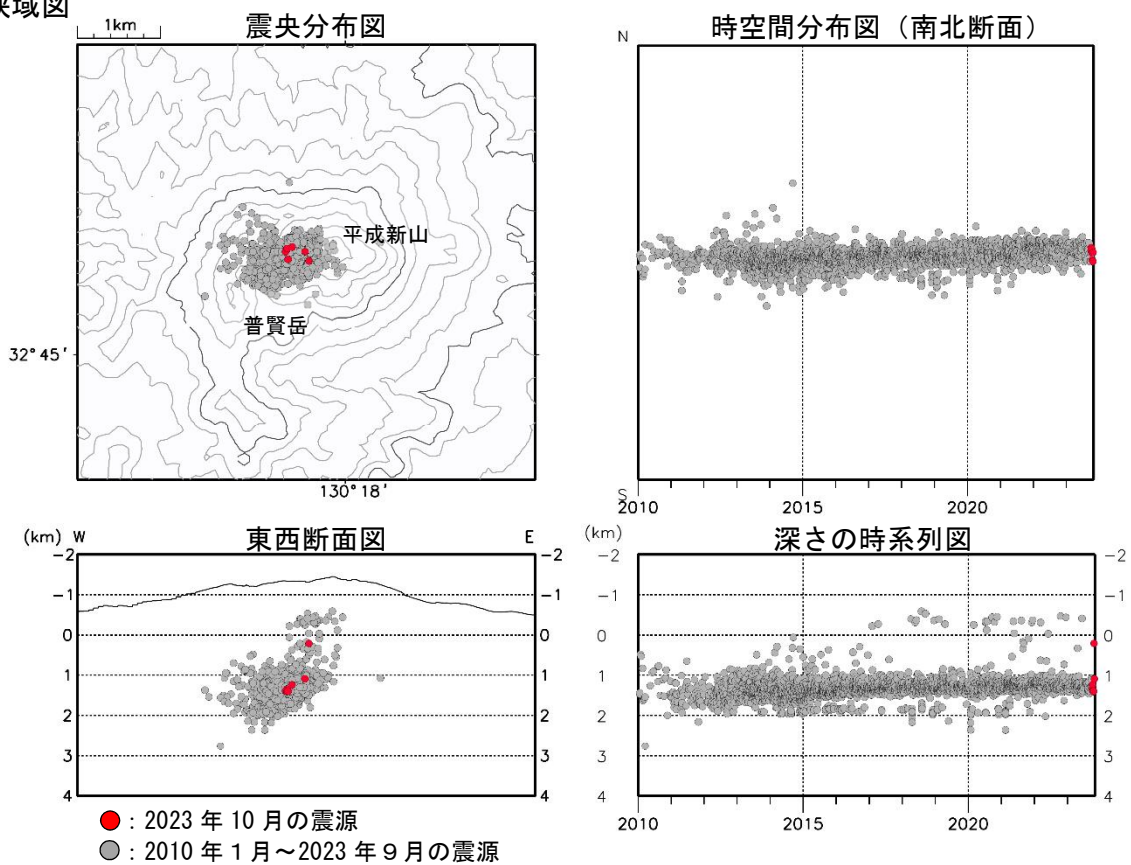
図5 雲仙岳 震源分布図 ①広域図 ②狭域図 (2010年1月～2023年10月)
