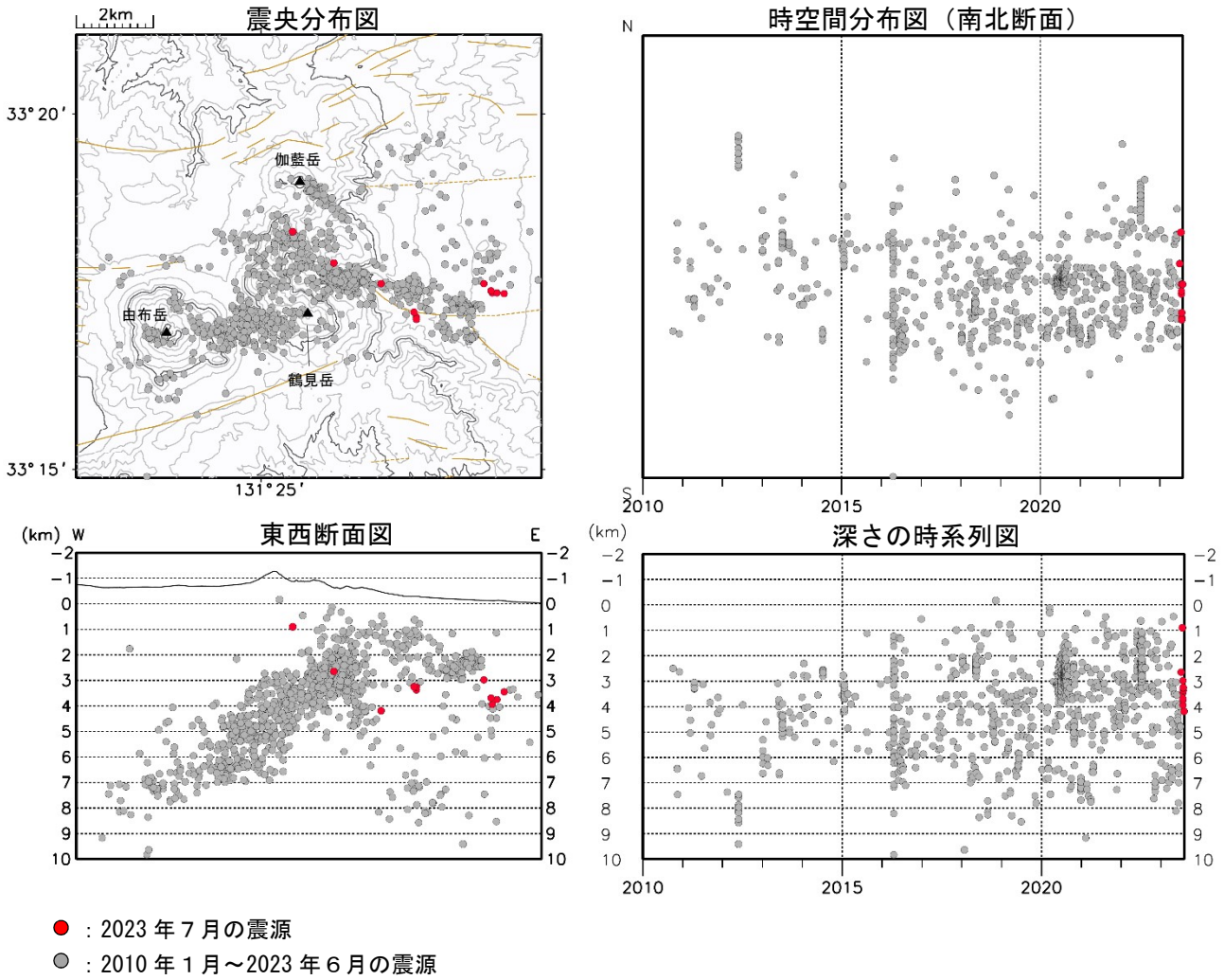
図3 鶴見岳・加藍岳 震源分布図（2010年1月～2023年7月）
