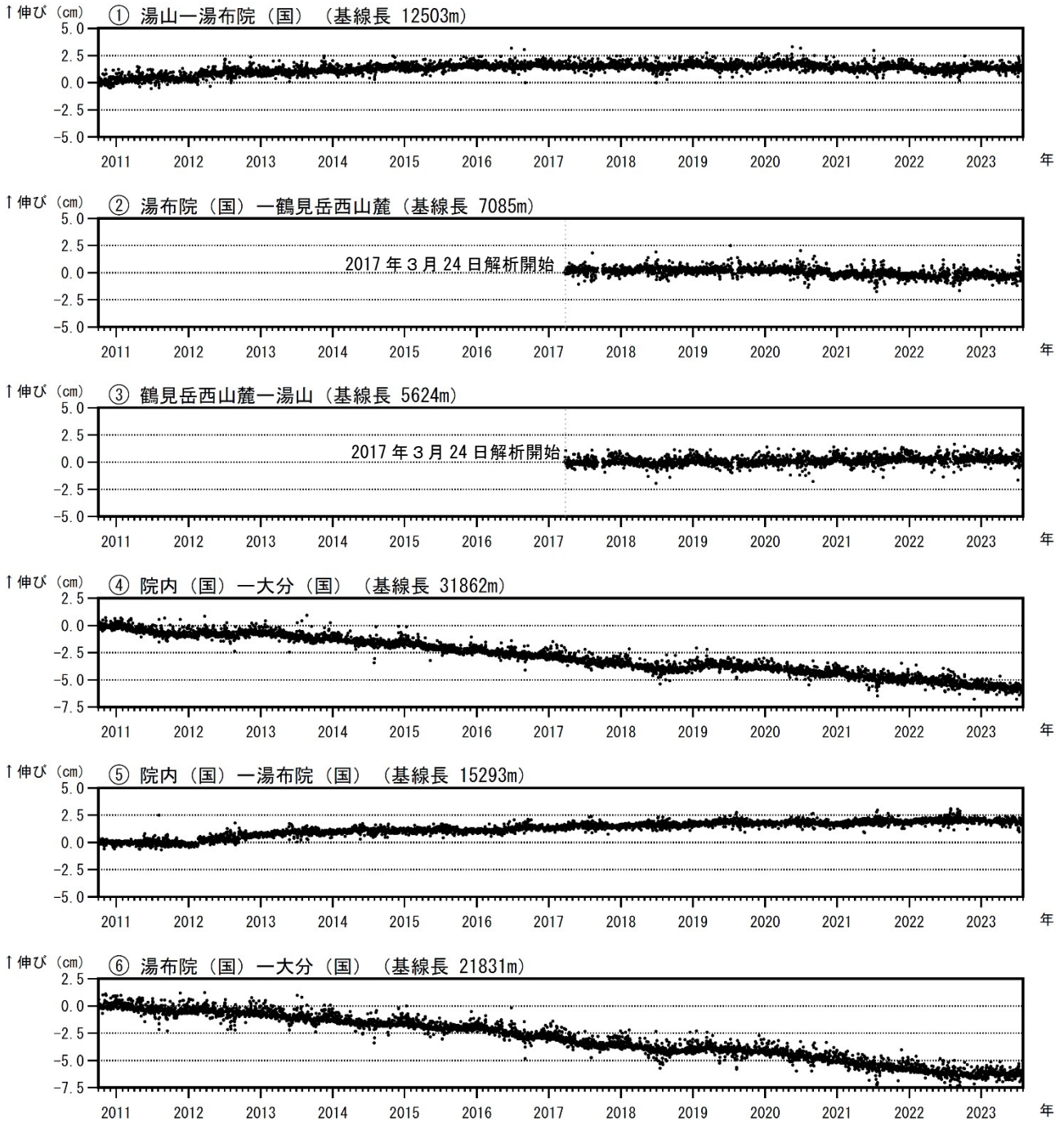
図4 鶴見岳・伽藍岳 GNSS連続観測による基線長変化（2010年10月～2023年7月）
