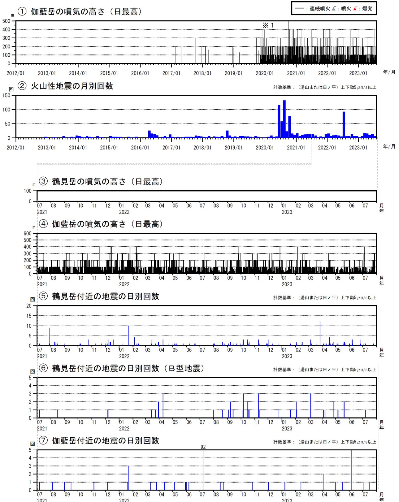
図2 鶴見岳・伽藍岳 火山活動経過図（2012年1月～2023年7月）
