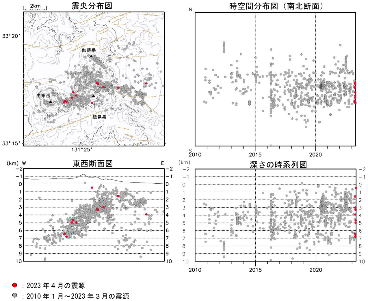
図3 鶴見岳・伽藍岳 震源分布図（2010年1月～2023年4月）
