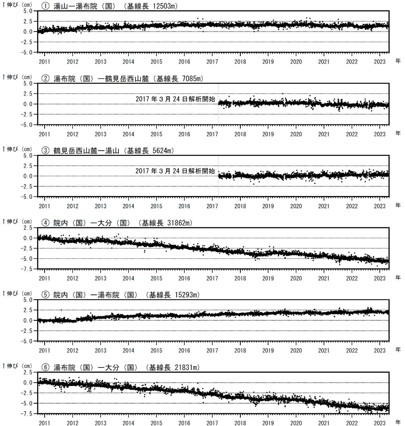
図4 鶴見岳・伽藍岳 GNSS連続観測による基線長変化（2010年10月～2023年4月）
