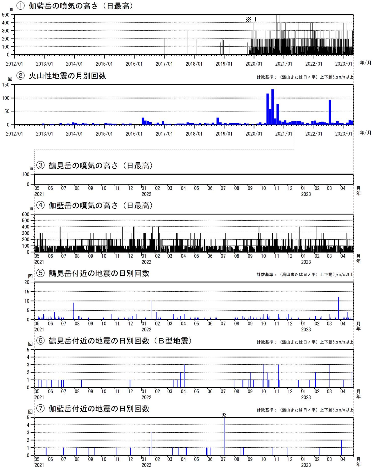
図2 鶴見岳・伽藍岳 火山活動経過図（2012年1月～2023年4月）
