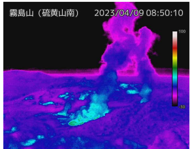
図1-2 霧島山（えびの高原（硫黄山）周辺） 硫黄山南側の状況
