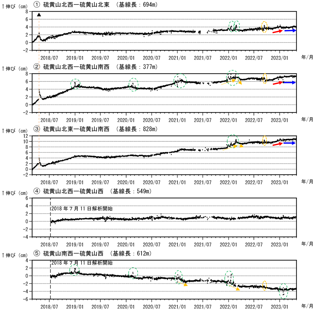
図7 霧島山（えびの高原（硫黄山）周辺） GNSS 連続観測による基線長変化 (2018年3月～2023年4月)
