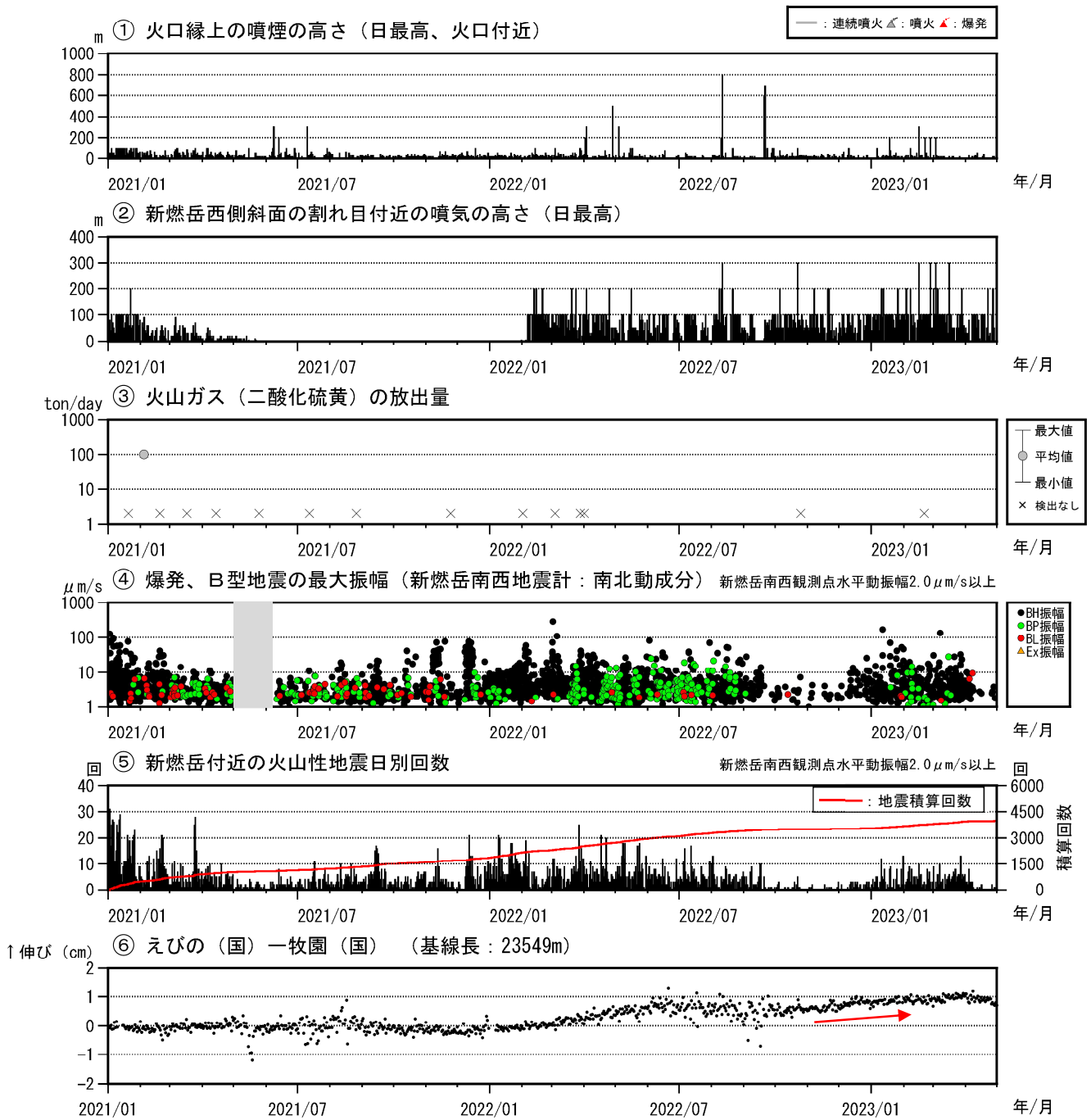
図 2-2 霧島山（新燃岳） 火山活動経過図（2021年1月～2023年4月）
