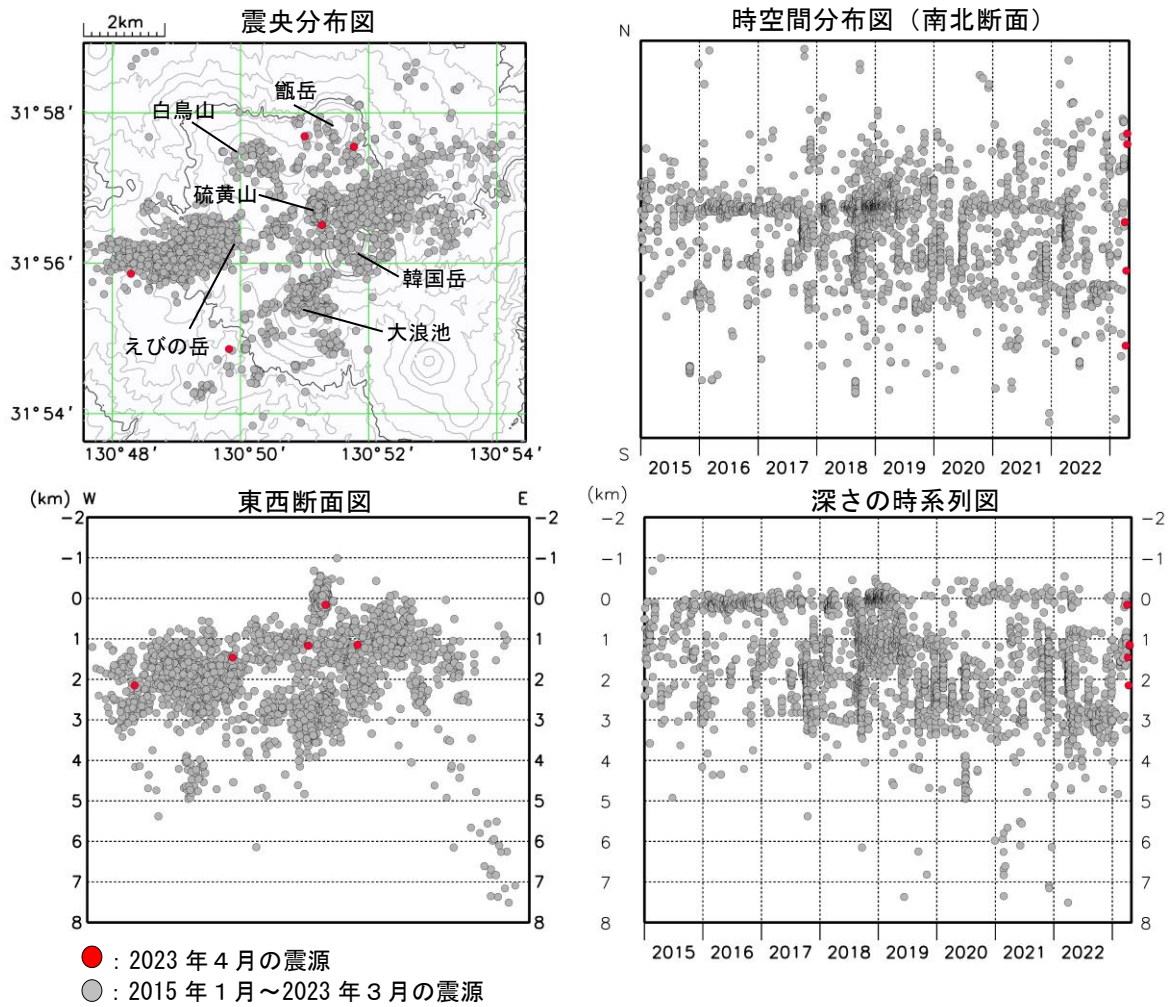
図5 霧島山（えびの高原（硫黄山）周辺） 震源分布図（2015年1月～2023年4月）
