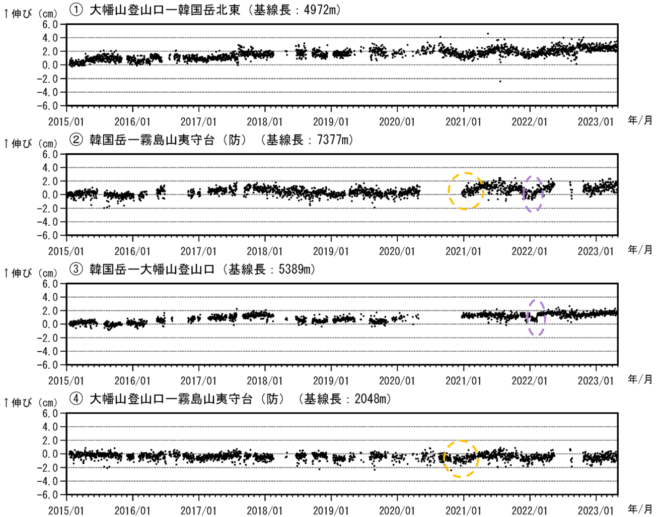
図4 霧島山（大幡池） GNSS 連続観測による基線長変化（2015年1月～2023年4月）
