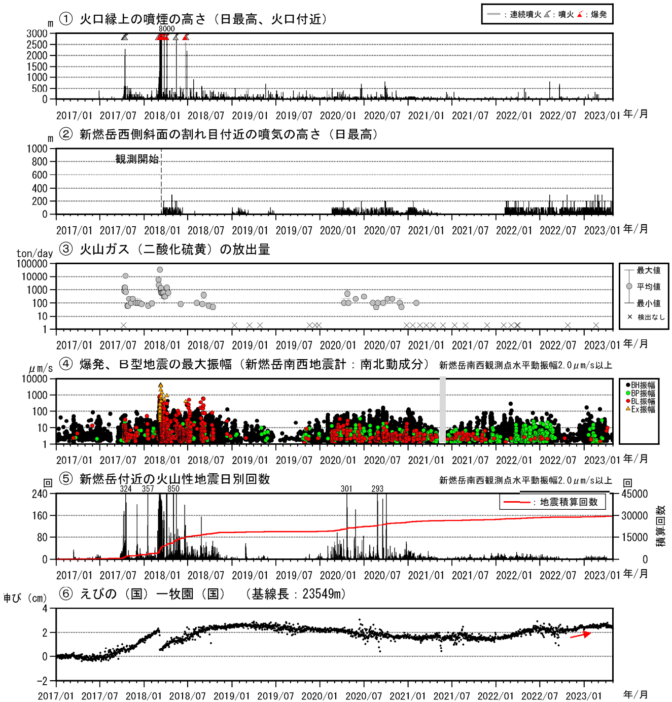
図 2-1 霧島山（新燃岳） 火山活動経過図（2017年1月～2023年4月）
