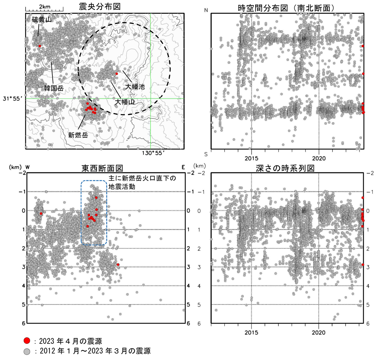
図3 霧島山（大幡池） 震源分布図（2012年1月～2023年4月）
