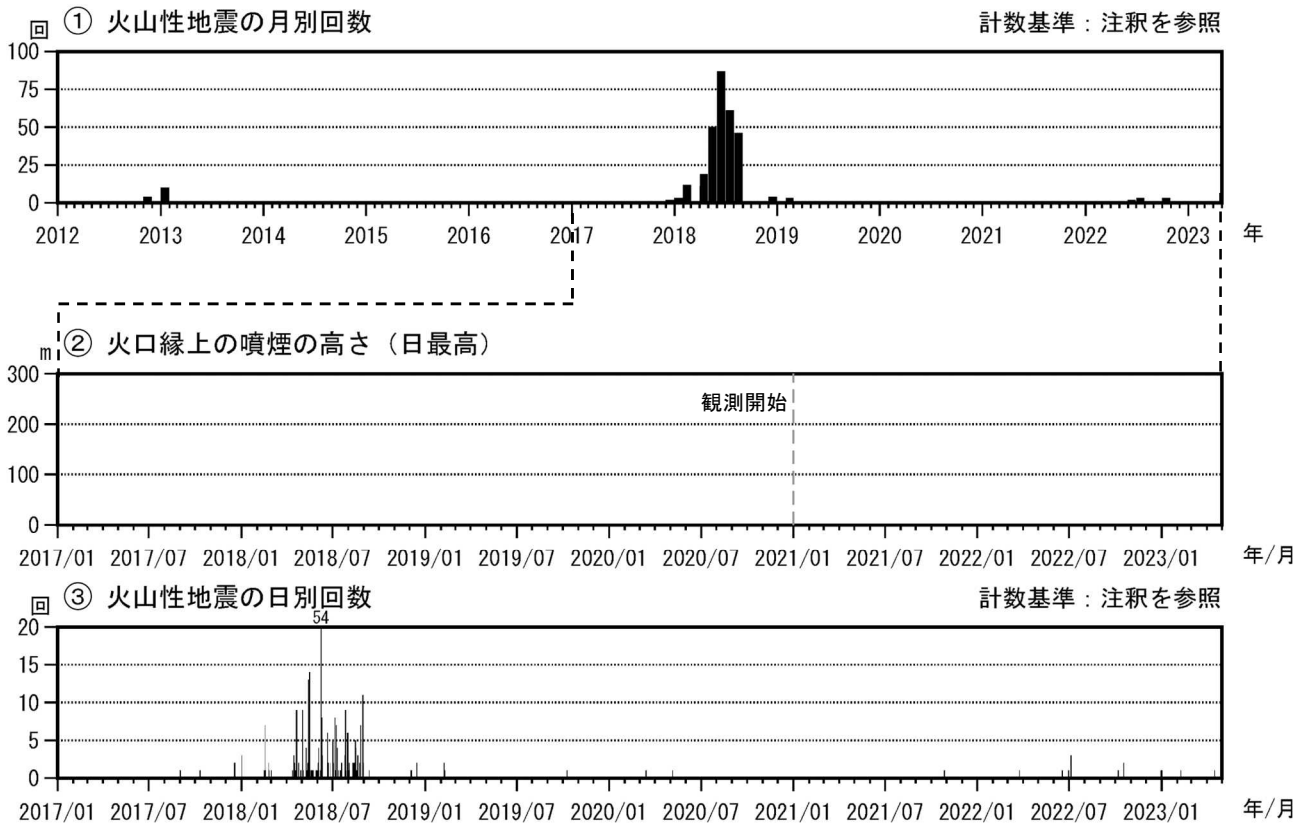
図2 霧島山（大幡池） 火山活動経過図（2012年1月～2023年4月）
