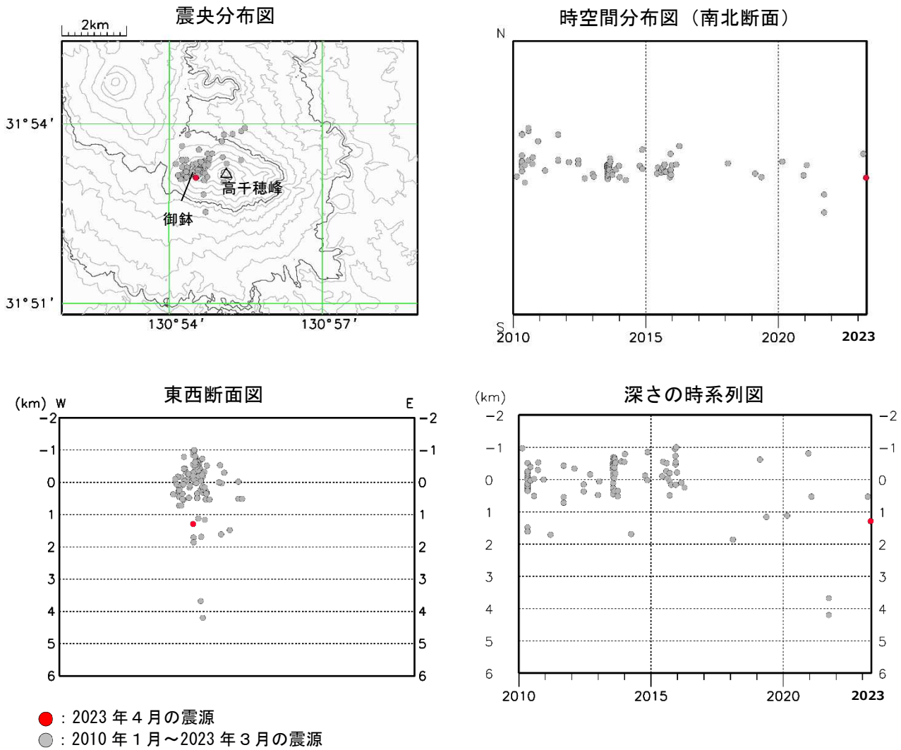
図2 霧島山（御鉢） 震源分布図（2010年1月～2023年4月）
