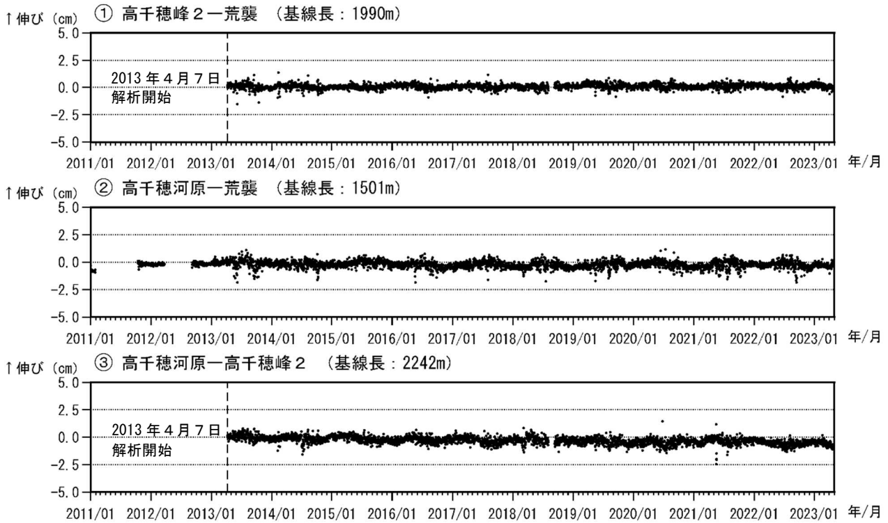
図4 霧島山（御鉢） GNSS 連続観測による基線長変化（2011年1月～2023年4月）
