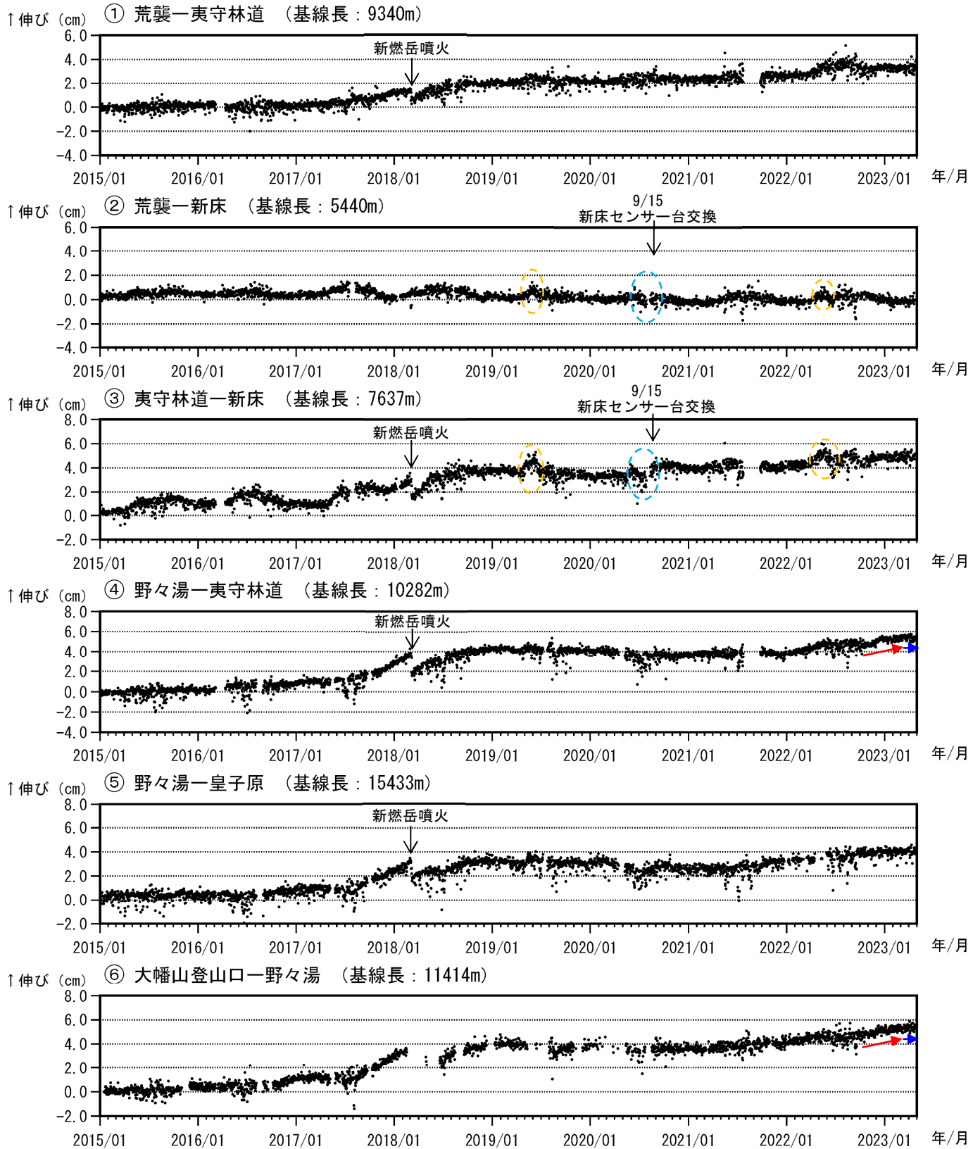
図4 霧島山（新燃岳） GNSS連続観測による基線長変化（2015年1月～2023年4月）
