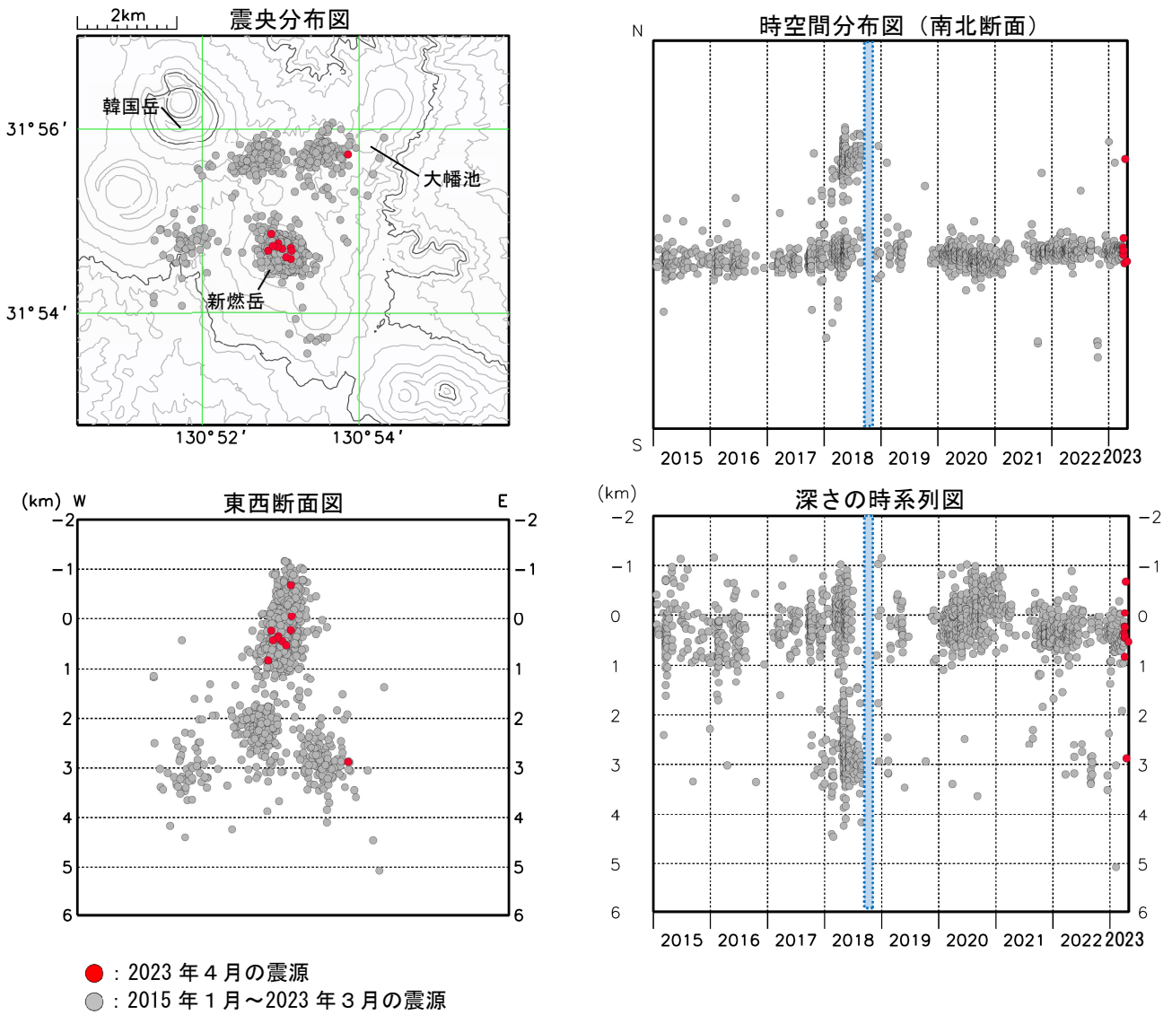
図3 霧島山（新燃岳）震源分布図（2015年1月～2023年4月）
