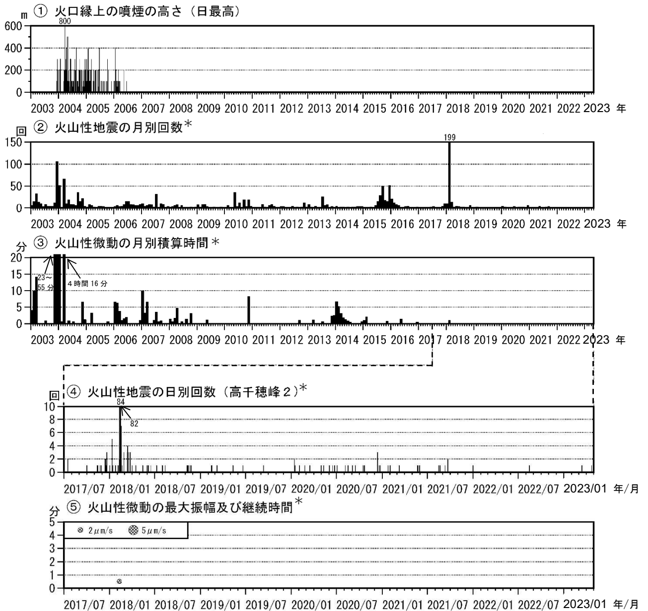
図3 霧島山（御鉢） 火山活動経過図（2003年1月～2023年4月）
