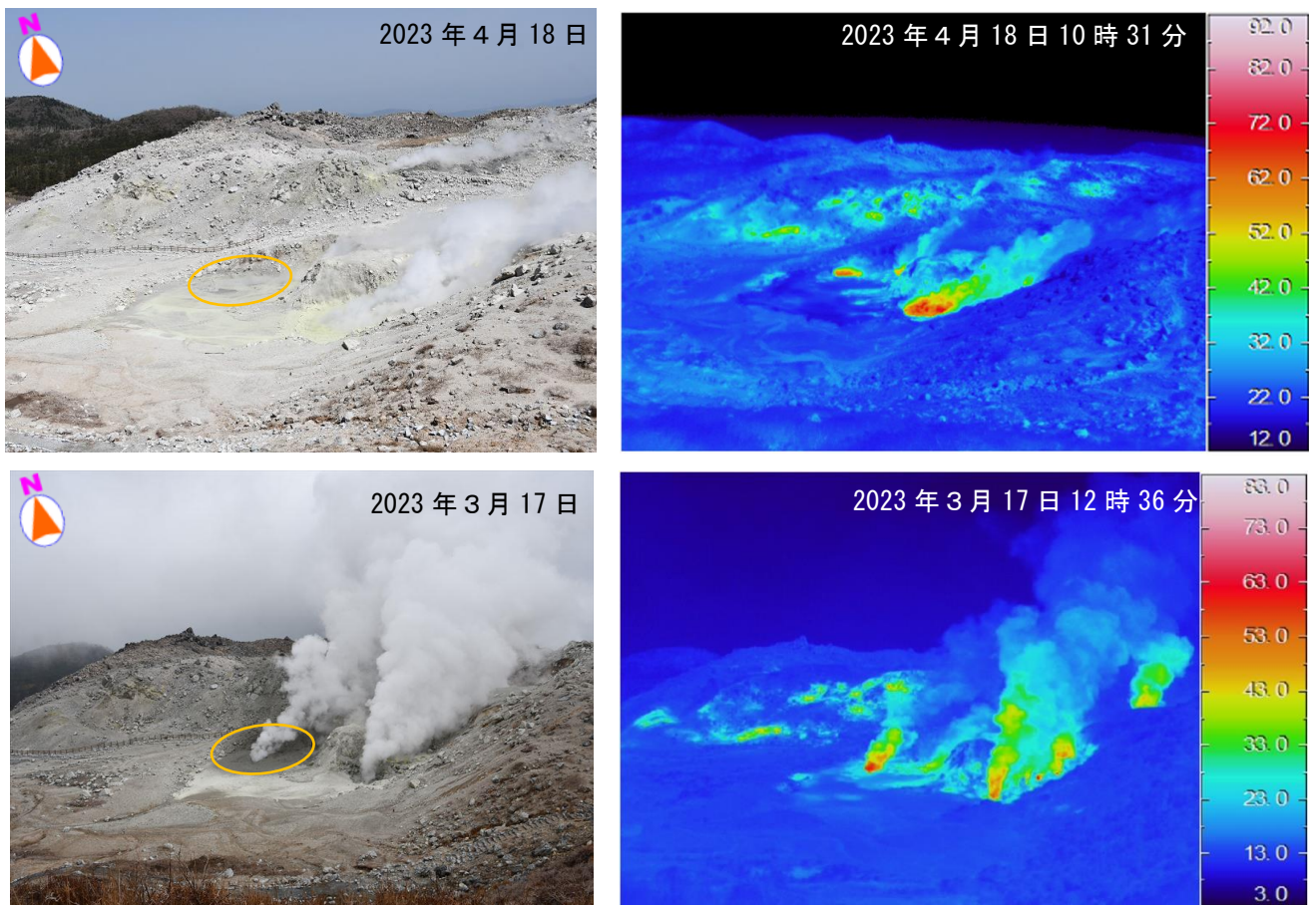
図3 霧島山（えびの高原（硫黄山）周辺） 硫黄山南側の地熱域の状況
