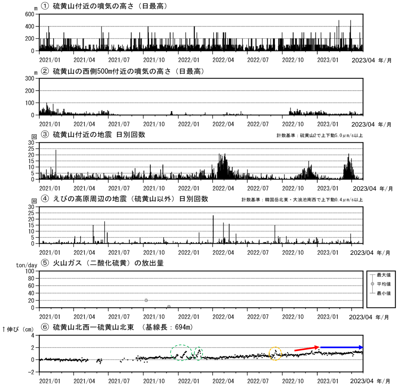
図4 霧島山（えびの高原（硫黄山）周辺）火山活動経過図（2021年1月～2023年4月）
