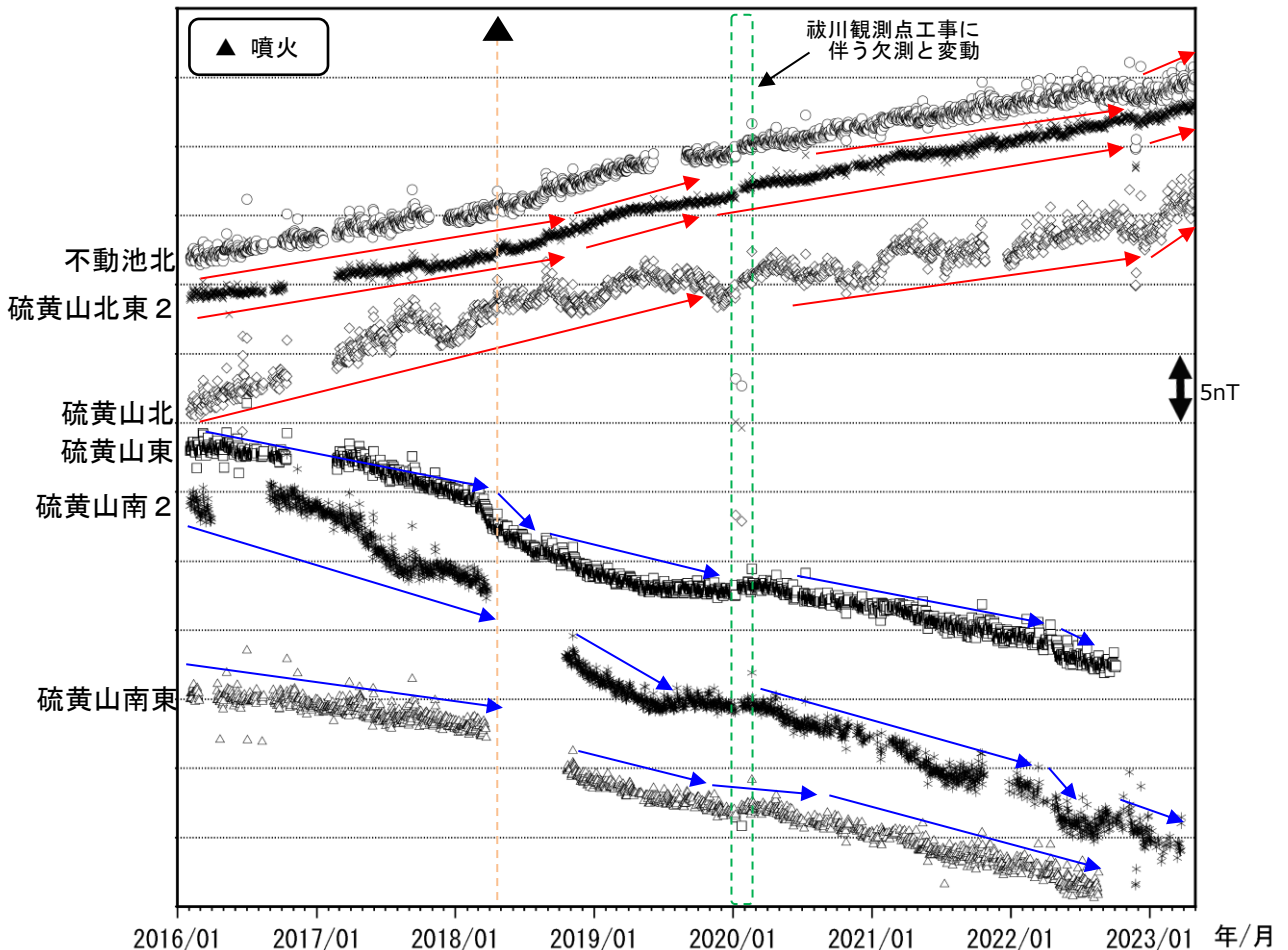
図 8-2 霧島山（えびの高原（硫黄山）周辺） 全磁力観測点で観測された全磁力変動（2016年1月～2023年4月）
