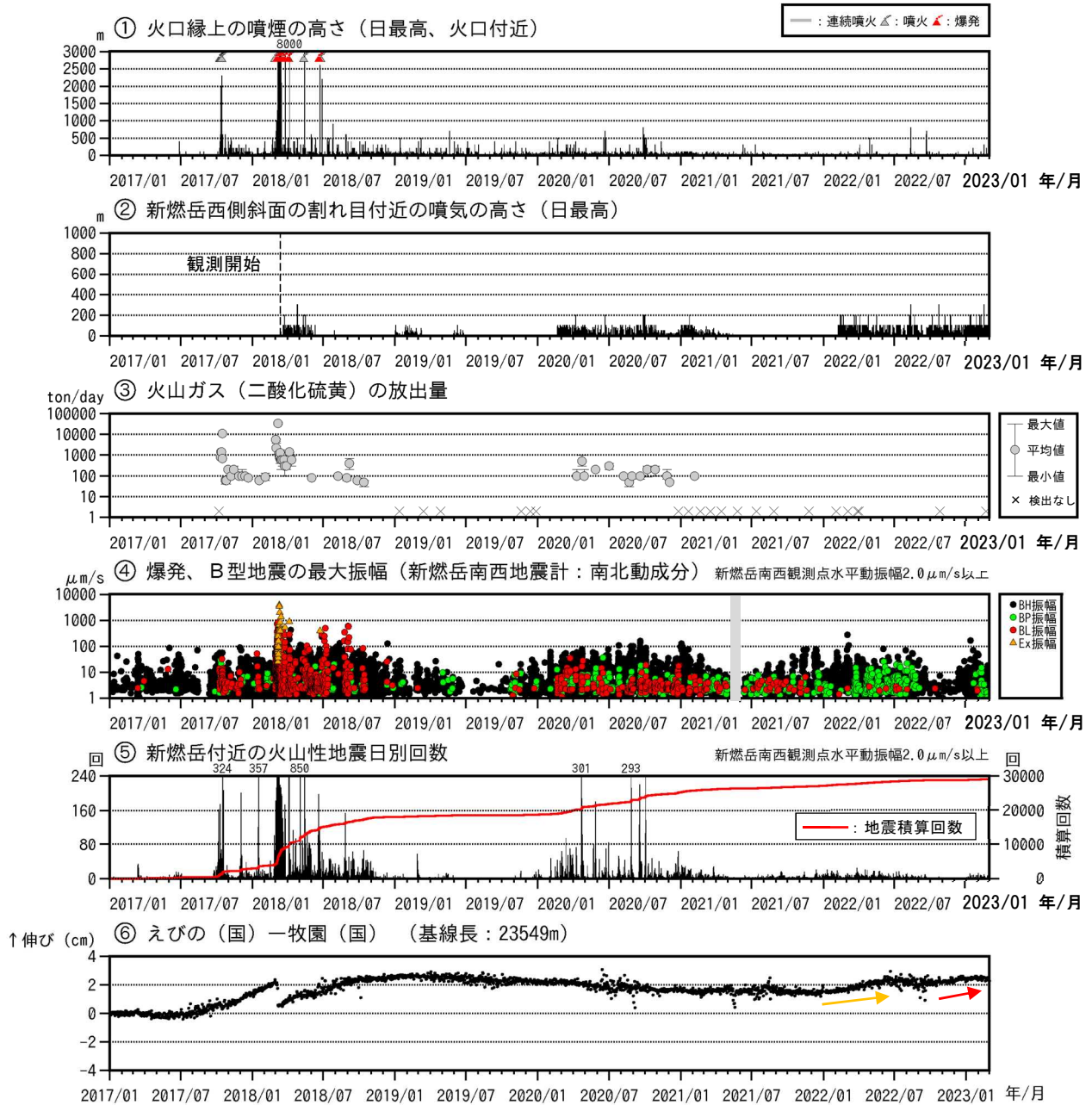
図 5-1 霧島山（新燃岳） 火山活動経過図（2017年1月～2023年2月）
