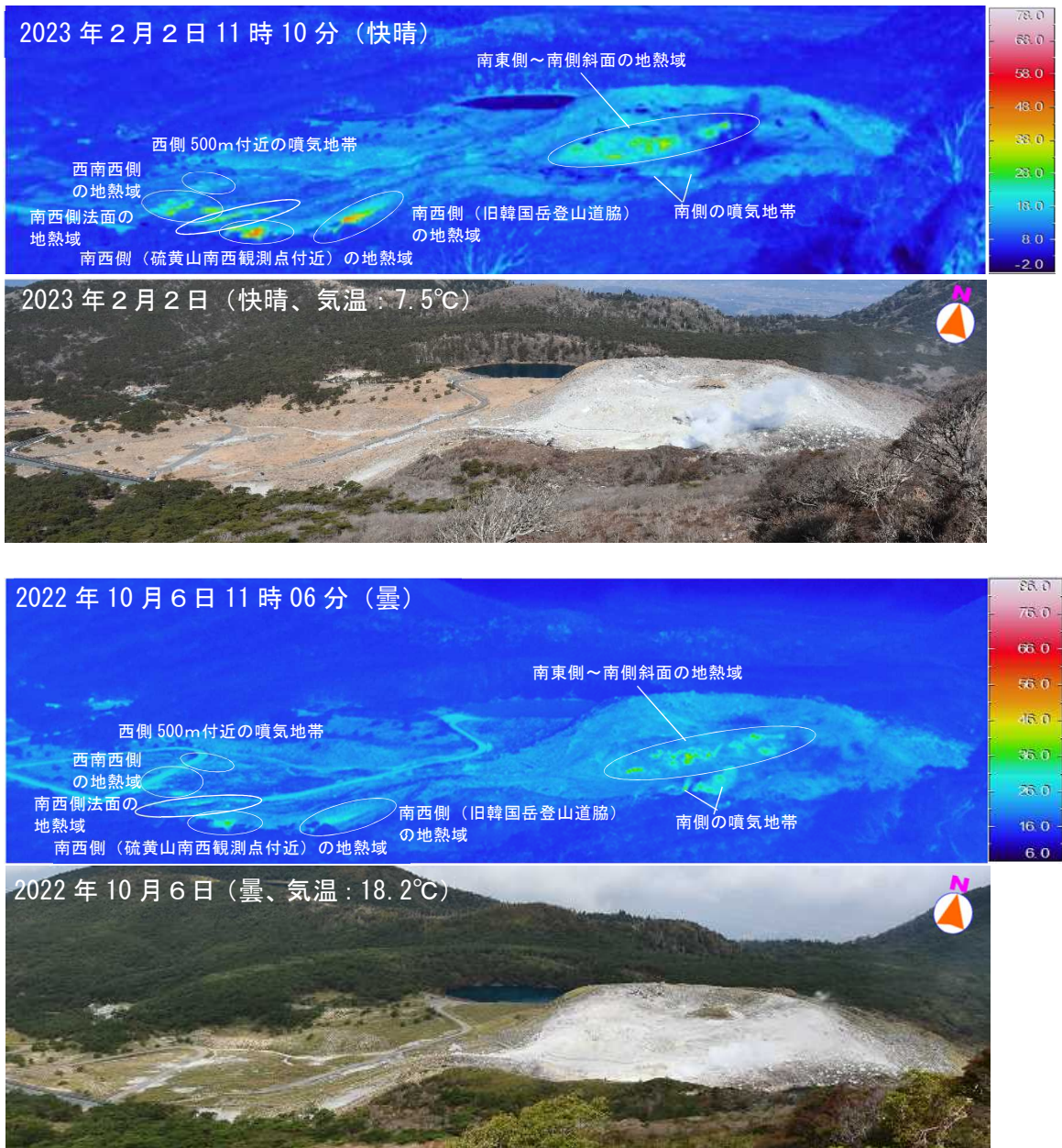
図2 霧島山（えびの高原（硫黄山）周辺） 硫黄山の火口及びその周辺の状況
