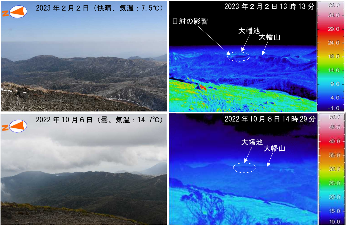
図2 霧島山（大幡池） 大幡池及び大幡山の状況（韓国岳山頂付近（図4参照）からの観測）
