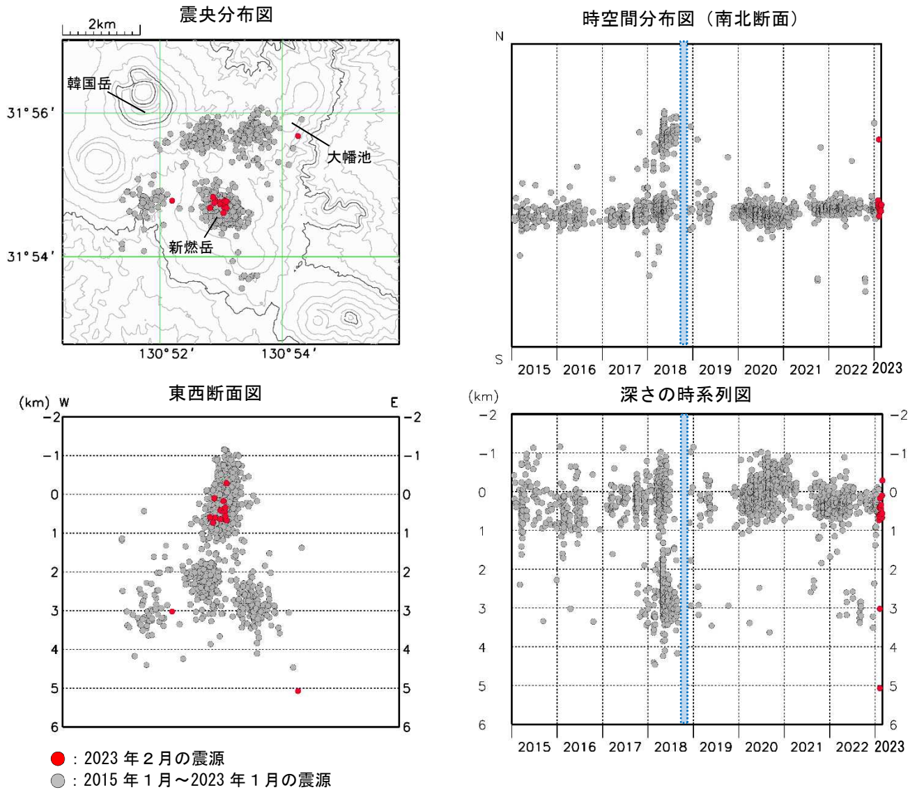
図 6-1 霧島山（新燃岳） 震源分布図（2015年1月～2023年2月）
