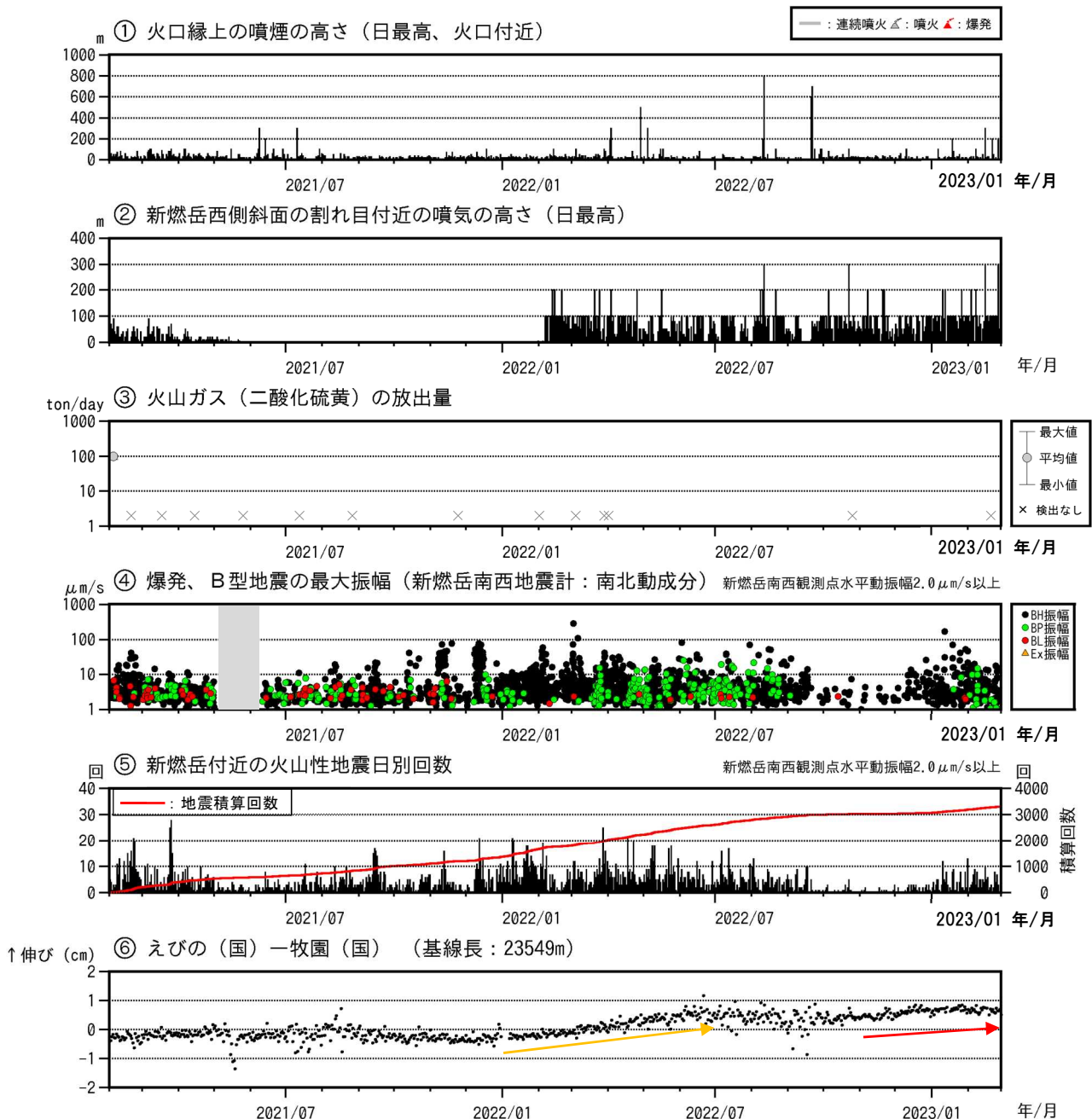
図 5-2 霧島山（新燃岳） 火山活動経過図（2021年2月～2023年2月）
