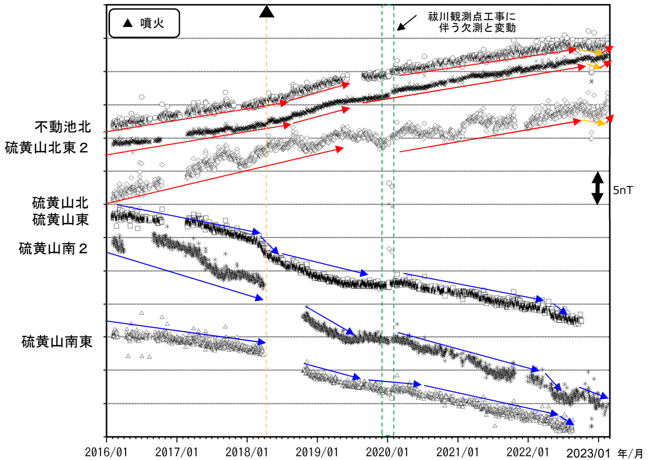
図 10-2 霧島山（えびの高原（硫黄山）周辺） 全磁力観測点で観測された全磁力変動（2016年1月～2023年2月）
