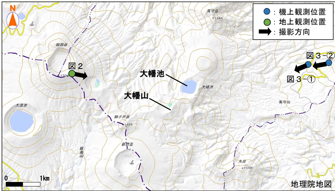
図4 霧島山（大幡池）図2、図3の観測位置及び撮影方向
