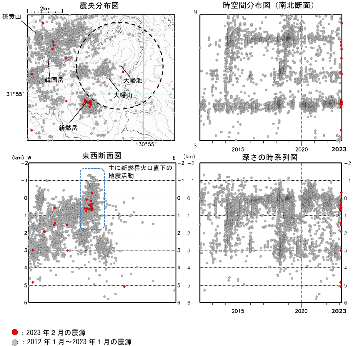
図6 霧島山（大幡池） 震源分布図（2012年1月～2023年2月）
