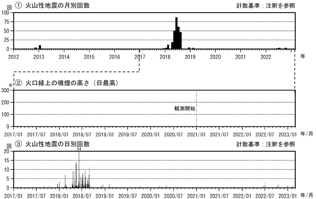
図5 霧島山（大幡池） 火山活動経過図（2012年1月～2023年2月）
