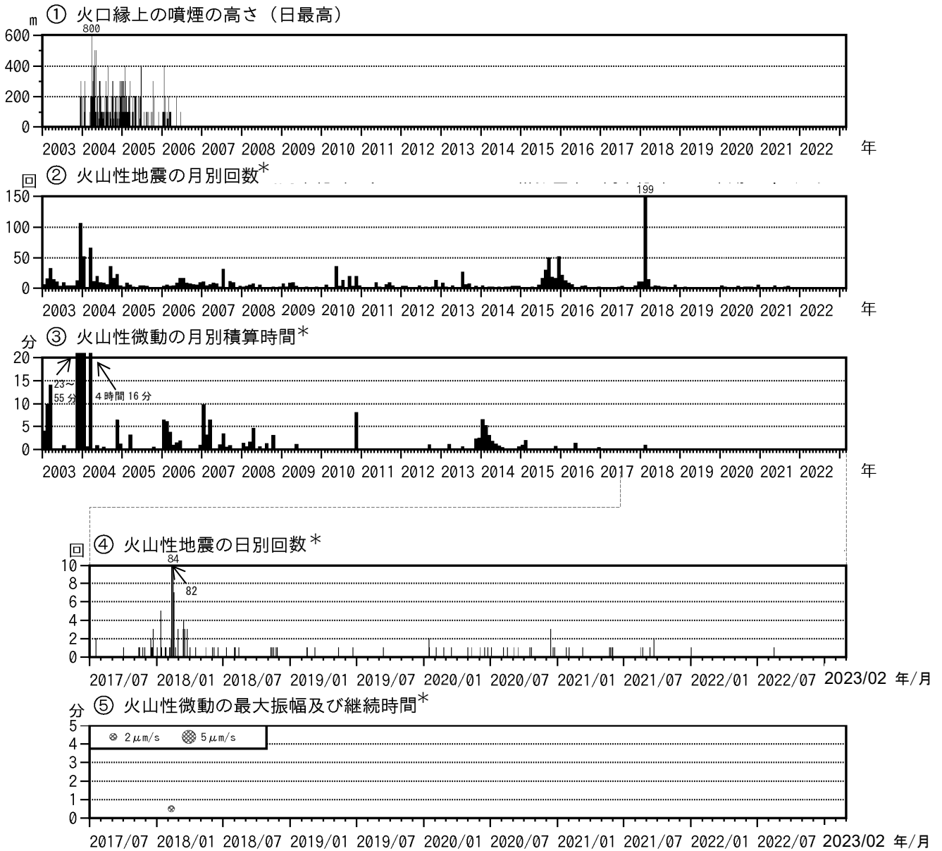
図5 霧島山（御鉢） 火山活動経過図（2003年1月～2023年2月）
