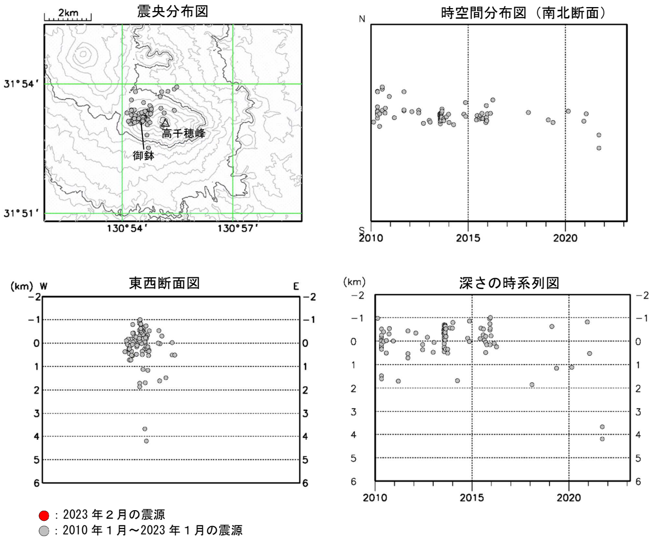
図4 霧島山（御鉢） 震源分布図（2010年1月～2023年2月）
