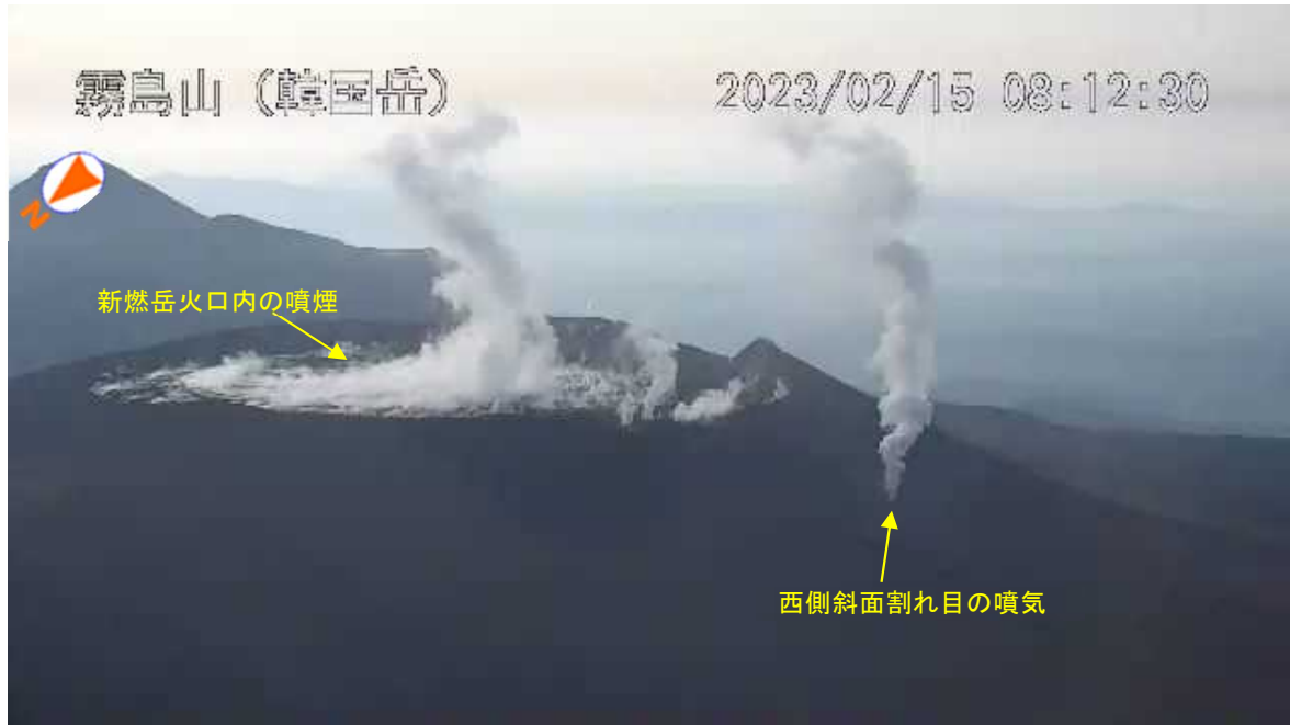
図1 霧島山（新燃岳） 噴煙の状況（2月15日、韓国岳監視カメラ）
