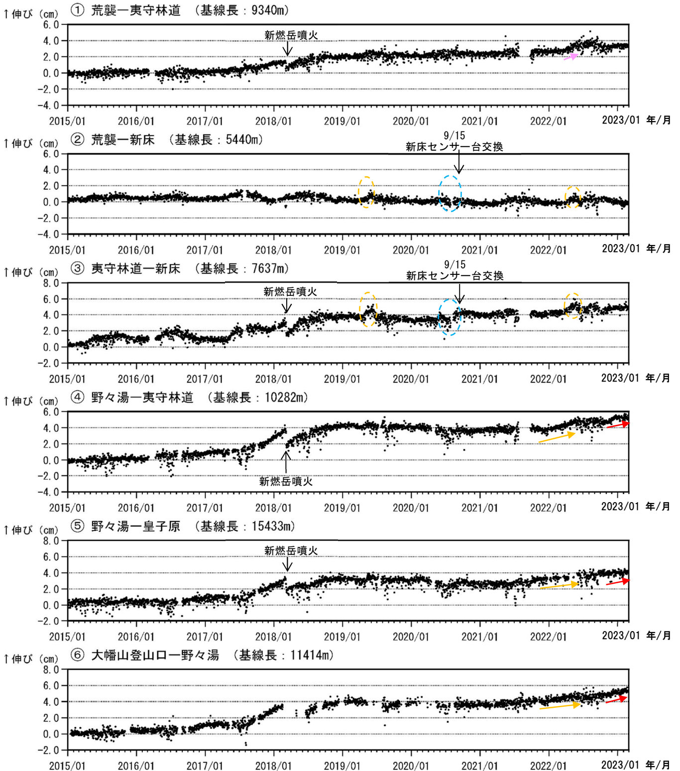
図7 霧島山（新燃岳） GNSS 連続観測による基線長変化（2015年1月～2023年2月）
