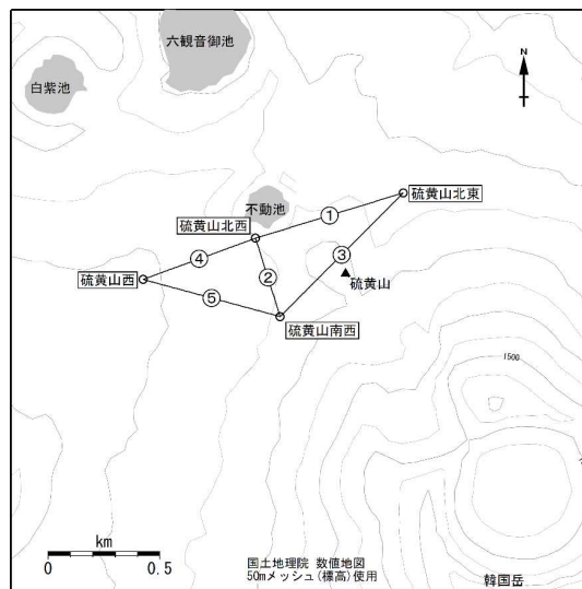
図8 霧島山（えびの高原（硫黄山）周辺） 図6及び図9のGNSS連続観測点と基線番号 小さな白丸（○）は気象庁の観測点位置を示しています。
