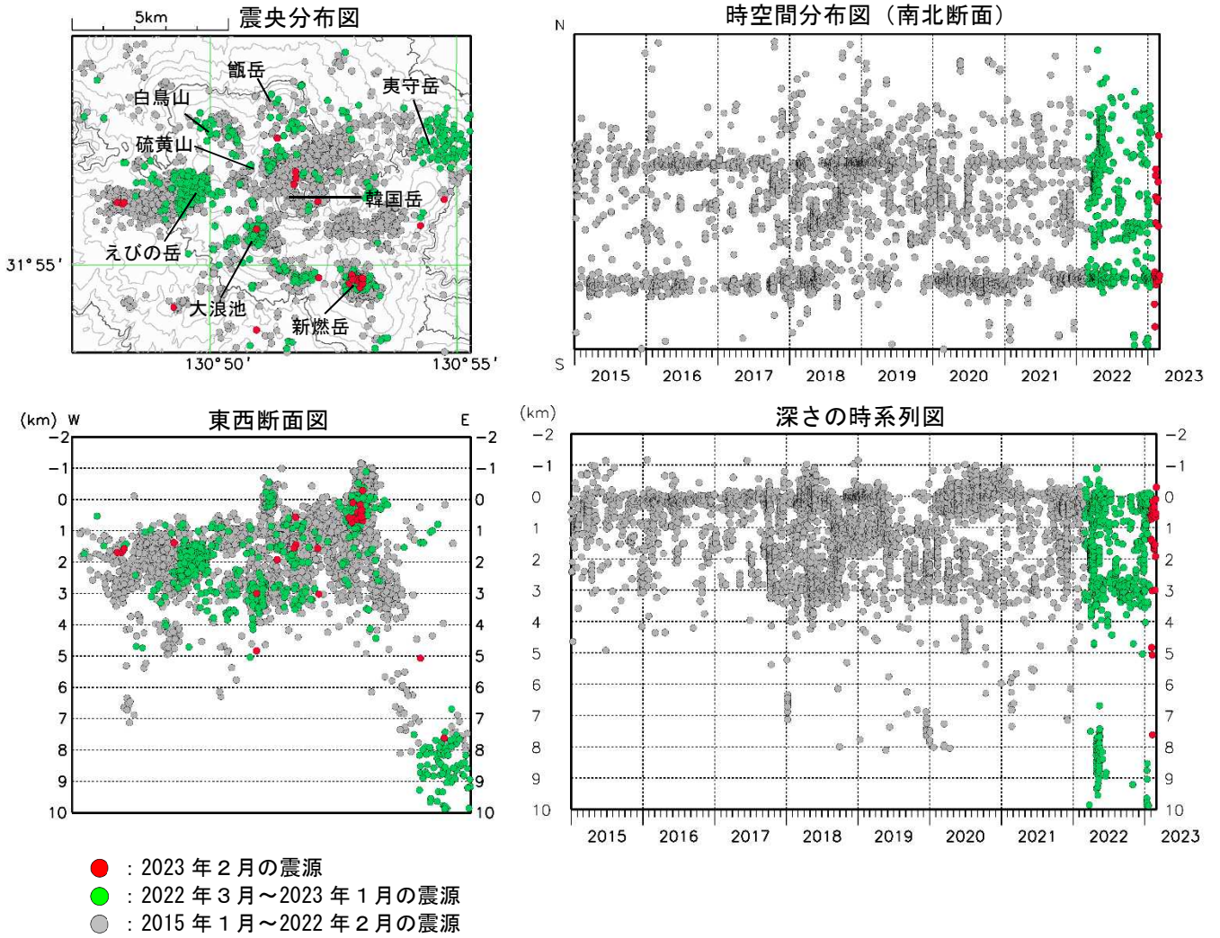
図6-2 霧島山（新燃岳及びえびの高原（硫黄山）周辺） 震源分布図 （2015年1月～2023年2月）
