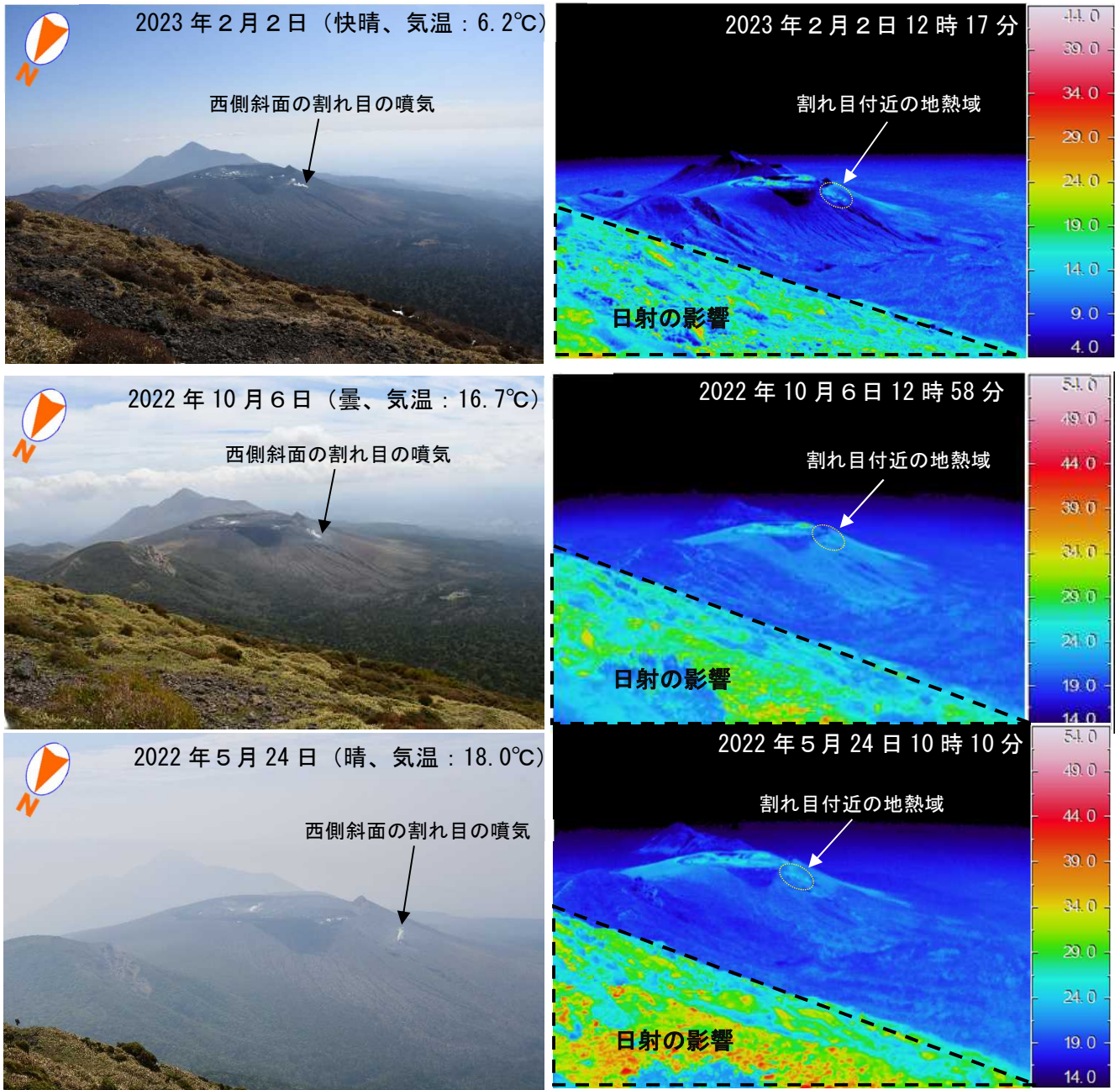
図3 霧島山（新燃岳） 新燃岳火口周辺の状況（2月2日、韓国岳山頂付近から観測）
