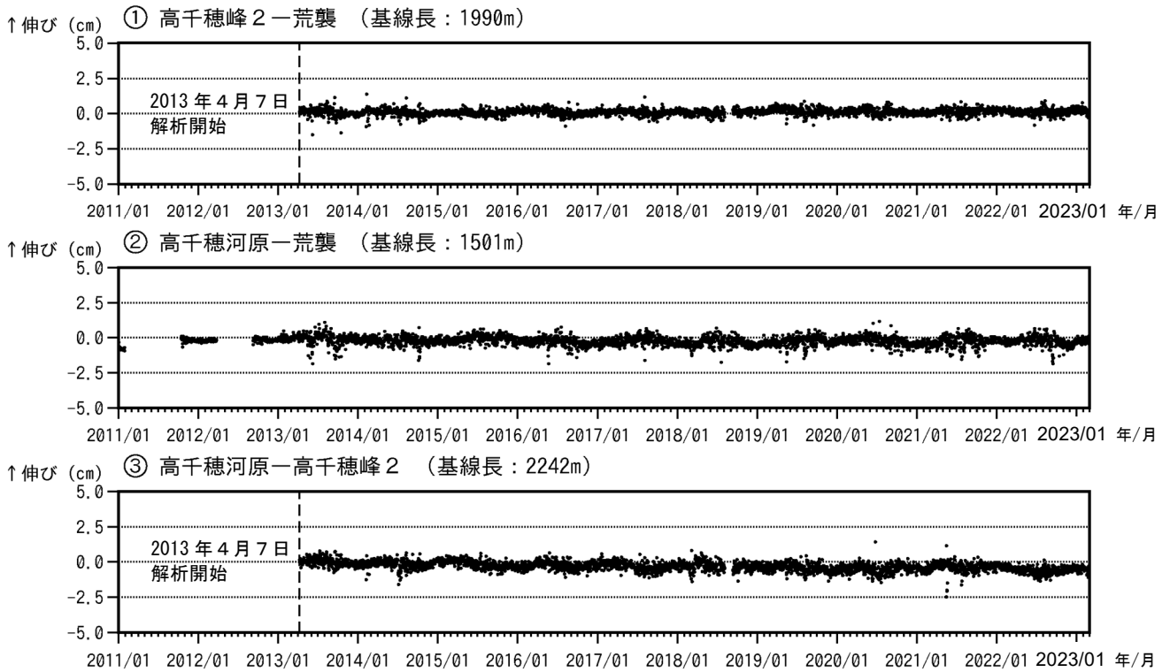
図6 霧島山（御鉢） GNSS連続観測による基線長変化（2011年1月～2023年2月）
