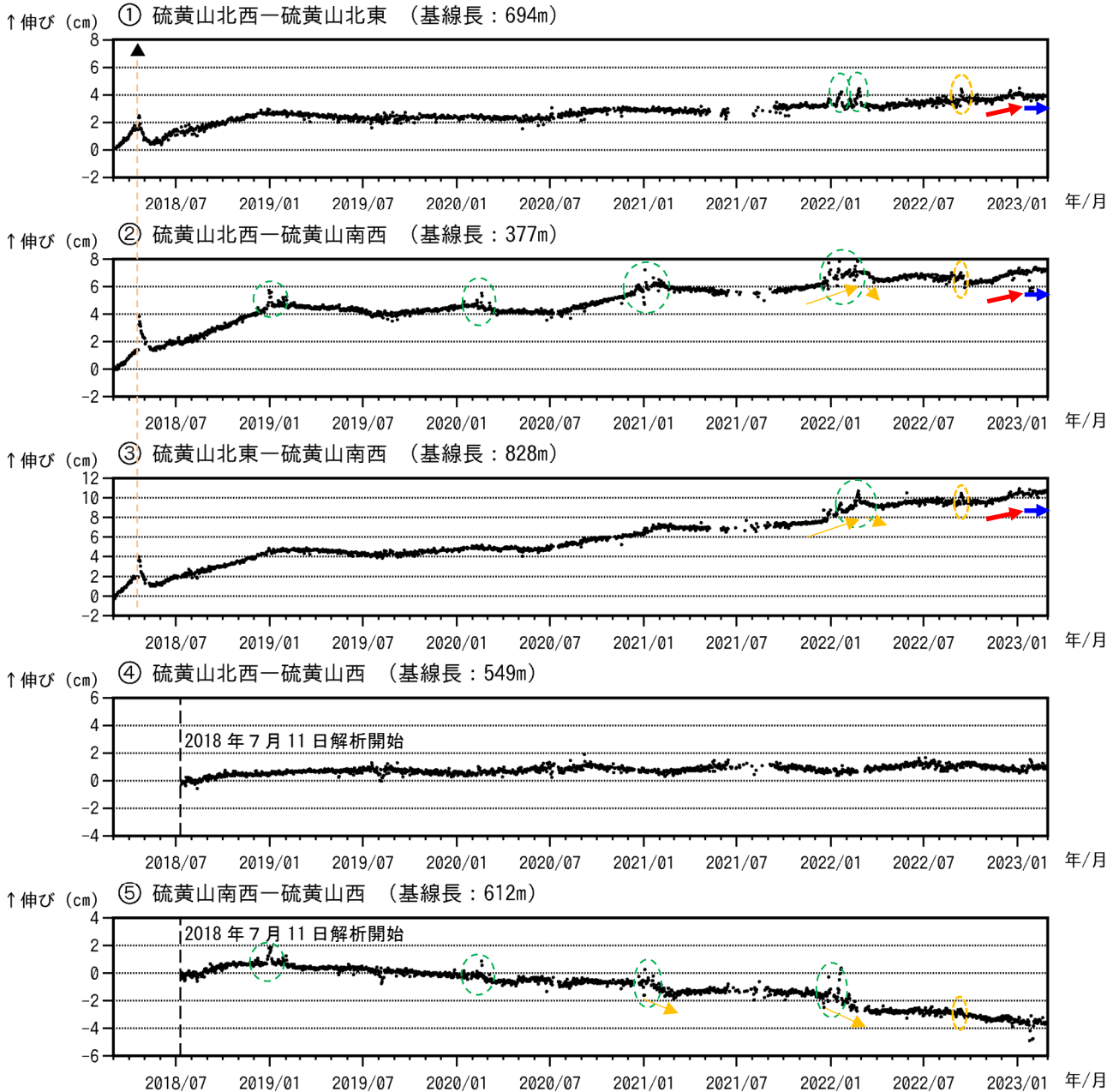
図9 霧島山（えびの高原（硫黄山）周辺） GNSS 連続観測による基線長変化 (2018年3月～2023年2月)
