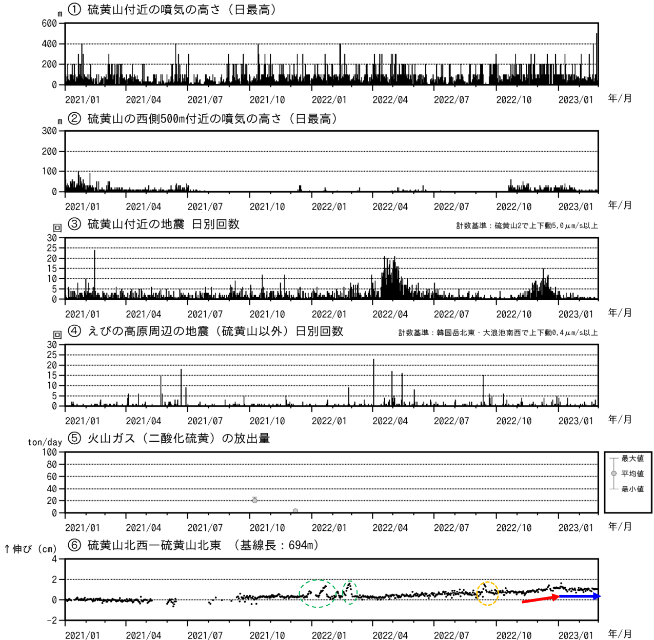
図6 霧島山（えびの高原（硫黄山）周辺）火山活動経過図（2021年1月～2023年2月）
