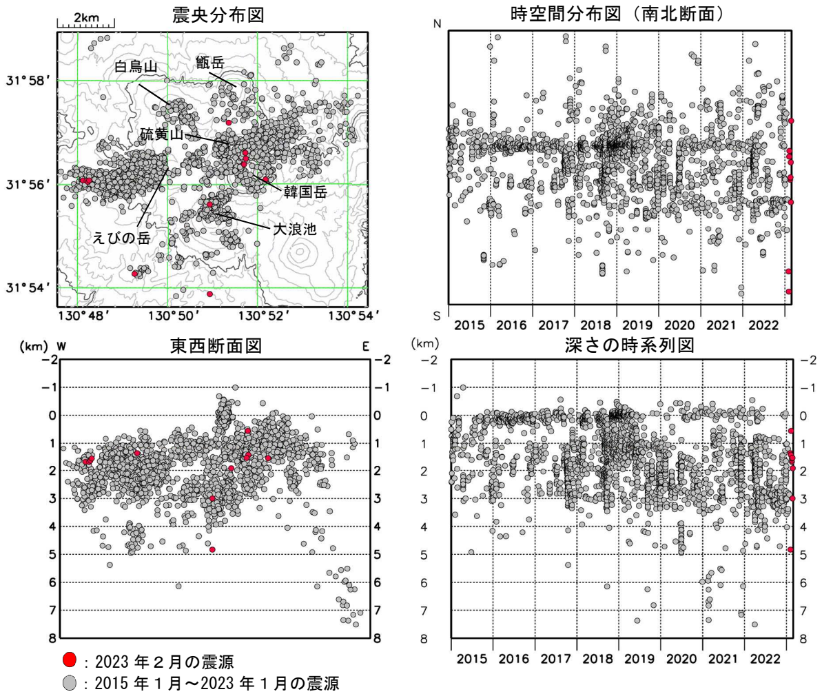
図7 霧島山（えびの高原（硫黄山）周辺） 震源分布図（2015年1月～2023年2月）
