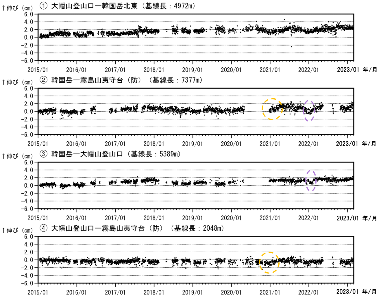
図7 霧島山（大幡池） GNSS 連続観測による基線長変化（2015年1月～2023年2月）
