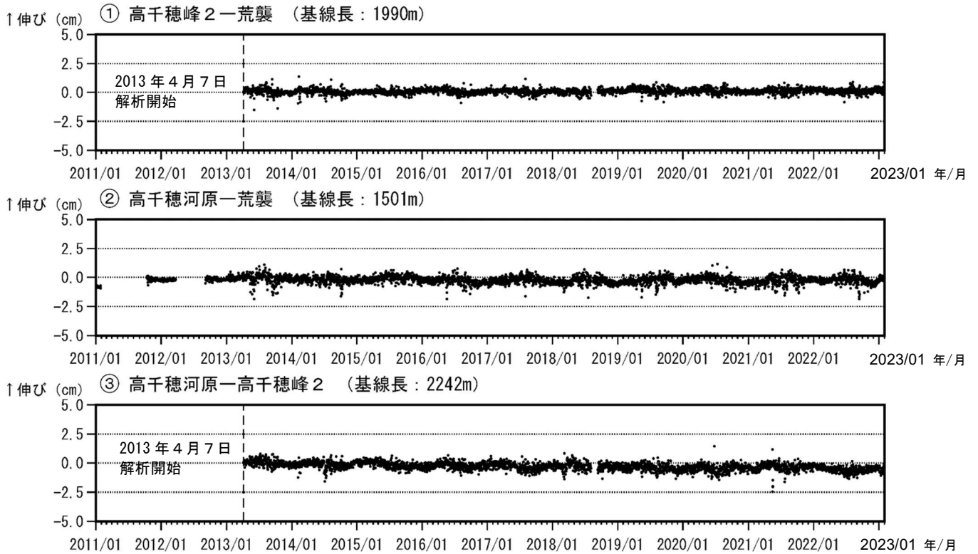
図4 霧島山（御鉢） GNSS 連続観測による基線長変化（2011年1月～2023年1月）
