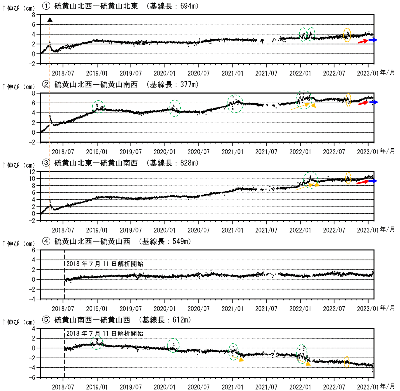
図5 霧島山（えびの高原（硫黄山）周辺） GNSS 連続観測による基線長変化 （2018年3月～2023年1月）
