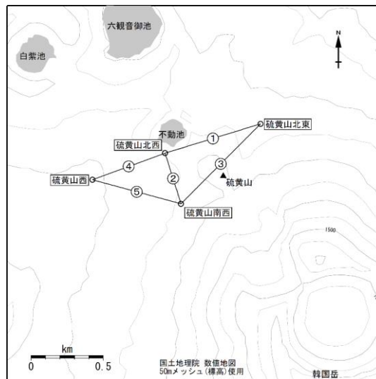
図4 霧島山（えびの高原（硫黄山）周辺） 図2及び図5のGNSS連続観測点と基線番号 小さな白丸（○）は気象庁の観測点位置を示しています。
