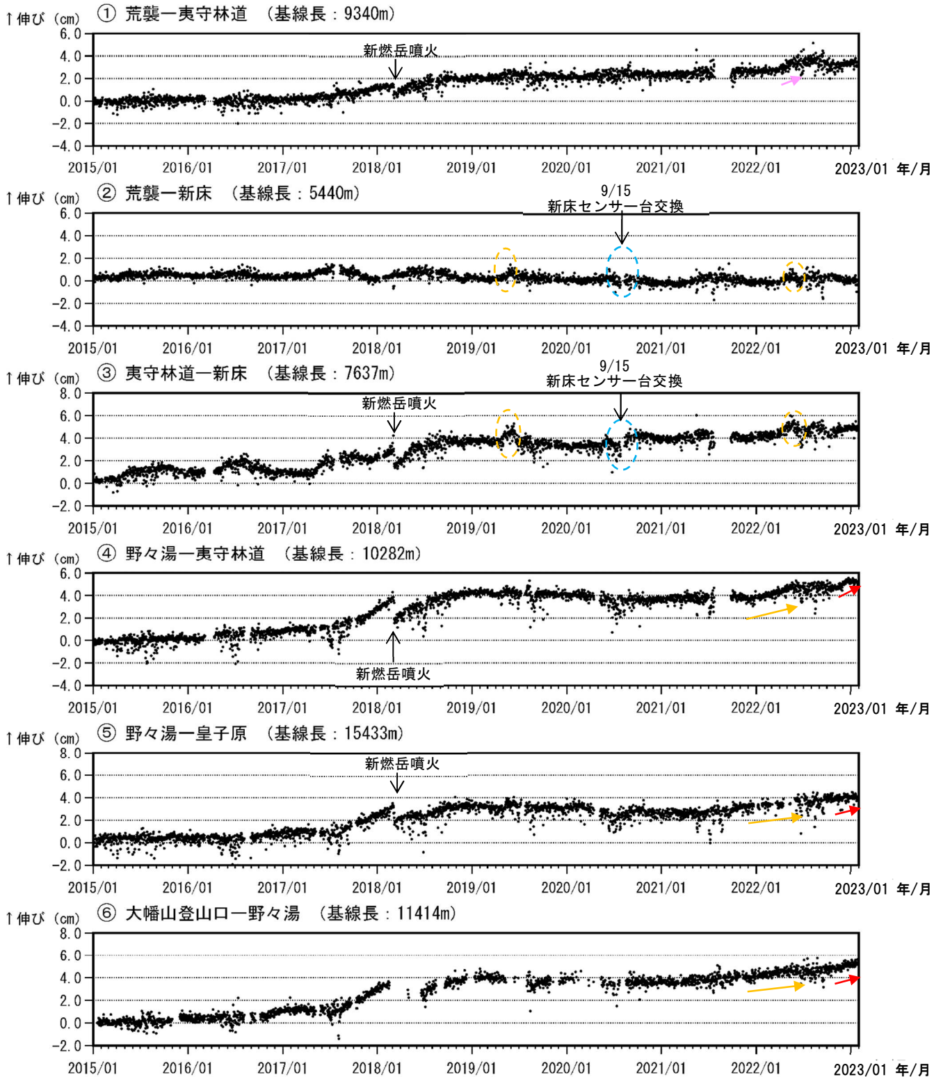
図6 霧島山（新燃岳） GNSS 連続観測による基線長変化（2015年1月～2023年1月）
