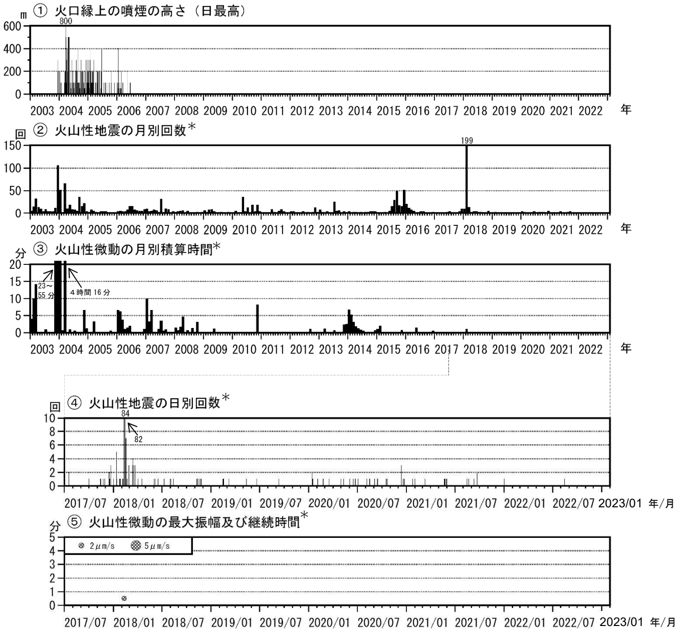
図3 霧島山（御鉢） 火山活動経過図（2003年1月～2023年1月）
