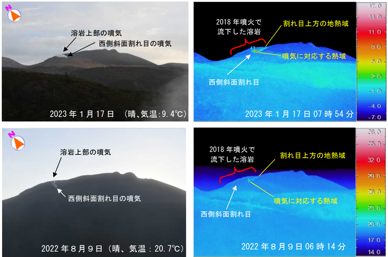
図3 霧島山（新燃岳） 新燃岳南西側の状況（新湯温泉付近（図2）から観測）
