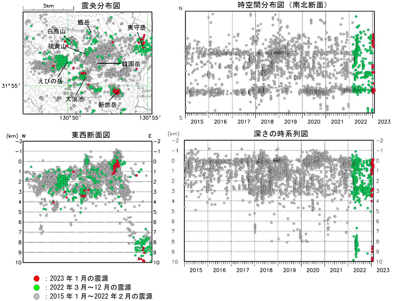
図5-2 霧島山（新燃岳及びえびの高原（硫黄山）周辺） 震源分布図 （2015年1月～2023年1月）
