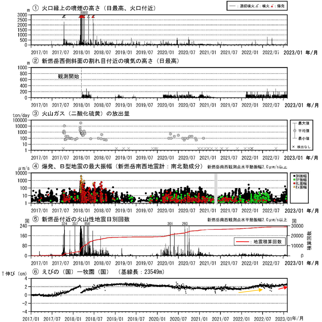
図 4-1 霧島山（新燃岳） 火山活動経過図（2017年1月～2023年1月）
