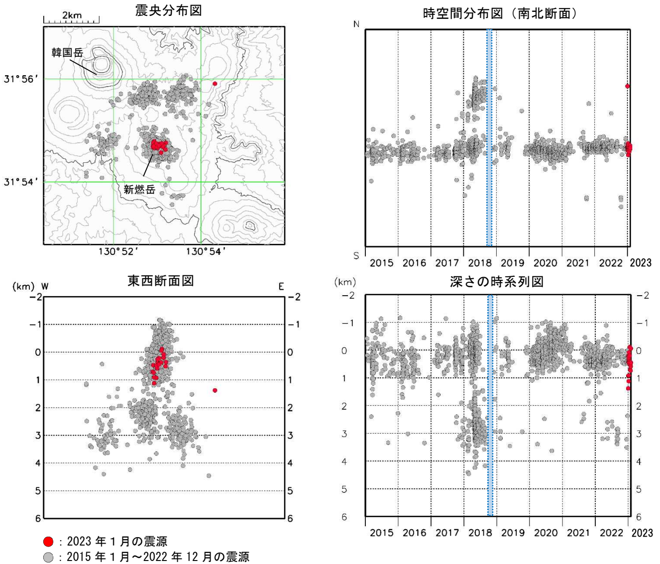
図 5-1 霧島山（新燃岳） 震源分布図（2015年1月～2023年1月）
