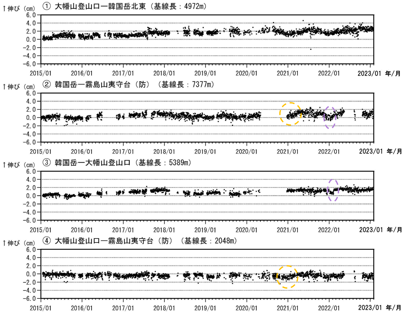
図4 霧島山（大幡池） GNSS 連続観測による基線長変化（2015年1月～2023年1月）
