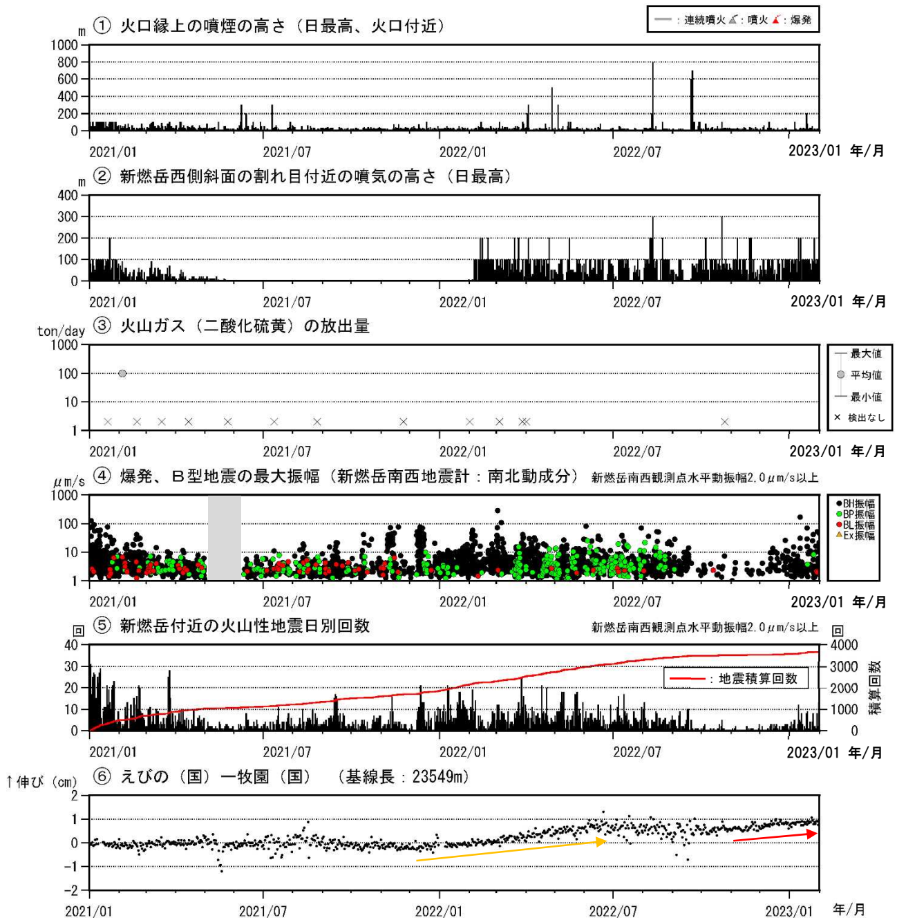
図 4-2 霧島山（新燃岳） 火山活動経過図（2021年1月～2023年1月）
