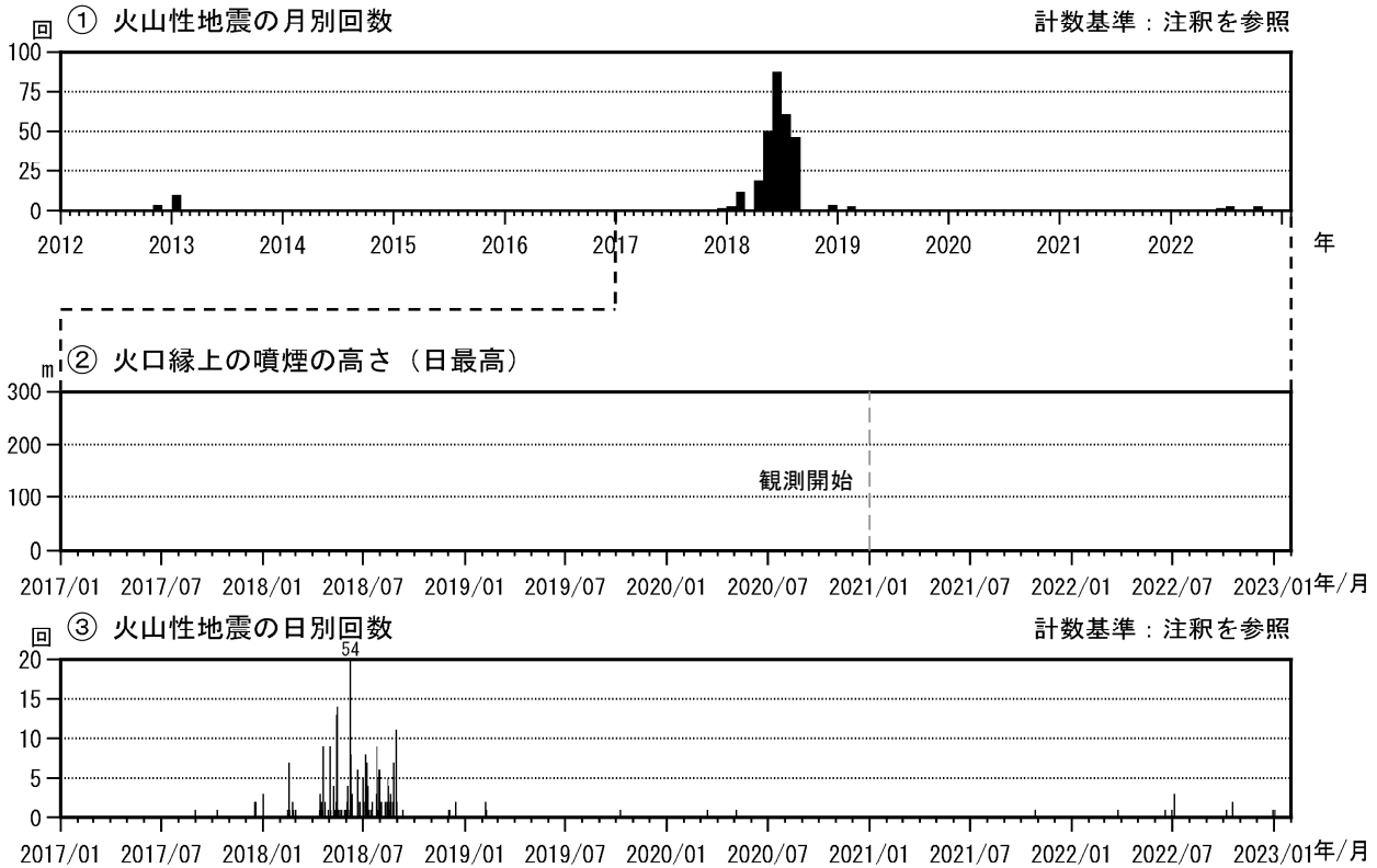
図2 霧島山（大幡池） 火山活動経過図（2012年1月～2023年1月）
