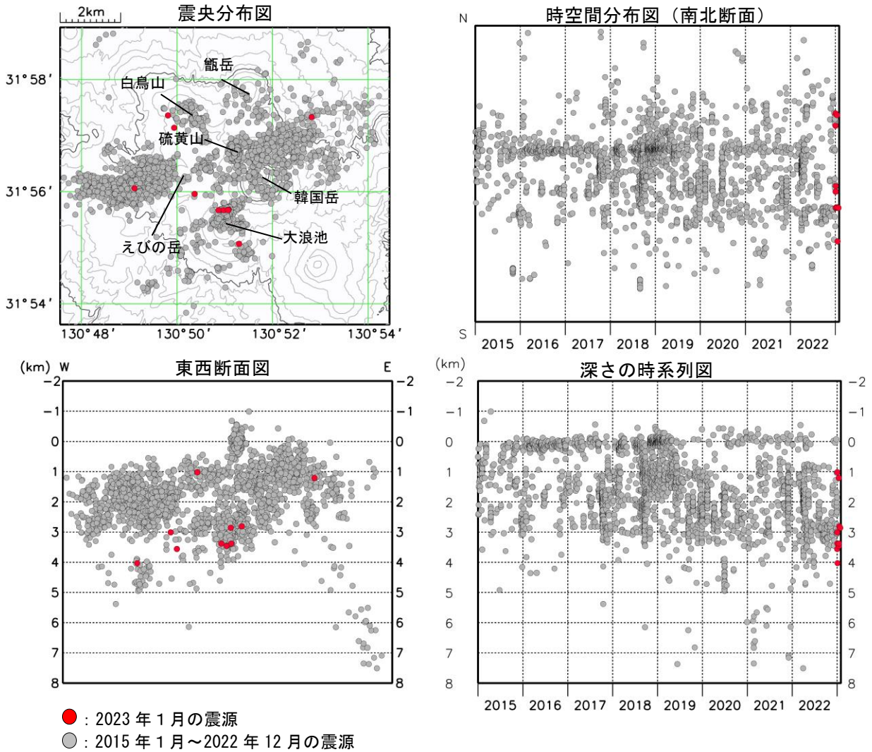
図3 霧島山（えびの高原（硫黄山）周辺） 震源分布図（2015年1月～2023年1月）
