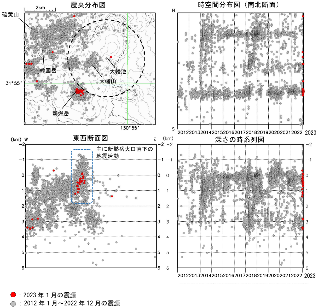
図3 霧島山（大幡池） 震源分布図（2012年1月～2023年1月）
