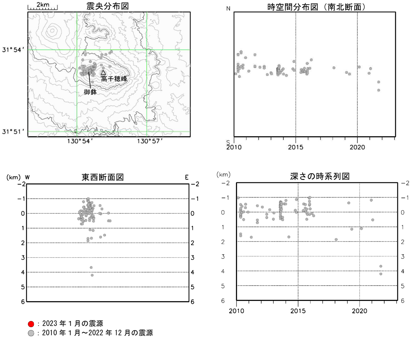
図2 霧島山（御鉢） 震源分布図（2010年1月～2023年1月）
