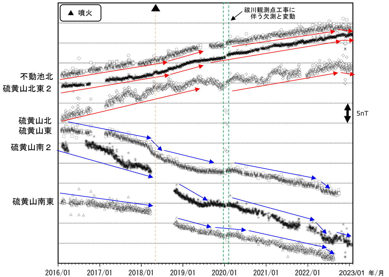
図 6-2 霧島山（えびの高原（硫黄山）周辺） 全磁力観測点で観測された全磁力変動 （2016年1月～2023年1月）
