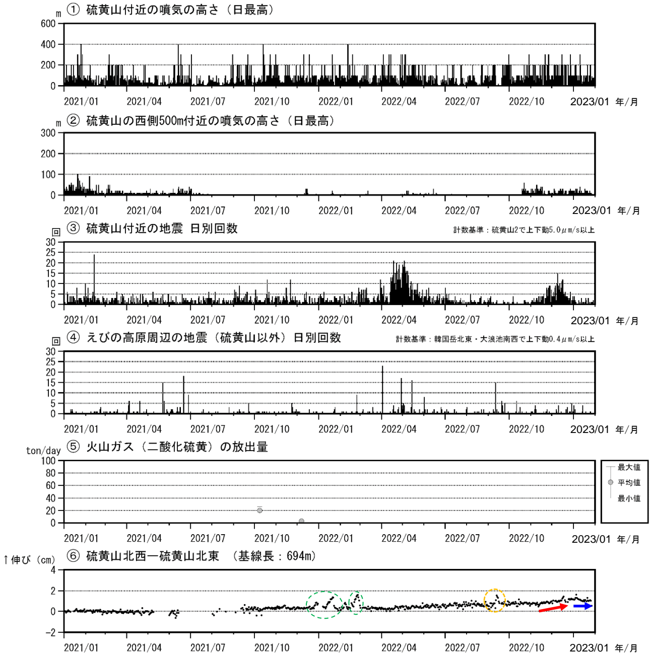
図2 霧島山（えびの高原（硫黄山）周辺）火山活動経過図（2021年1月～2023年1月）
