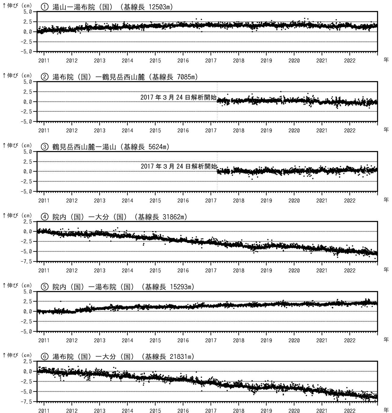
図4 鶴見岳・伽藍岳 GNSS連続観測による基線長変化（2010年10月～2022年12月）
