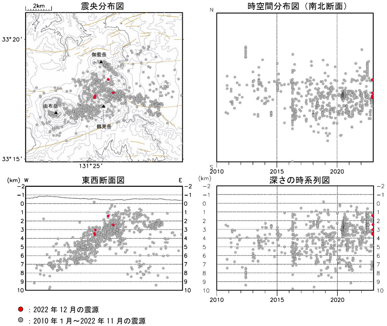
図3 鶴見岳・伽藍岳 震源分布図（2010年1月～2022年12月）
