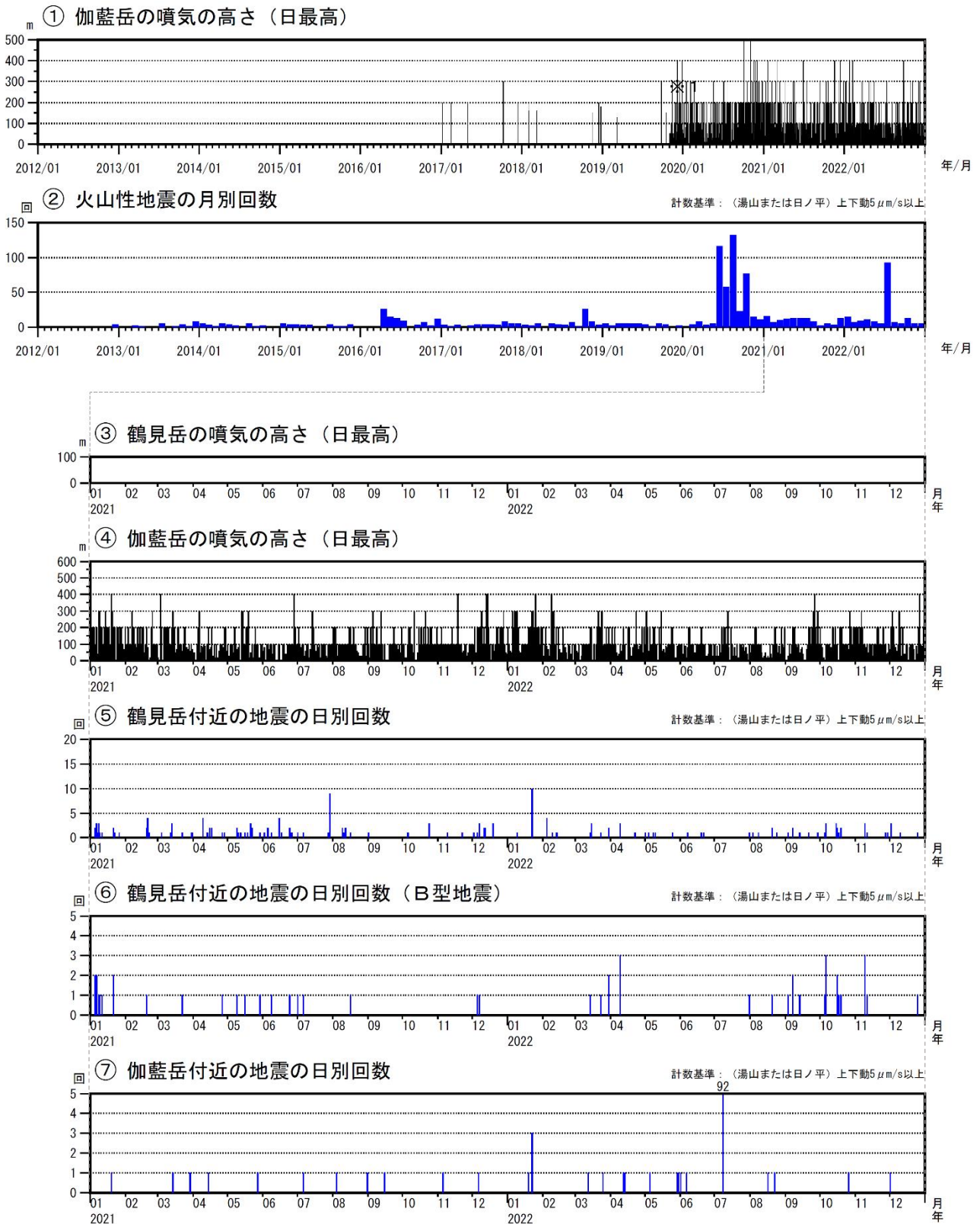
図2 鶴見岳・伽藍岳 火山活動経過図（2012年1月～2022年12月）
