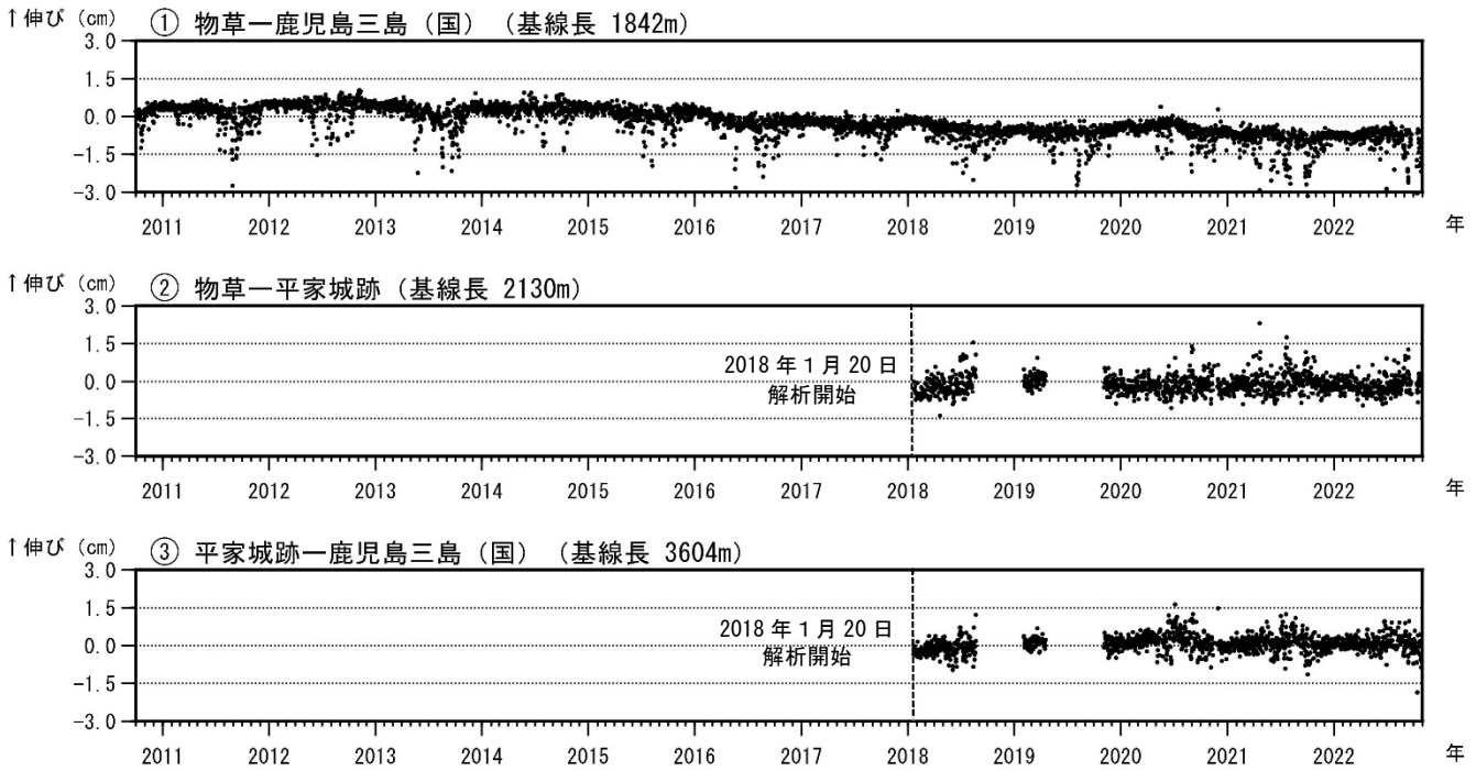
図5 薩摩硫黄島 GNSS連続観測による基線長変化 (2010年10月~2022年10月)
