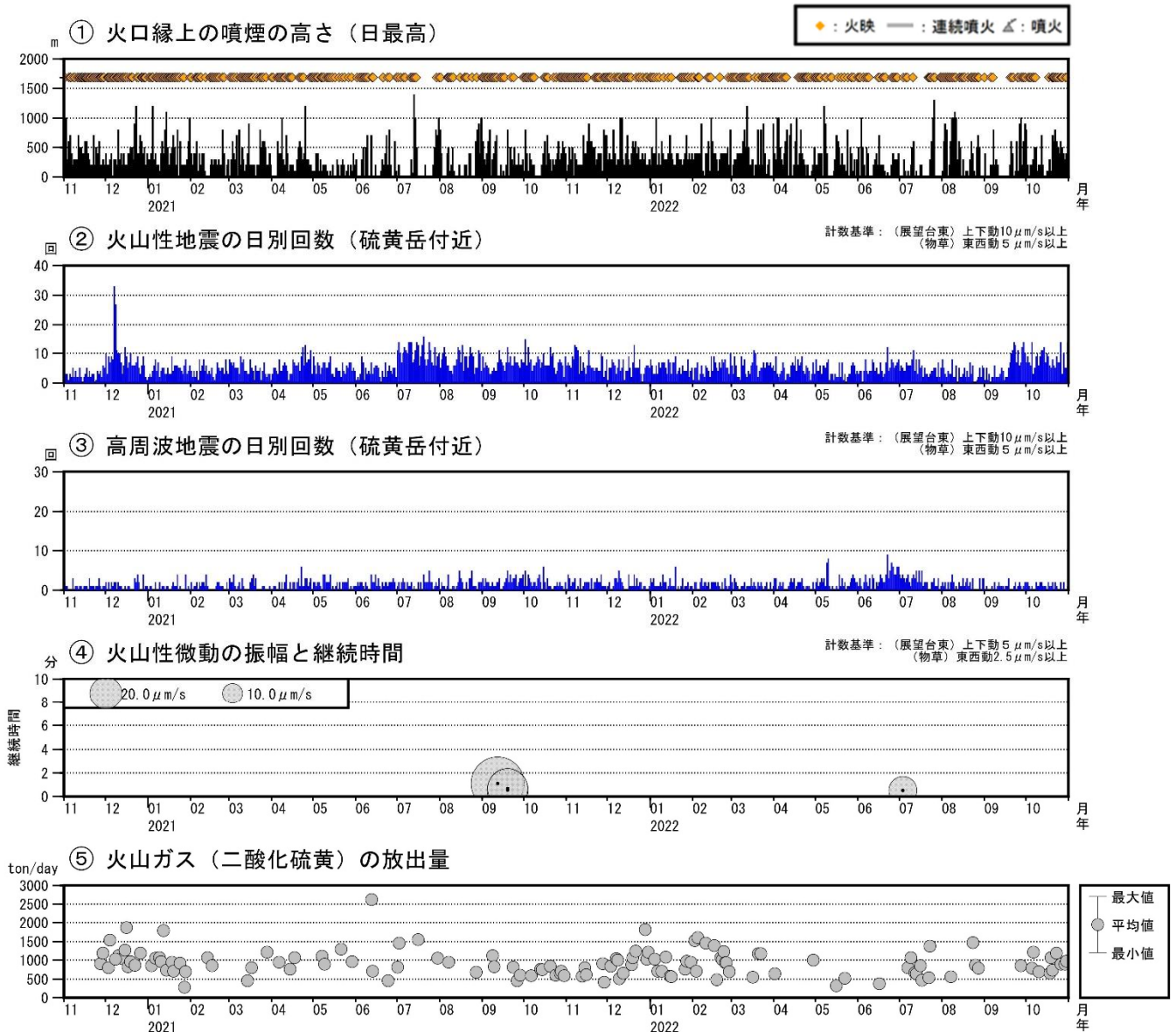
図4 薩摩硫黄島 火山活動経過図（2020年11月～2022年10月）
