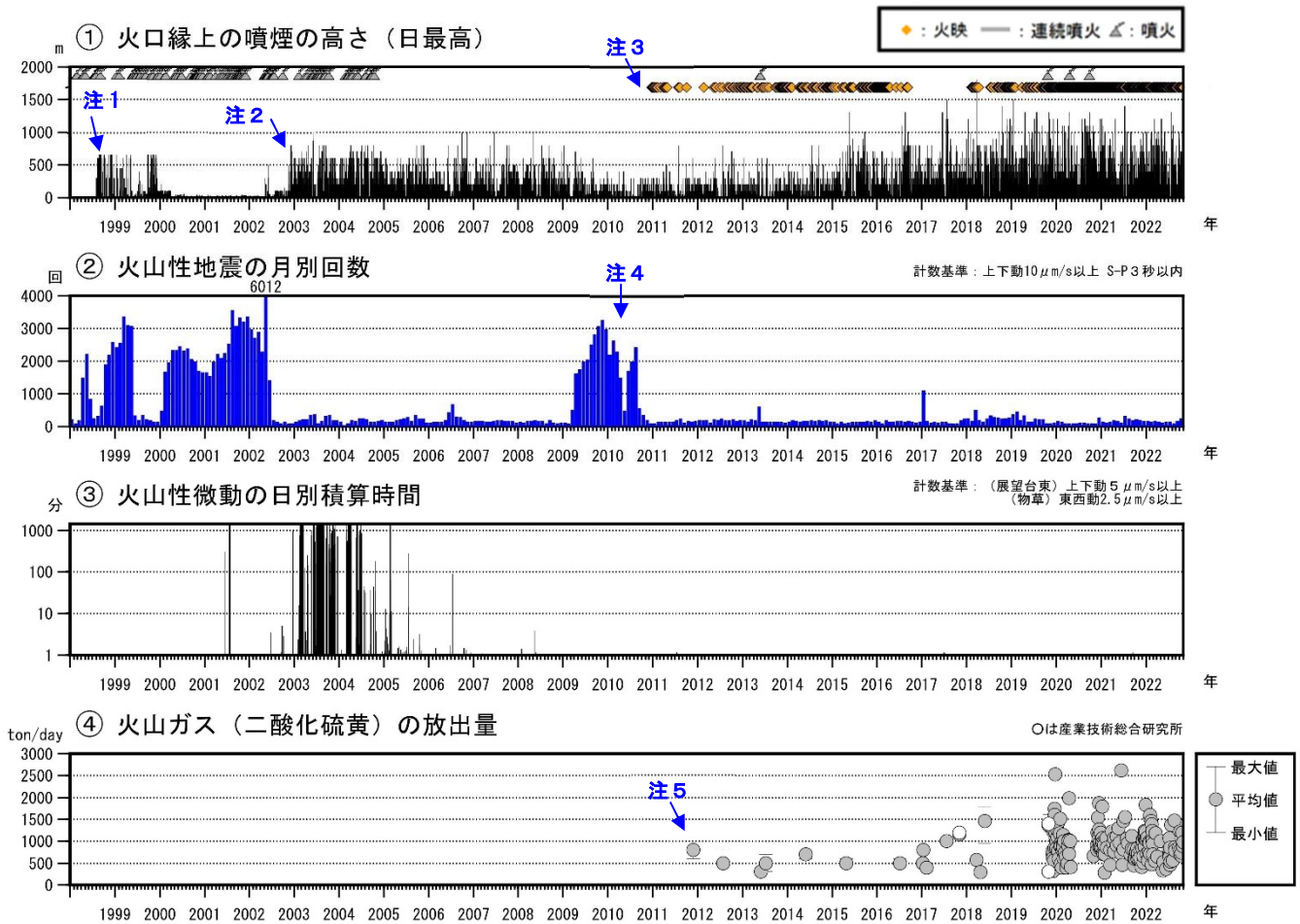
図3 薩摩硫黄島 火山活動経過図（1998年1月～2022年10月）
