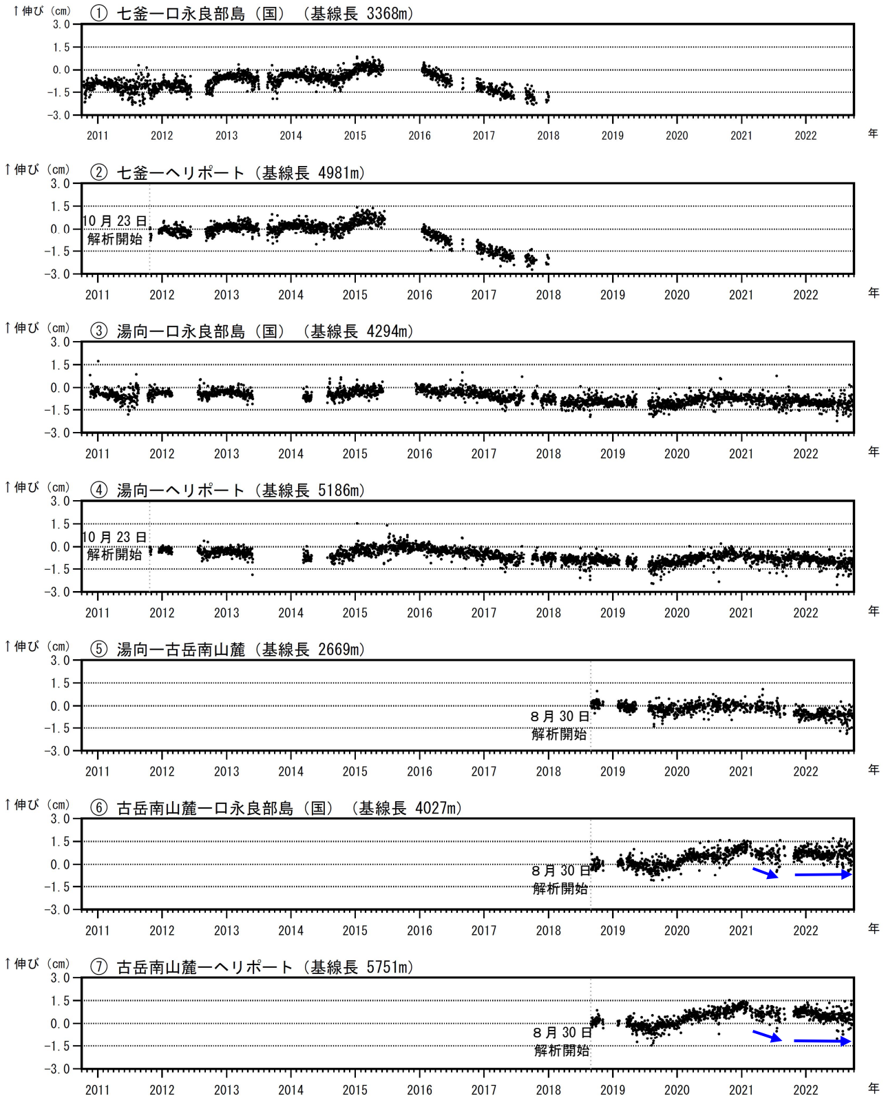
図8 口永良部島 GNSS 連続観測による基線長変化（2010年10月～2022年9月）
