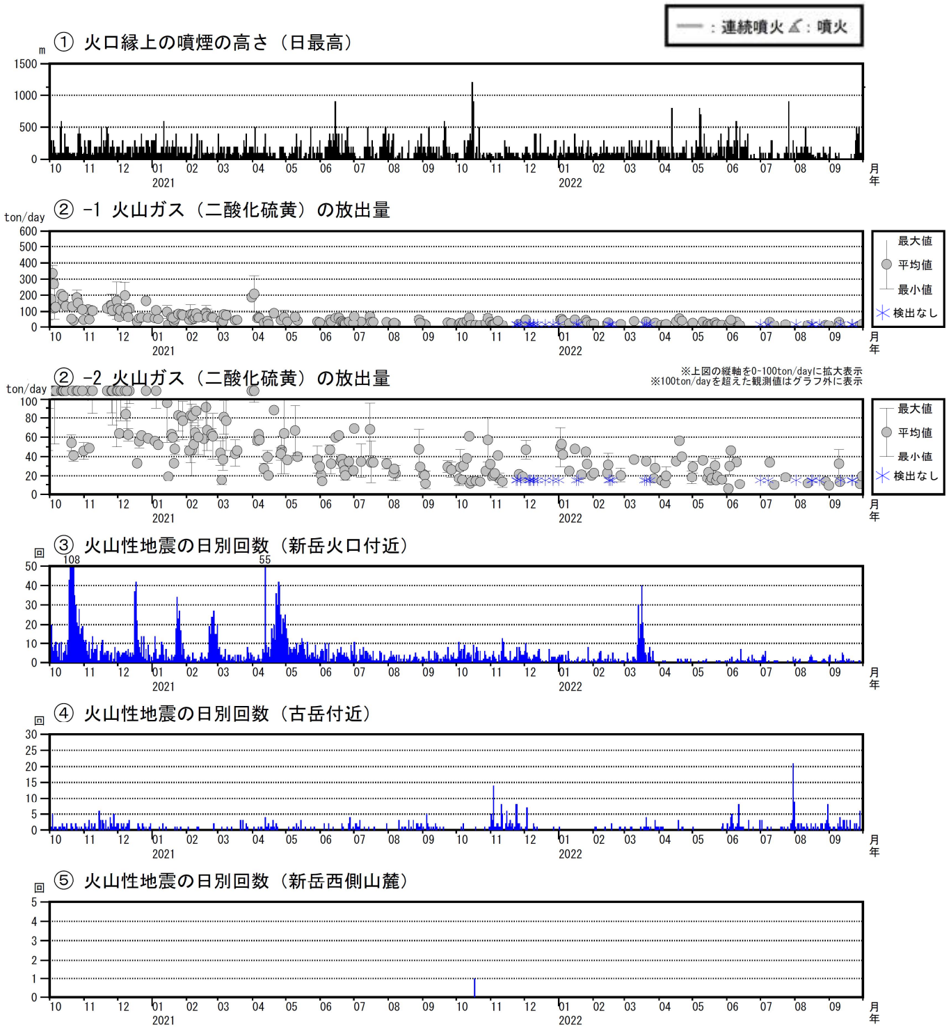
図6 口永良部島 最近の火山活動経過図（2020年10月～2022年9月）
