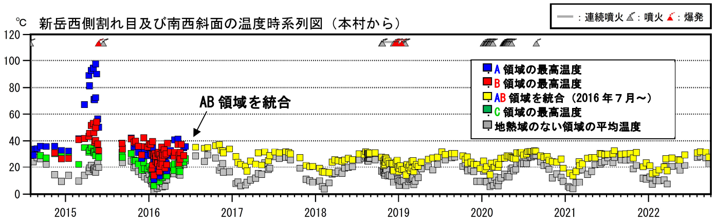
図3 口永良部島 新岳火口西側割れ目付近及び新岳南西側斜面の地熱域の温度時系列 (2014年8月～2022年9月)
