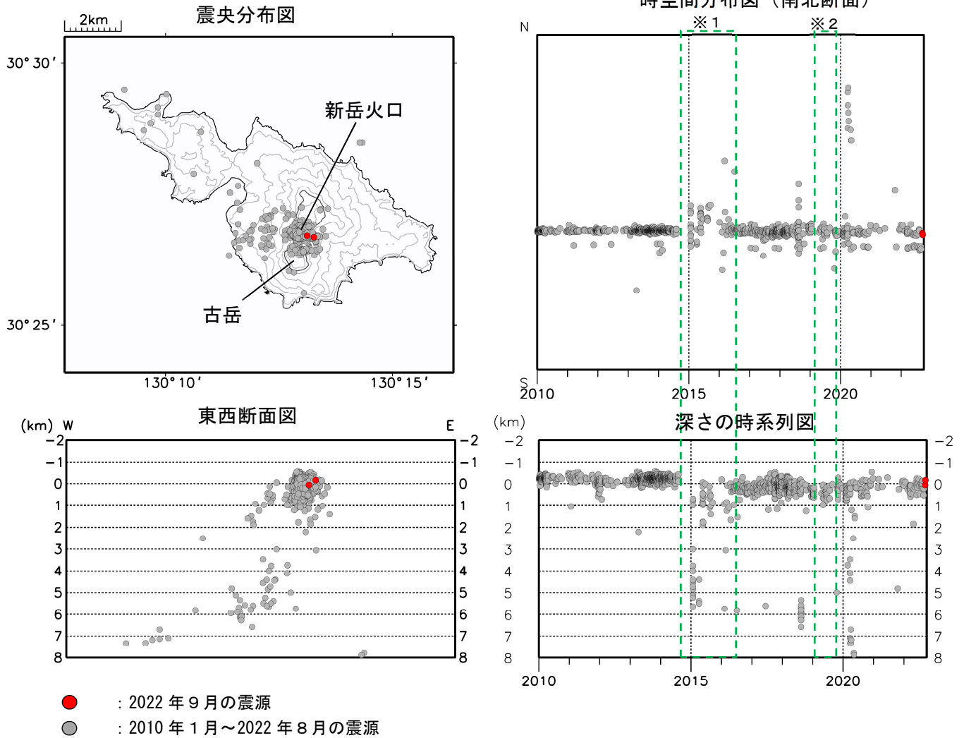
図7 口永良部島 震源分布図（2010年1月～2022年9月）
