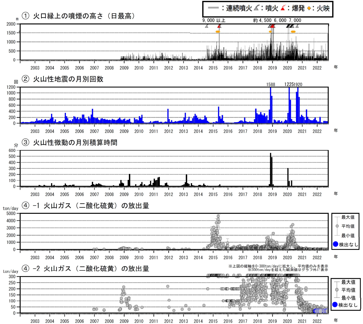
図5 口永良部島 火山活動経過図（2002年1月～2022年9月）
