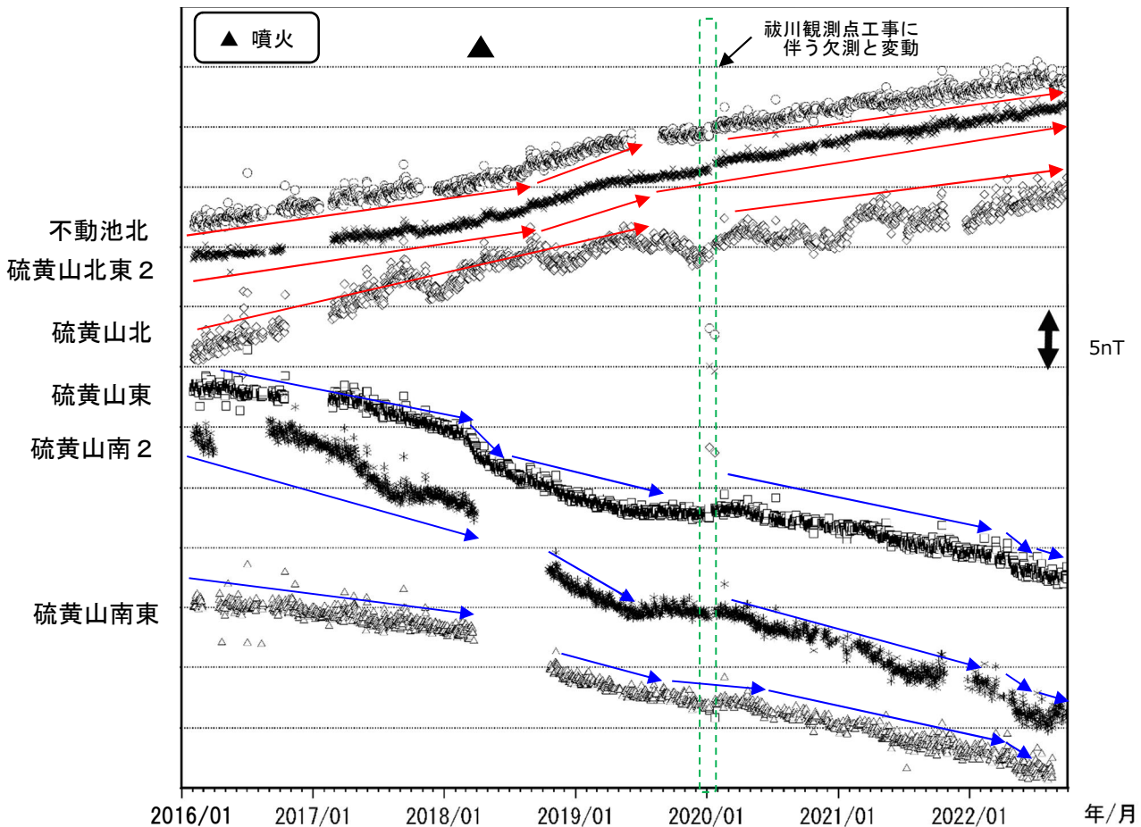
図 6-2 霧島山（えびの高原（硫黄山）周辺） 全磁力観測点で観測された全磁力変動（2016年1月～2022年9月）
