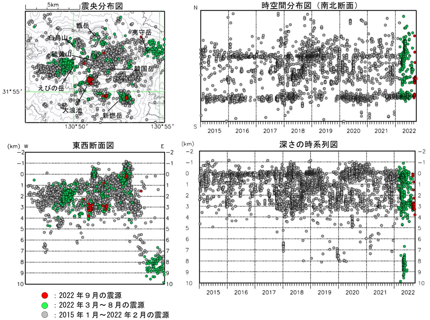
図 3-2 霧島山（新燃岳及びえびの高原（硫黄山）周辺） 震源分布図 （2015年1月～2022年9月）
