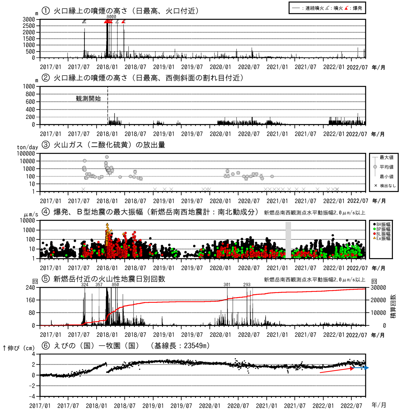
図2 霧島山（新燃岳） 火山活動経過図（2017年1月～2022年9月）
