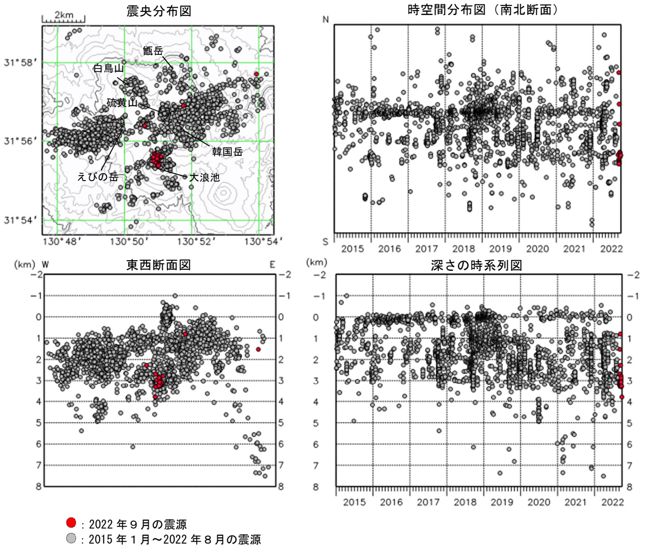
図3 霧島山（えびの高原（硫黄山）周辺）震源分布図（2015年1月～2022年9月）
