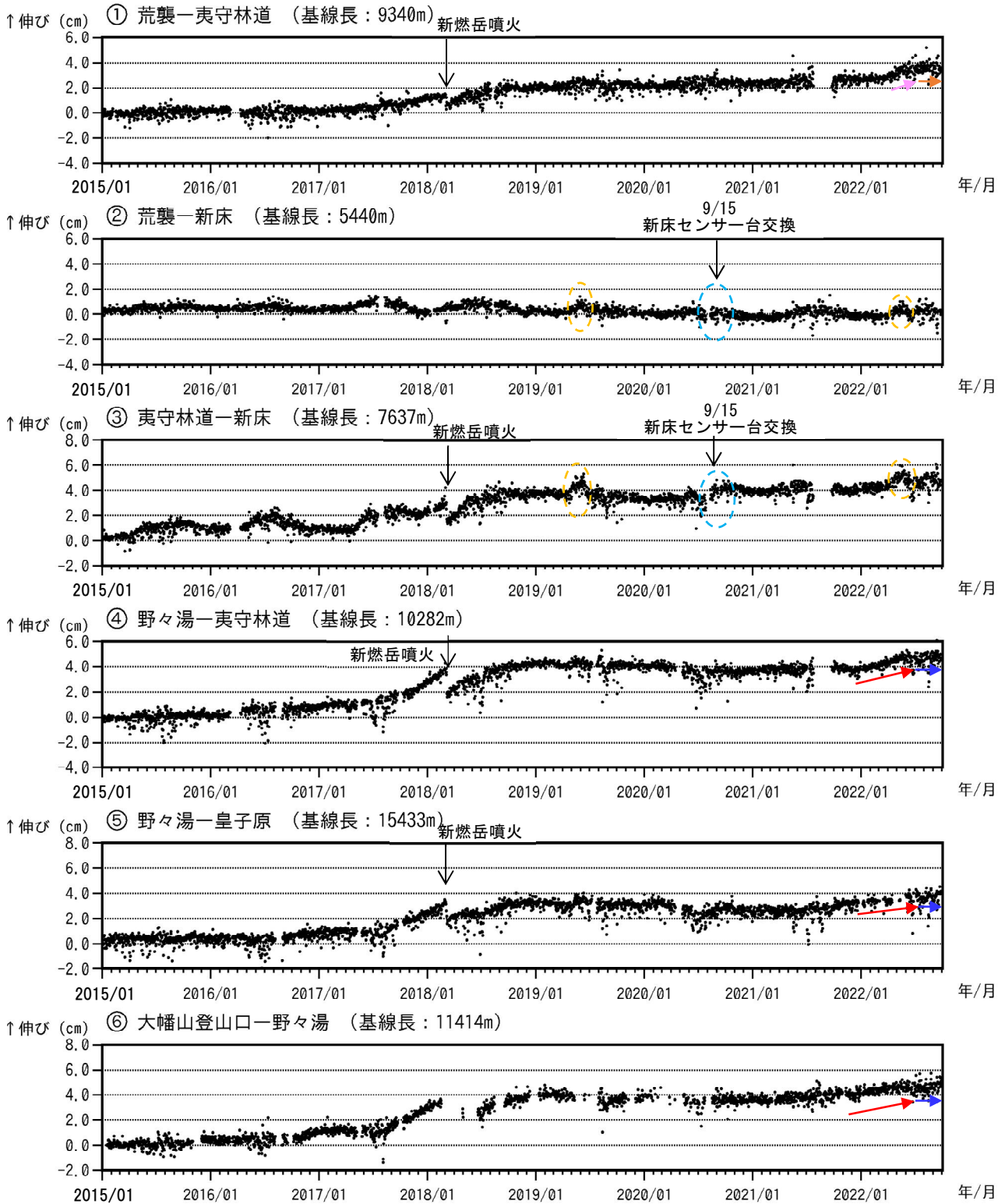
図4 霧島山（新燃岳） GNSS連続観測による基線長変化（2015年1月～2022年9月）
