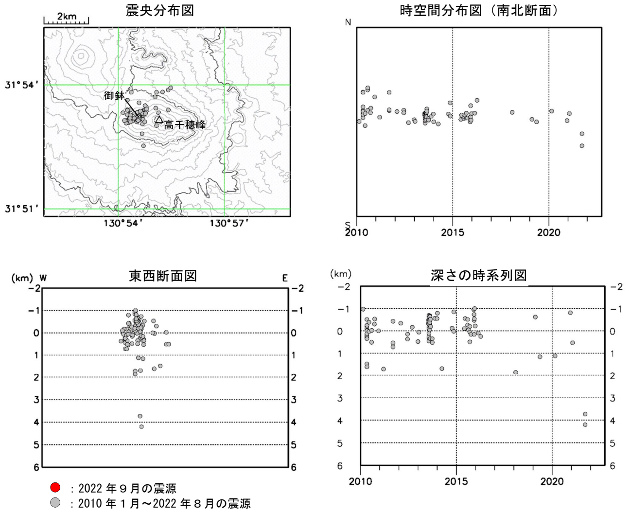
図3 霧島山（御鉢） 震源分布図（2010年1月～2022年9月）
