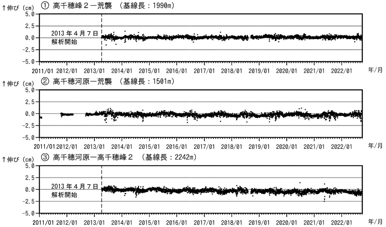
図4 霧島山（御鉢） GNSS 連続観測による基線長変化（2011年1月～2022年9月）
