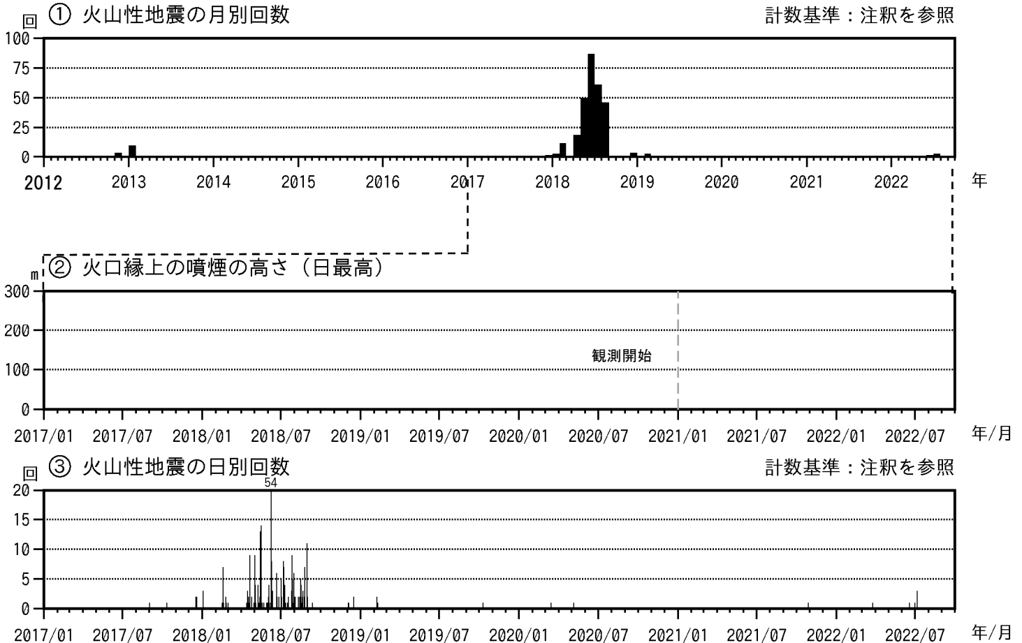
図2 霧島山（大幡池） 火山活動経過図（2012年1月～2022年9月）
