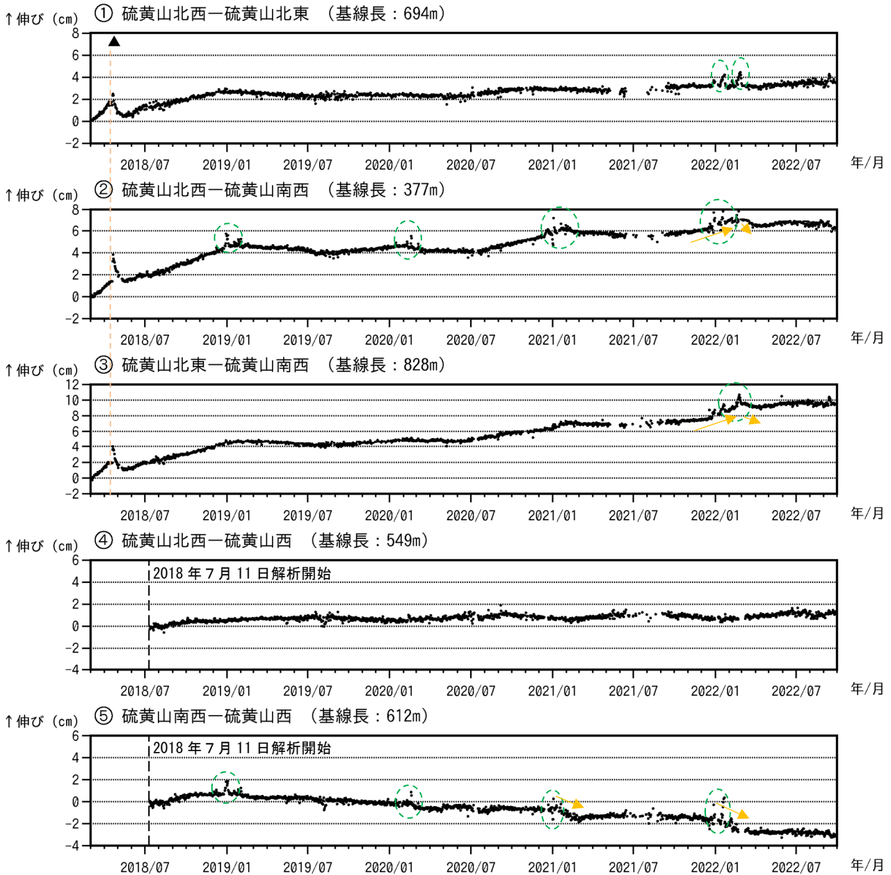
図4 霧島山（えびの高原（硫黄山）周辺） GNSS 連続観測による基線長変化 (2018年3月～2022年9月)
