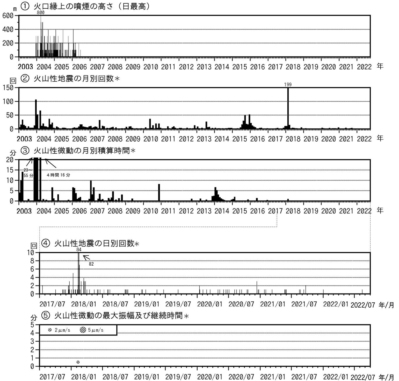
図2 霧島山（御鉢） 火山活動経過図（2003年1月～2022年9月）
