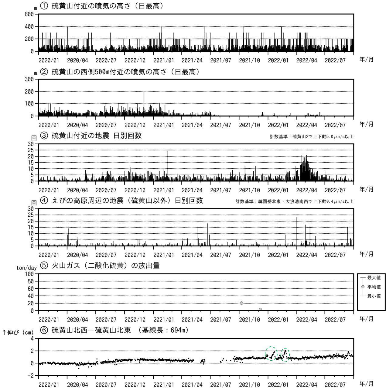
図2 霧島山（えびの高原（硫黄山）周辺） 火山活動経過図（2020年1月～2022年9月）
