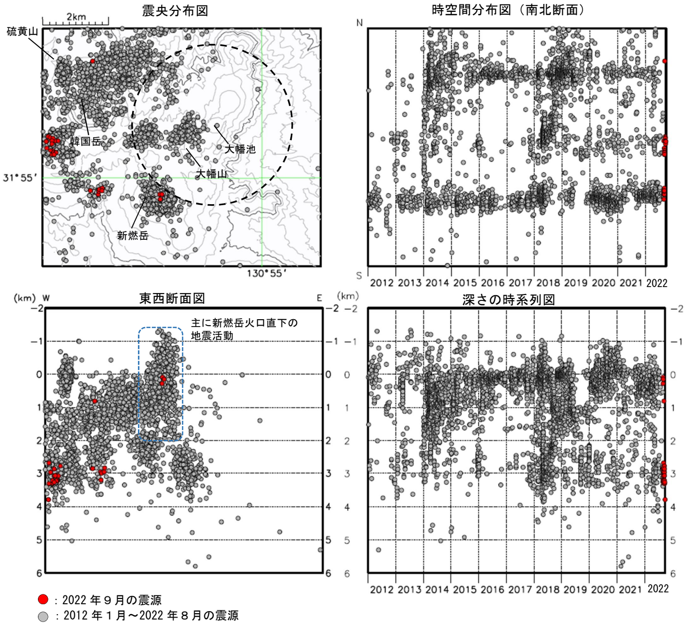
図3 霧島山（大幡池） 震源分布図（2012年1月～2022年9月）
