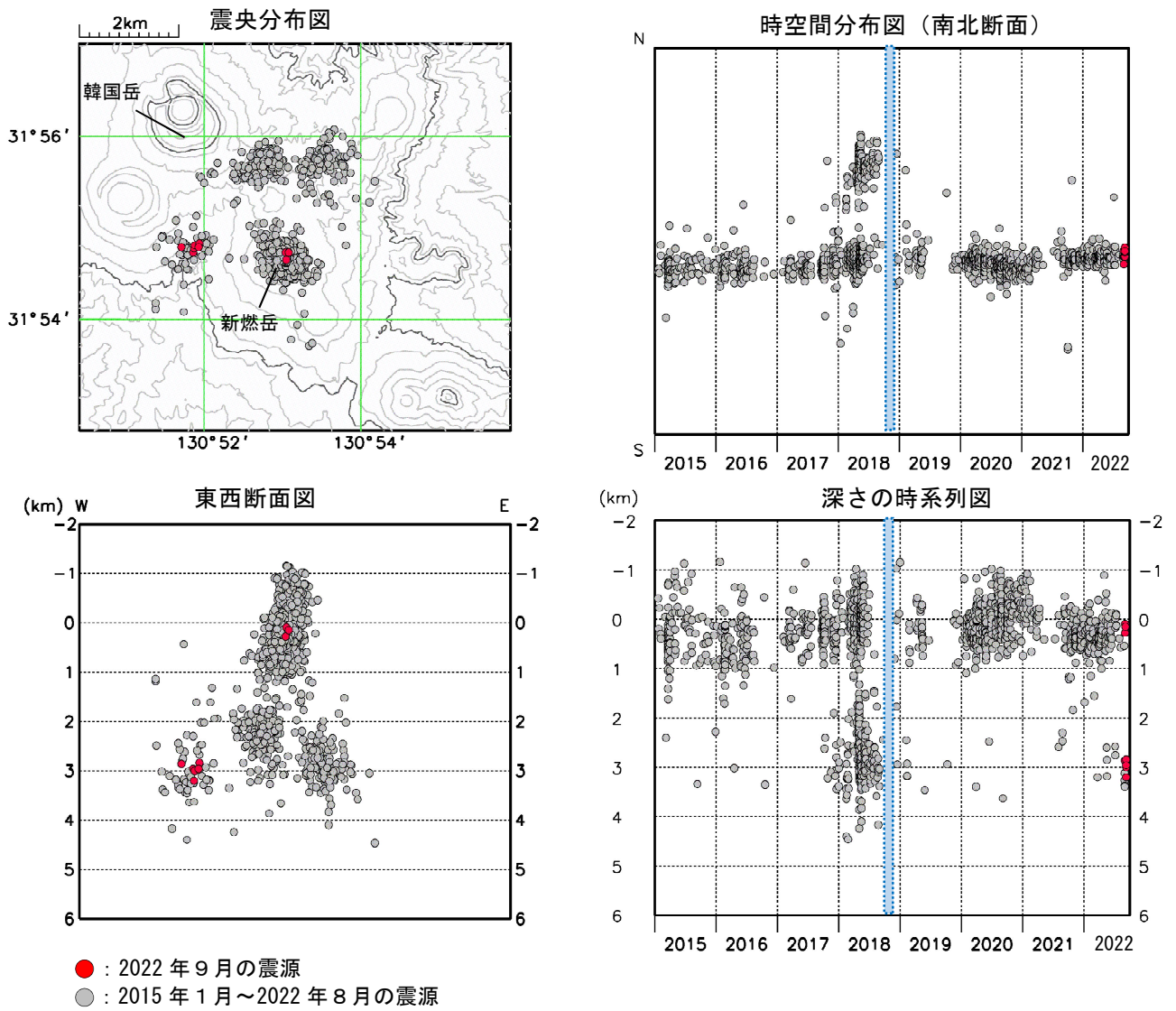
図 3-1 霧島山（新燃岳） 震源分布図（2015年1月～2022年9月）
