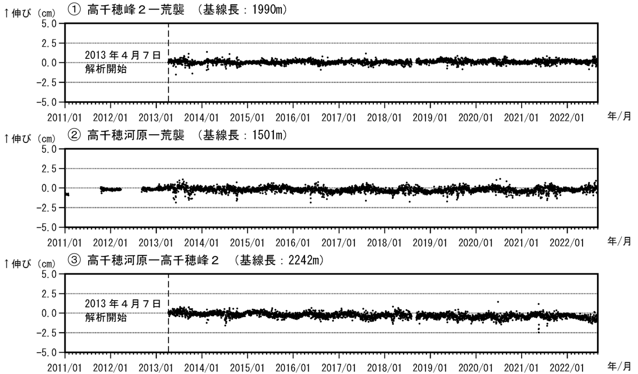
図4 霧島山（御鉢） GNSS 連続観測による基線長変化（2011年1月～2022年8月）
