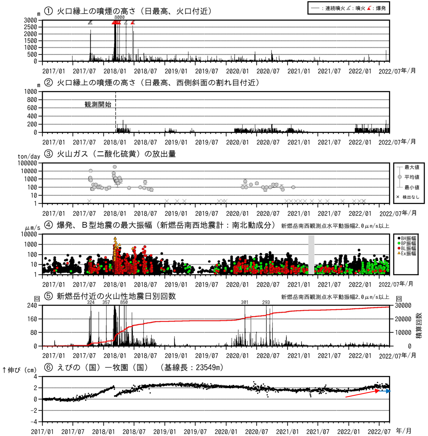
図4 霧島山（新燃岳） 火山活動経過図（2017年1月～2022年8月）
