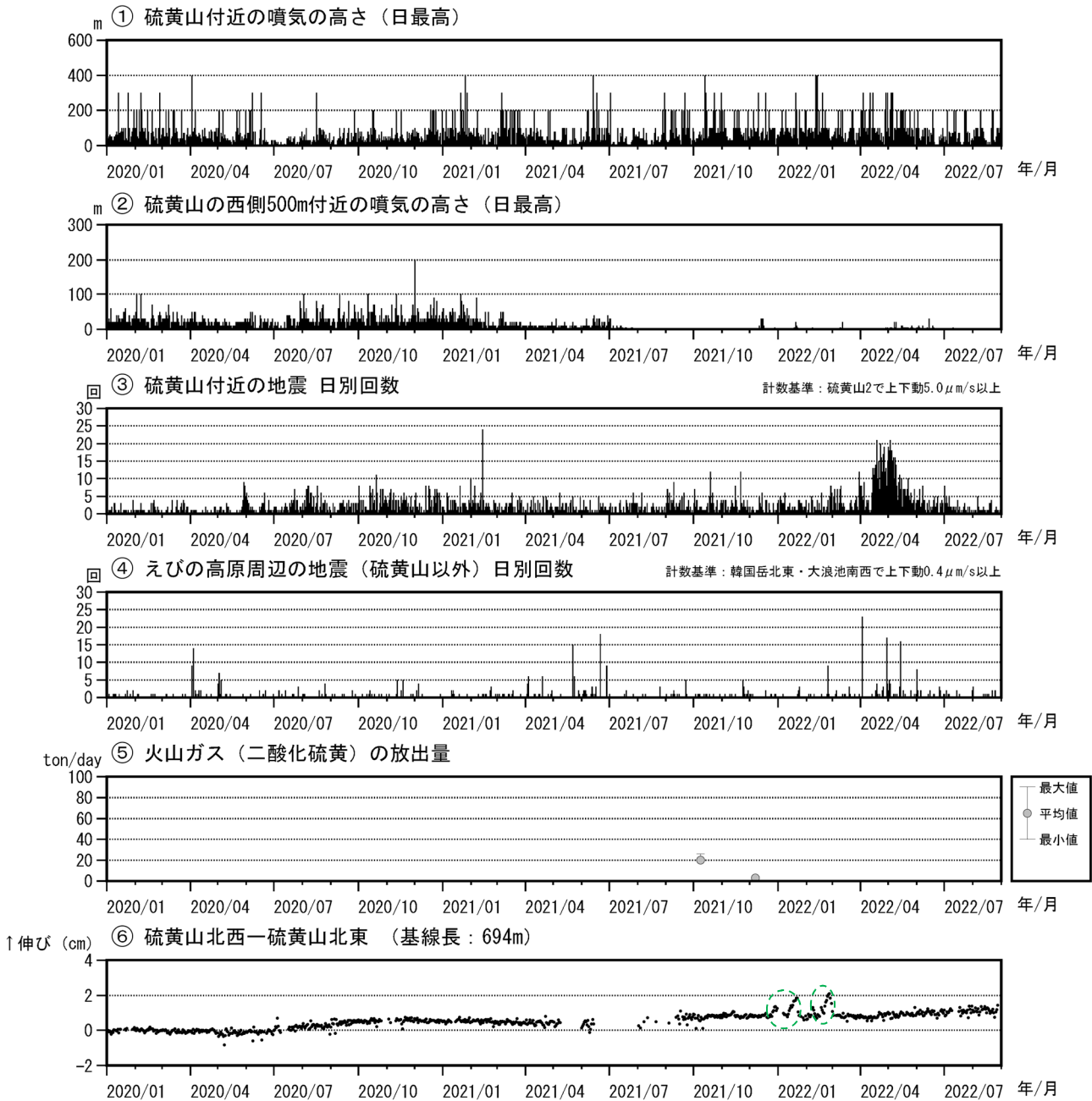
図2 霧島山（えびの高原（硫黄山）周辺） 火山活動経過図（2020年1月～2022年8月）
