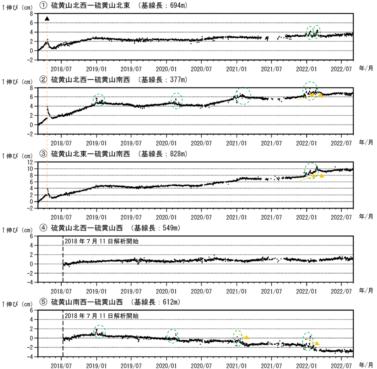
図4 霧島山（えびの高原（硫黄山）周辺） GNSS 連続観測による基線長変化 (2018年3月～2022年8月)
