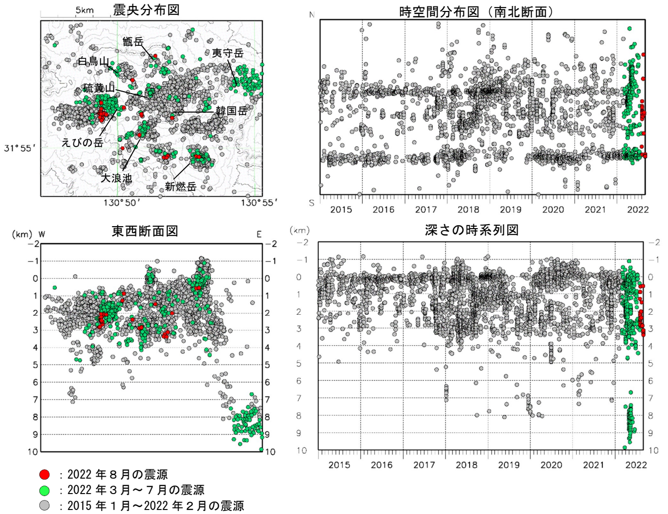
図 5-2 霧島山（新燃岳及びえびの高原（硫黄山）周辺） 震源分布図 (2015年1月～2022年8月)
