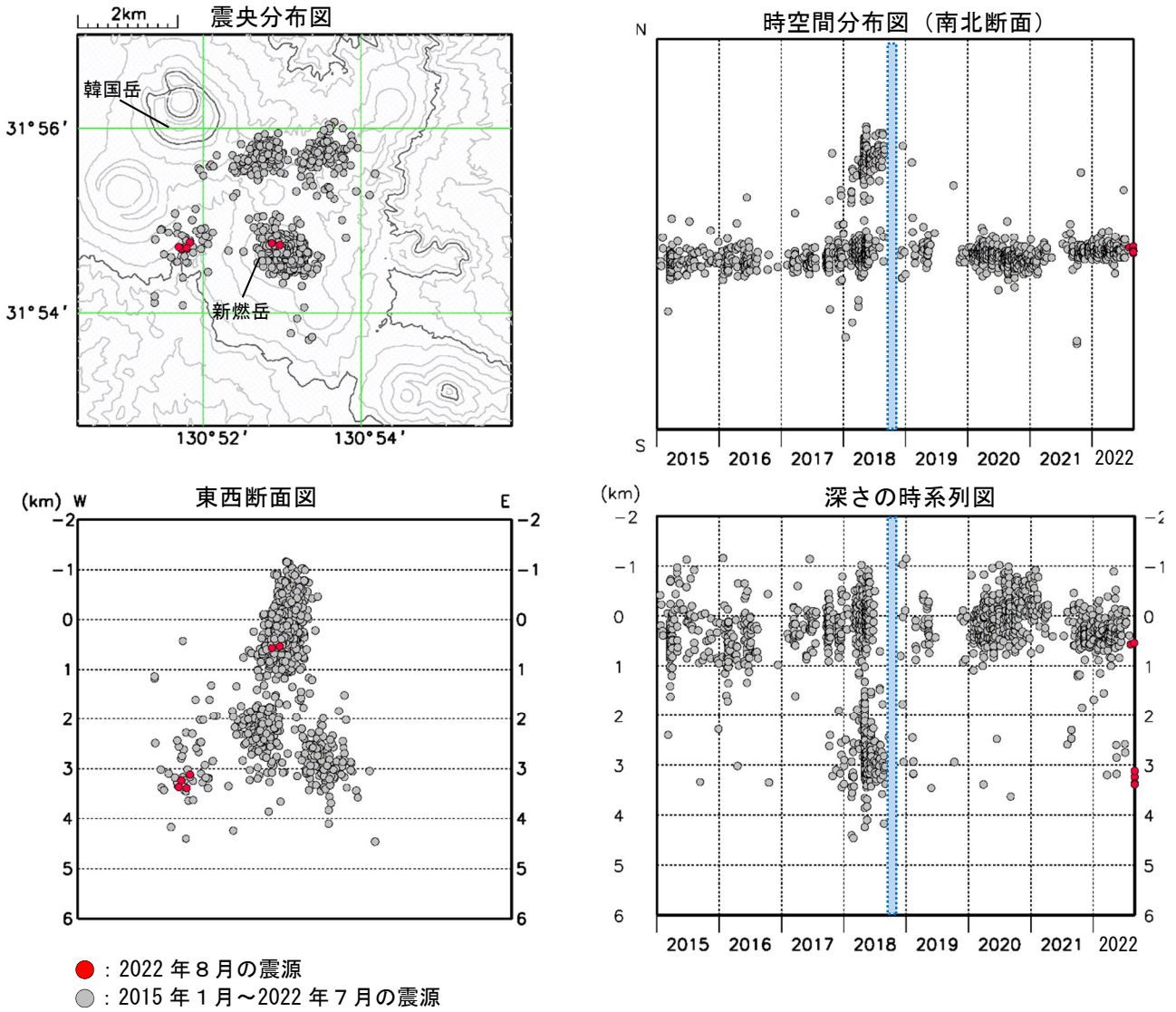
図 5-1 霧島山（新燃岳） 震源分布図（2015年1月～2022年8月）
