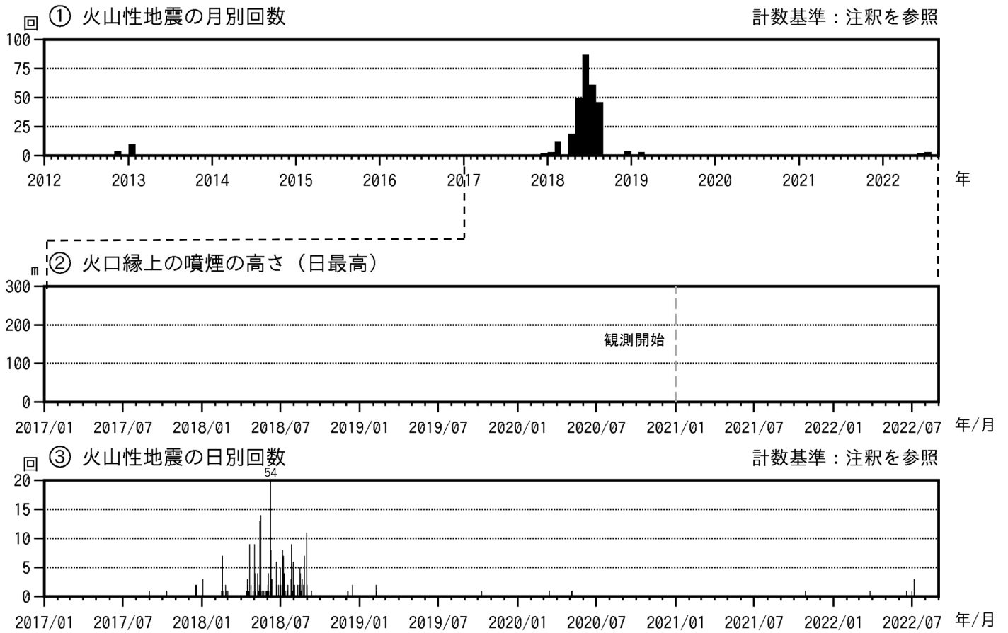
図2 霧島山（大幡池） 火山活動経過図（2012年1月～2022年8月）
