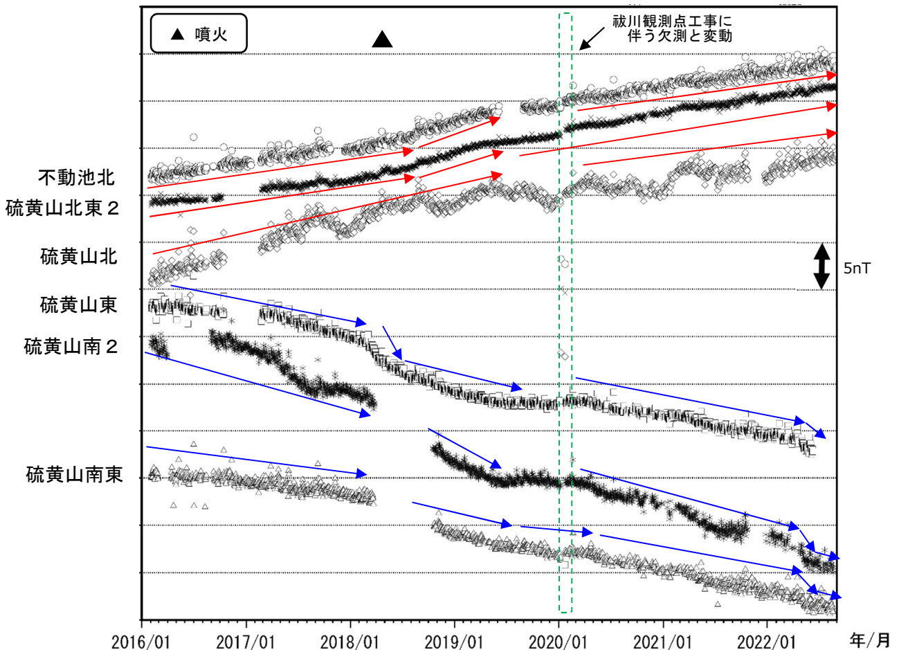
図 6-2 霧島山（えびの高原（硫黄山）周辺） 全磁力観測点で観測された全磁力変動（2016年1月～2022年8月）
