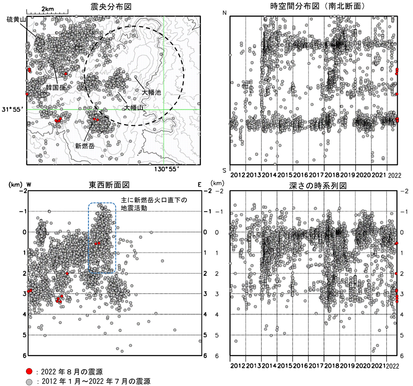
図3 霧島山（大幡池） 震源分布図（2012年1月～2022年8月）
