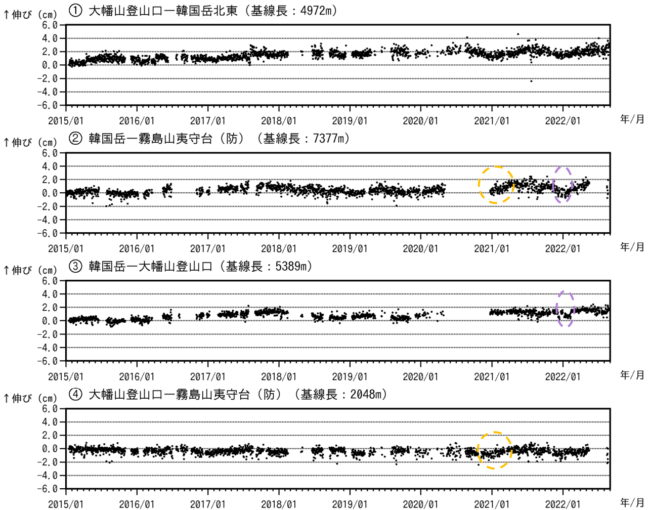
図4 霧島山（大幡池） GNSS 連続観測による基線長変化（2015年1月～2022年8月）
