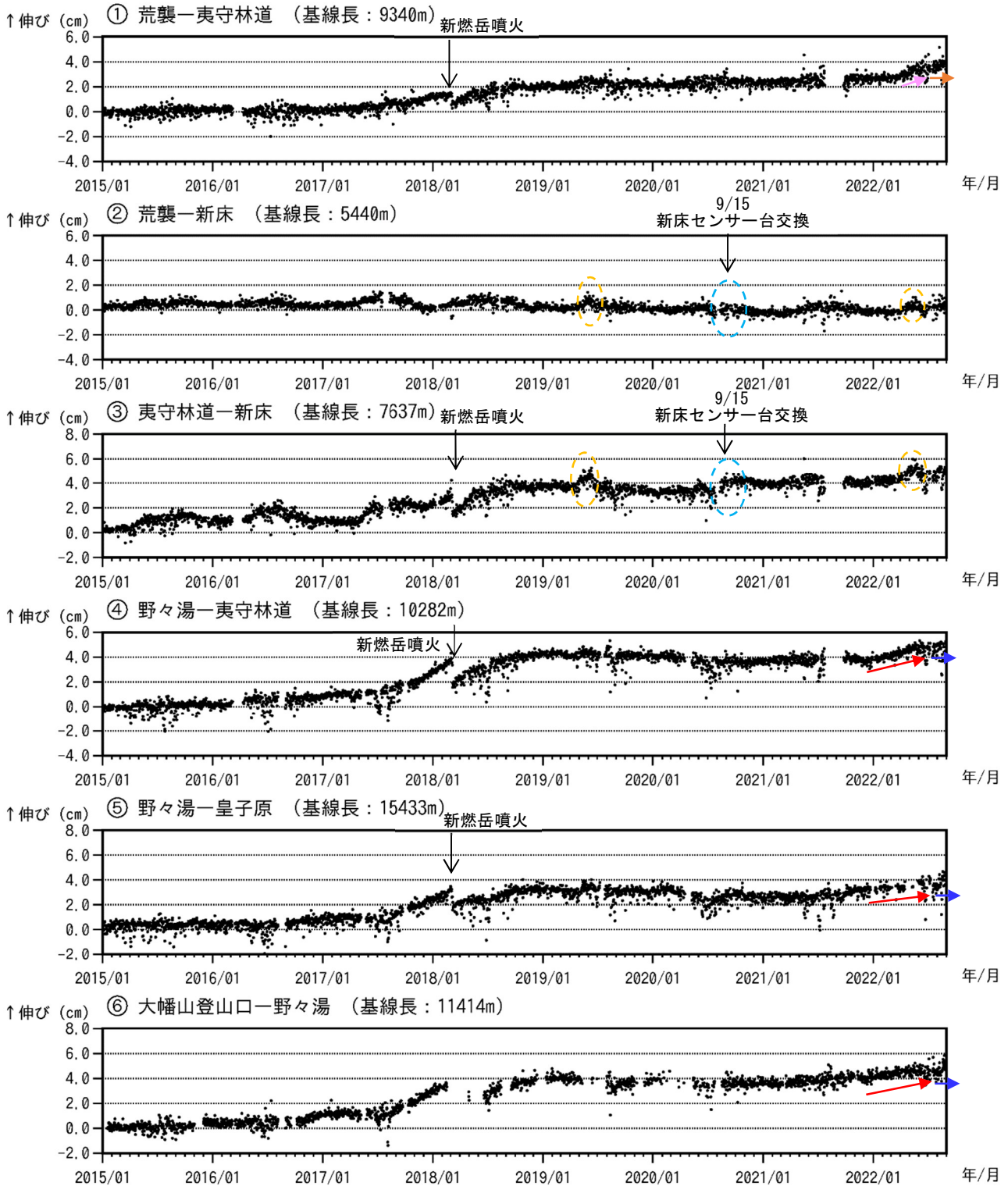
図6 霧島山（新燃岳） GNSS連続観測による基線長変化（2015年1月～2022年8月）
