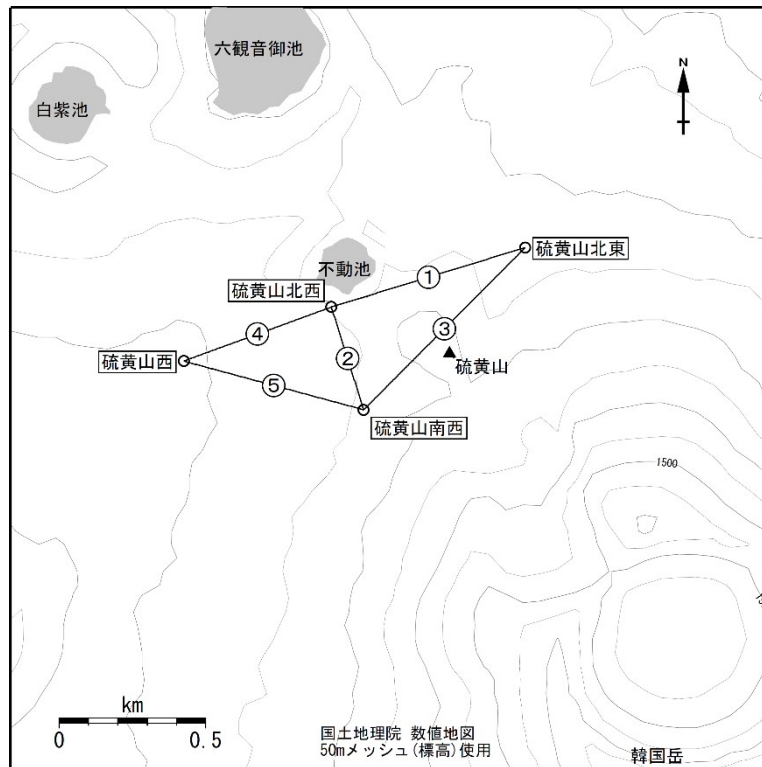
図5 霧島山（えびの高原（硫黄山）周辺） 図2及び図4のGNSS連続観測点と基線番号 小さな白丸（○）は気象庁の観測点位置を示しています。
