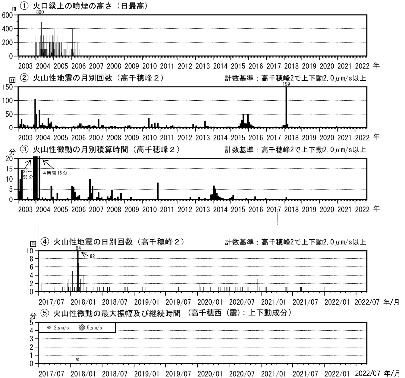
図2 霧島山（御鉢） 火山活動経過図（2003年1月～2022年8月）
