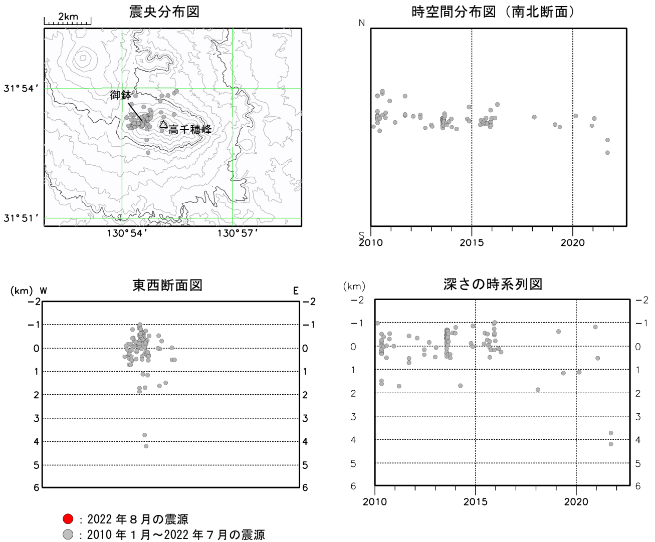
図3 霧島山（御鉢） 震源分布図（2010年1月～2022年8月）
