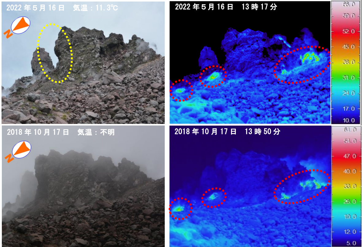
図 3-1 赤外熱映像装置による平成新山の地表面温度分布および可視画像（平成新山山腹から観測）
