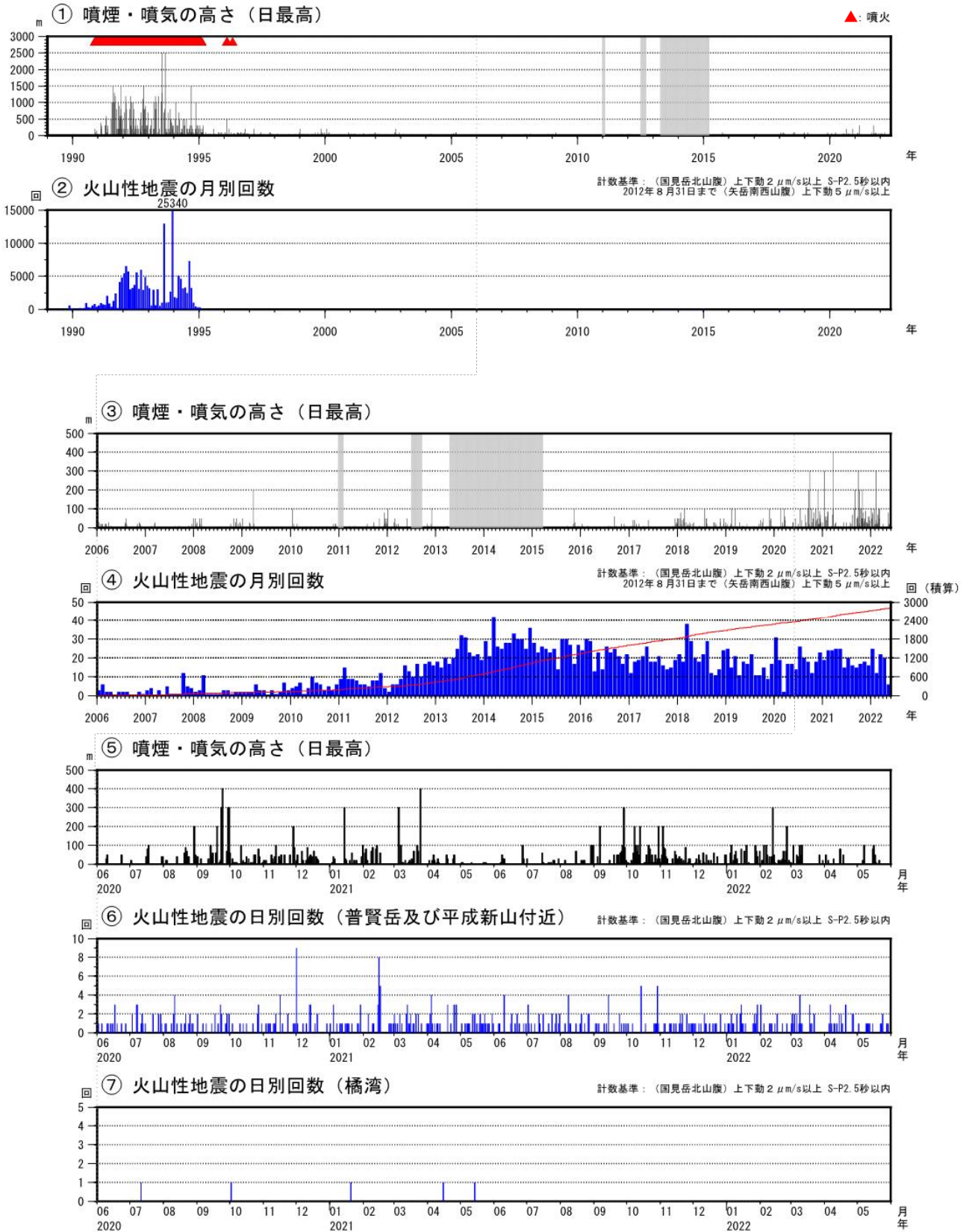
図4 雲仙岳 火山活動経過図（1989年1月～2022年5月）
