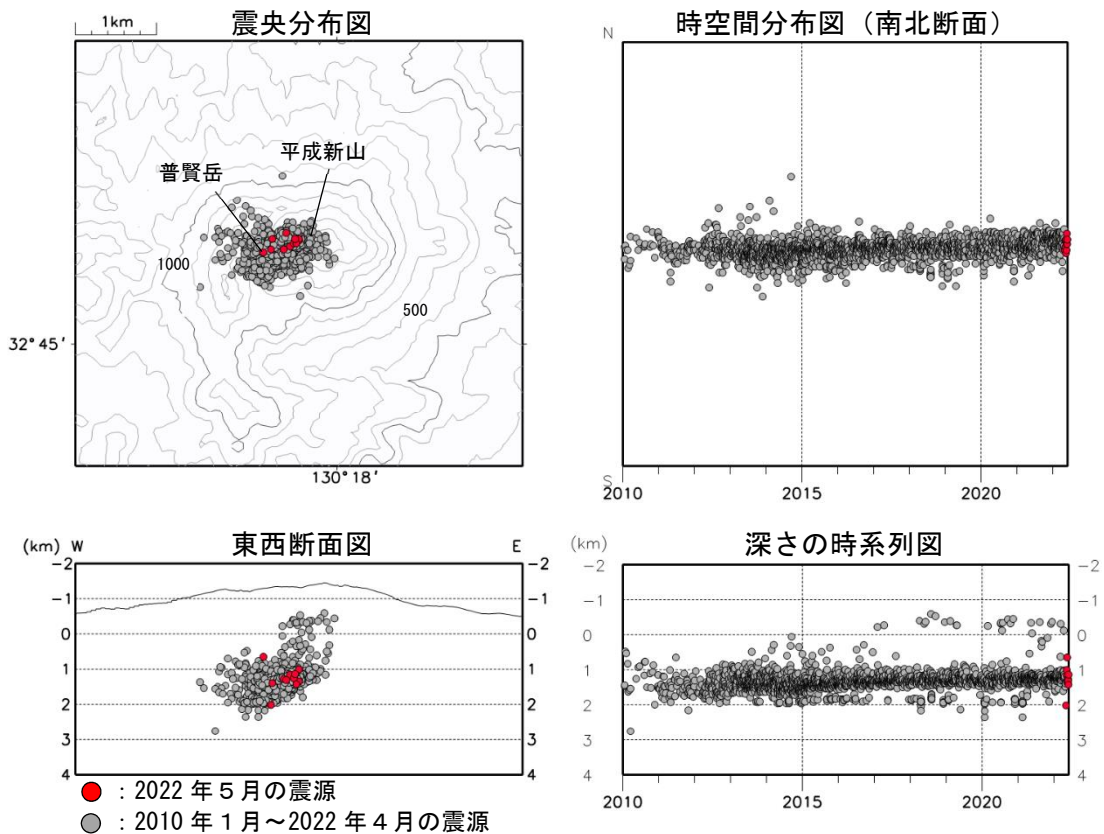
図 5-2 雲仙岳 震源分布図（普賢岳・平成新山付近の地震）（2010年1月～2022年5月）
