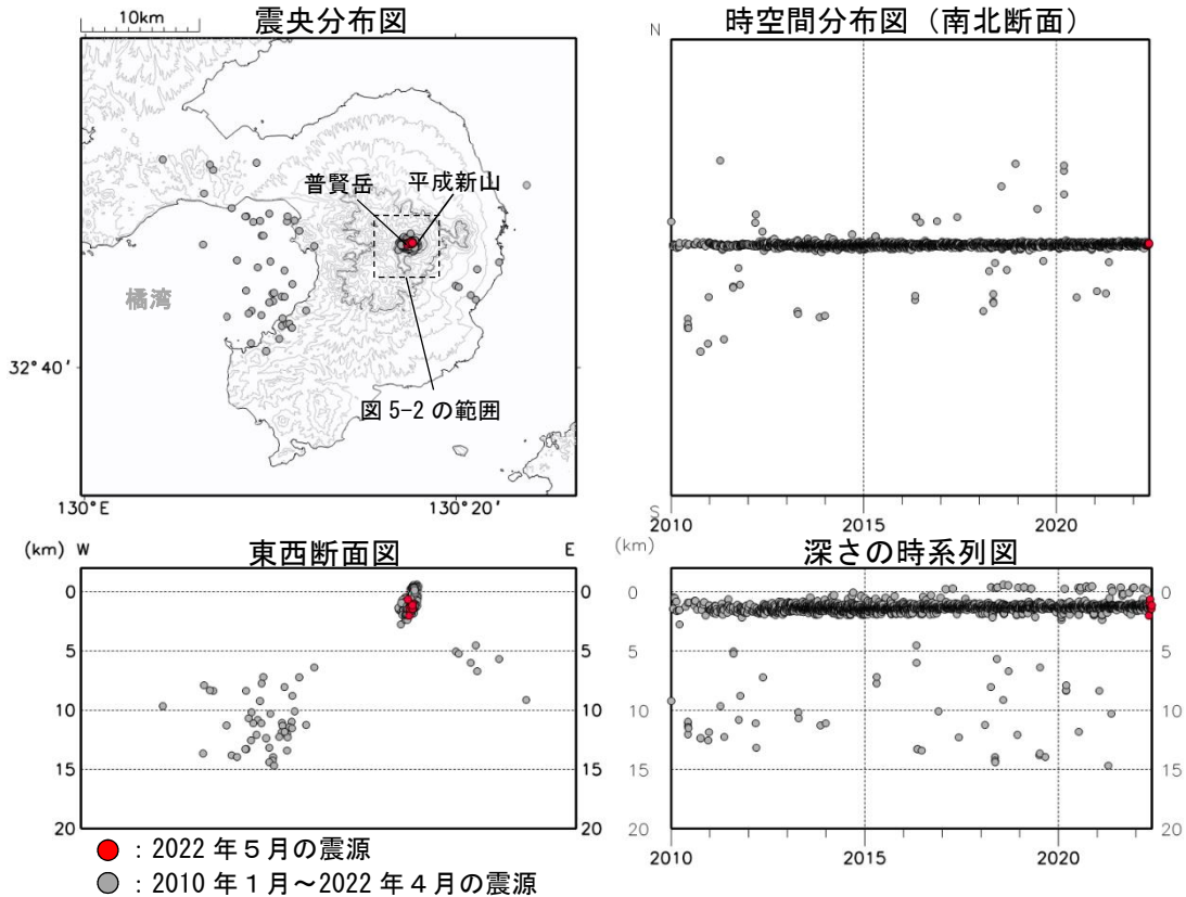
図 5-1 雲仙岳 震源分布図（広域）（2010年1月～2022年5月）
