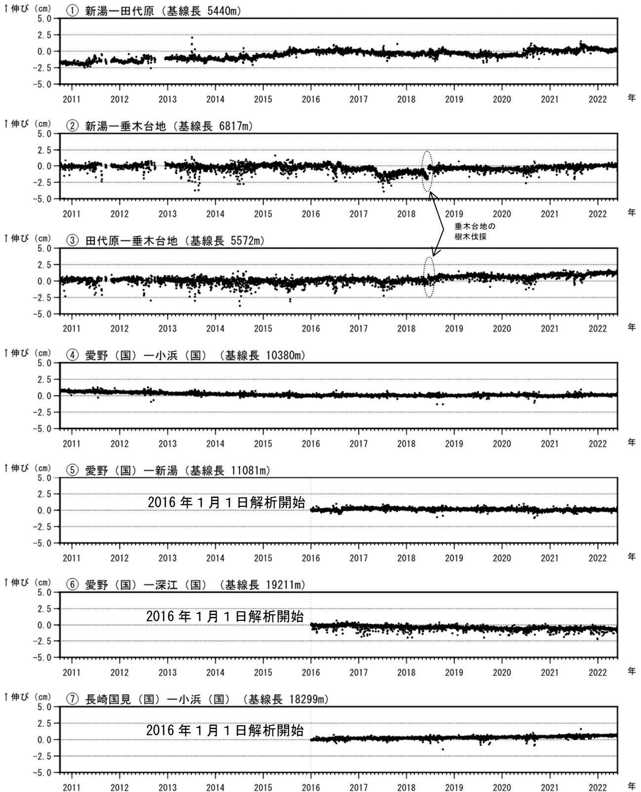
図6 雲仙岳 GNSS連続観測による基線長変化（2010年10月～2022年5月）
