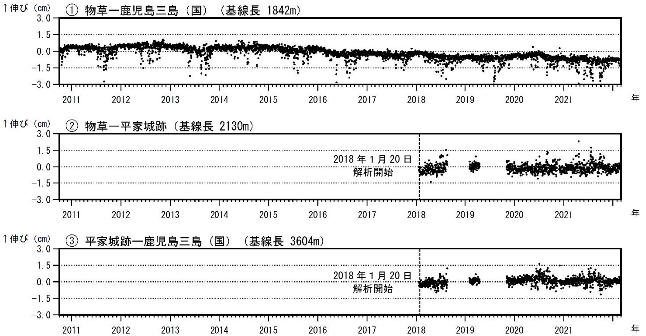
図6 薩摩硫黄島 GNSS連続観測による基線長変化 (2010年10月～2022年2月)
