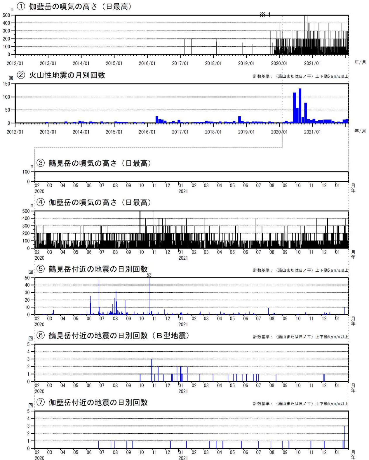
図2 鶴見岳・伽藍岳 火山活動経過図（2012年1月～2022年1月）
