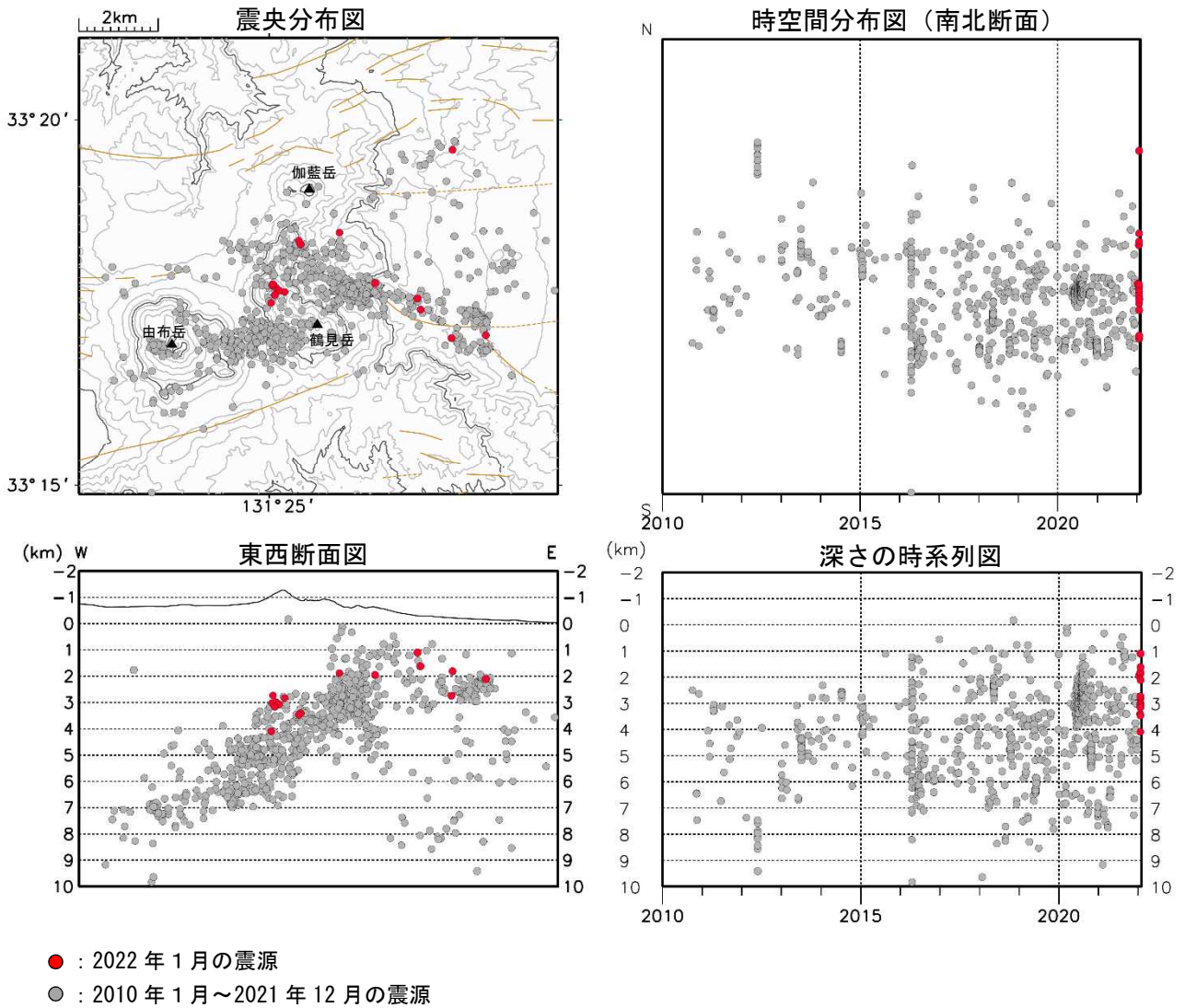
図3 鶴見岳・伽藍岳 震源分布図（2010年1月～2022年1月）
