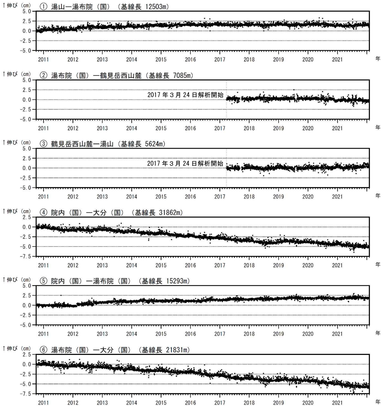
図4 鶴見岳・伽藍岳 GNSS連続観測による基線長変化（2010年10月～2022年1月）
