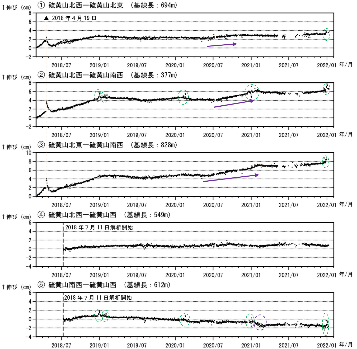
図4 霧島山（えびの高原（硫黄山）周辺） GNSS 連続観測による基線長変化 （2018年3月～2022年1月）
