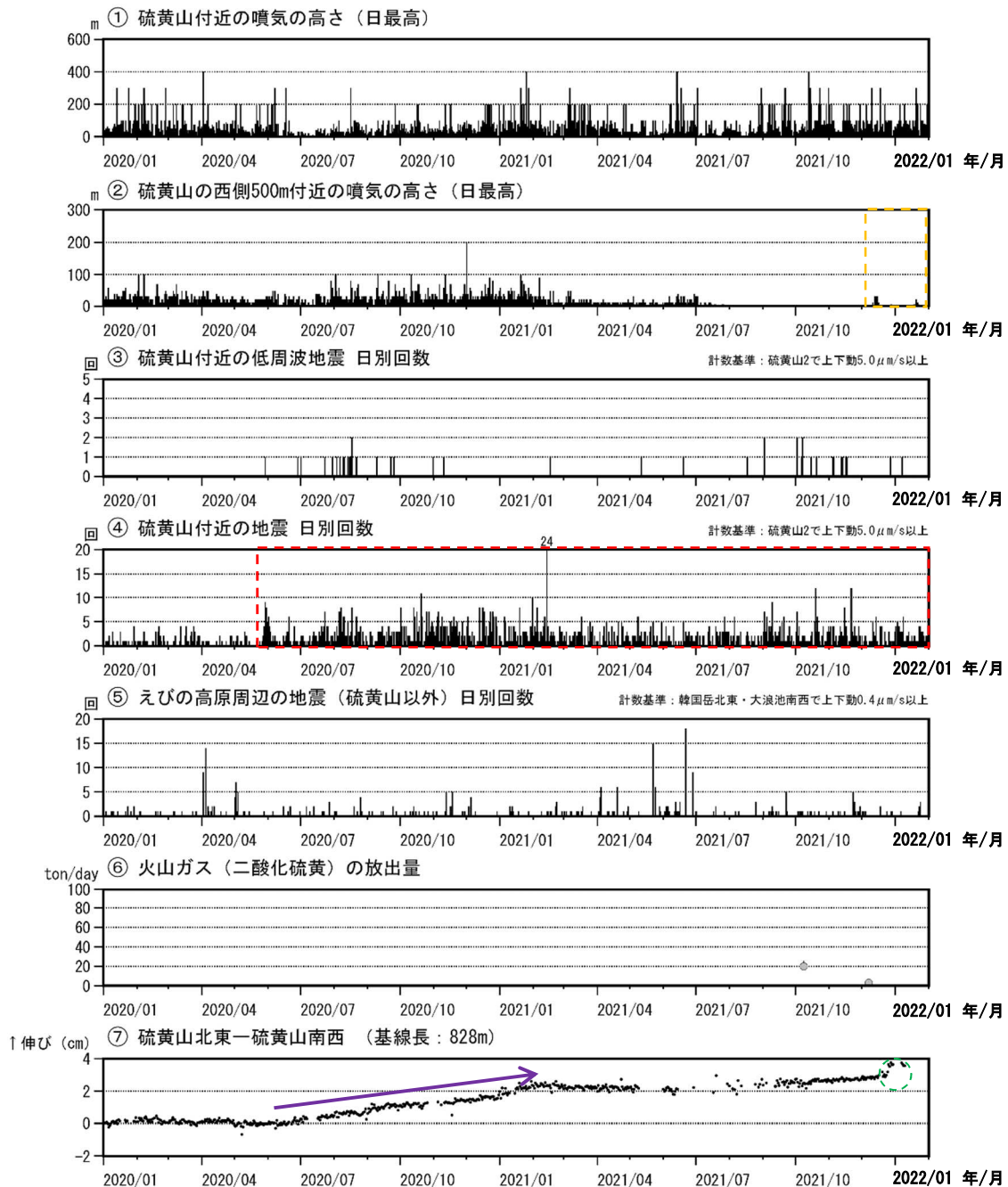
図3 霧島山（えびの高原（硫黄山）周辺） 火山活動経過図（2020年1月～2022年1月）
