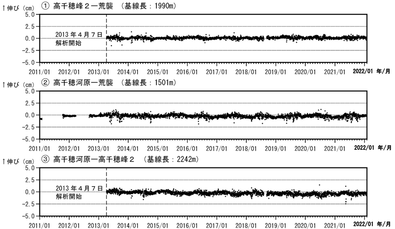
図4 霧島山（御鉢） GNSS 連続観測による基線長変化（2011年1月～2022年1月）
