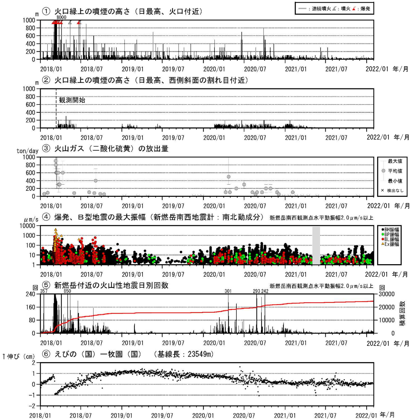
図4 霧島山（新燃岳） 火山活動経過図（2018年1月～2022年2月1日）
