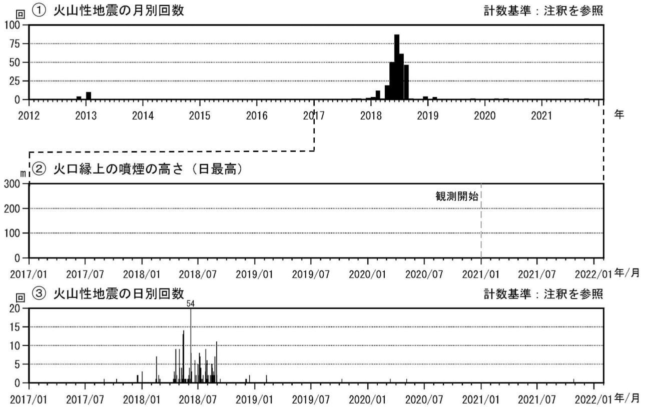
図2 霧島山（大幡池） 火山活動経過図（2012年1月～2022年1月）
