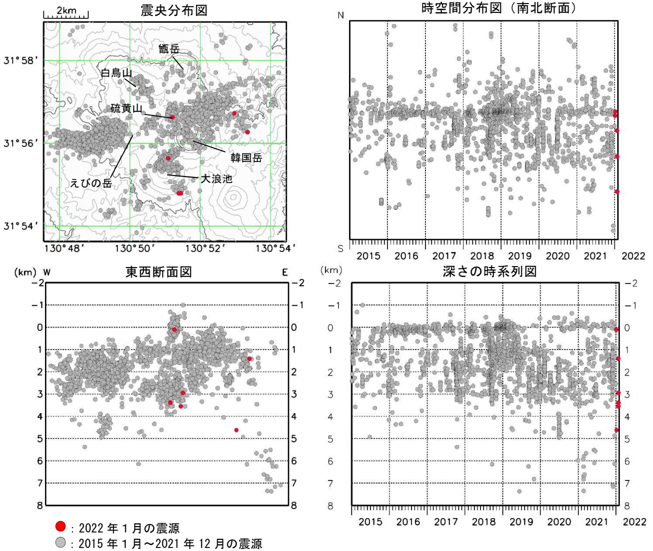
図2 霧島山（えびの高原（硫黄山）周辺） 震源分布図（2015年1月～2022年1月）
