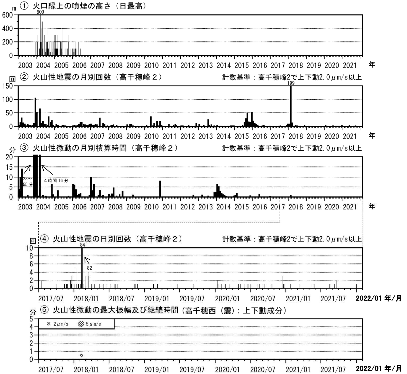
図2 霧島山（御鉢） 火山活動経過図（2003年1月～2022年1月）
