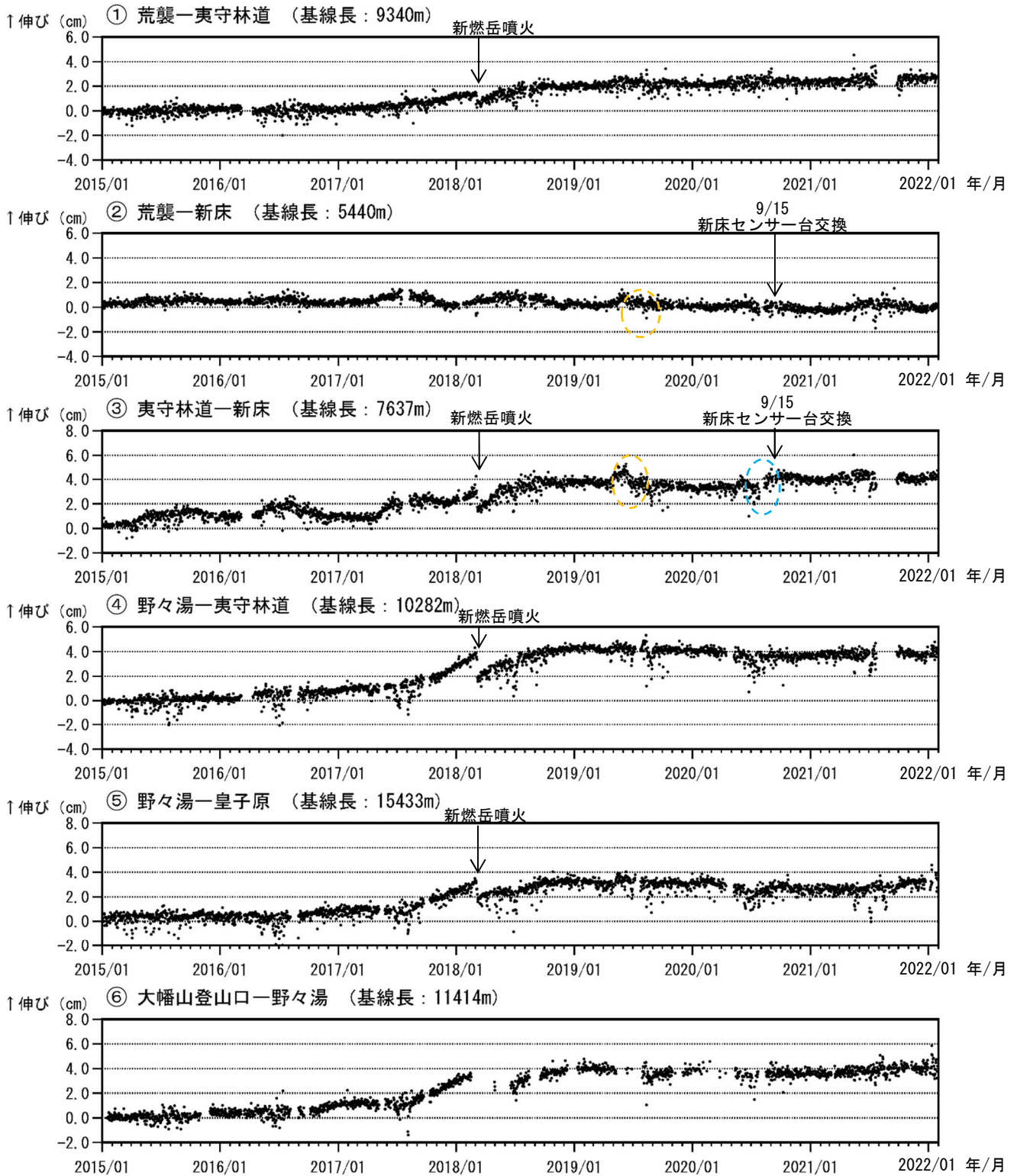
図6 霧島山（新燃岳） GNSS連続観測による基線長変化（2015年1月～2022年1月）
