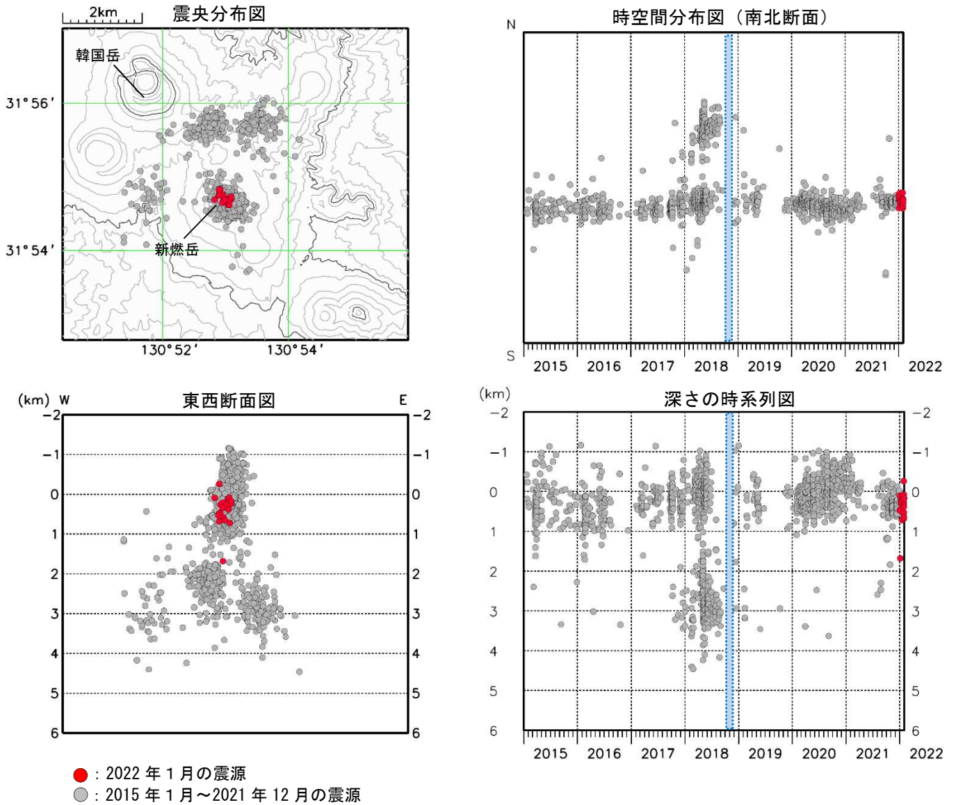
図5 霧島山（新燃岳） 震源分布図（2015年1月～2022年1月）
