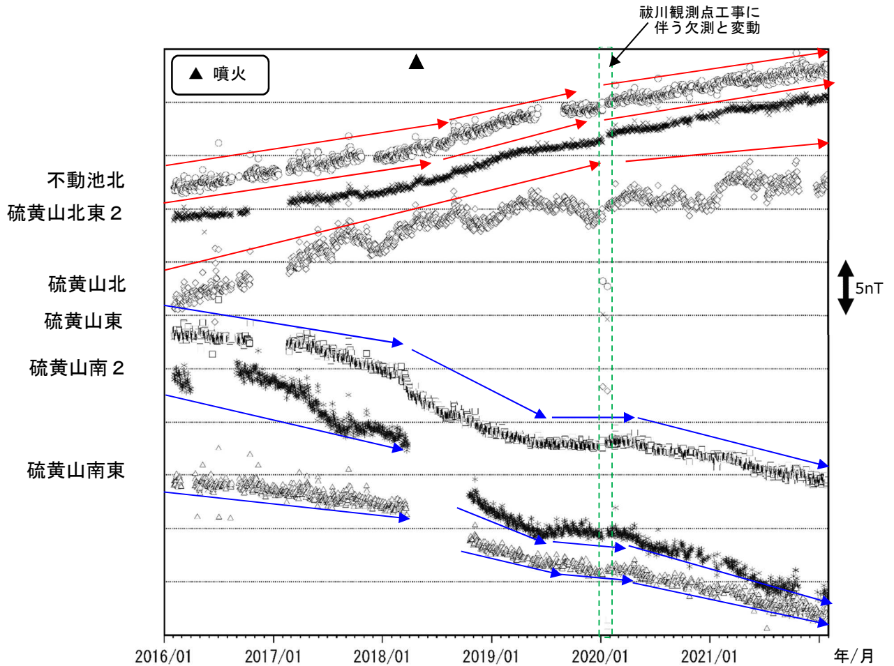
図 6-2 霧島山（えびの高原（硫黄山）周辺） 全磁力観測点で観測された全磁力変動（2016年1月～2022年1月）
