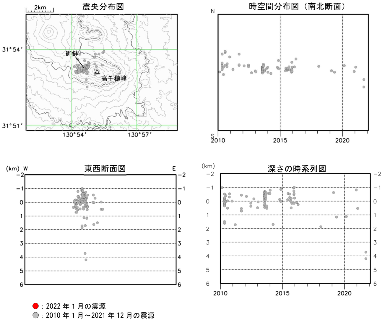
図3 霧島山（御鉢） 震源分布図（2010年1月～2022年1月）
