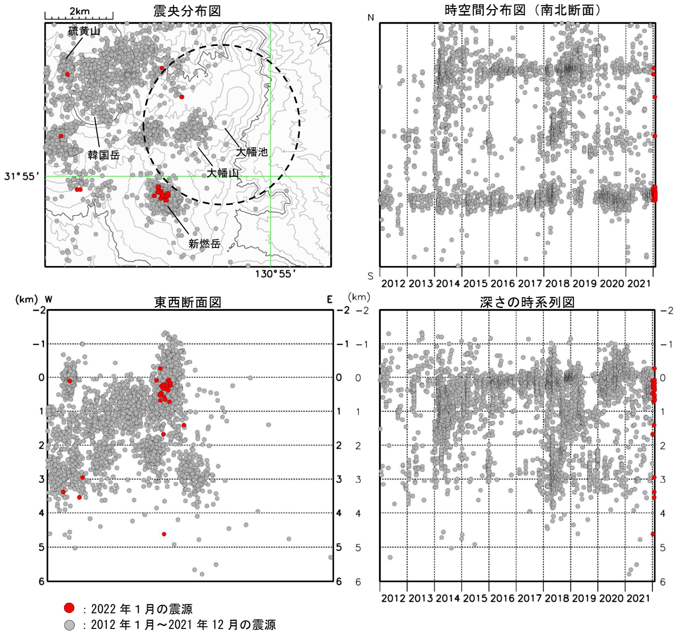
図3 霧島山（大幡池） 震源分布図（2012年1月～2022年1月）
