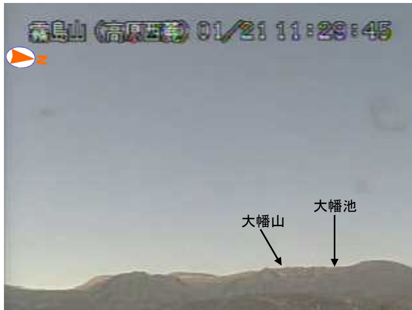
図1 霧島山（大幡池） 大幡池及び大幡山の状況（1月21日、高原西麓監視カメラ）
