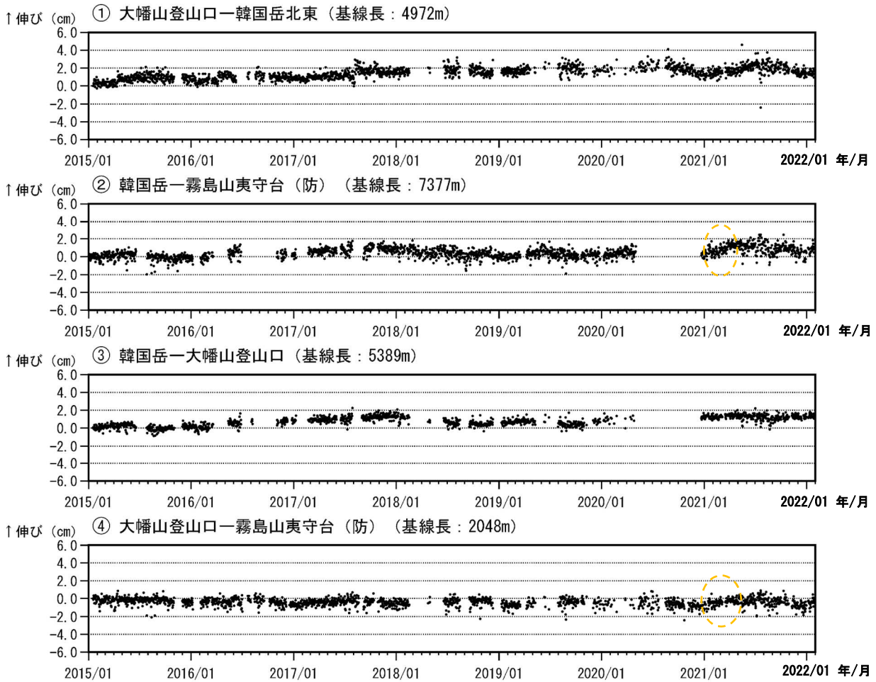
図4 霧島山（大幡池） GNSS 連続観測による基線長変化（2015年1月～2022年1月）
