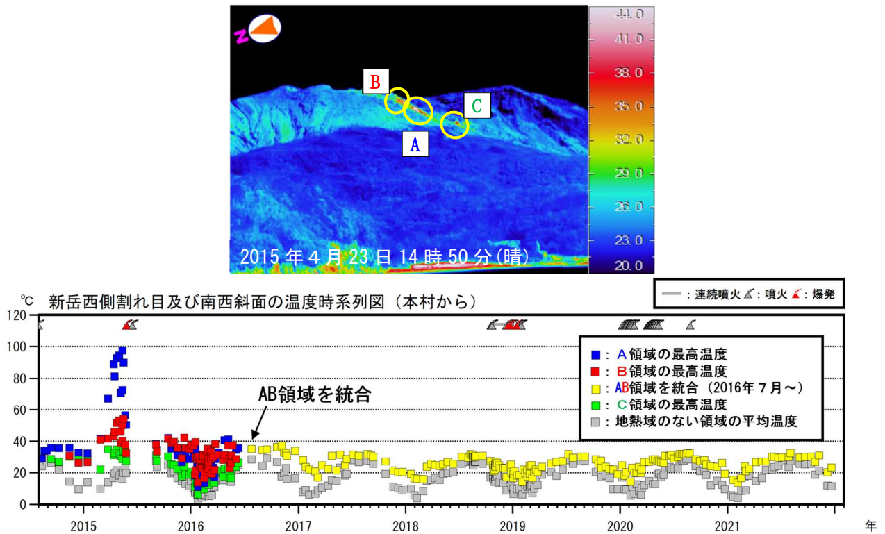
図3 口永良部島 新岳火口西側割れ目付近及び新岳南西側斜面の地熱域の温度時系列図 (2014年8月～2021年12月)
