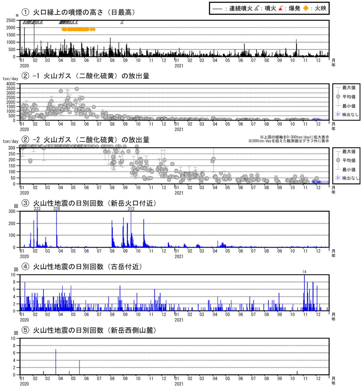
図6 口永良部島 最近の火山活動経過図（2020年1月～2021年12月）
