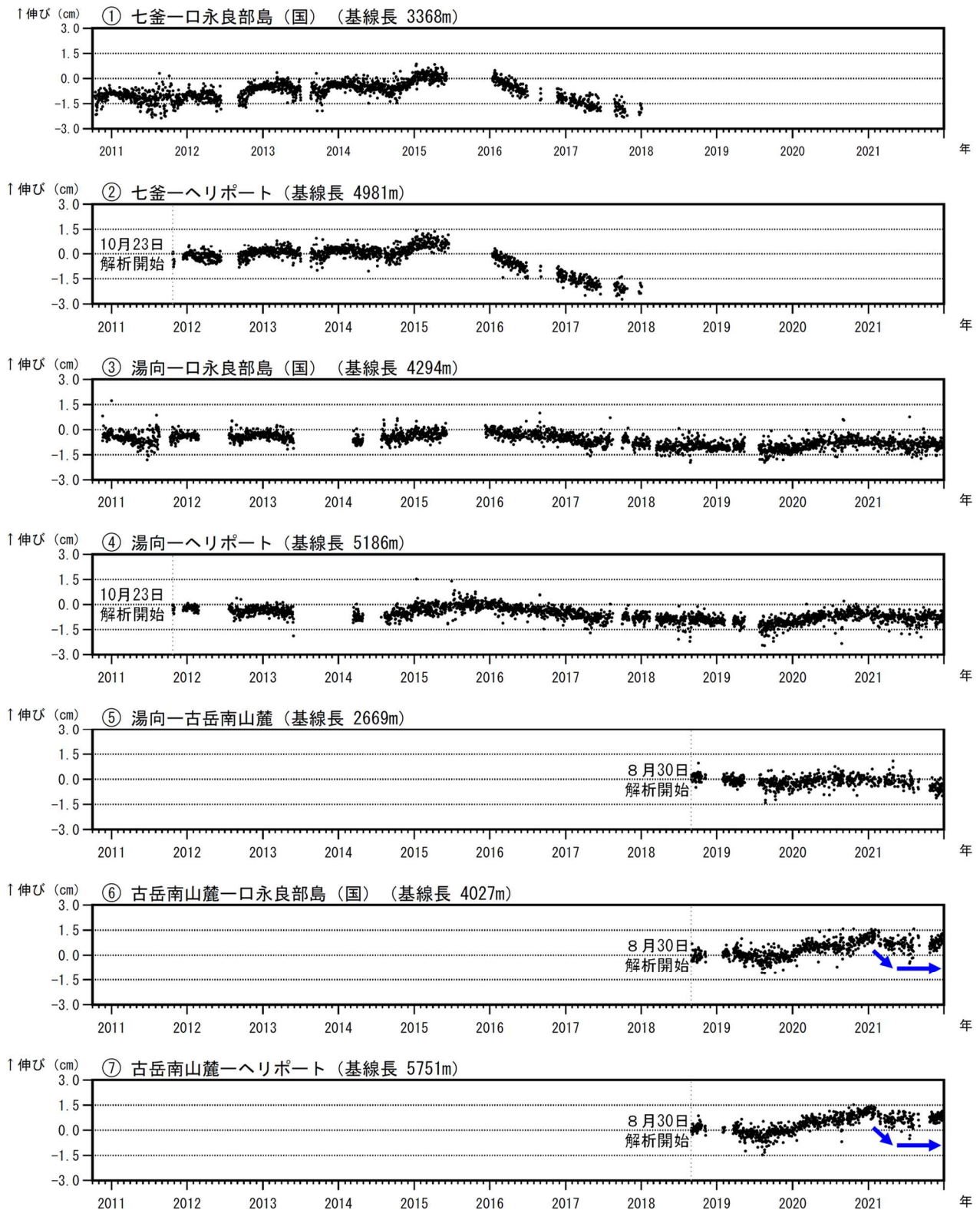
図8 口永良部島 GNSS 連続観測による基線長変化 (2010年10月~2021年12月)
