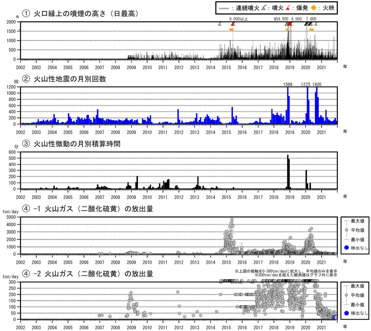
図5 口永良部島 火山活動経過図（2002年1月～2021年12月）
