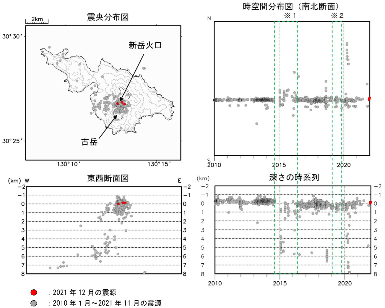
図7 口永良部島 震源分布図（2010年1月～2021年12月）
