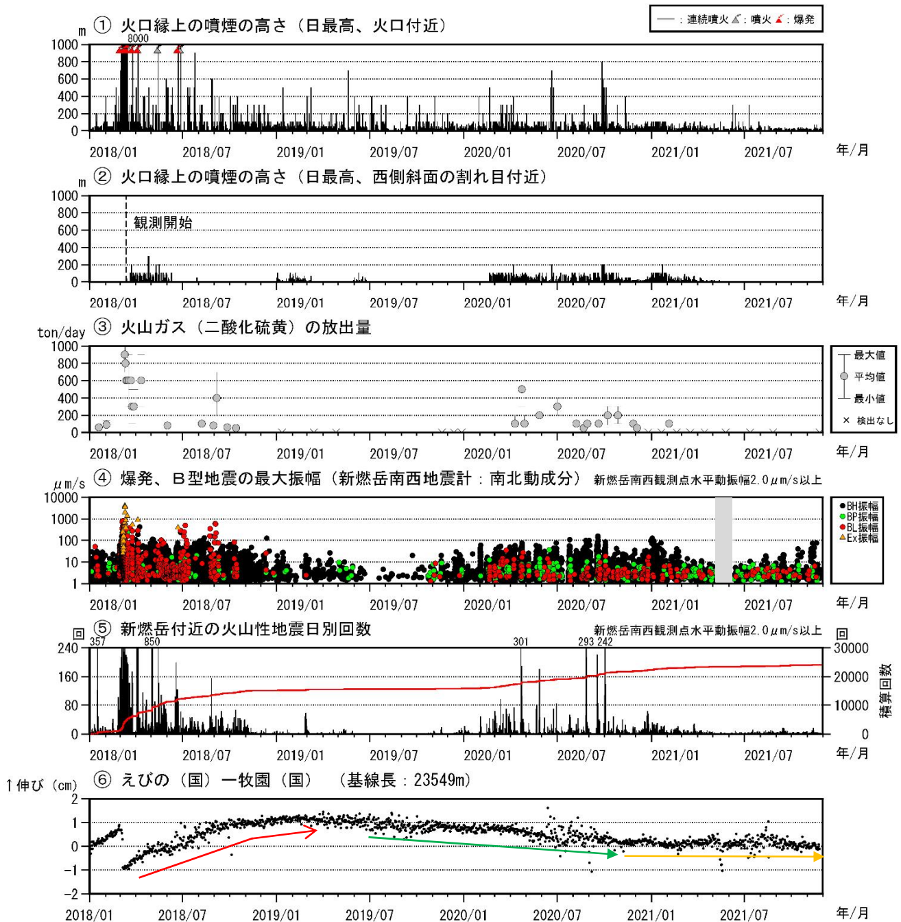
図2 霧島山（新燃岳） 火山活動経過図（2018年1月～2021年11月）
