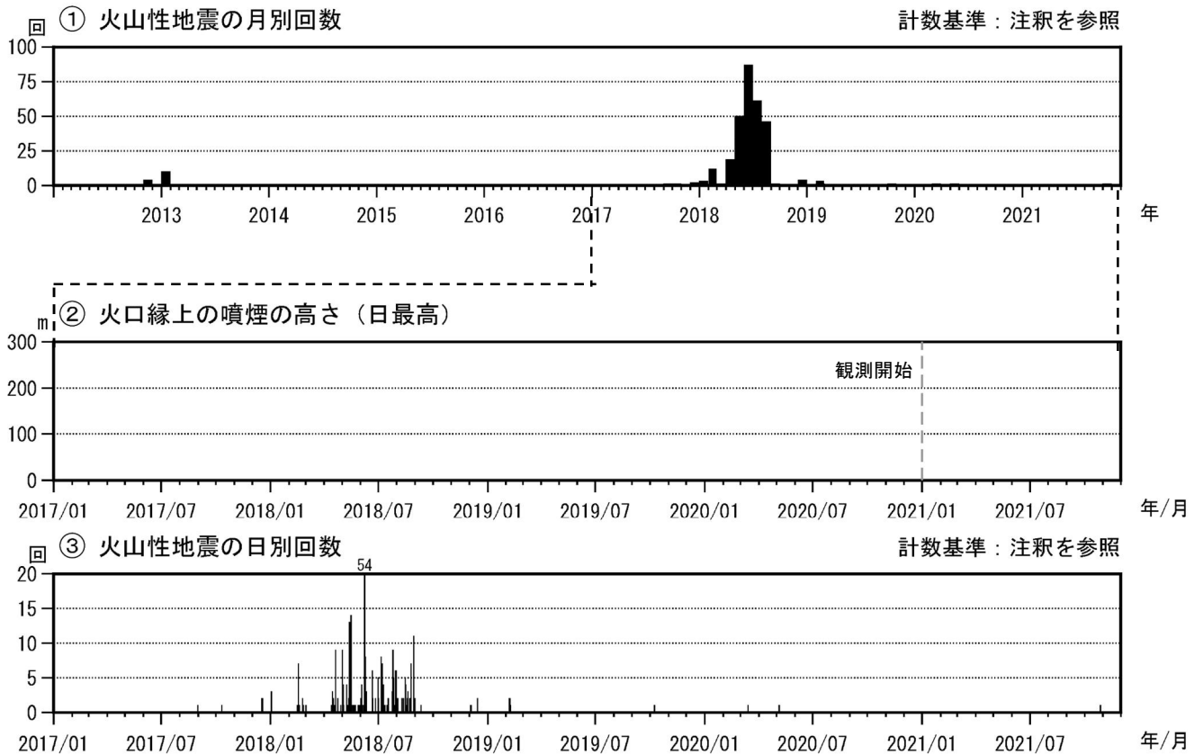
図2 霧島山（大幡池） 火山活動経過図（2012年1月～2021年11月）
