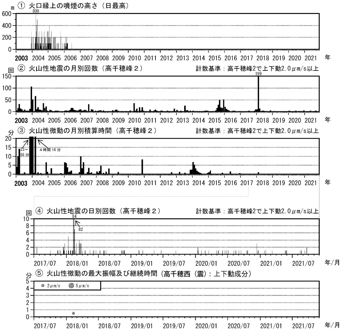
図2 霧島山（御鉢） 火山活動経過図（2003年1月～2021年11月）
