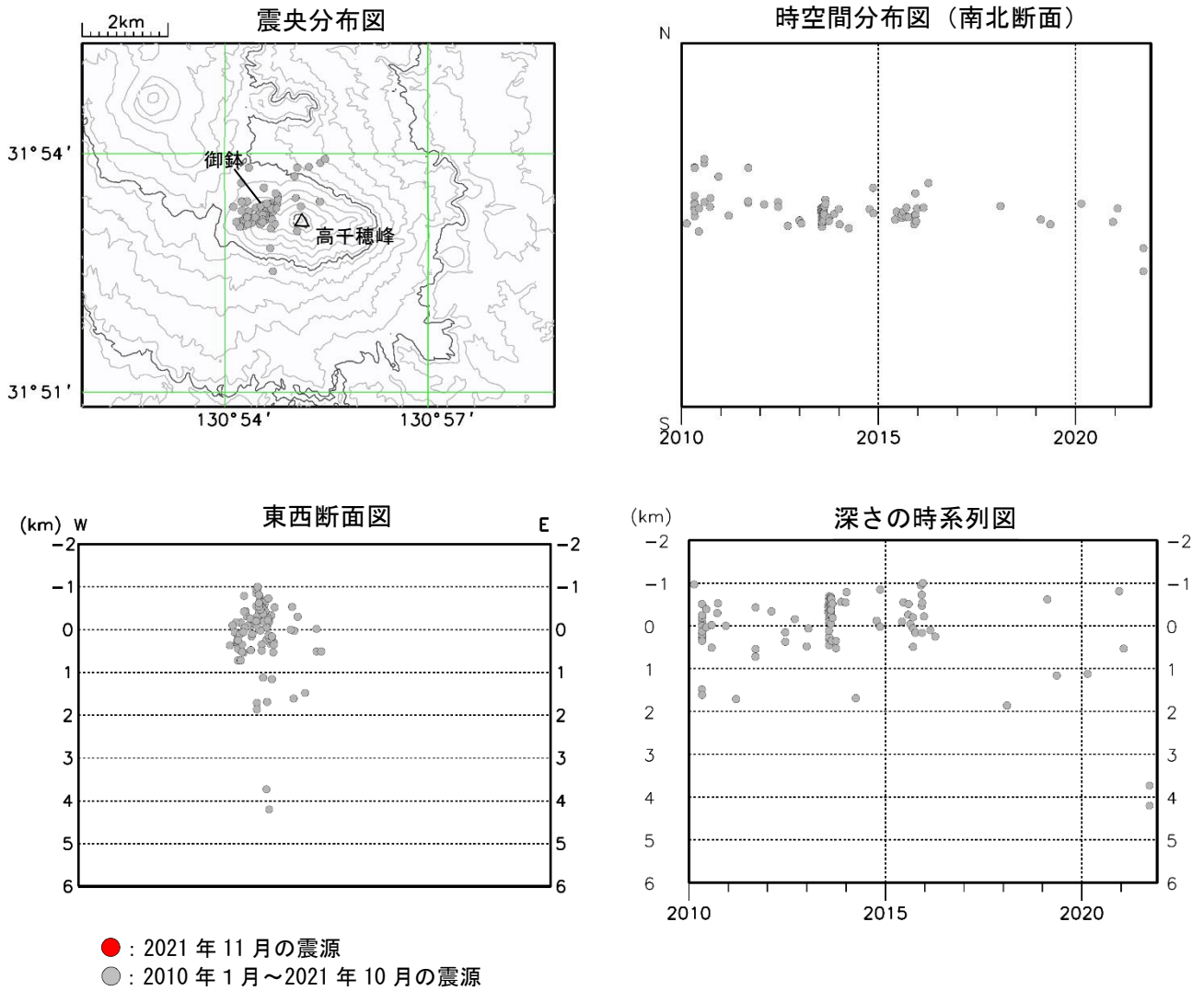
図3 霧島山（御鉢） 震源分布図（2010年1月～2021年11月）
