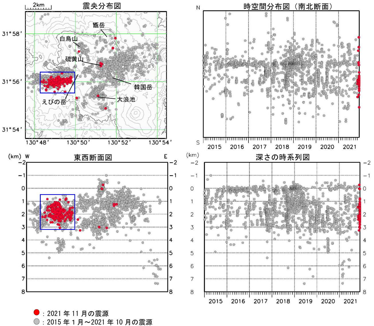
図2 霧島山（えびの高原（硫黄山）周辺） 震源分布図（2015年1月～2021年11月）
