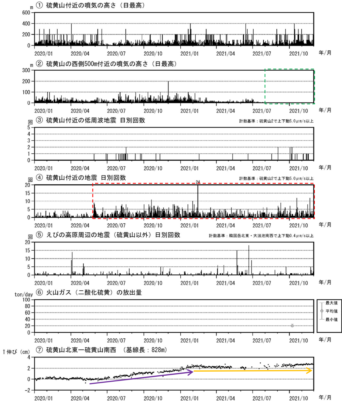
図3 霧島山（えびの高原（硫黄山）周辺）火山活動経過図（2020年1月～2021年11月）
