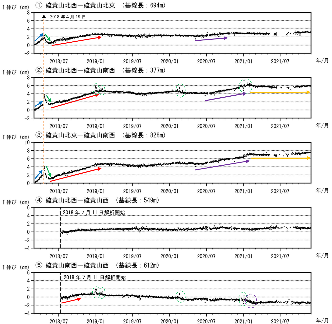
図4 霧島山（えびの高原（硫黄山）周辺） GNSS連続観測による基線長変化 （2018年3月～2021年11月）
