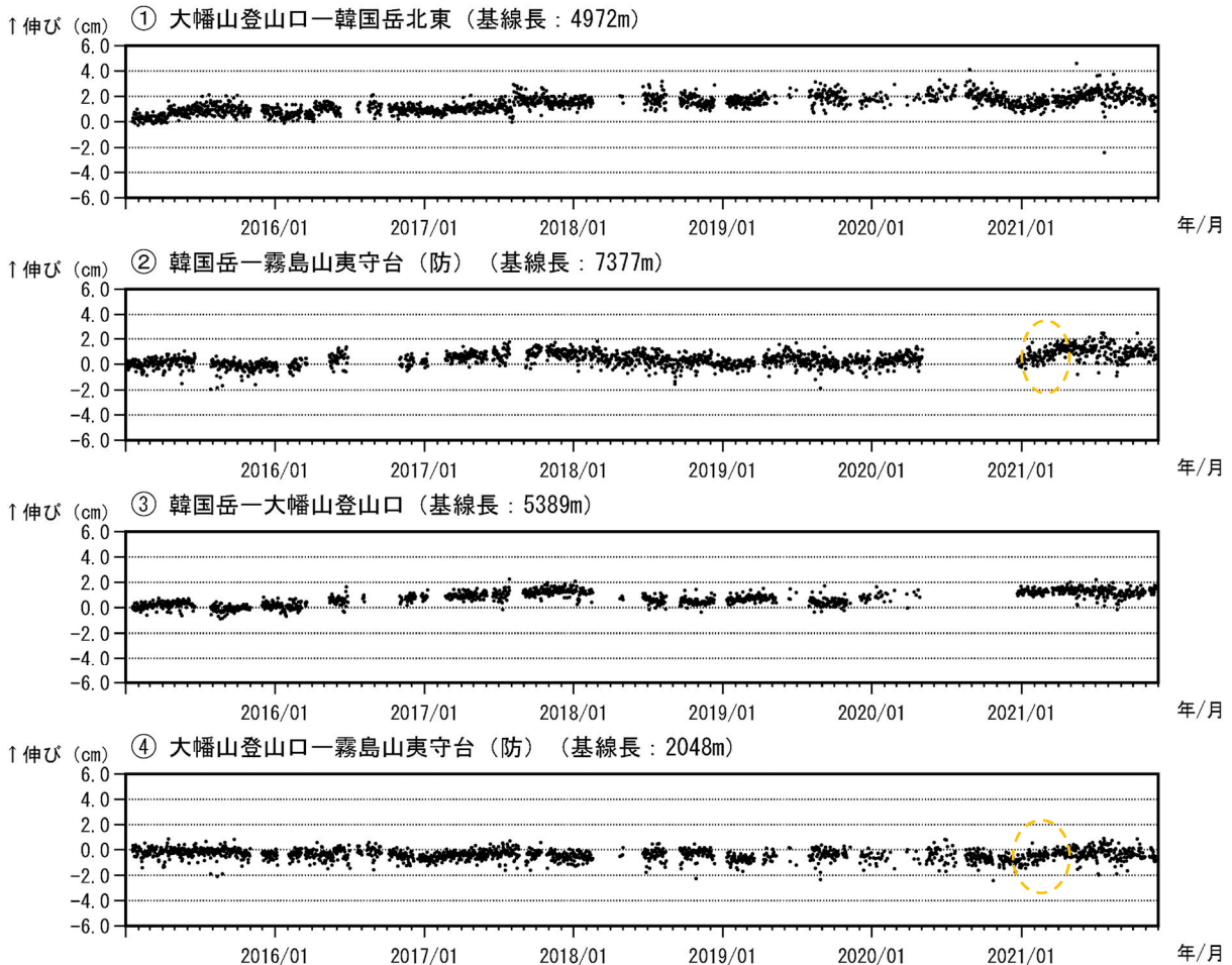
図4 霧島山 (大幡池) GNSS 連続観測による基線長変化 (2015年1月~2021年11月)
