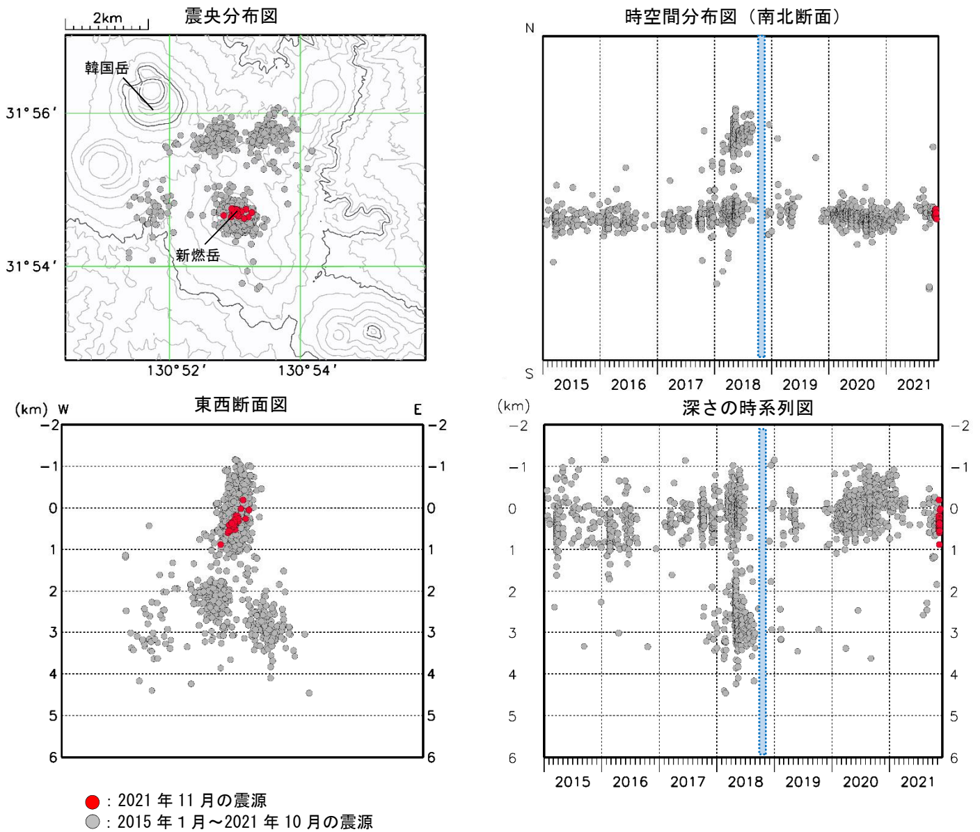
図3 霧島山（新燃岳） 震源分布図（2015年1月～2021年11月）
