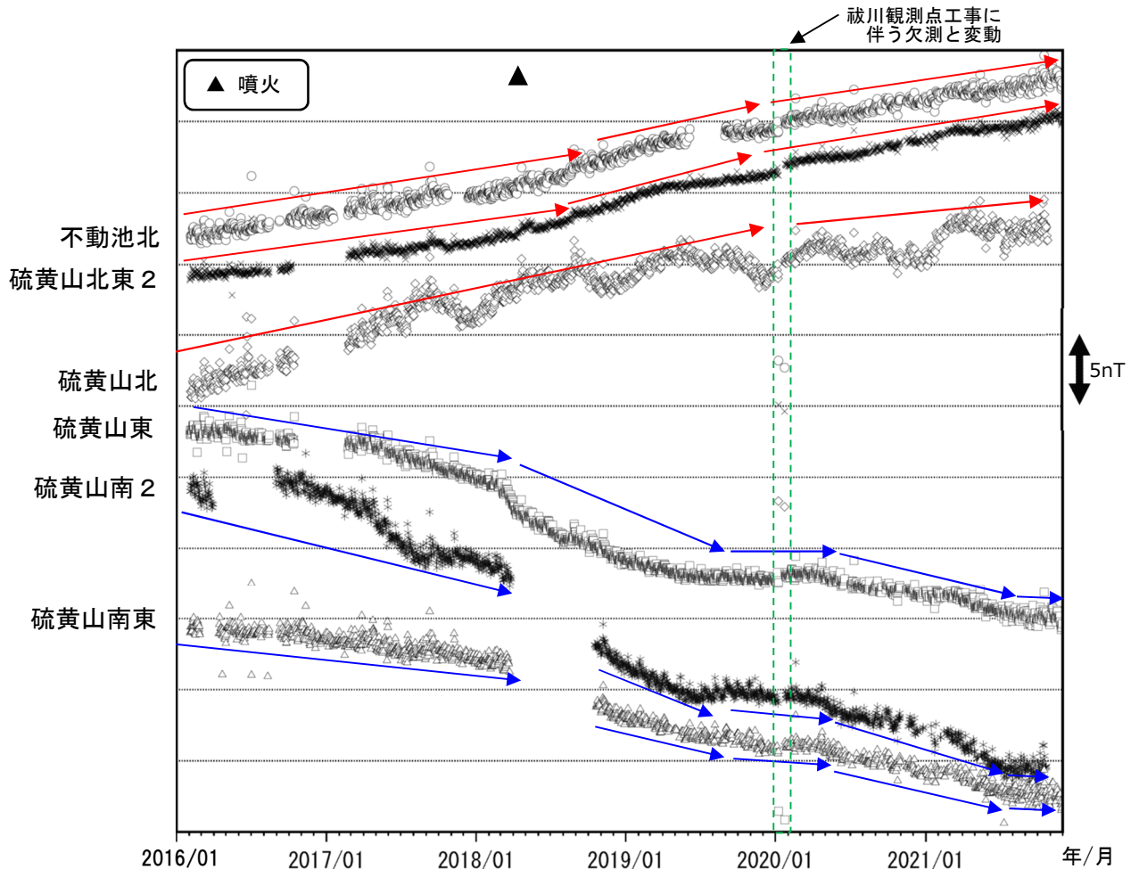
図 6-2 霧島山（えびの高原（硫黄山）周辺） 全磁力観測点で観測された全磁力変動（2016年1月～2021年11月）
