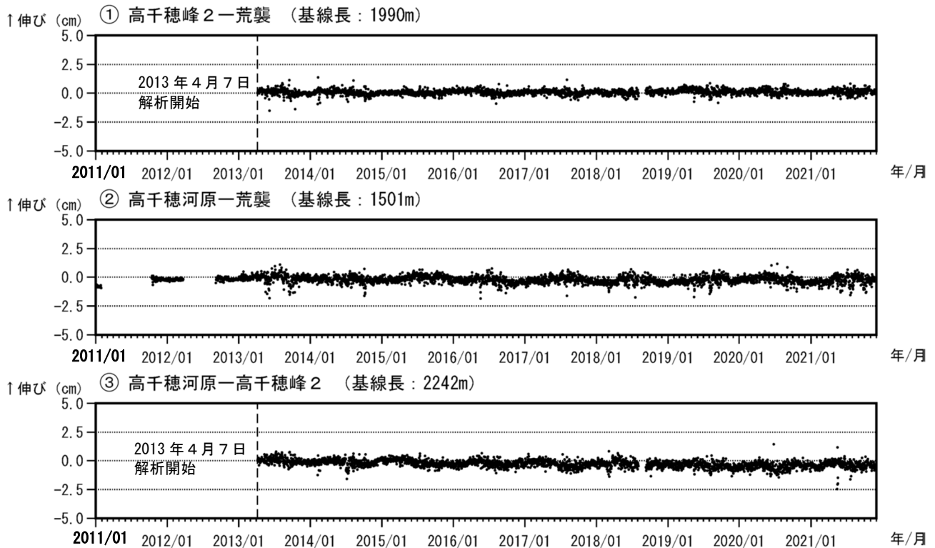
図4 霧島山（御鉢） GNSS 連続観測による基線長変化（2011年1月～2021年11月）
