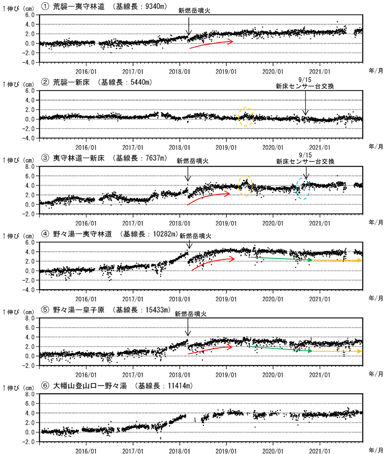
図4 霧島山（新燃岳） GNSS連続観測による基線長変化（2015年1月～2021年11月）
