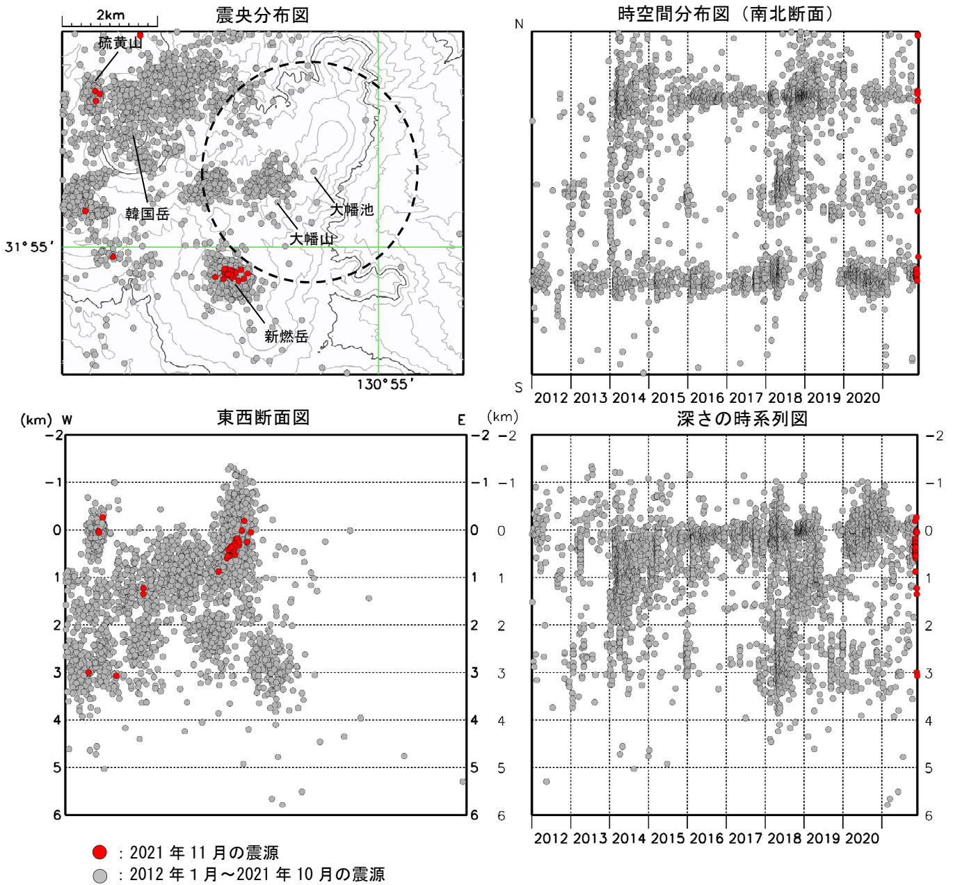
図3 霧島山（大幡池） 震源分布図（2012年1月～2021年11月）
