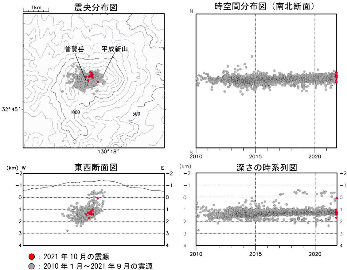
図 3-2 雲仙岳 震源分布図（普賢岳・平成新山付近の地震）（2010年1月～2021年10月）
