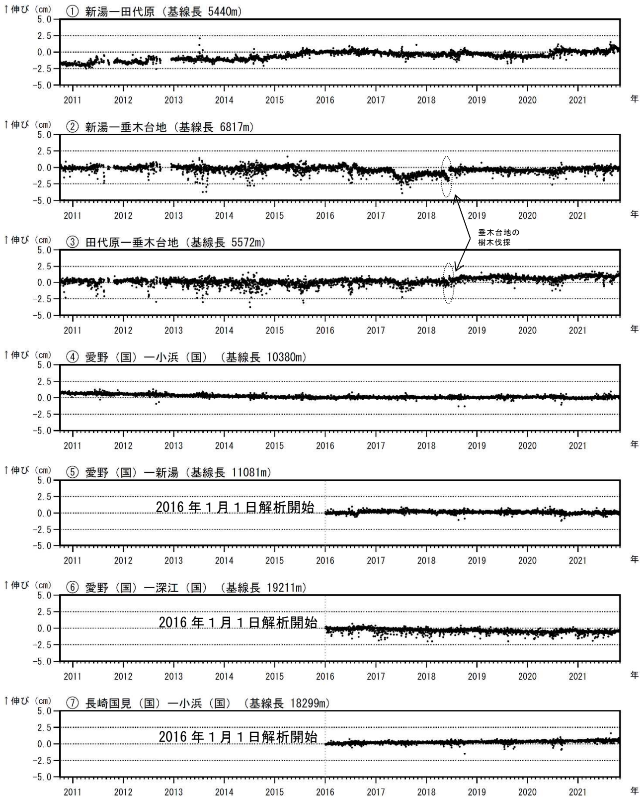
図4 雲仙岳 GNSS連続観測による基線長変化（2010年10月～2021年10月）
