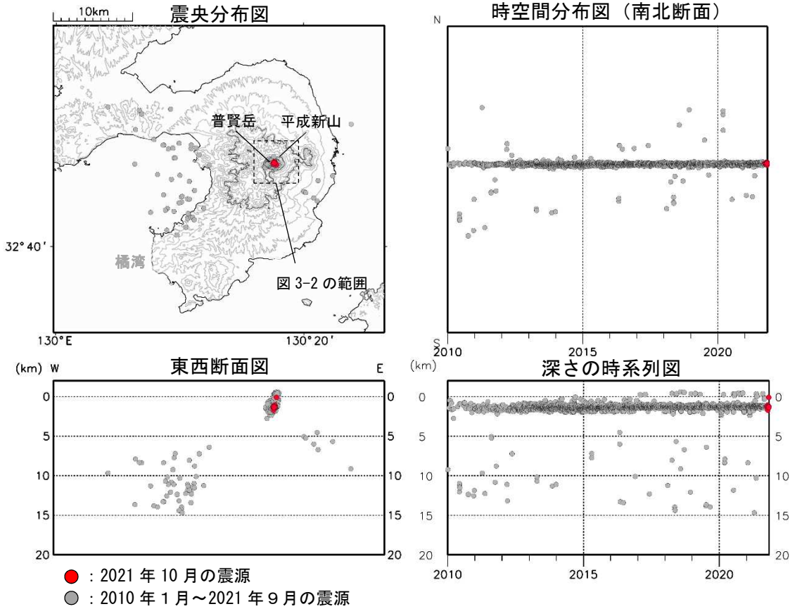
図 3-1 雲仙岳 震源分布図（広域）（2010年1月～2021年10月）
