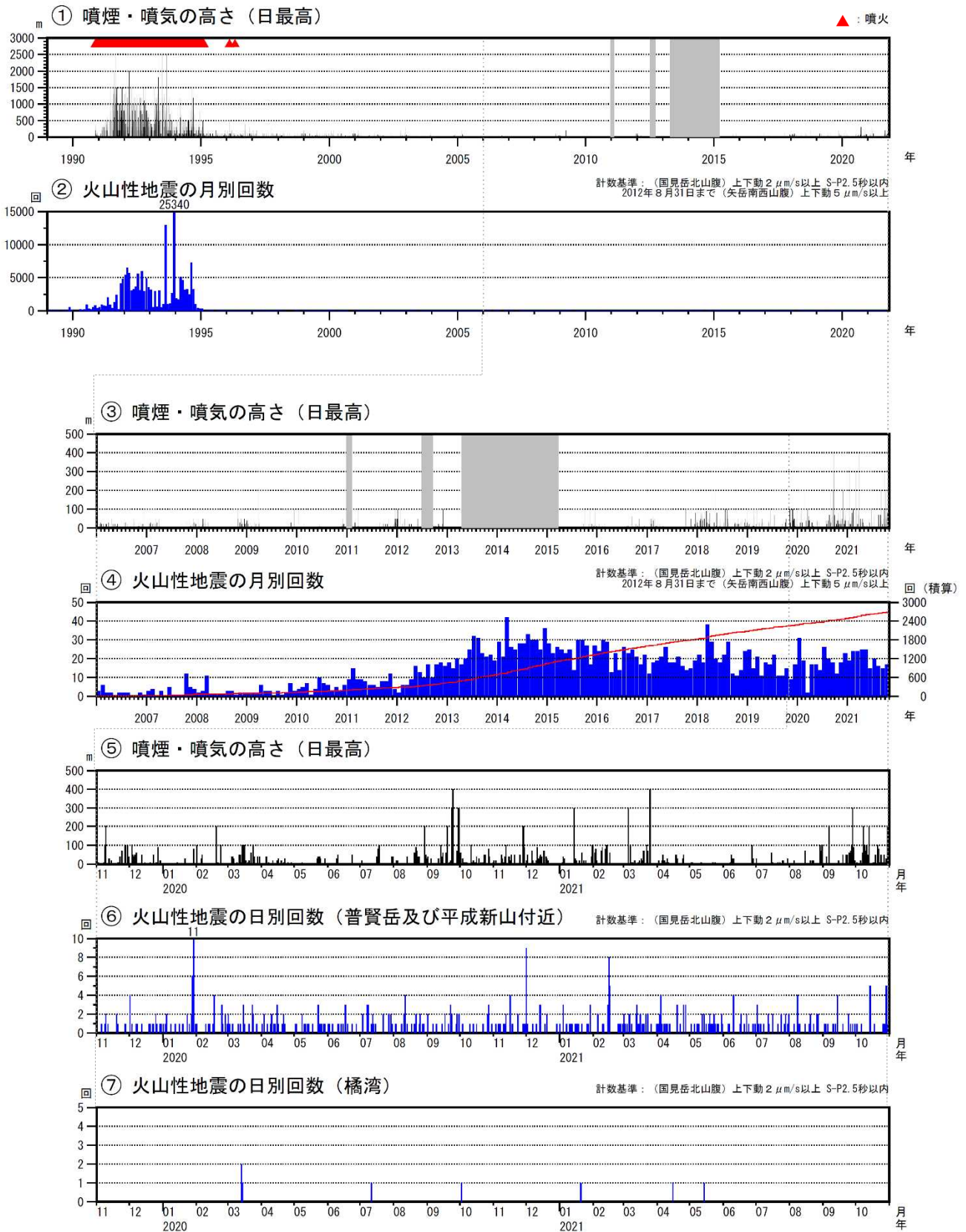
図2 雲仙岳 火山活動経過図（1989年1月～2021年10月）
