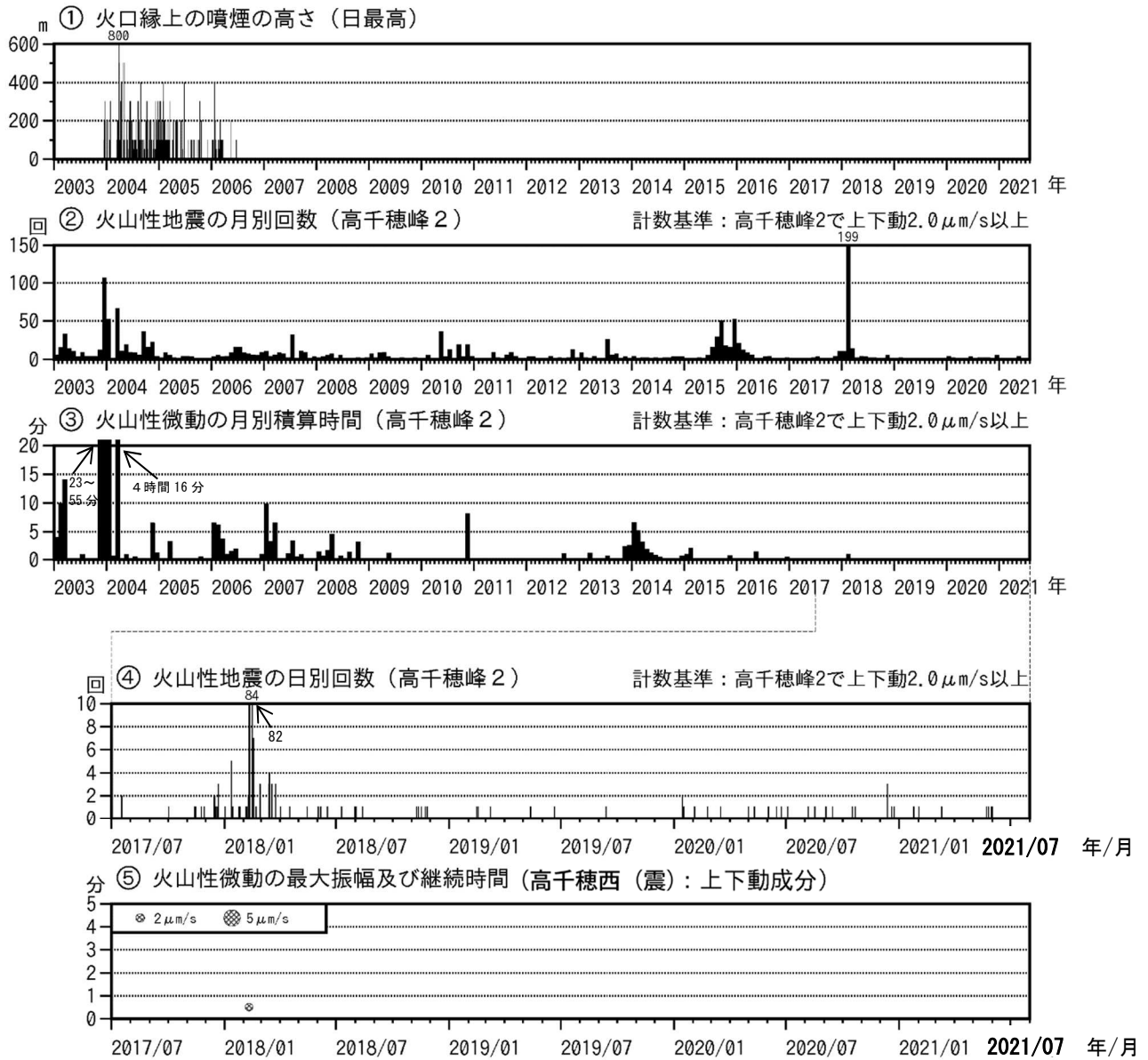
図2 霧島山（御鉢） 火山活動経過図（2003年1月～2021年7月）
