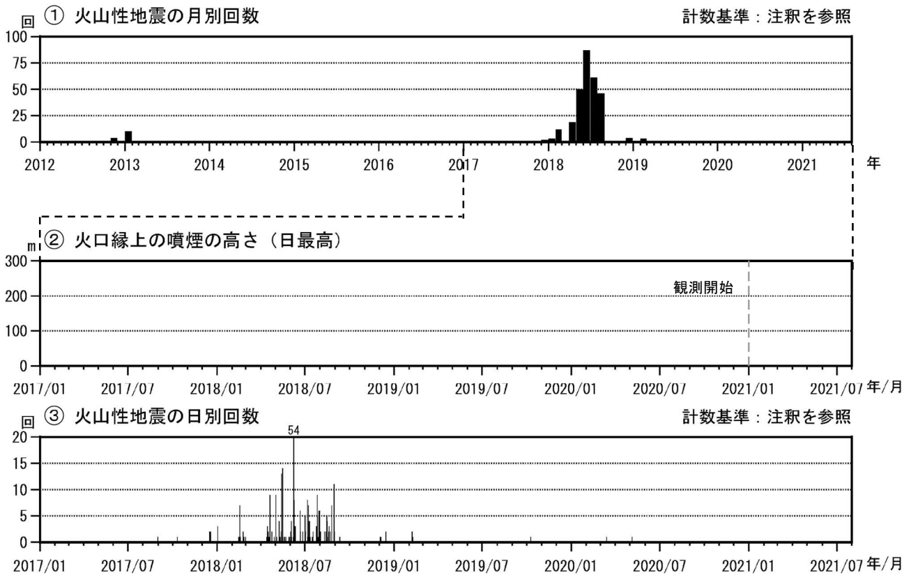
図2 霧島山（大幡池） 火山活動経過図（2012年1月～2021年7月）
