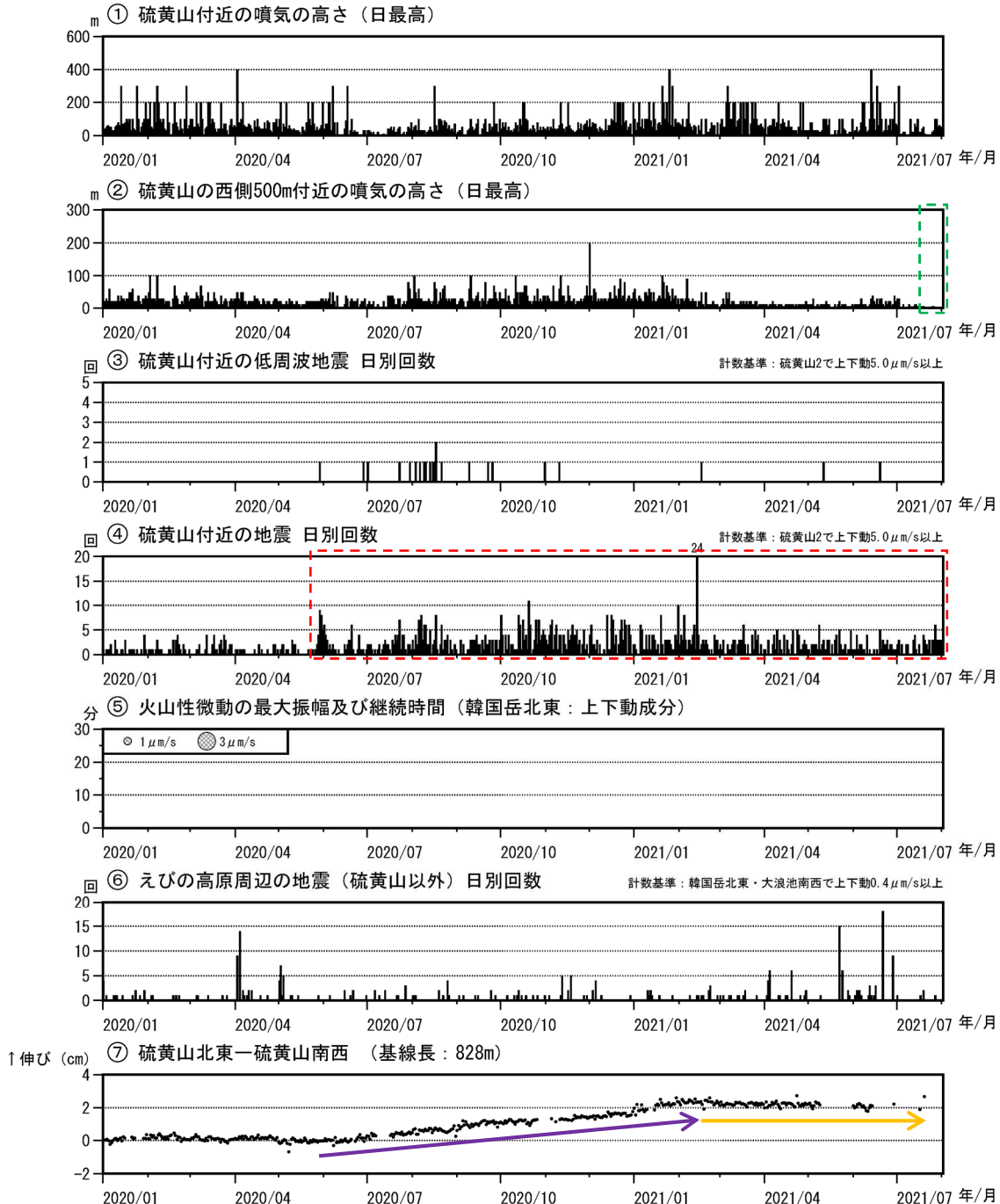
図3 霧島山（えびの高原（硫黄山）周辺）火山活動経過図（2020年1月～2021年7月）
