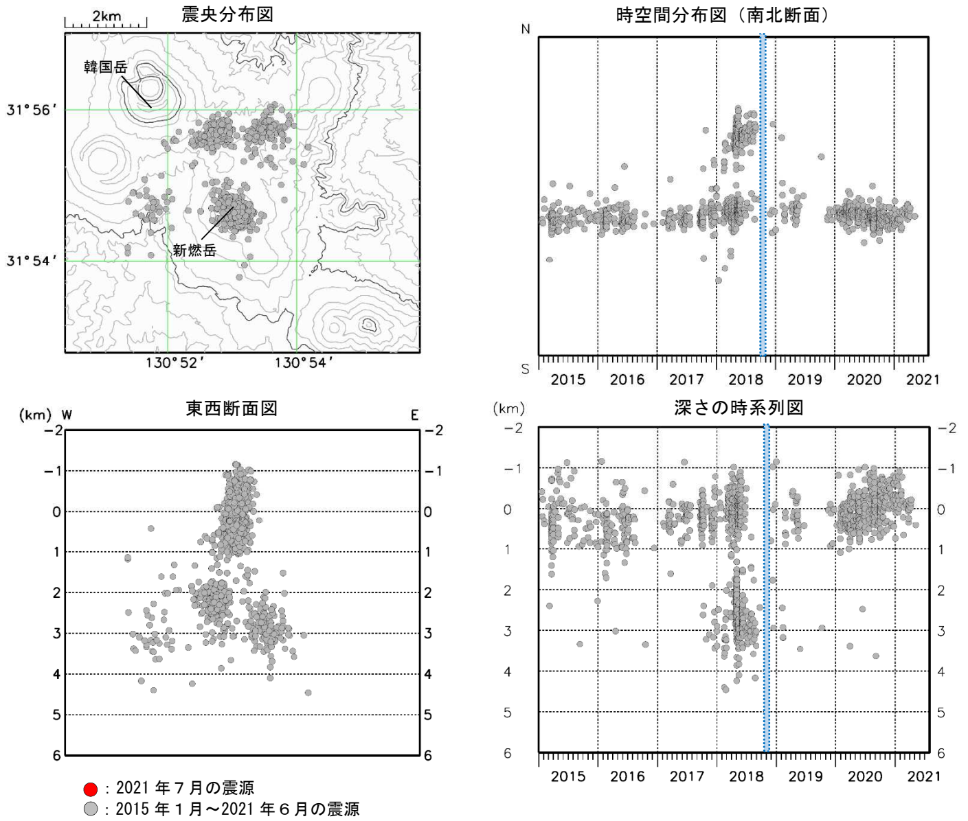
図3 霧島山（新燃岳） 震源分布図（2015年1月～2021年7月）
