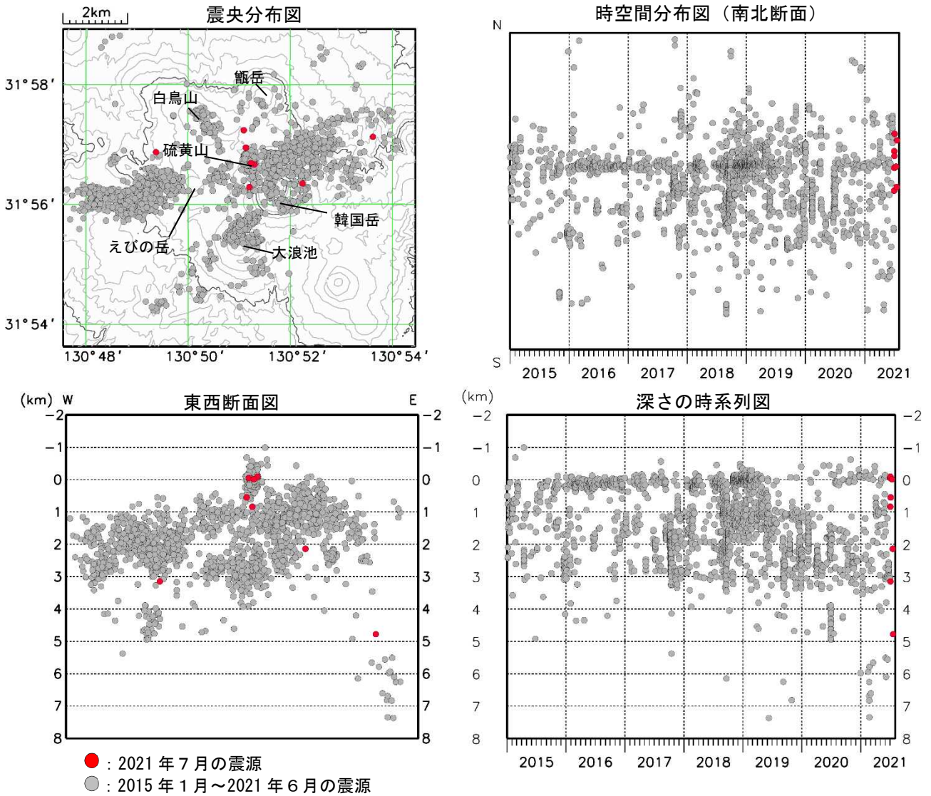
図2 霧島山（えびの高原（硫黄山）周辺） 震源分布図（2015年1月～2021年7月）
