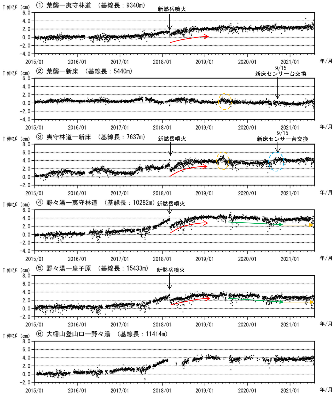
図4 霧島山（新燃岳） GNSS連続観測による基線長変化（2015年1月～2021年7月）
