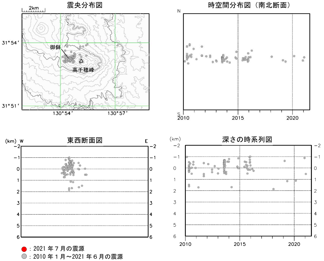
図3 霧島山（御鉢） 震源分布図（2010年1月～2021年7月）
