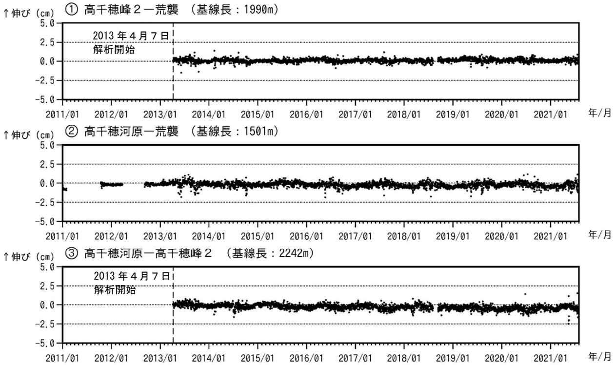
図4 霧島山（御鉢） GNSS 連続観測による基線長変化（2011年1月～2021年7月）
