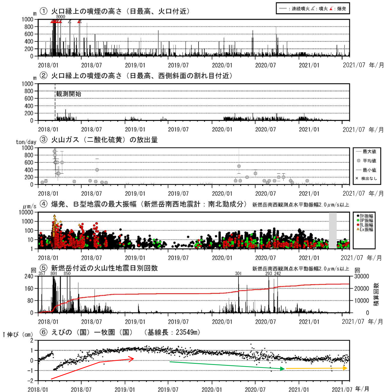
図2 霧島山（新燃岳） 火山活動経過図（2018年1月～2021年7月）
