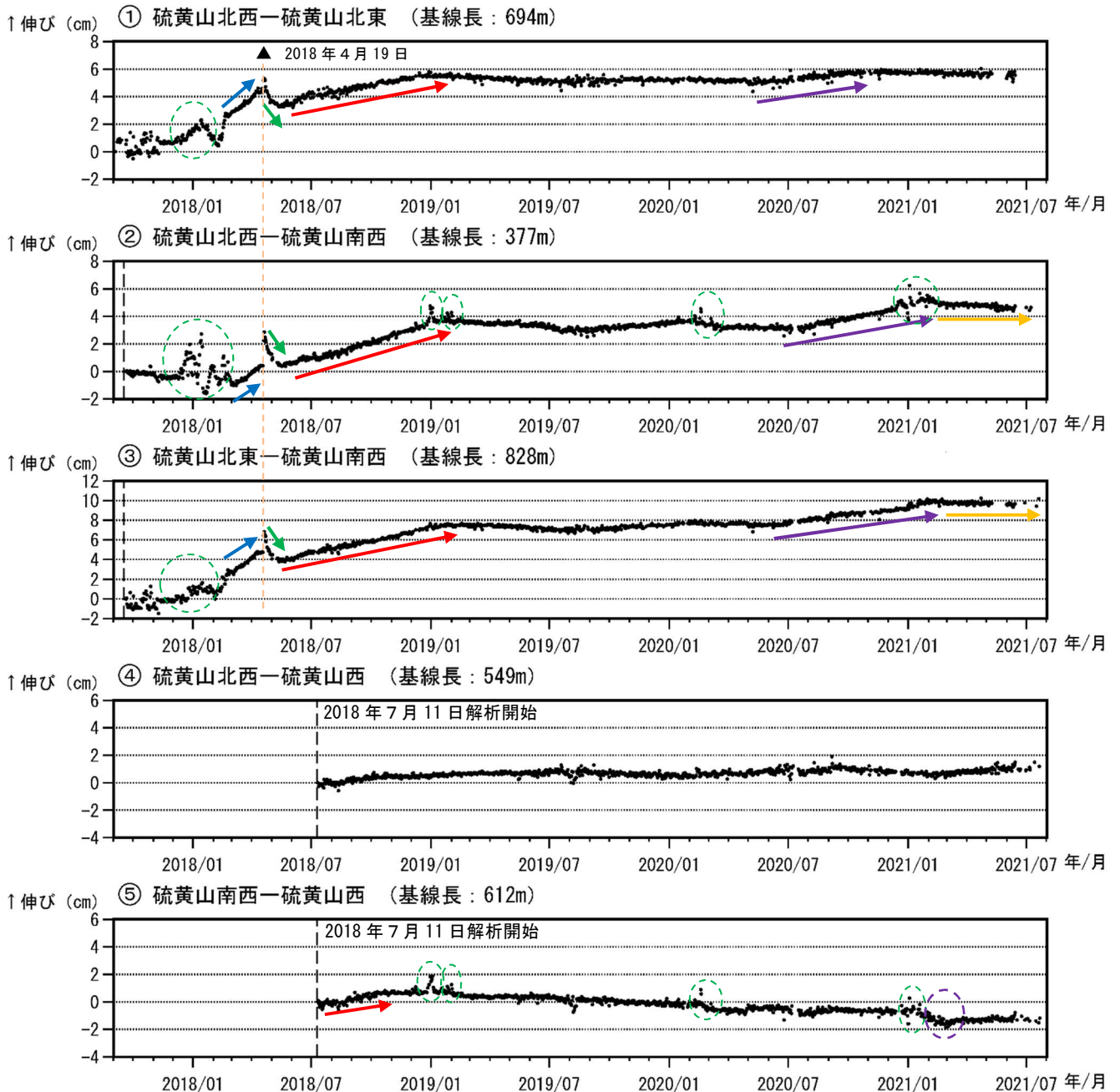
図4 霧島山（えびの高原（硫黄山）周辺） GNSS 連続観測による基線長変化 （2017年9月～2021年7月）
