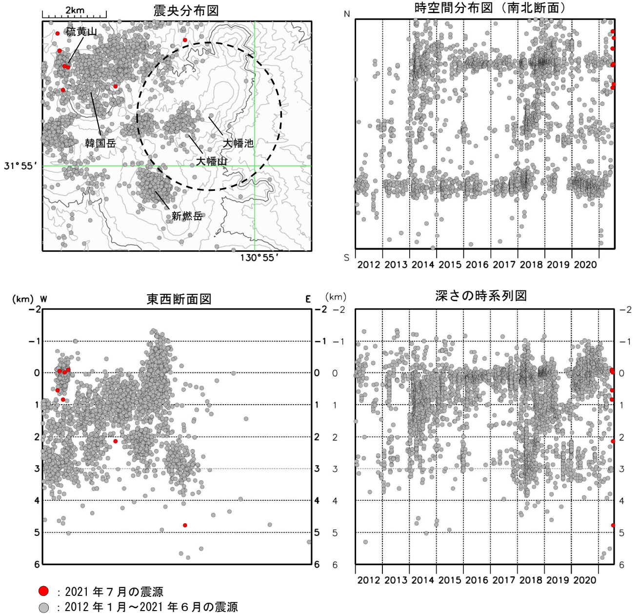
図3 霧島山（大幡池） 震源分布図（2012年1月～2021年7月）
