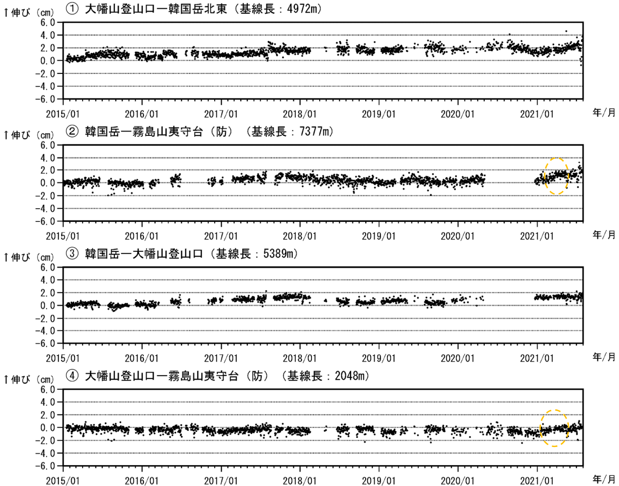
図4 霧島山（大幡池） GNSS 連続観測による基線長変化（2015年1月～2021年7月）
